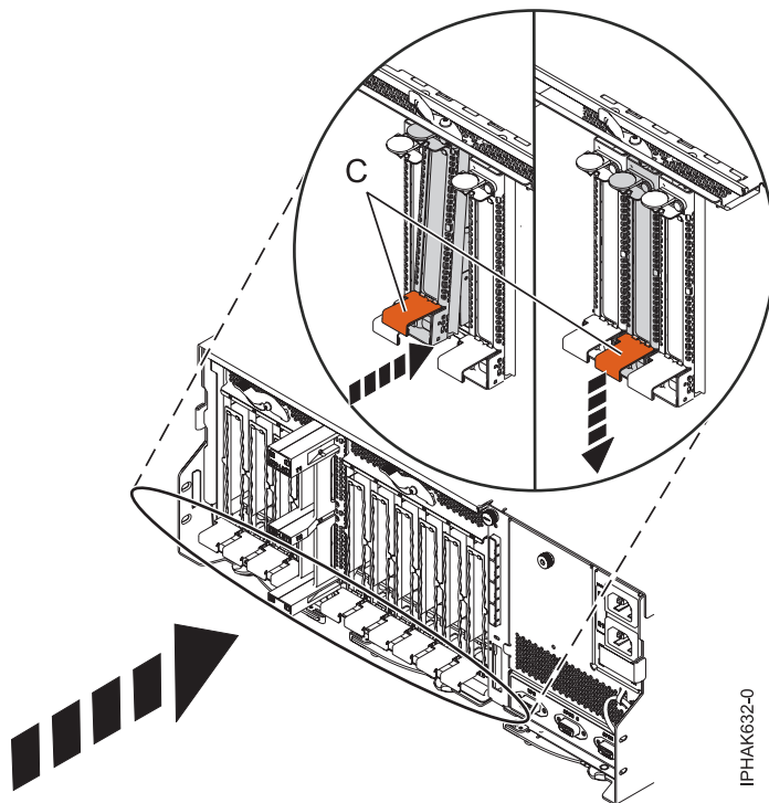
Figura 77. Instalación de la casete de adaptador PCI
