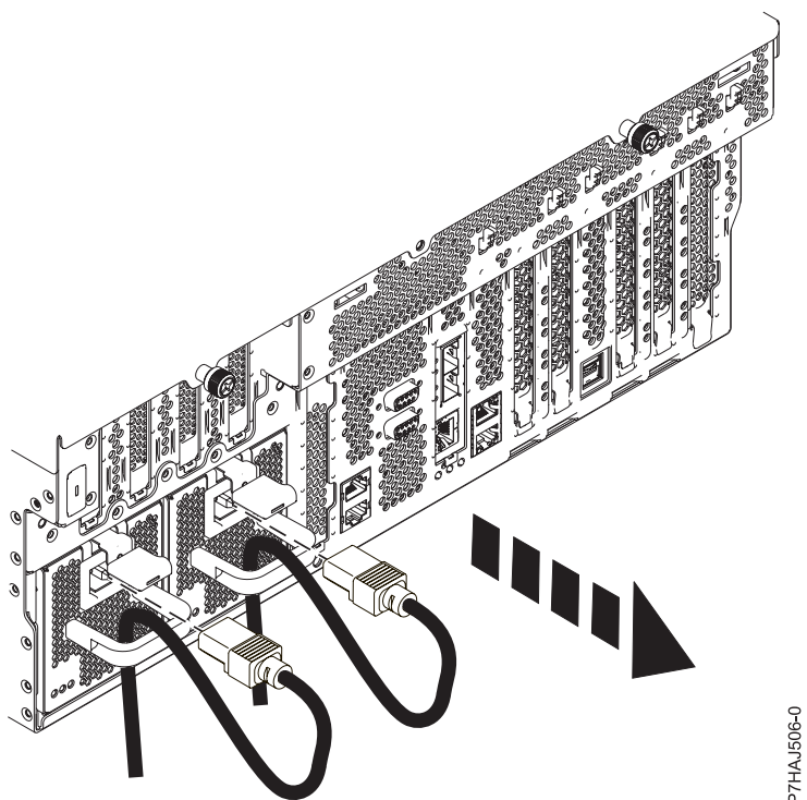
Figura 35. Desconexión de los cables de alimentación
