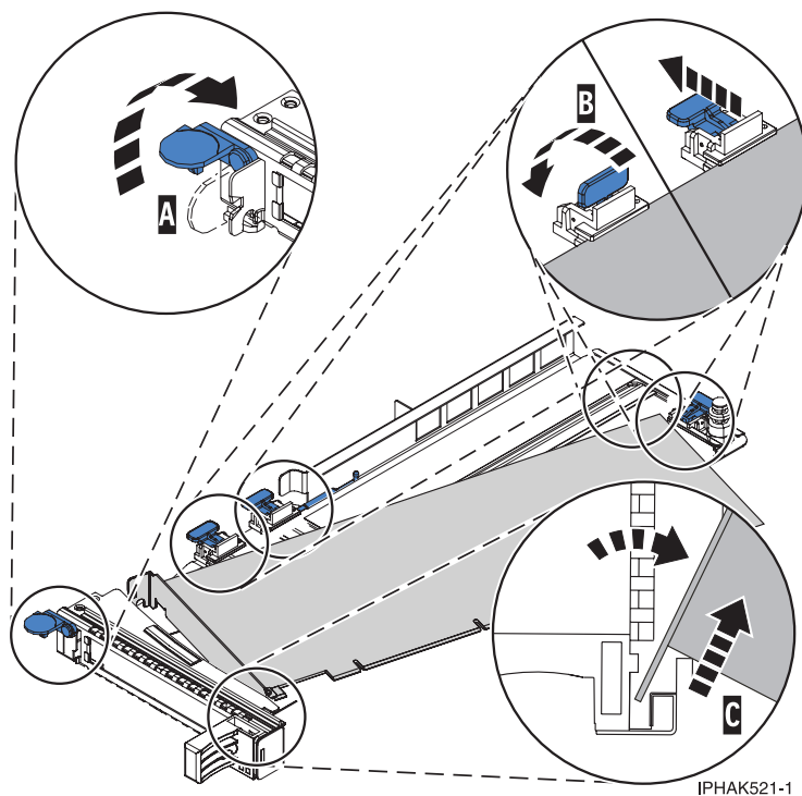
Figura 68. Adaptador que se ha quitado de la casete de adaptadores PCI
