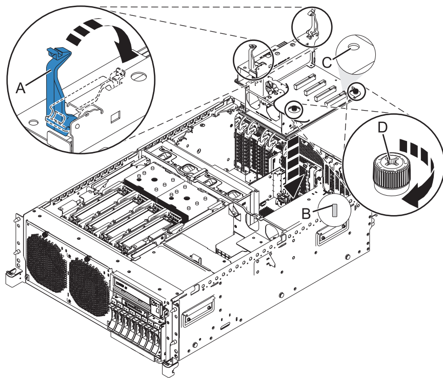
Figura 43. Sustitución de una tarjeta de expansión en una unidad del sistema montada en bastidor
