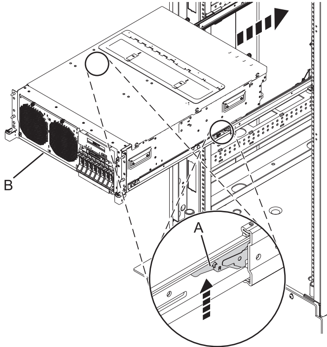
Figura 120. Colocación de la unidad del sistema en la posición operativa
