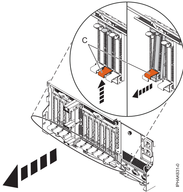
Figura 80. Extracción de una casete de adaptador PCI
