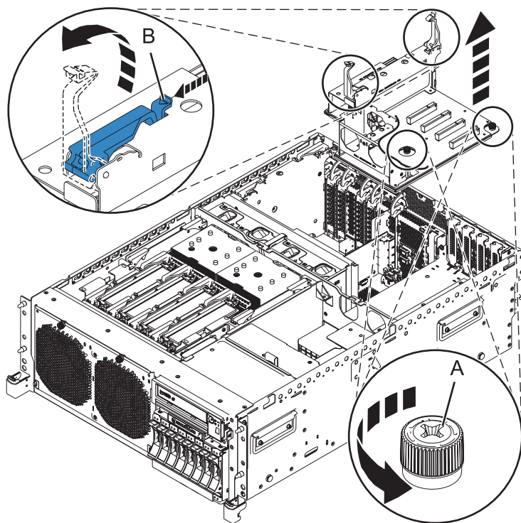
Figura 41. Extracción de una tarjeta de expansión de en una unidad del sistema montada en bastidor
