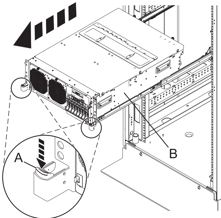
Figura 119. Fijación de la unidad del sistema en posición de servicio
