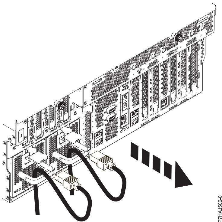
Figura 16. Desconexión de los cables de alimentación
