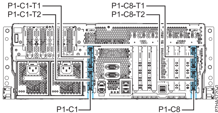
Figura 37. Vista posterior que muestra las ranuras P1-C1 y P1-C8
