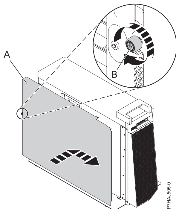
Figura 117. Instalación de la cubierta de acceso de servicio externa
