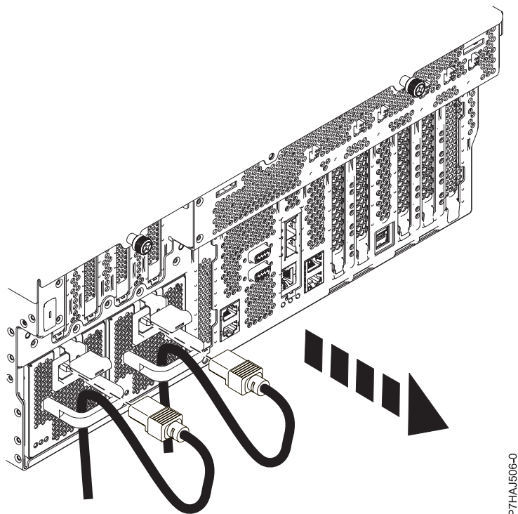
Figura 1. Desconexión de los cables de alimentación
