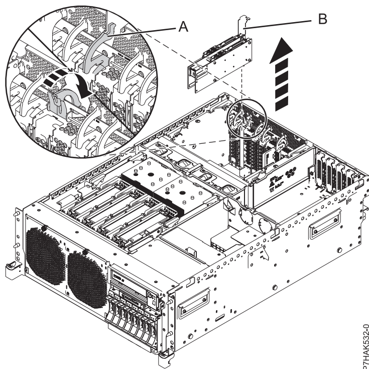
Figura 22. Extracción de un adaptador RAID PCIe y SAS SSD de una unidad del sistema montada en bastidor
