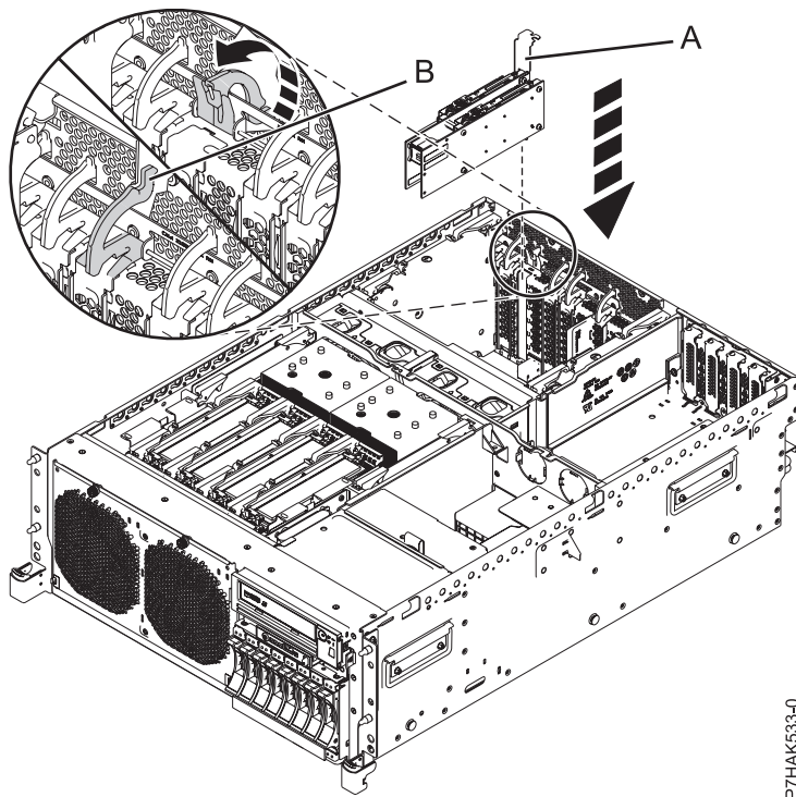
Figura 27. Sustitución de un adaptador RAID PCIe y SAS SSD en una unidad del sistema montada en bastidor
