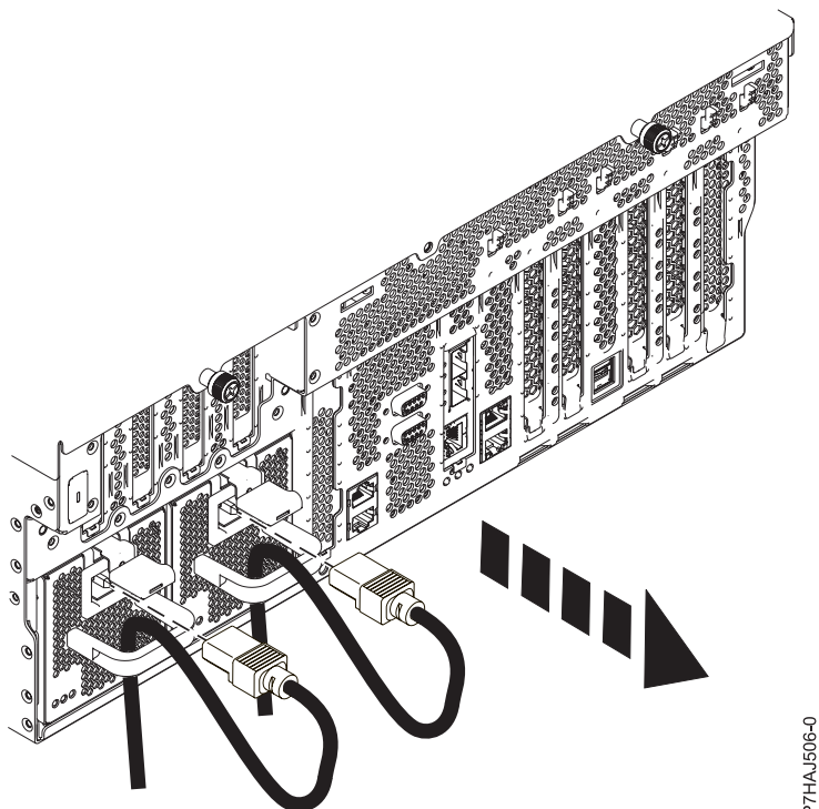
Figura 21. Desconexión de los cables de alimentación
