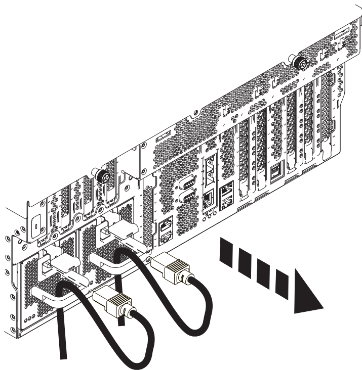
Figura 11. Desconexión de los cables de alimentación
