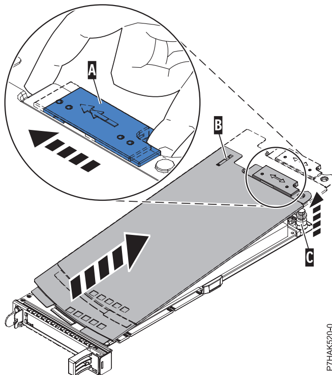
Figura 81. Se ha quitado la cubierta de la casete del adaptador PCI
