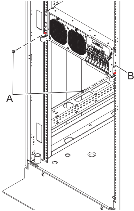
Figura 121. Colocación de la unidad del sistema en la posición operativa
