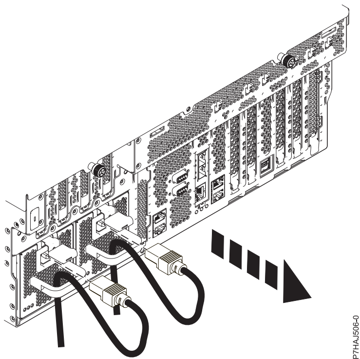
Figura 122. Extracción de los cables de alimentación para un sistema montado en bastidor
