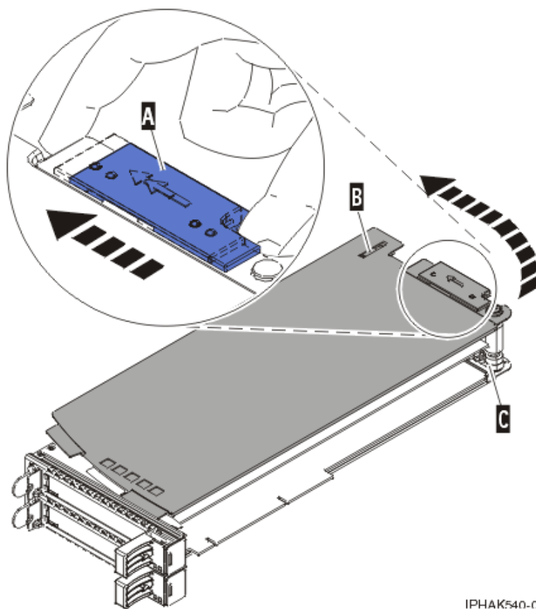
Figura 76. Cubierta que se ha sustituido de la casete de adaptador PCI
