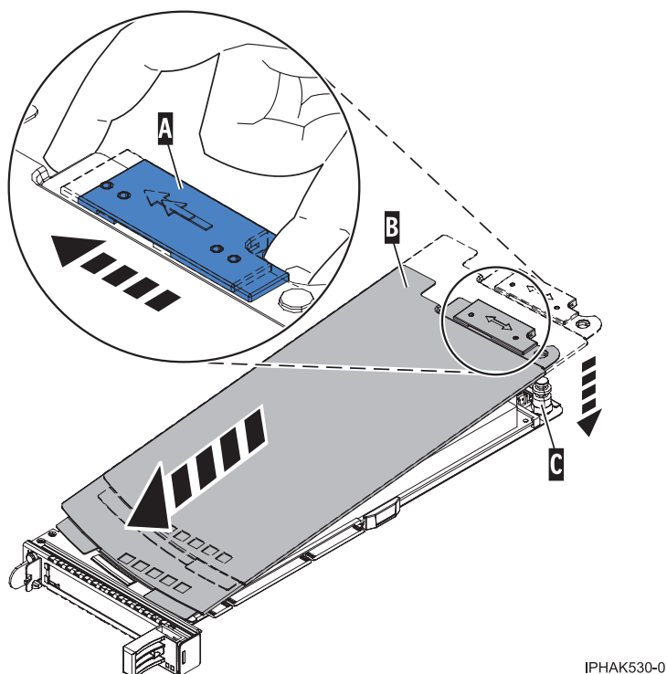
Figura 83. Cubierta que se ha sustituido de la casete de adaptador PCI
