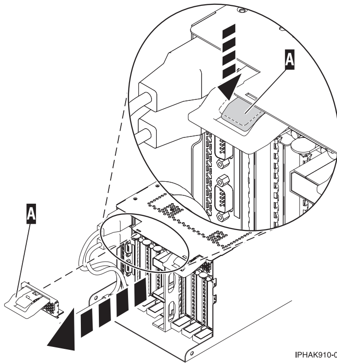
Figura 51. Quite el protector de EMC
