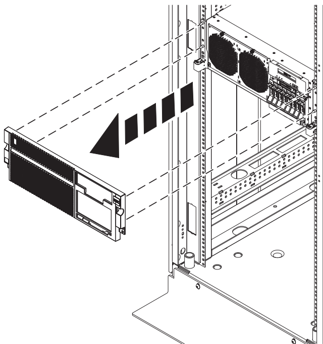
Figura 107. Extracción de la cubierta frontal
