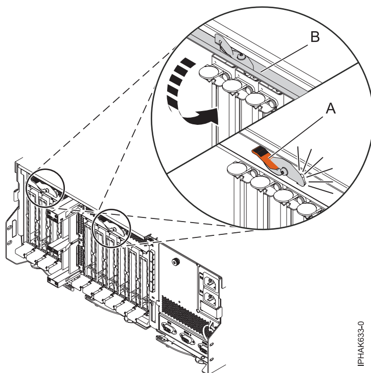
Figura 78. Cierre de la puerta de acceso
