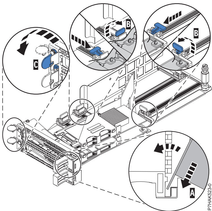
Figura 99. Sustitución de un adaptador RAID PCIe y SAS SSD en la casete del adaptador PCI
