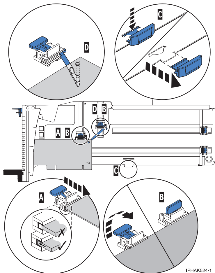
Figura 90. Adaptador pequeño en la casete de adaptador PCI con los soportes y el brazo de enganche en su sitio
