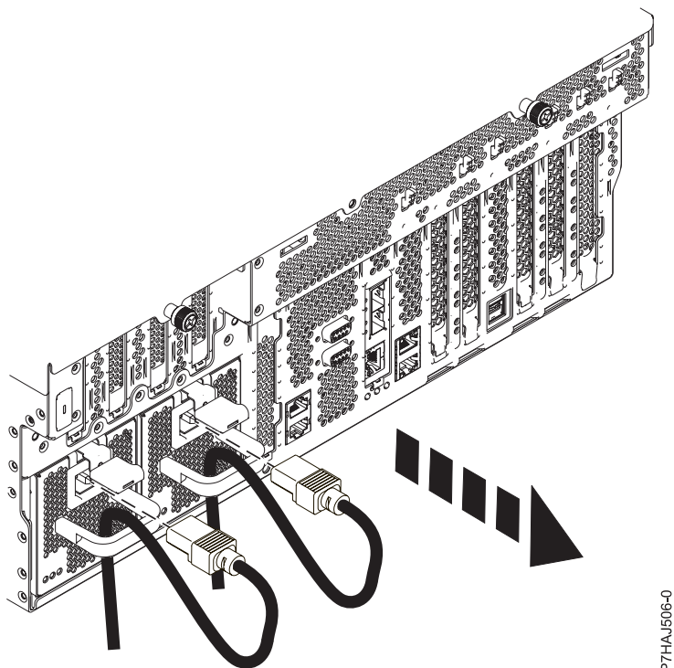
Figura 26. Desconexión de los cables de alimentación
