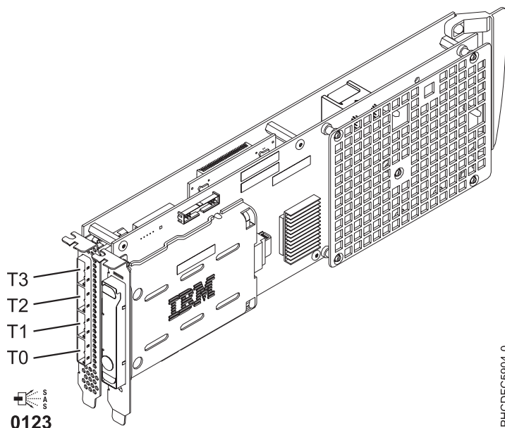
Figura 105. Adaptador PCI-X DDR con memoria caché de 1,5 GB SAS RAID
