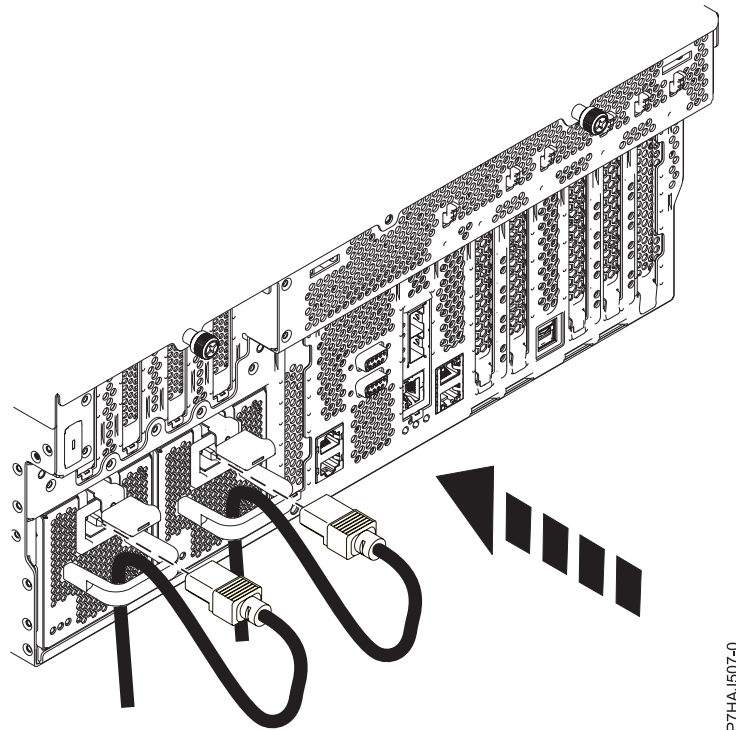
Figura 124. Conexión de los cables de alimentación
