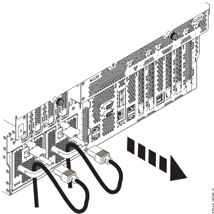
Figura 6. Desconexión de los cables de alimentación
