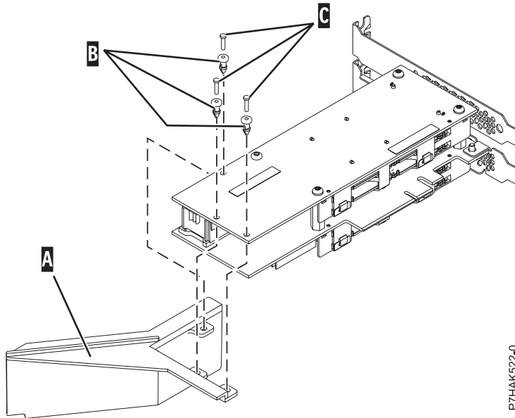
Figura 97. Instalación de un deflector de aire en el nuevo adaptador RAID PCIe y SAS SSD
