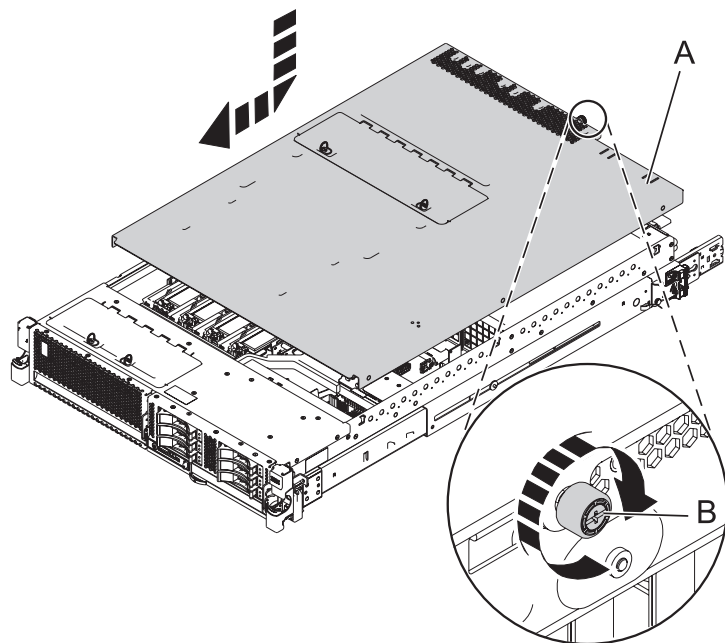
Figura 20. Instalación de la cubierta de acceso de servicio
