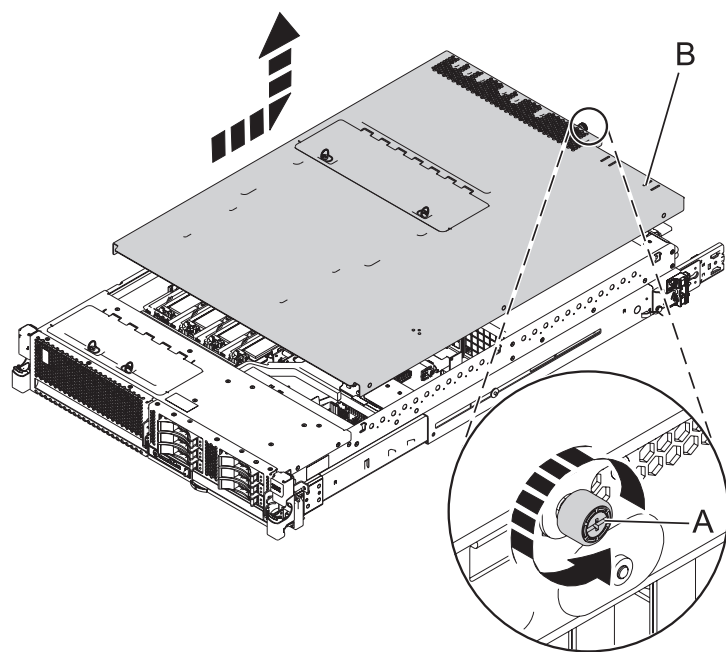
Figura 19. Extracción de la cubierta de acceso de servicio
