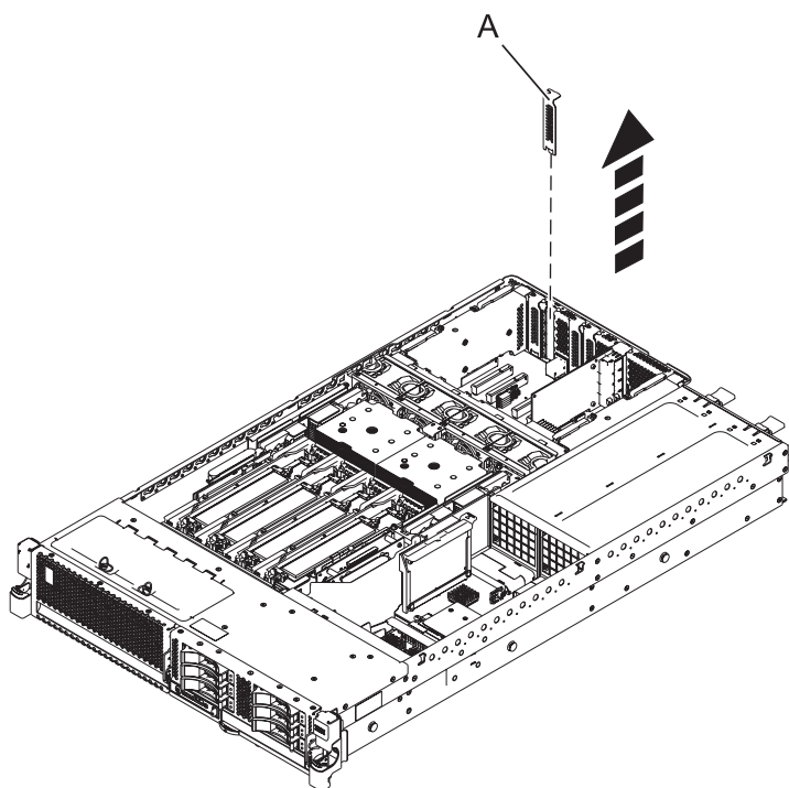
Figura 1. Extracción del adaptador PCI o de la placa de relleno de la unidad del sistema montada en bastidor.
