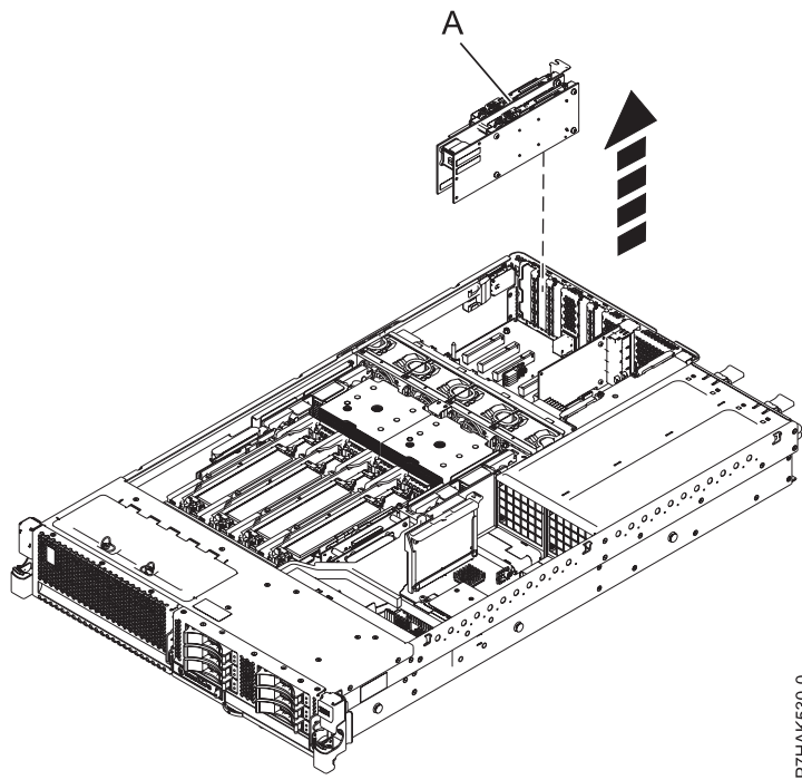
Figura 8. Extracción de un adaptador RAID PCIe y SAS SSD de una unidad del sistema montada en bastidor
