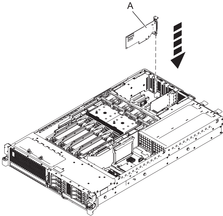
Figura 5. Sustitución del adaptador PCI en la unidad del sistema montada en bastidor
