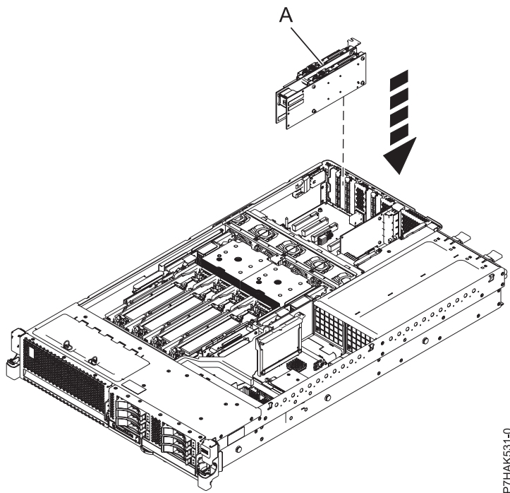
Figura 9. Instalación de un adaptador RAID PCIe y SAS SSD en una unidad del sistema montada en bastidor
