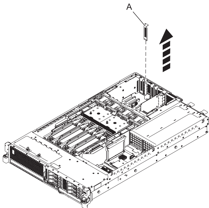
Figura 4. Extracción del adaptador PCI o de la placa de relleno de la unidad del sistema montada en bastidor.
