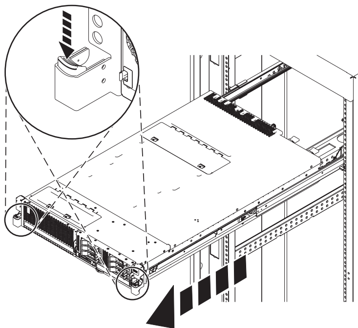
Figura 16. Colocación del sistema en la posición de servicio
