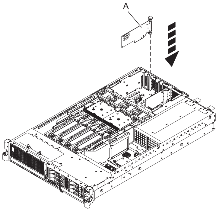
Figura 2. Sustitución del adaptador PCI en la unidad del sistema montada en bastidor
