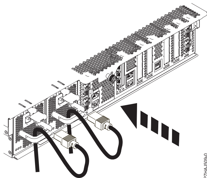
Figura 22. Conexión de los cables de alimentación
