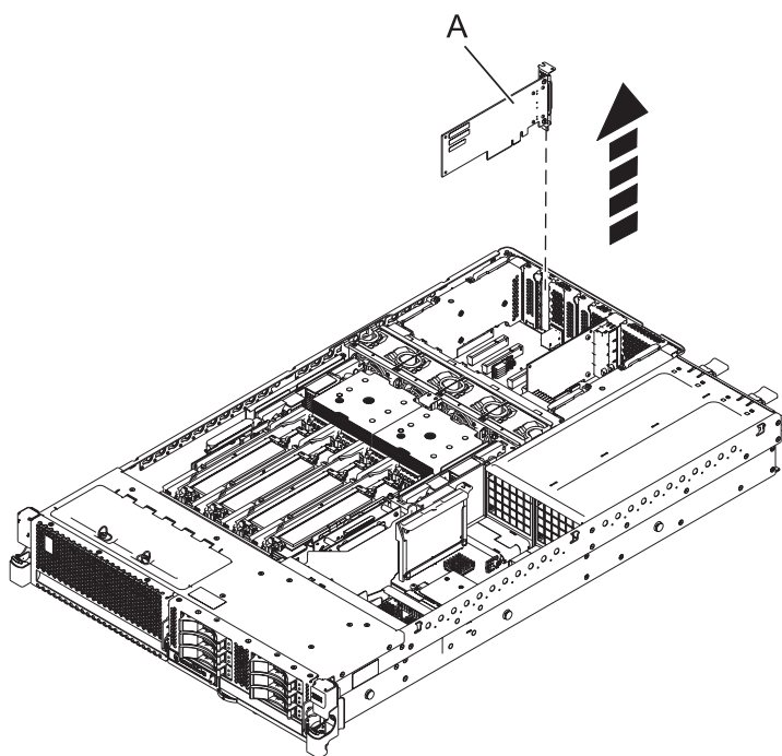
Figura 3. Extracción del adaptador PCI de la unidad del sistema montada en bastidor
