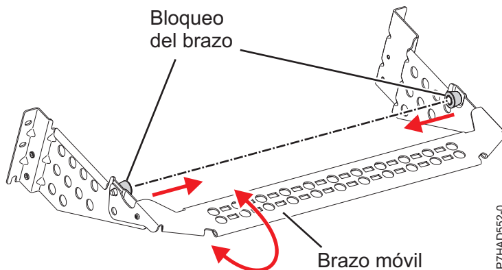
Figura 136. Abrazadera portacables
