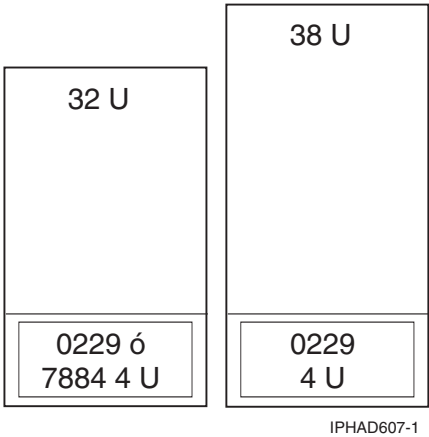
Figura 5. Código de característica 7884: 9406-520 y 9111-520 en un bastidor
