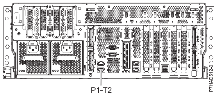
Figura 132. Vista posterior de 8202-E4B, 8202-E4C, 8202-E4D, 8205-E6B, 8205-E6C y 8205-E6D con la ubicación de instalación de los cables
