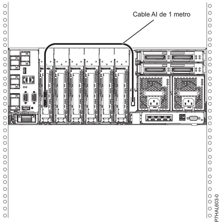
Figura 147. Conexión de un adaptador SAS con ranuras de disco SAS internas mediante el puerto SAS externo del sistema
