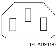
Figura 124. Tipo de enchufe 26
