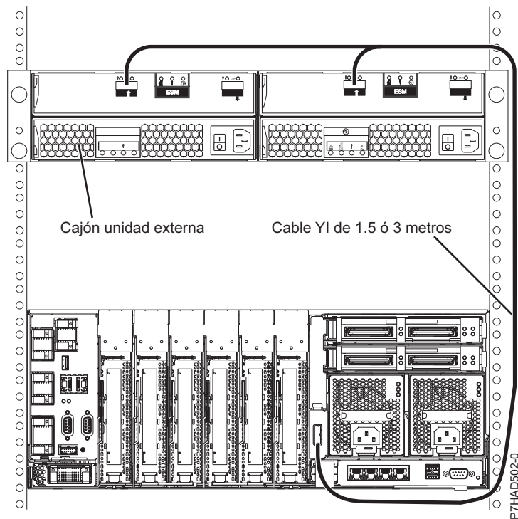
Figura 146. Conexión de un puerto de adaptador SAS externo del sistema con un cajón de expansión de disco (Modelos 9117-MMB y 9179-MHB)
