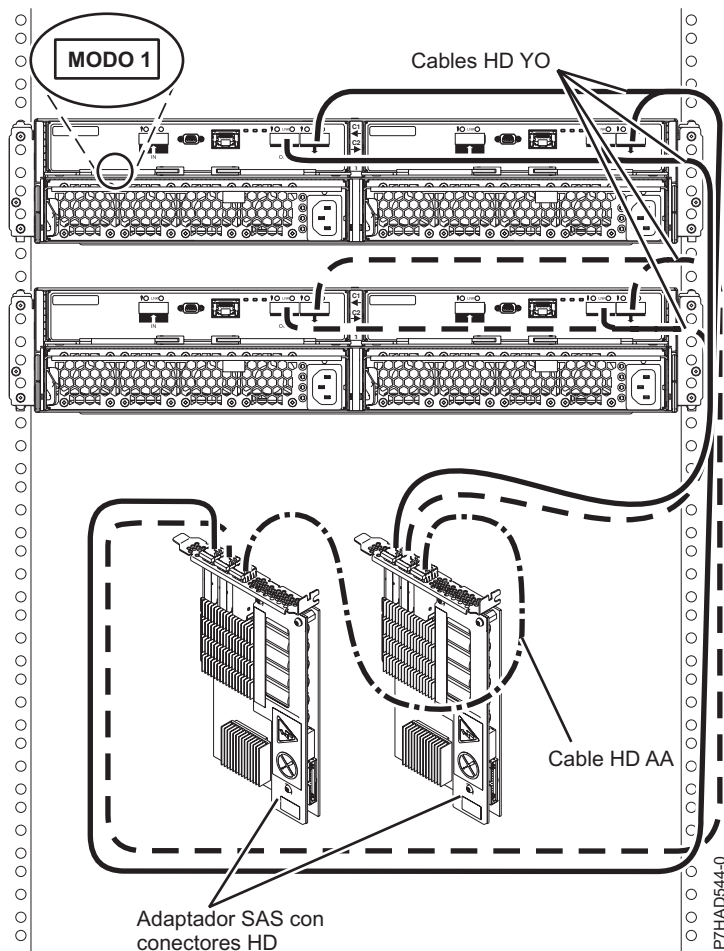
Figura 174. Conexión de modalidad 1 de dos cajones 5887 mediante conectores HD a dos adaptadores SAS
