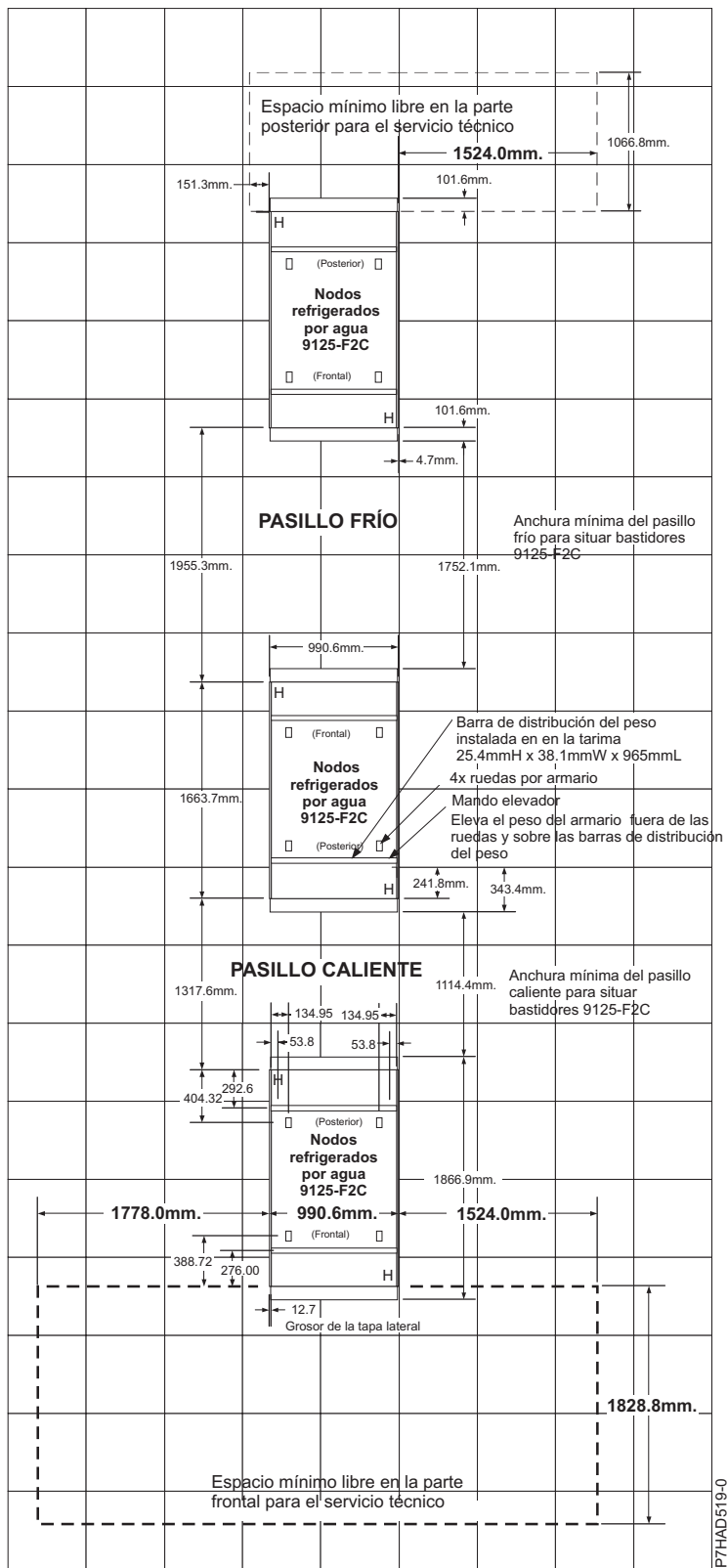
Figura 1. Espacio libre de servicio para un solo bastidor: pasillo frío y pasillo caliente
