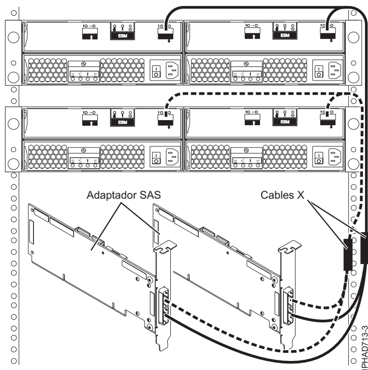
Figura 155. Conexión de dos adaptadores RAID SAS con dos cajones de expansión de disco en una configuración RAID HA de multi-iniciador.
