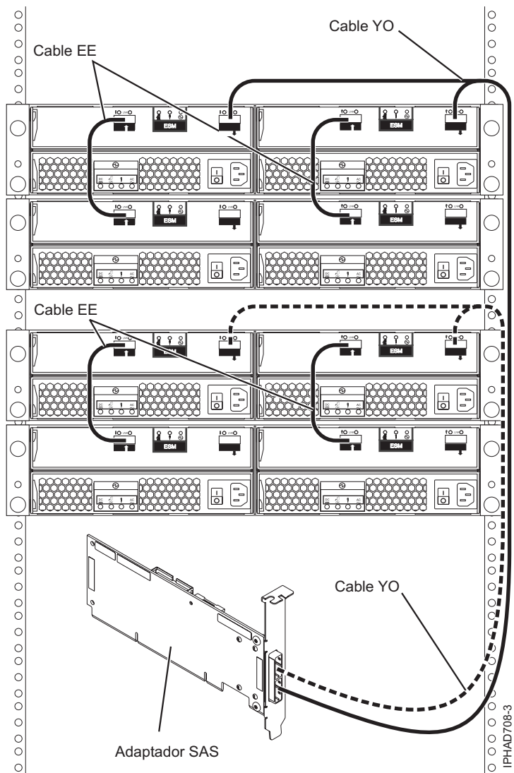
Figura 147. Conexión de un adaptador SAS con cuatro cajones de expansión de disco
