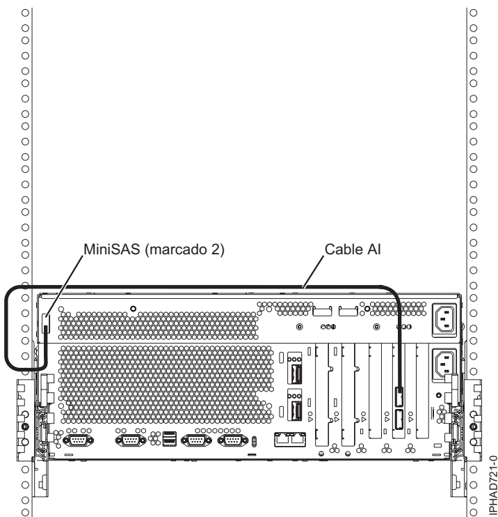
Figura 152. Conexión de un adaptador SAS con ranuras de disco SAS internas mediante el puerto SAS externo del sistema
