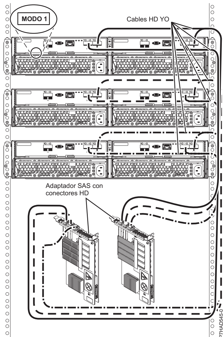
Figura 175. Conexión de modalidad 1 de tres cajones 5887 a dos adaptadores SAS con conectores HD
