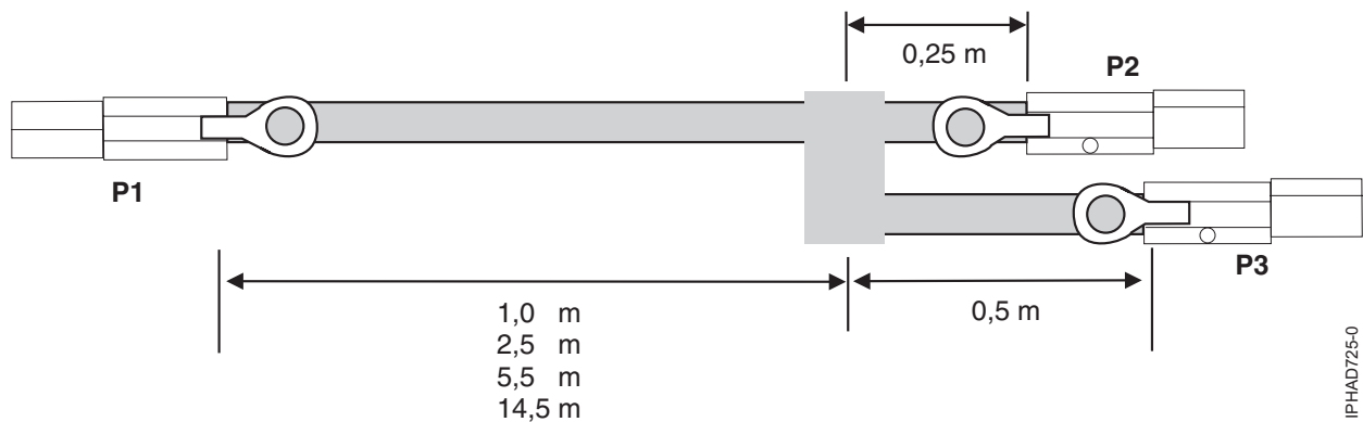
Figura 143. Longitudes de cable de conjunto de cables YO SAS externos
