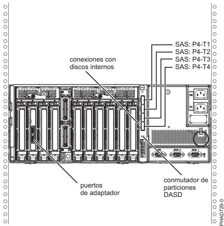
Figura 163. Conexión de dos adaptadores RAID SAS con un cajón de expansión de disco en una configuración JBOD HA de multi-iniciador.
