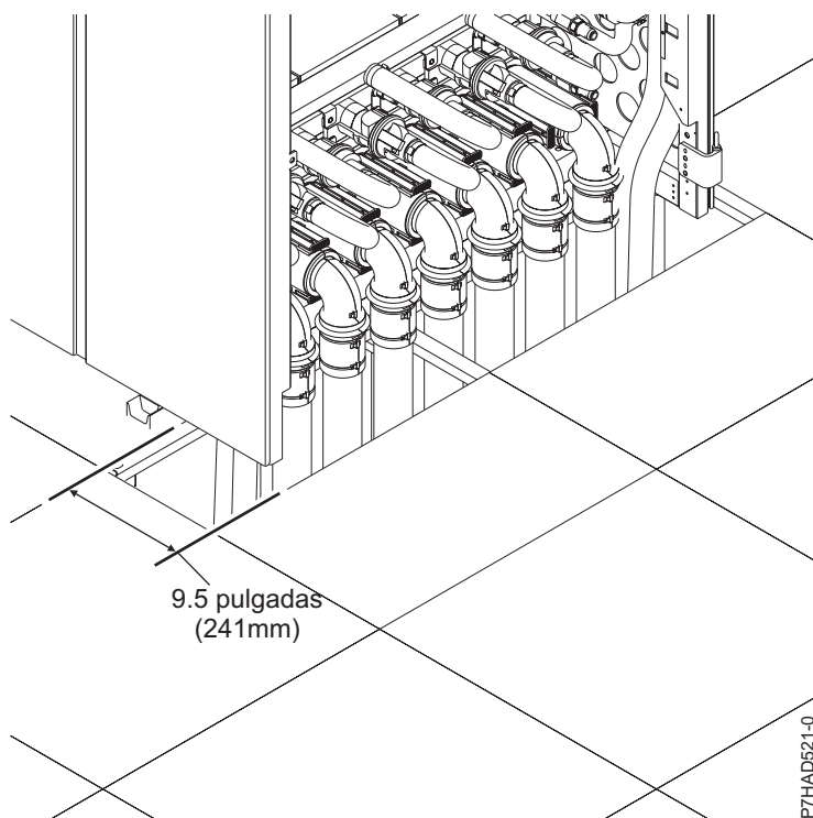
Figura 3. Abertura de suelo
