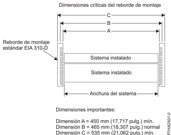
Figura 179. Dimensiones críticas del reborde de montaje
