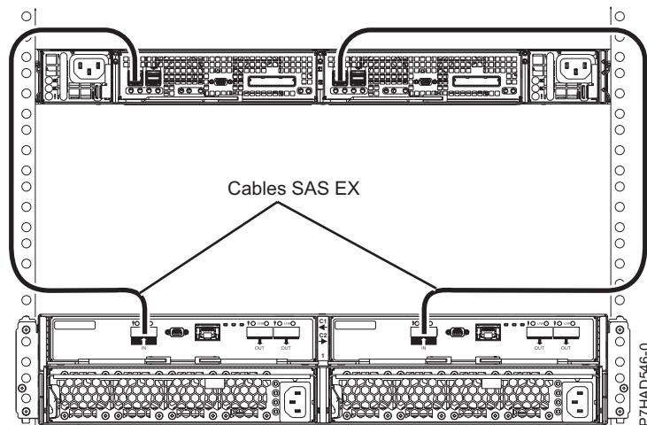
Figura 177. Conexión de un cajón 5887 mediante cables HD EX con un EDR1
