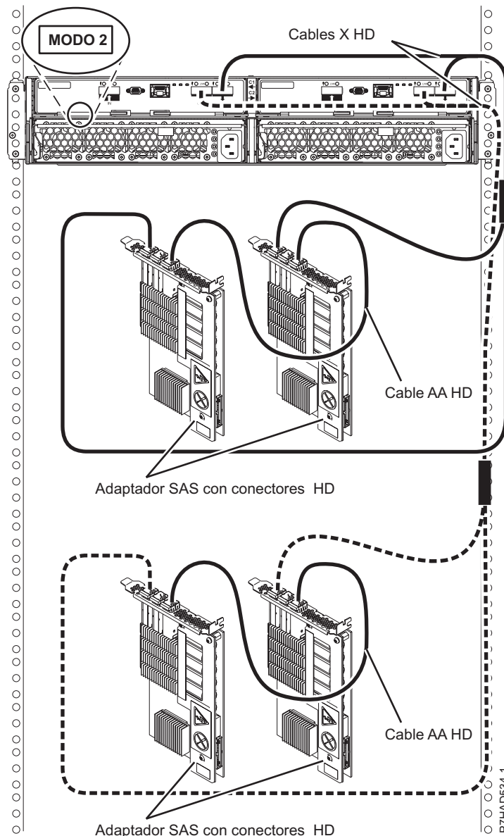
Figura 176. Conexión de modalidad 2 de un cajón 5887 mediante conectores HD a dos pares de adaptadores SAS
