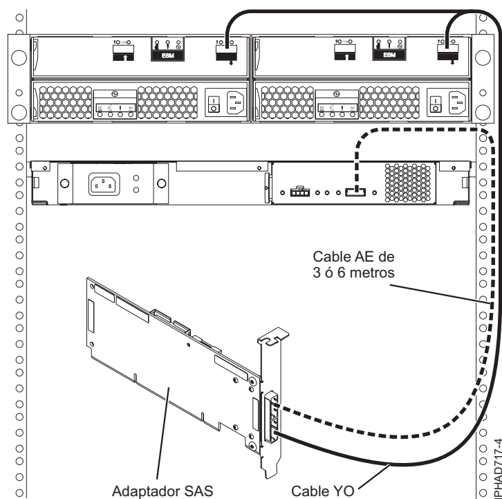
Figura 150. Conexión de un adaptador SAS con un cajón de expansión de disco y con un cajón de expansión de soporte
