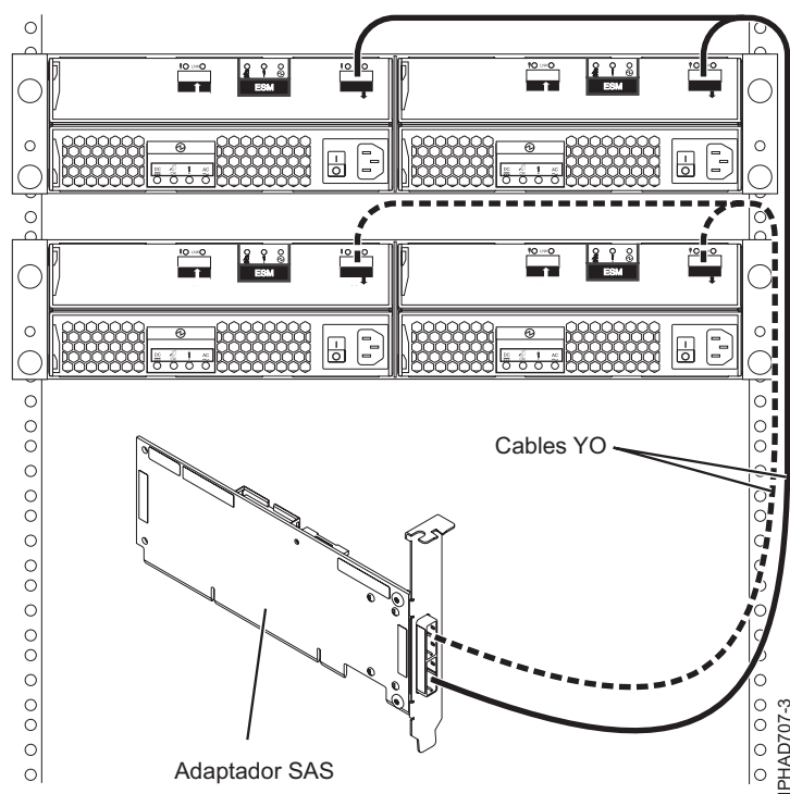
Figura 146. Conexión de un adaptador SAS con dos cajones de expansión de disco
