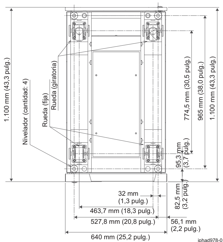
Figura 26. Ubicaciones de ruedas giratorias y niveladores
