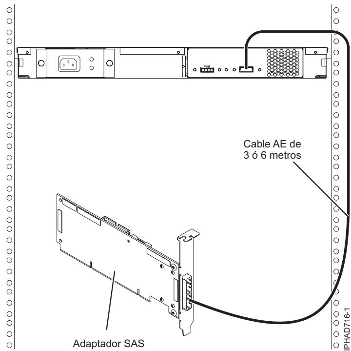
Figura 149. Conexión de un adaptador SAS con un cajón de expansión de soporte
