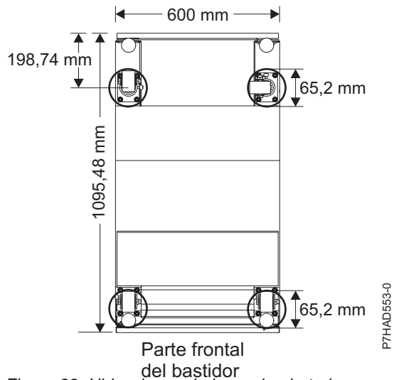
Figura 28. Ubicaciones de la rueda giratoria
