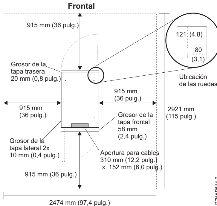
Figura 27. Ubicación de las ruedas giratorias y espacios libres de servicio de los bastidores 7014-T00, 7014-T42 y 0553
