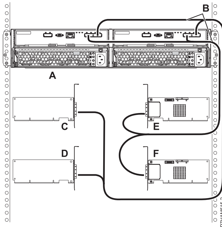
Figura 168. Conexión de modalidad 4 de un cajón 5887 mediante cables X a cuatro adaptadores SAS únicos
