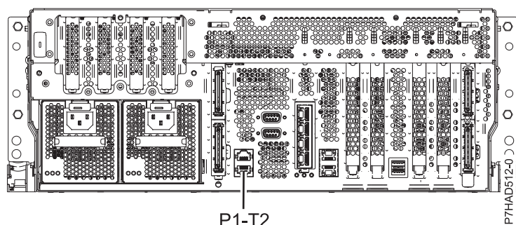
Figura 137. Vista posterior de 8202-E4B, 8202-E4C, 8202-E4D, 8205-E6B, 8205-E6C y 8205-E6D con la ubicación de instalación de los cables
