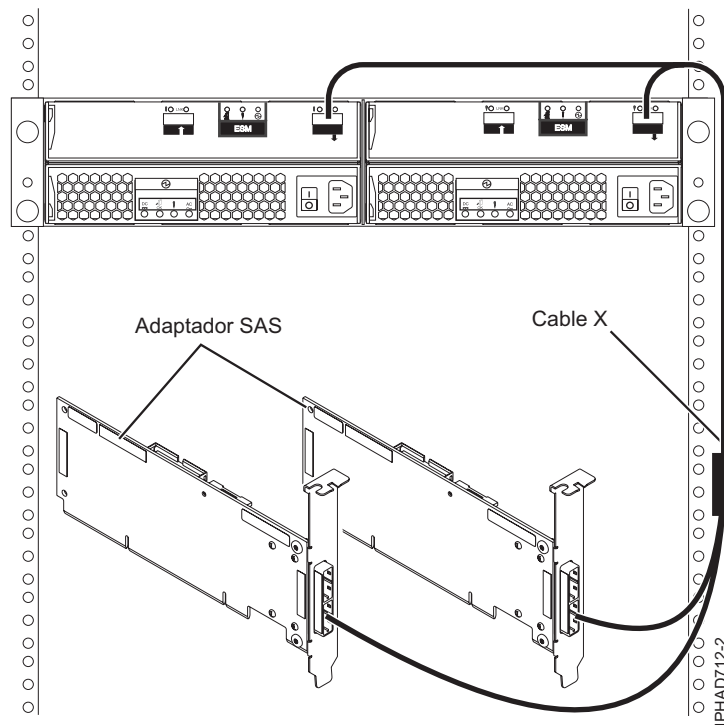
Figura 154. Conexión de dos adaptadores RAID SAS con un cajón de expansión de disco en una configuración RAID HA de multi-iniciador.
