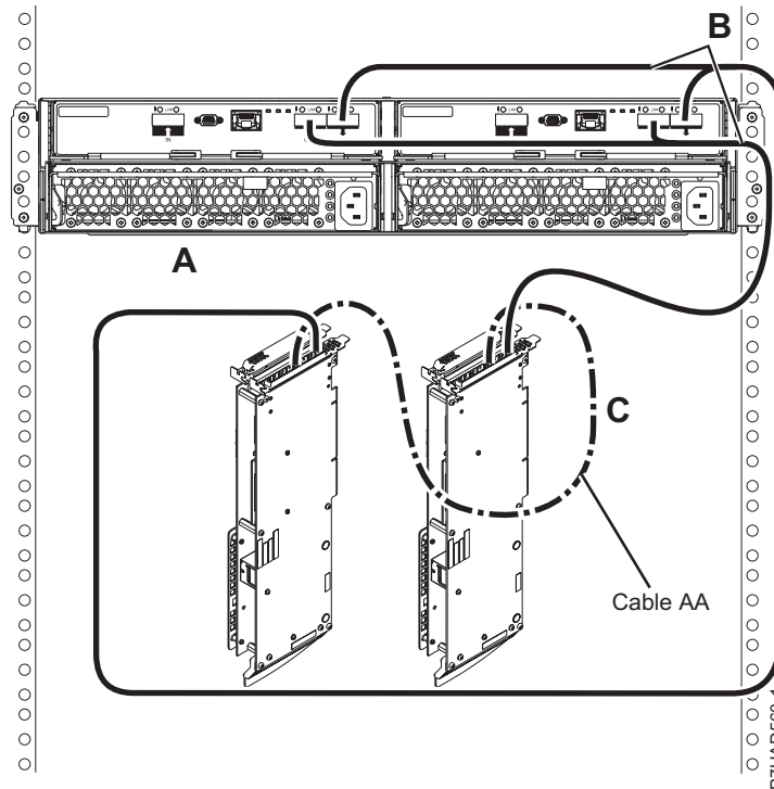
Figura 172. Conexión de modalidad 1 de un cajón 5887 mediante cables YO a adaptadores SAS duales
