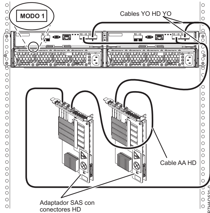
Figura 173. Conexión de modalidad 1 de un cajón 5887 a dos adaptadores SAS con conectores HD
