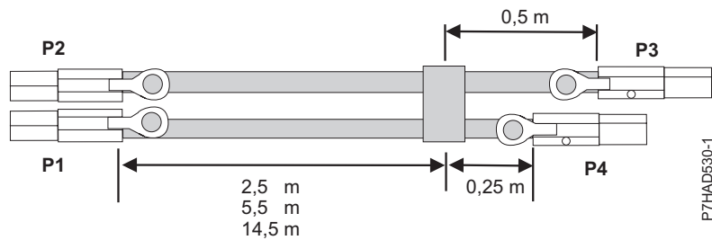
Figura 142. Longitudes de cable de conjunto de cables X SAS externos
