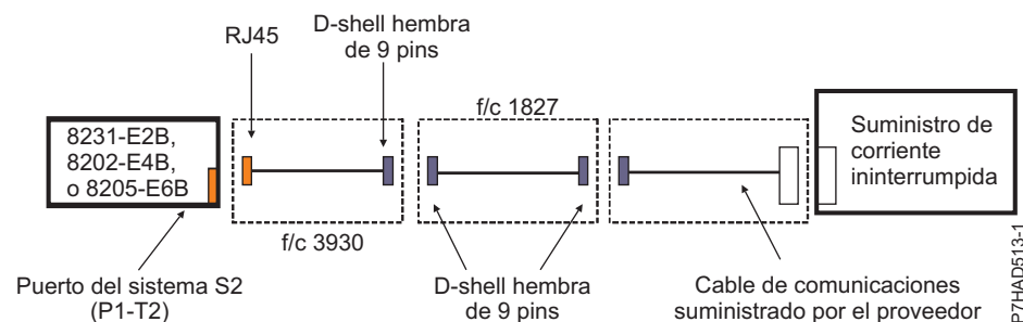
Figura 138. Conexión del sistema de alimentación ininterrumpible para 8202-E4B, 8202-E4C, 8205-E6B, 8205-E6C, 8231-E2B, 8231-E1C, 8231-E1D, 8231-E2C, 8231-E2D y 8268-E1D
