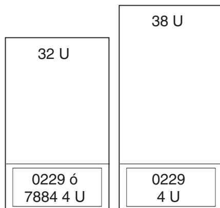
Figura 10. Código de característica 7884: 9406-520 y 9111-520 en un bastidor
