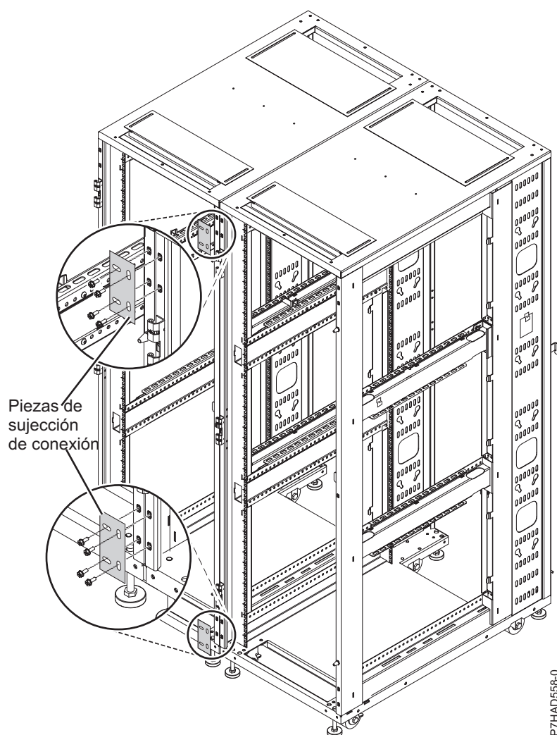
Figura 33. Piezas de sujeción de conexión
