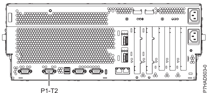
Figura 134. Vista posterior de 8233-E8B y 8236-E8C con ubicación de instalación del cable
