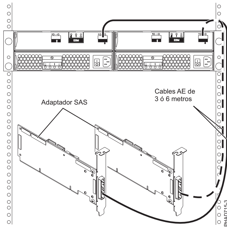
Figura 162. Conexión de dos adaptadores RAID SAS con un cajón de expansión de disco en una configuración JBOD HA de multi-iniciador.
