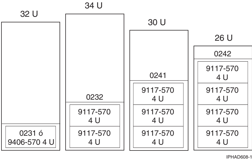
Figura 12. 570 en bastidor
