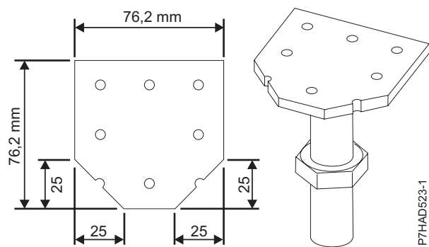
Figura 4. Dimensiones de pedestal cortado
