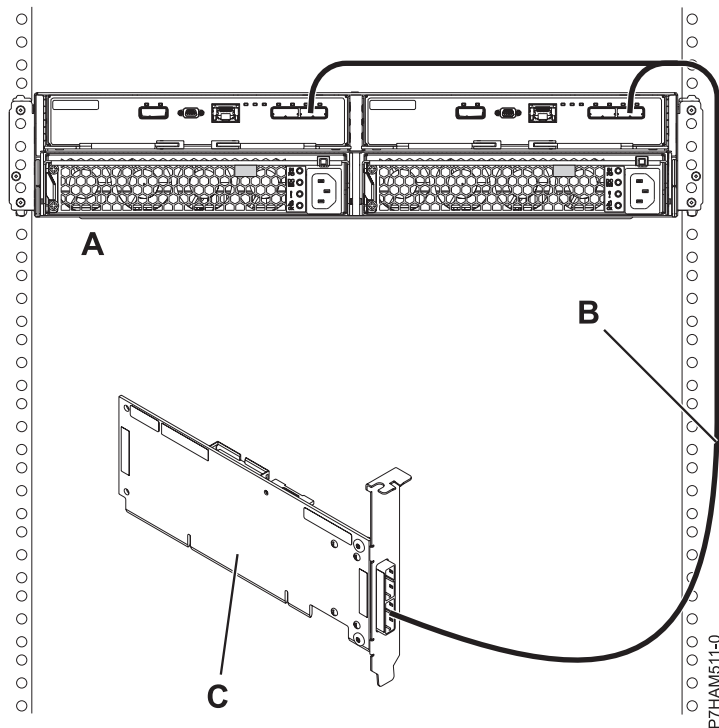
Figura 164. Conexión de modalidad 1 de un cajón 5887 mediante un cable YO a un único adaptador SAS
