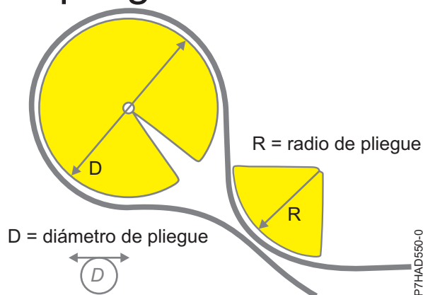
Figura 140. Radio de curvatura del cable
