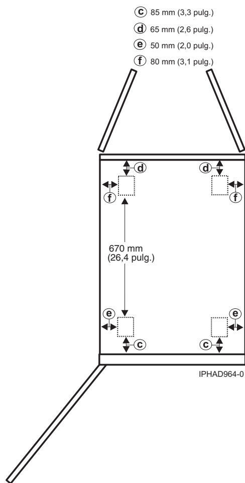
Figura 25. Ubicación de las ruedas giratorias del modelo 0555 y 7014-S25
