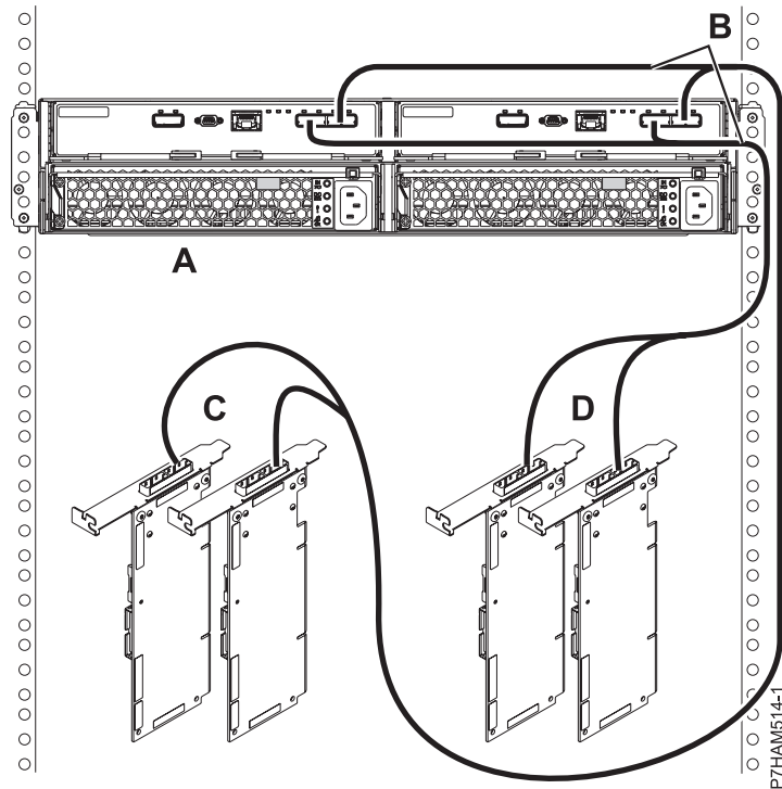
Figura 167. Conexión de modalidad 2 de un cajón 5887 mediante cables X a dos pares de adaptadores SAS
