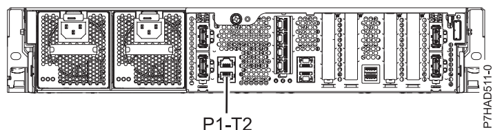
Figura 136. Vista posterior de 8231-E2B, 8231-E1C, 8231-E1D, 8231-E2C, 8231-E2D y 8268-E1D con la ubicación de instalación de los cables
