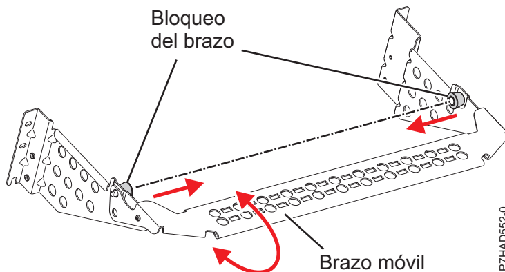
Figura 141. Abrazadera portacables
