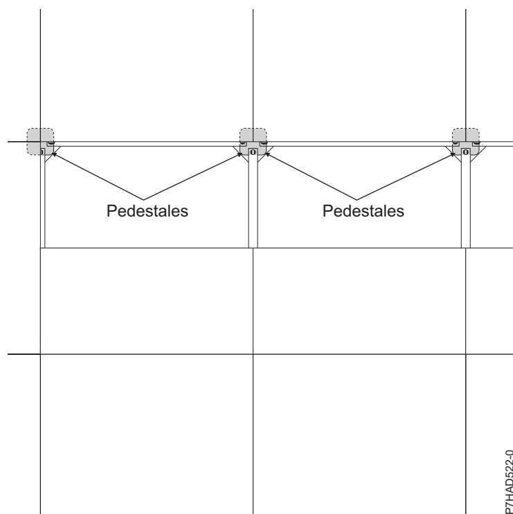
Figura 5. Pedestales cortados
