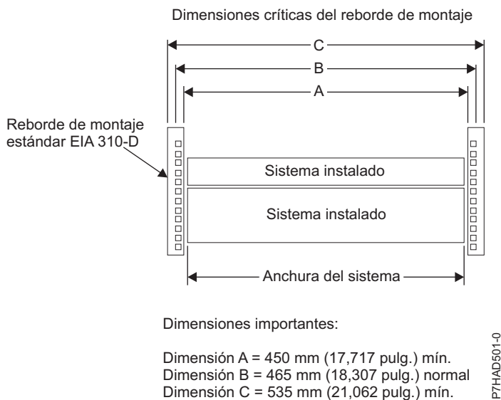
Figura 34. Dimensiones críticas del reborde de montaje
