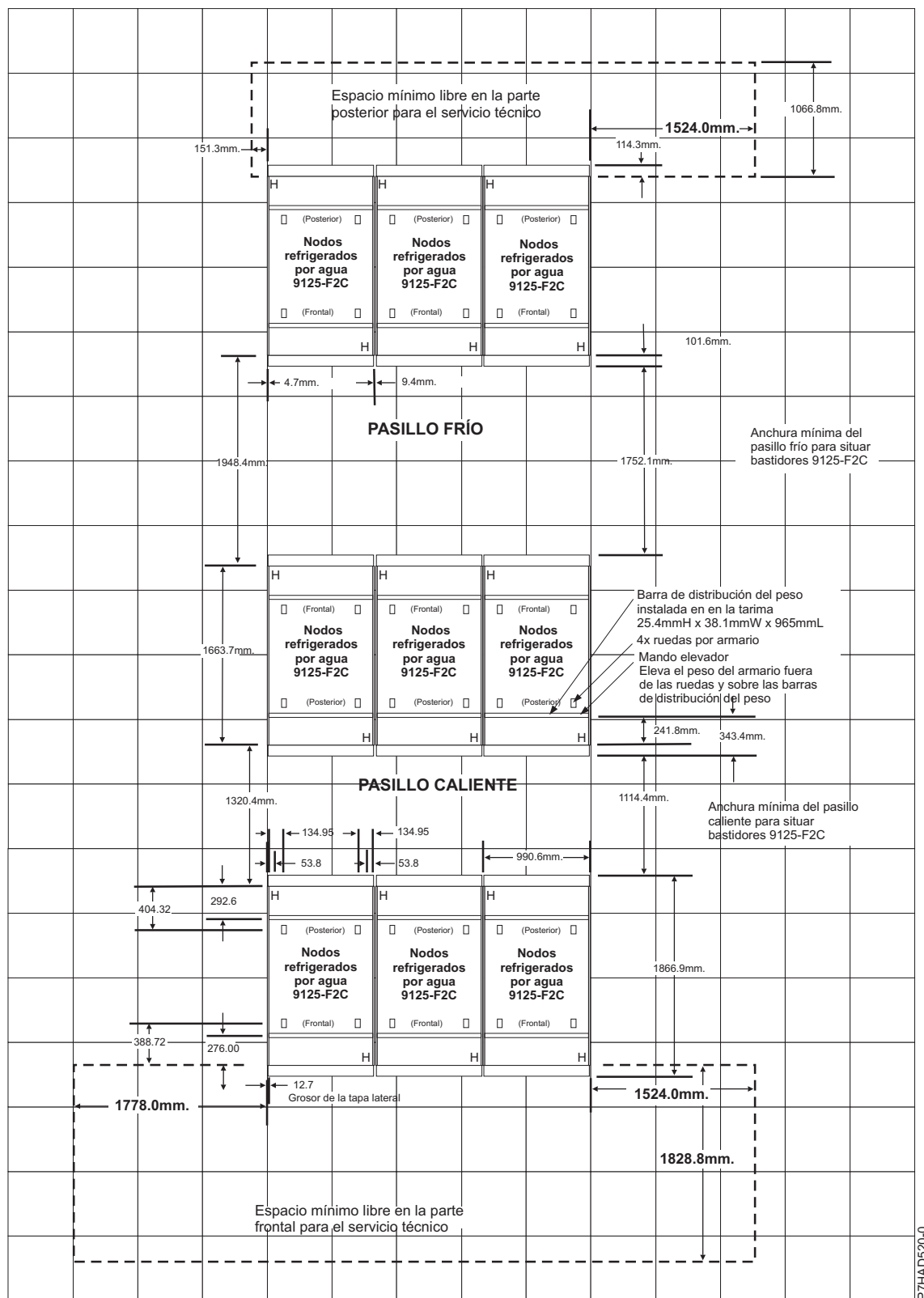
Figura 2. Espacio libre de servicio para varios bastidores: pasillo frío y pasillo caliente
