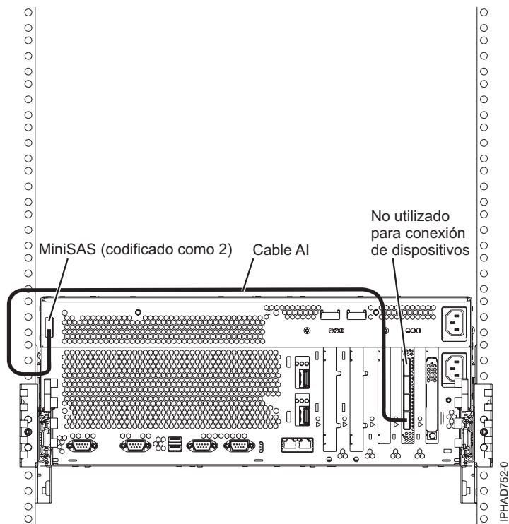
Figura 153. Adaptador FC5904 o FC5908 conectado a cajones de expansión de disco
