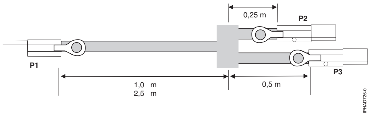
Figura 144. Longitudes de cable de conjunto de cables YI SAS externos
