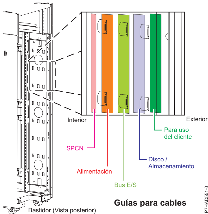
Figura 139. Lanzas puente portacables
