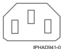
Figura 77. Tipo de enchufe 15
