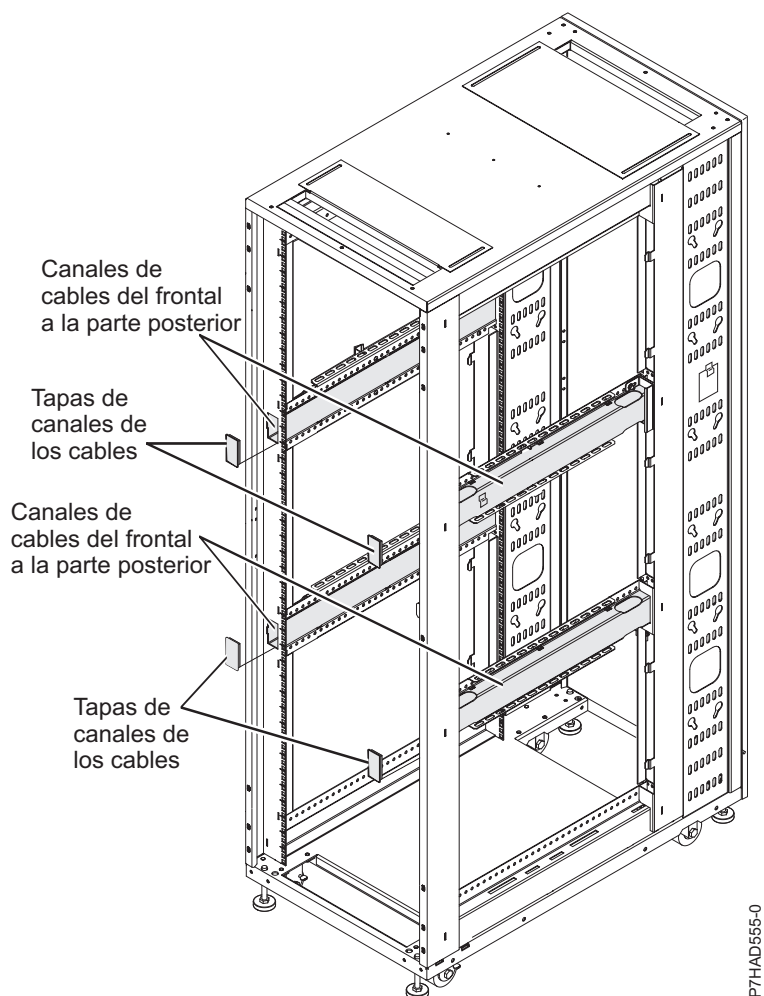
Figura 29. Cableado dentro del bastidor
