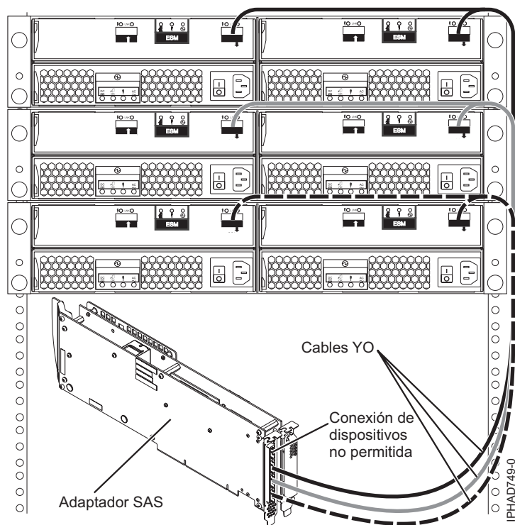
Figura 148. Conexión de adaptador SAS de tres puertos con cajones de expansión de disco
