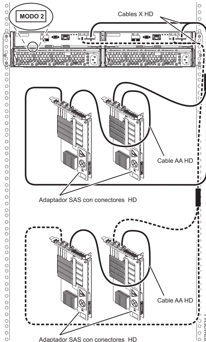
Figura 172. Conexión de modalidad 2 de un cajón 5887 mediante conectores HD a dos pares de adaptadores SAS
