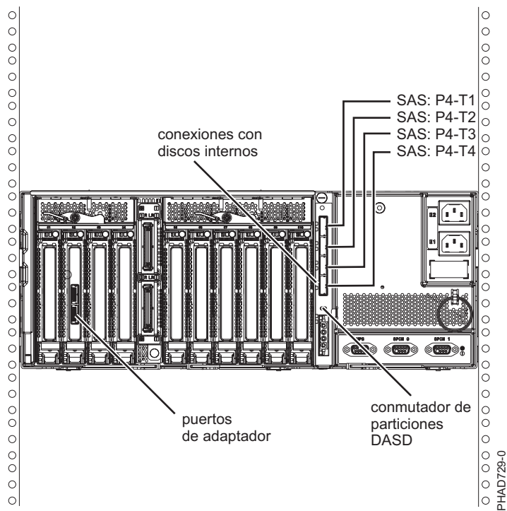
Figura 159. Conexión de dos adaptadores RAID SAS con un cajón de expansión de disco en una configuración JBOD HA de multi-iniciador.
