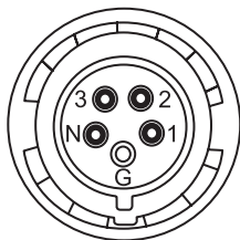
Figura 32. Sujeción de enchufe
