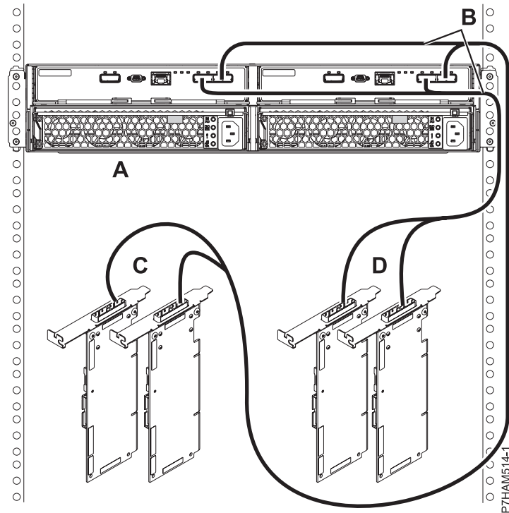
Figura 163. Conexión de modalidad 2 de un cajón 5887 mediante cables X a dos pares de adaptadores SAS
