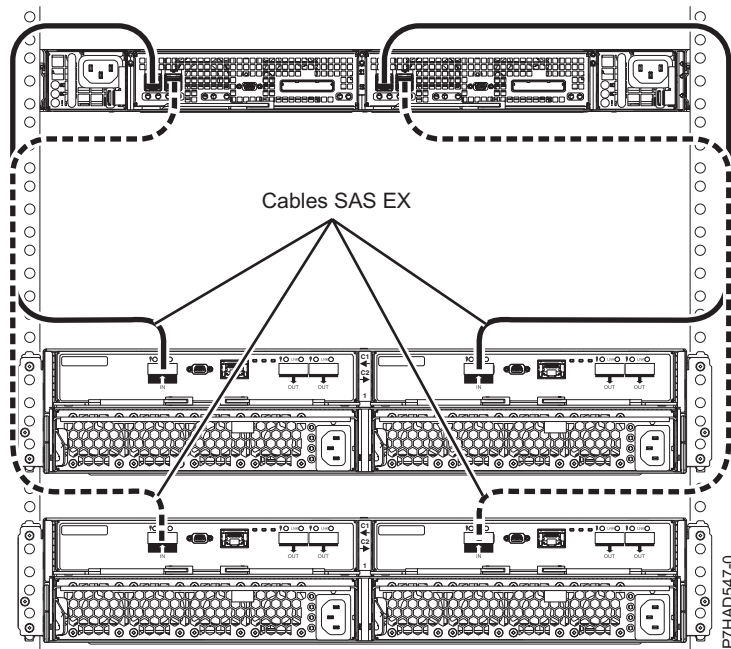
Figura 174. Conexión de dos cajones 5887 mediante cables HD EX con un EDR1
