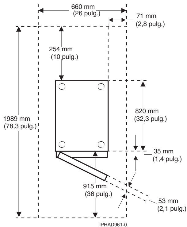
Figura 17. Vista de planta del modelo 0554 y 7014-S11
