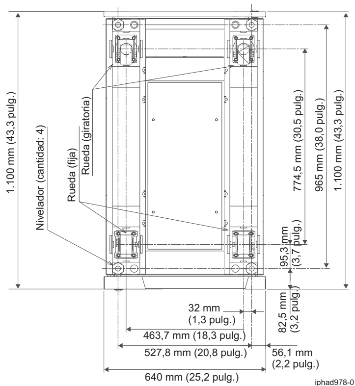
Figura 5. Ubicaciones de ruedas giratorias y niveladores
