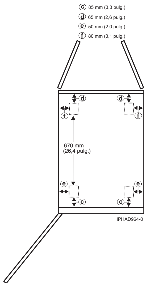
Figura 21. Ubicación de las ruedas giratorias del modelo 0555 y 7014-S25
