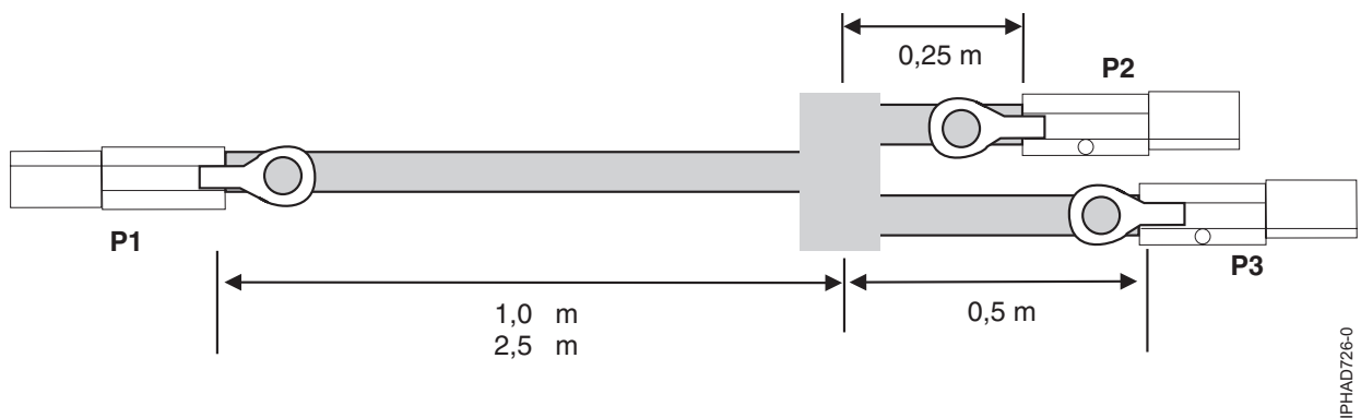
Figura 140. Longitudes de cable de conjunto de cables YI SAS externos
