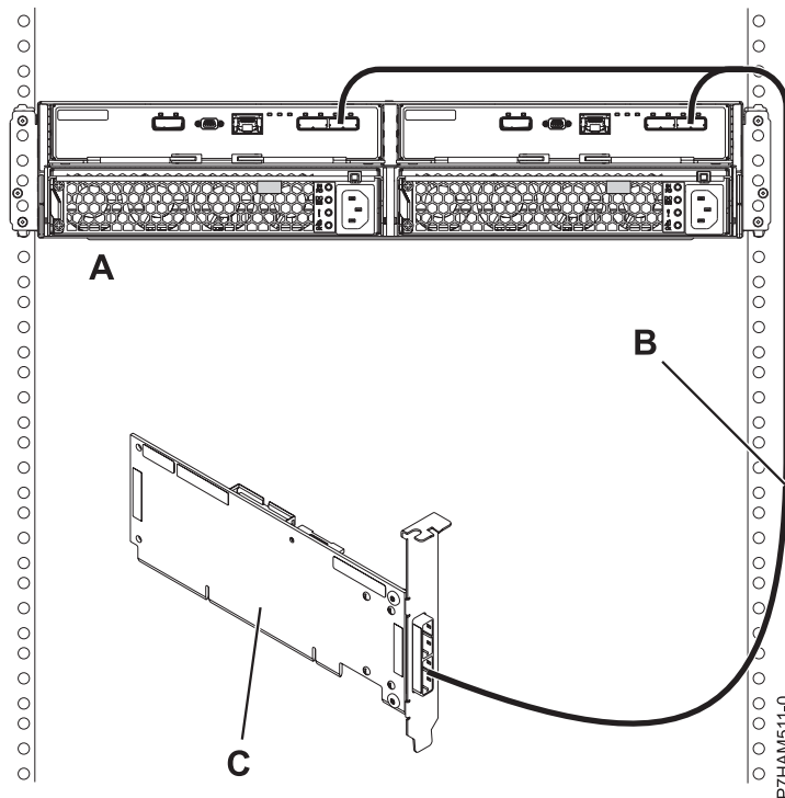
Figura 160. Conexión de modalidad 1 de un cajón 5887 mediante un cable YO a un único adaptador SAS
