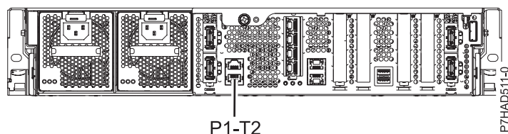
Figura 132. Vista posterior de 8231-E2B, 8231-E1C, 8231-E1D, 8231-E2C, 8231-E2D y 8268-E1D con la ubicación de instalación de los cables
