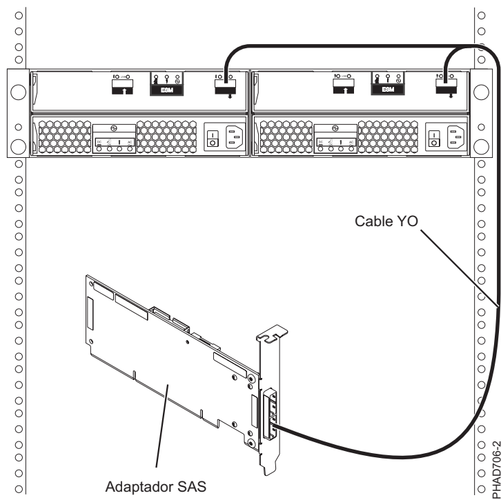
Figura 141. Conexión de un adaptador SAS con un cajón de expansión de disco
