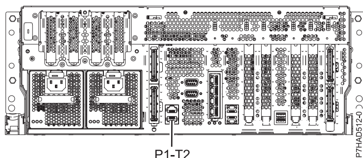
Figura 133. Vista posterior de 8202-E4B, 8202-E4C, 8202-E4D, 8205-E6B, 8205-E6C y 8205-E6D con la ubicación de instalación de los cables
