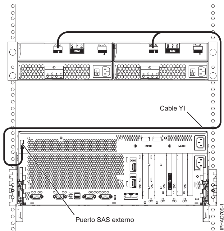
Figura 147. Conexión de un puerto de adaptador SAS externo del sistema con un cajón de expansión de disco
