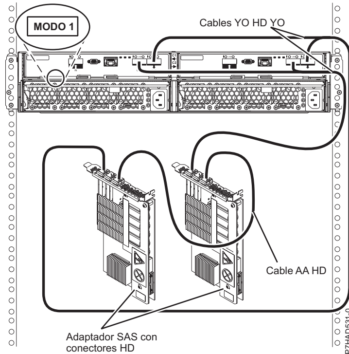
Figura 169. Conexión de modalidad 1 de un cajón 5887 a dos adaptadores SAS con conectores HD
