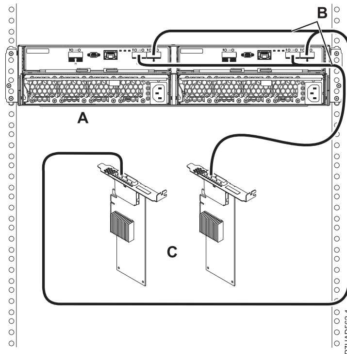
Figura 161. Conexión de modalidad 1 de un cajón 5887 mediante cables YO a adaptadores SAS duales
