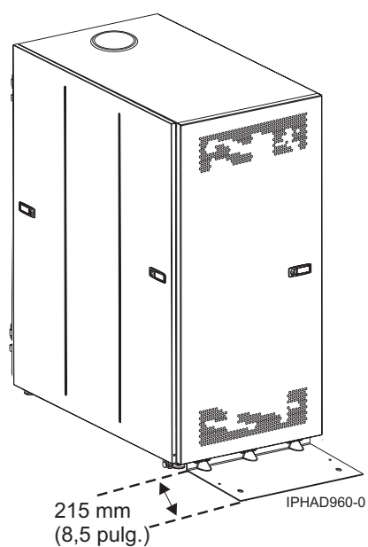
Figura 19. Modelo 0555 y 7014-S25 con pie estabilizador
