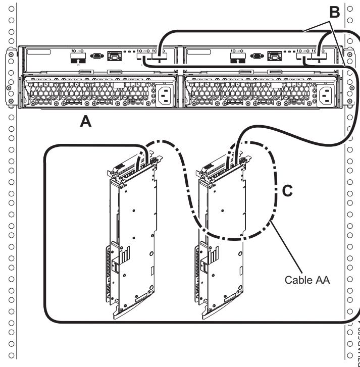
Figura 168. Conexión de modalidad 1 de un cajón 5887 mediante cables YO a adaptadores SAS duales
