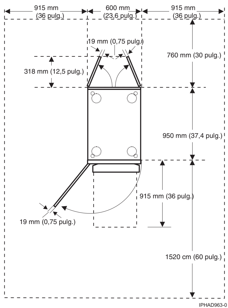
Figura 20. Vista de planta del modelo 0555 y 7014-S25
