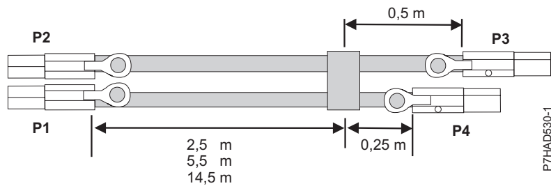
Figura 138. Longitudes de cable de conjunto de cables X SAS externos
