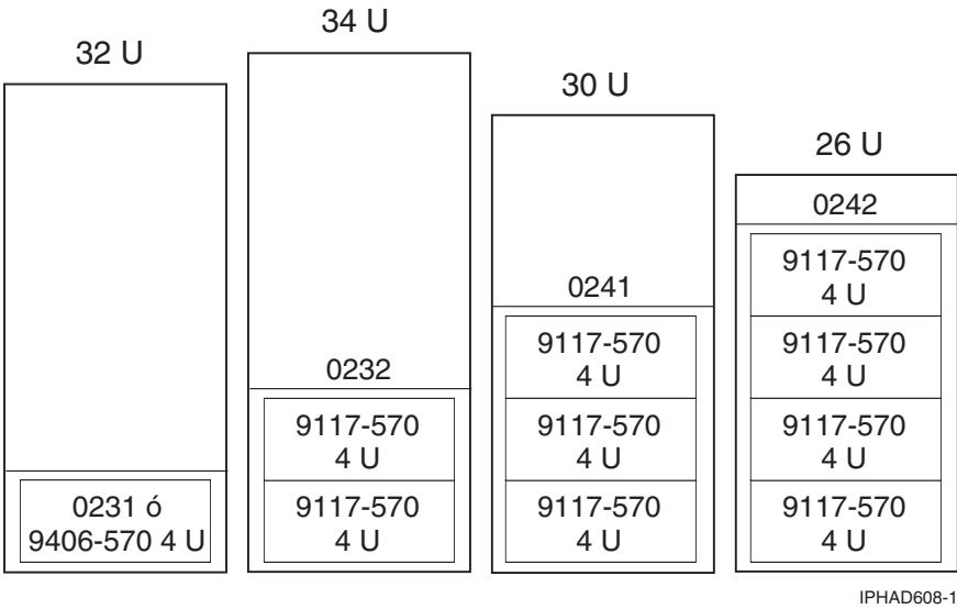
Figura 8. 570 en bastidor
