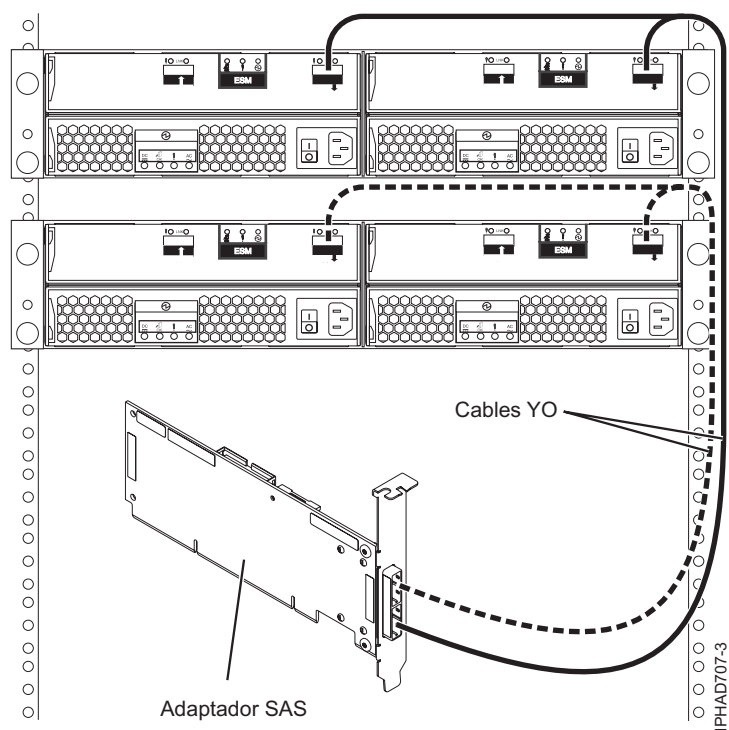
Figura 142. Conexión de un adaptador SAS con dos cajones de expansión de disco
