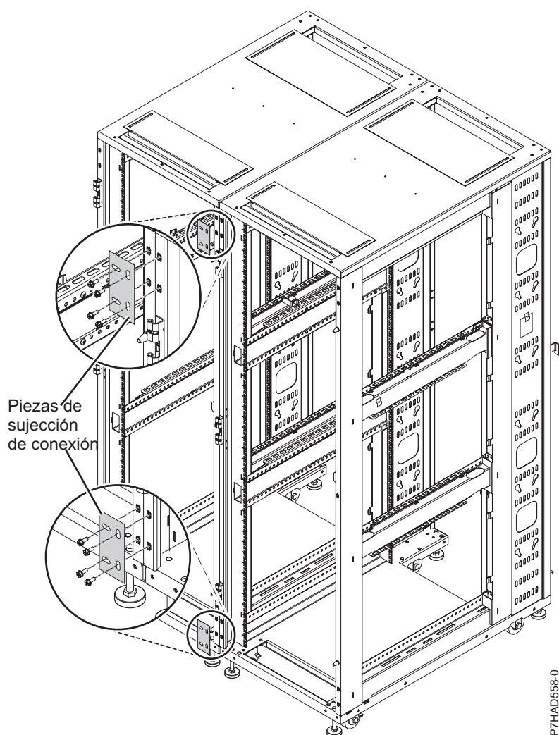
Figura 29. Piezas de sujeción de conexión
