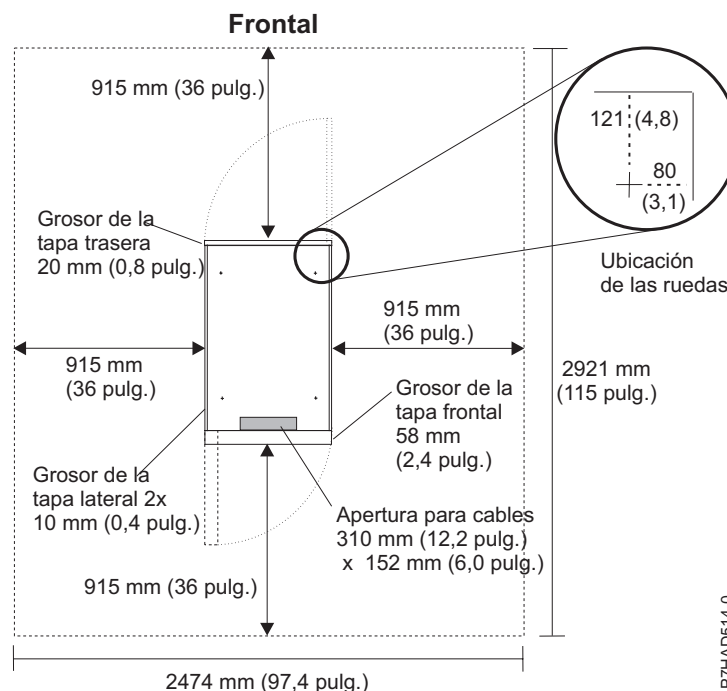
Figura 23. Ubicación de las ruedas giratorias y espacios libres de servicio de los bastidores 7014-T00, 7014-T42 y 0553
