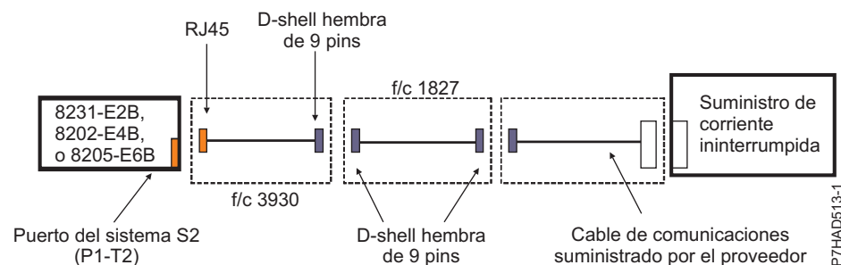
Figura 134. Conexión del sistema de alimentación ininterrumpible para 8202-E4B, 8202-E4C, 8205-E6B, 8205-E6C, 8231-E2B, 8231-E1C, 8231-E1D, 8231-E2C, 8231-E2D y 8268-E1D
