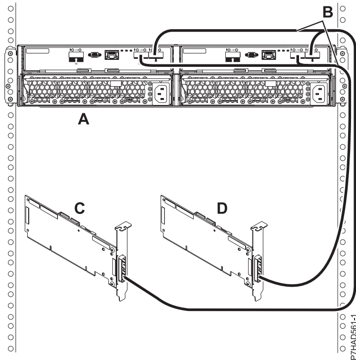
Figura 162. Conexión de modalidad 2 de un cajón 5887 mediante cables YO a dos adaptadores SAS únicos
