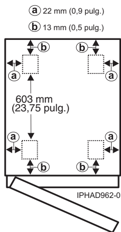
Figura 18. Ubicación de las ruedas giratorias del modelo 0554 y 7014-S11
