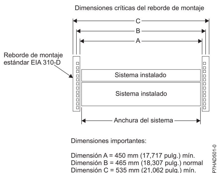
Figura 175. Dimensiones críticas del reborde de montaje
