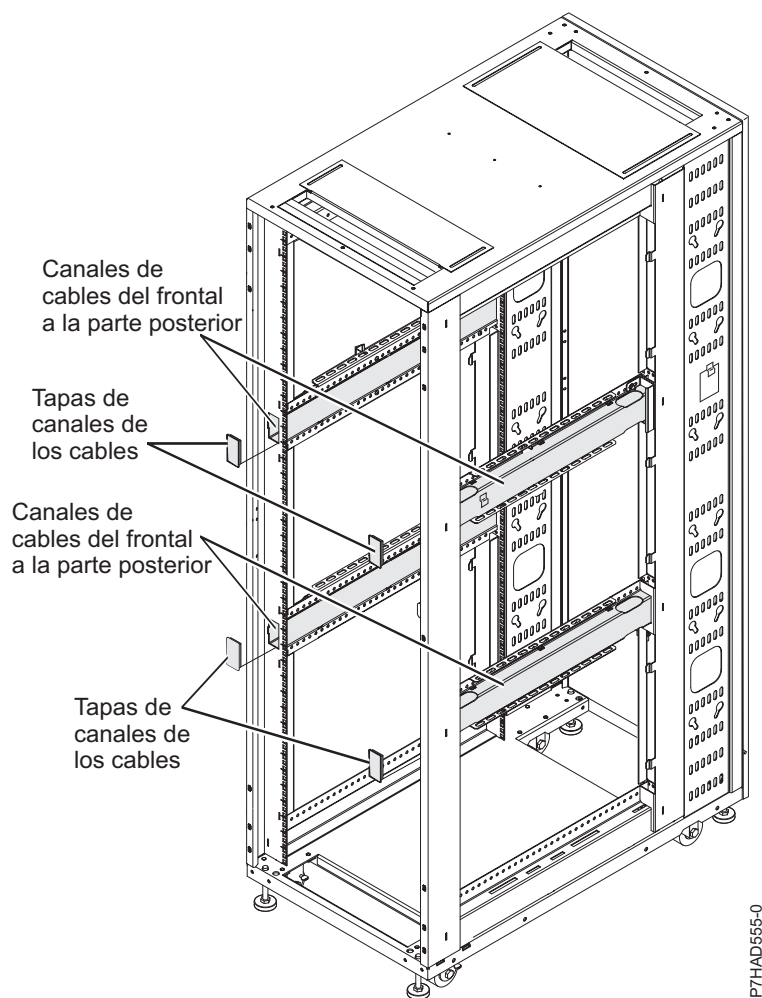
Figura 25. Cableado dentro del bastidor
