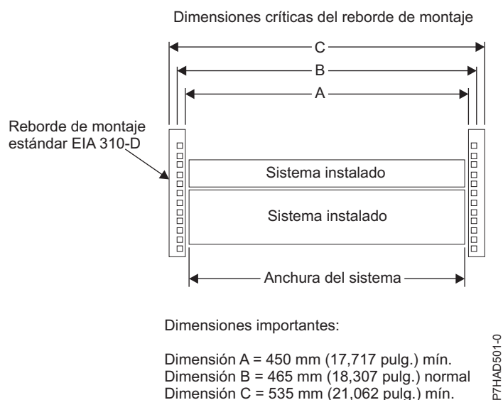
Figura 30. Dimensiones críticas del reborde de montaje
