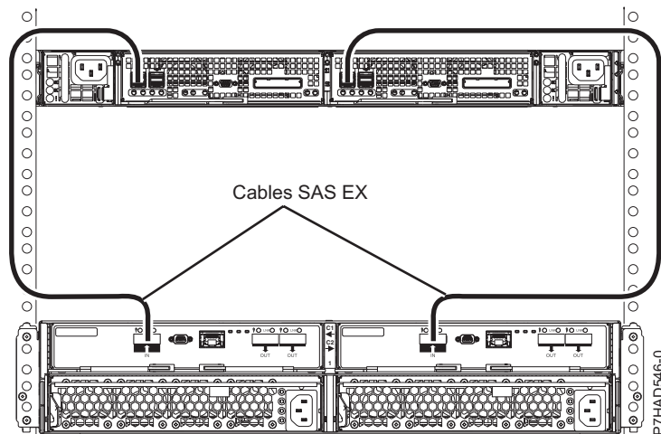
Figura 173. Conexión de un cajón 5887 mediante cables HD EX con un EDR1
