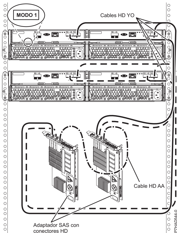
Figura 170. Conexión de modalidad 1 de dos cajones 5887 mediante conectores HD a dos adaptadores SAS
