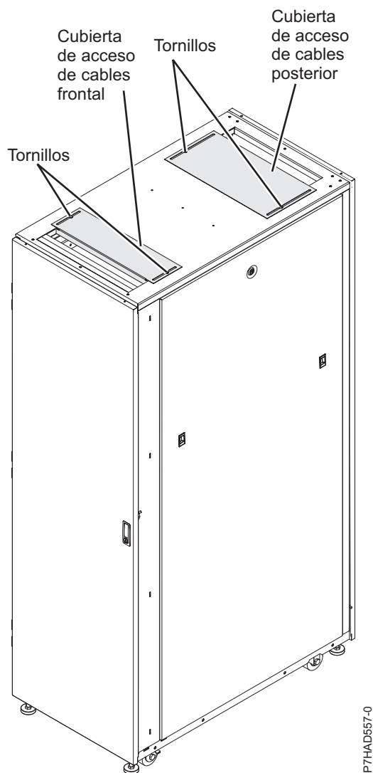
Figura 27. Cubiertas de acceso de cables
