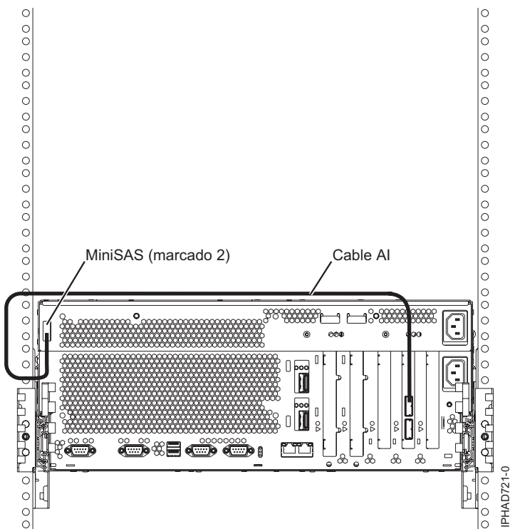
Figura 148. Conexión de un adaptador SAS con ranuras de disco SAS internas mediante el puerto SAS externo del sistema
