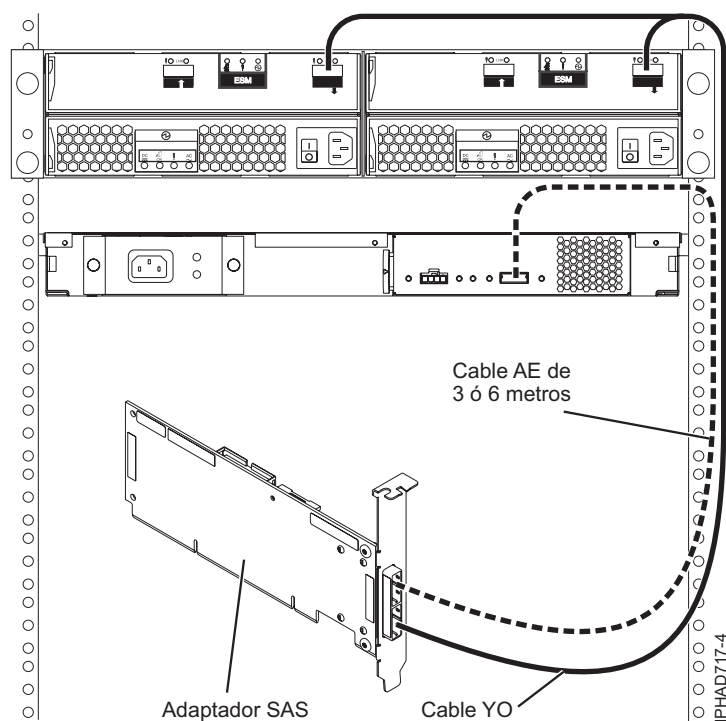
Figura 146. Conexión de un adaptador SAS con un cajón de expansión de disco y con un cajón de expansión de soporte
