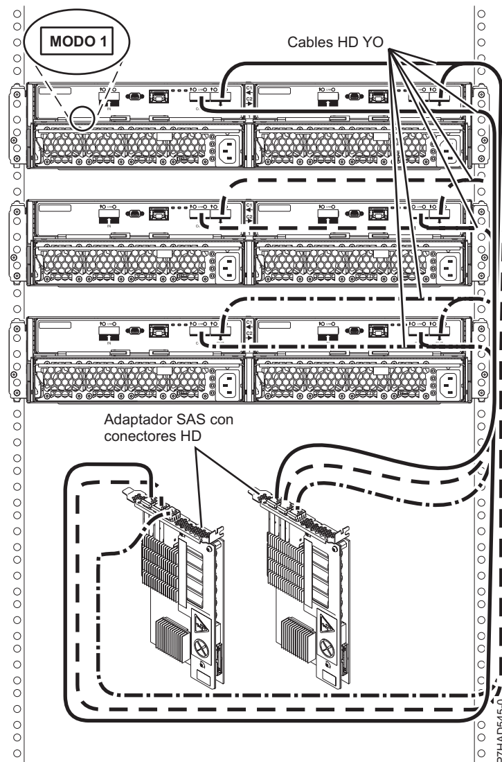
Figura 171. Conexión de modalidad 1 de tres cajones 5887 a dos adaptadores SAS con conectores HD
