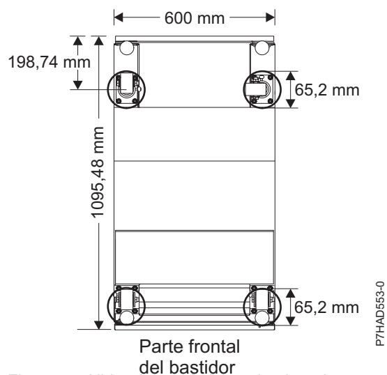
Figura 24. Ubicaciones de la rueda giratoria
