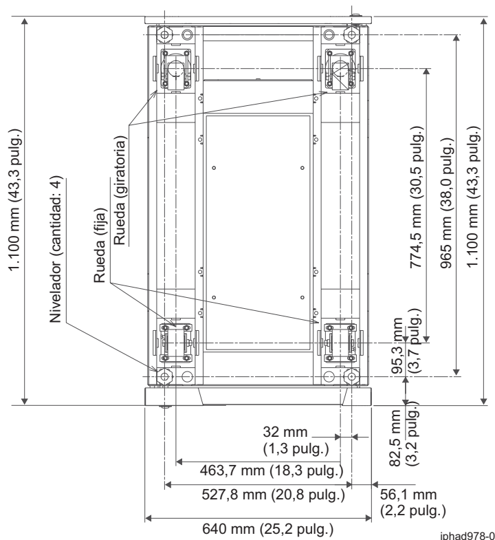
Figura 22. Ubicaciones de ruedas giratorias y niveladores
