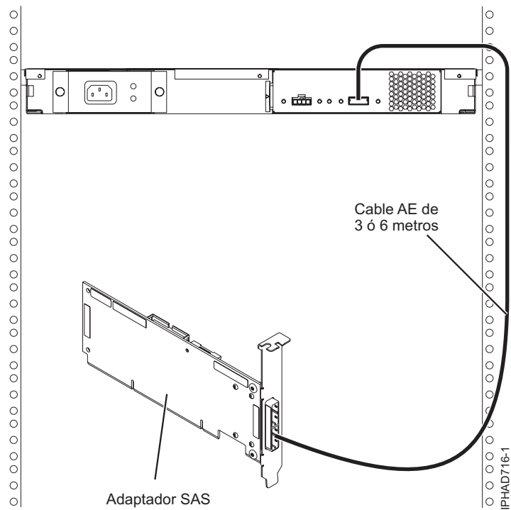
Figura 145. Conexión de un adaptador SAS con un cajón de expansión de soporte
