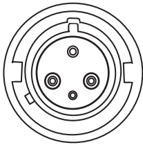
Figura 50. Tipo de receptáculo IEC 60309 2P+E
