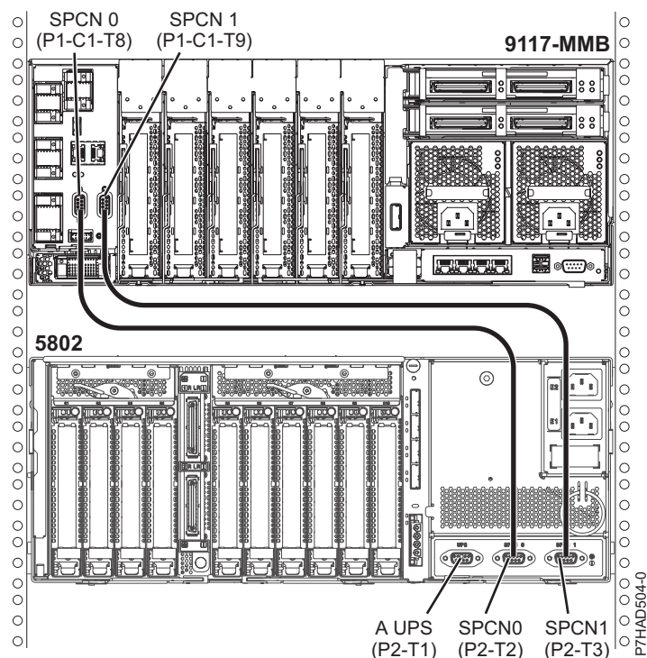
Figura 131. Vista posterior de 8412-EAD, 9117-MMB, 9117-MMC, 9117-MMD, 9179-MHB, 9179-MHC, 9179-MHD y 5208 o 5877 con la ubicación de instalación de los cables
