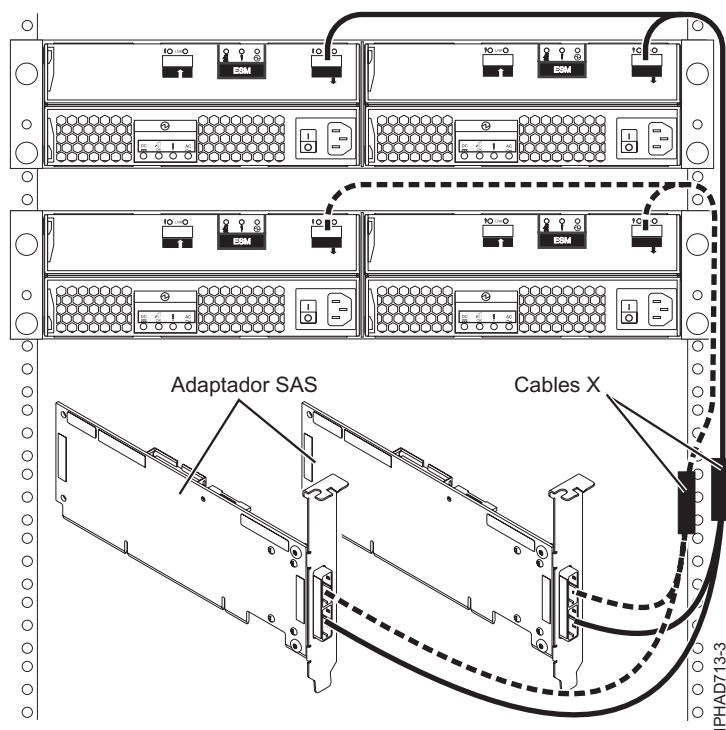
Figura 132. Conexión de dos adaptadores RAID SAS con dos cajones de expansión de disco en una configuración RAID HA de multi-iniciador.
