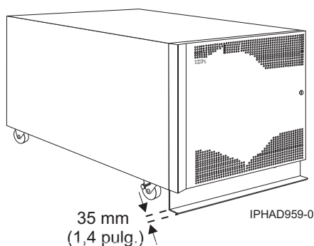
Figura 4. Modelo 0554 y 7014-S11 con barra estabilizadora
