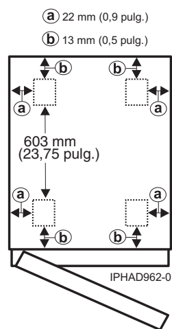
Figura 6. Ubicación de las ruedas giratorias del modelo 0554 y 7014-S11
