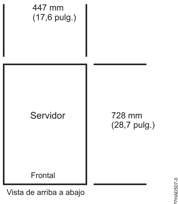
Figura 1. Vista de planificación de los modelos 8246-L1C, 8246-L1D, 8246-L1S, 8246-L1T, 8246-L2C, 8246-L2D, 8246-L2S y 8246-L2T (servidor montado en bastidor)
