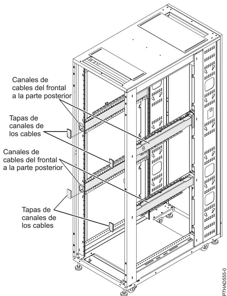
Figura 13. Cableado dentro del bastidor
