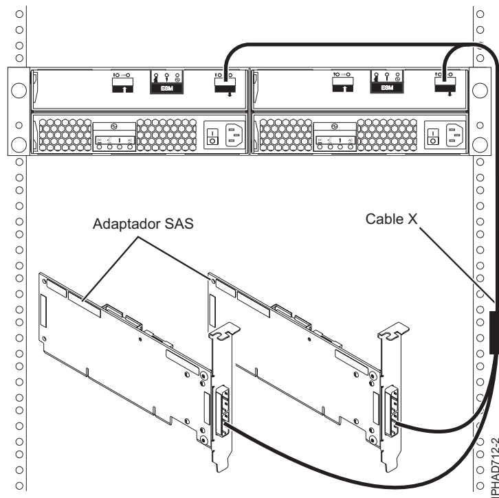
Figura 131. Conexión de dos adaptadores RAID SAS con un cajón de expansión de disco en una configuración RAID HA de multi-iniciador.
