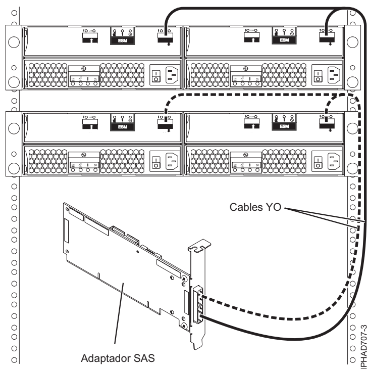
Figura 123. Conexión de un adaptador SAS con dos cajones de expansión de disco
