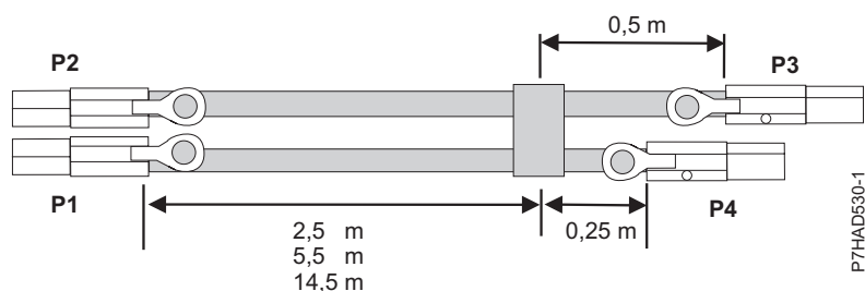
Figura 119. Longitudes de cable de conjunto de cables X SAS externos
