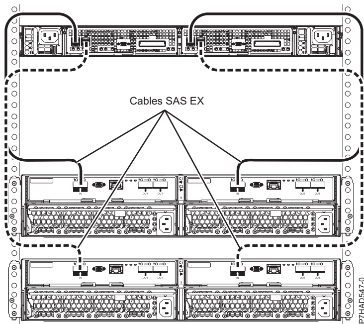
Figura 155. Conexión de dos cajones 5887 mediante cables HD EX con un EDR1
