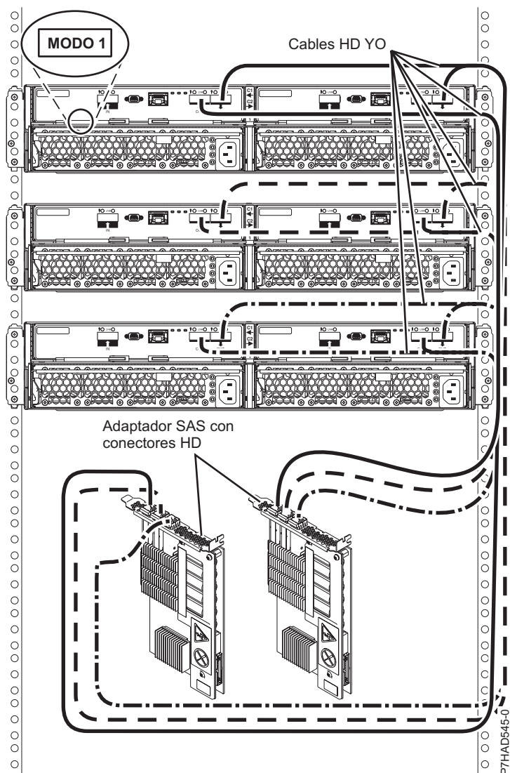
Figura 152. Conexión de modalidad 1 de tres cajones 5887 a dos adaptadores SAS con conectores HD
