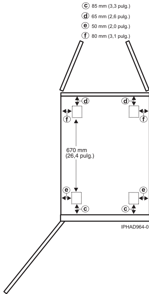
Figura 9. Ubicación de las ruedas giratorias del modelo 0555 y 7014-S25
