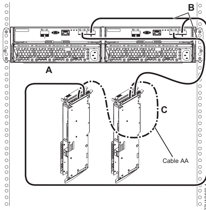
Figura 149. Conexión de modalidad 1 de un cajón 5887 mediante cables YO a adaptadores SAS duales
