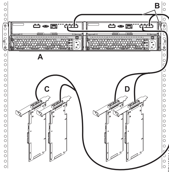
Figura 144. Conexión de modalidad 2 de un cajón 5887 mediante cables X a dos pares de adaptadores SAS
