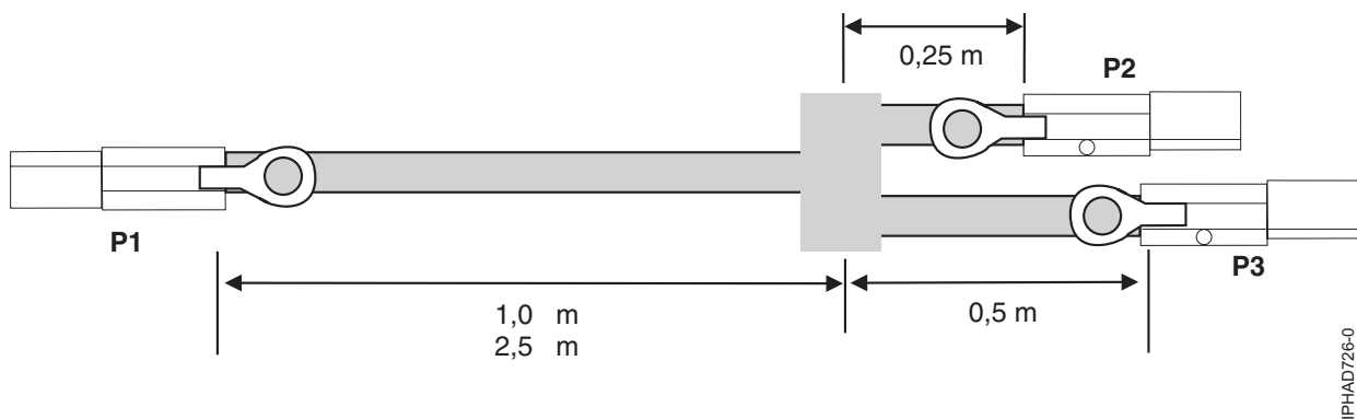
Figura 121. Longitudes de cable de conjunto de cables YI SAS externos
