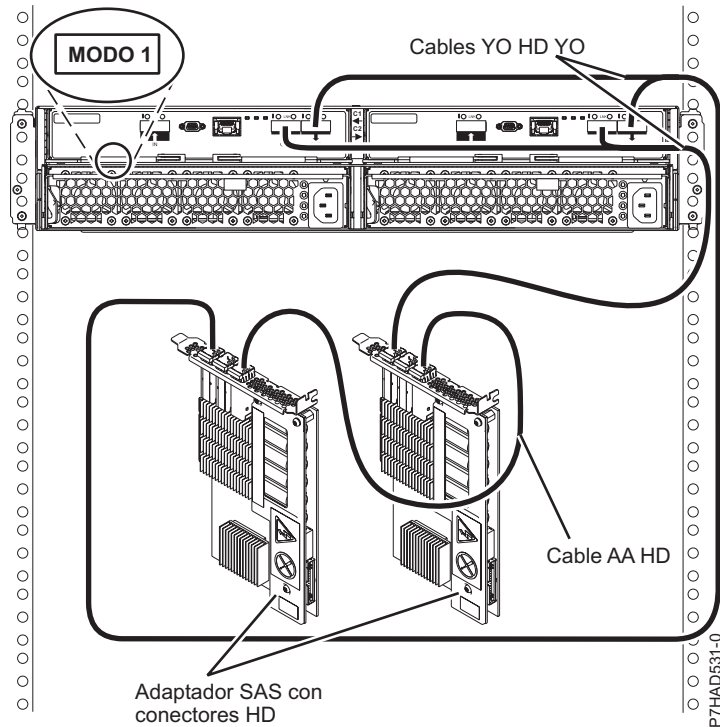
Figura 150. Conexión de modalidad 1 de un cajón 5887 a dos adaptadores SAS con conectores HD
