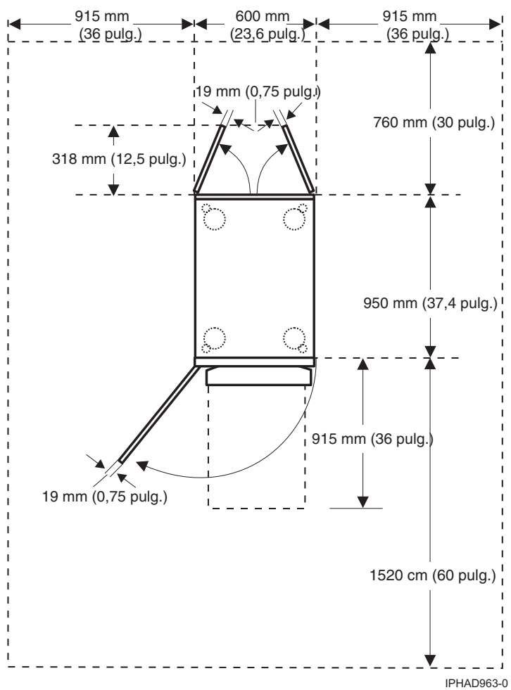
Figura 8. Vista de planta del modelo 0555 y 7014-S25
