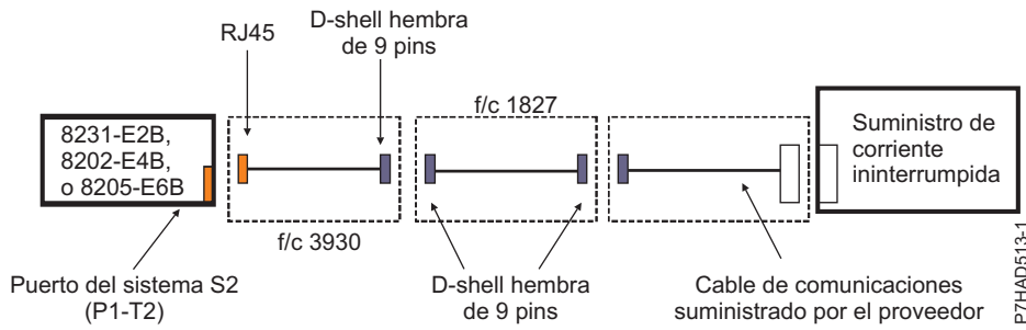
Figura 115. Conexión del sistema de alimentación ininterrumpible para 8246-L1C, 8246-L1S, 8246-L2C, y 8246-L2S
