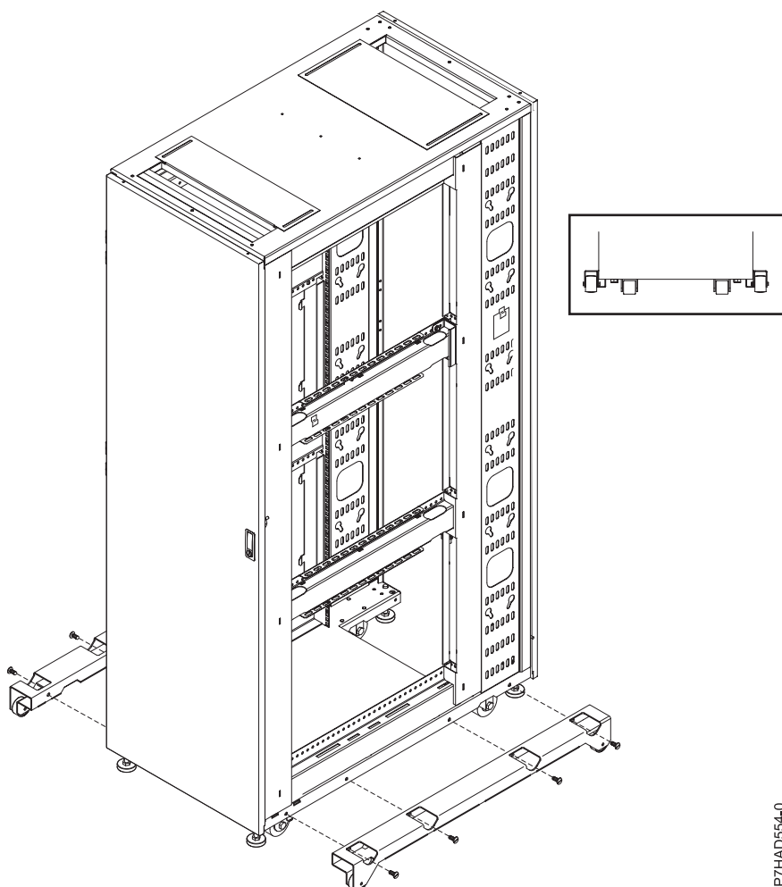
Figura 16. Ubicaciones del estabilizador
