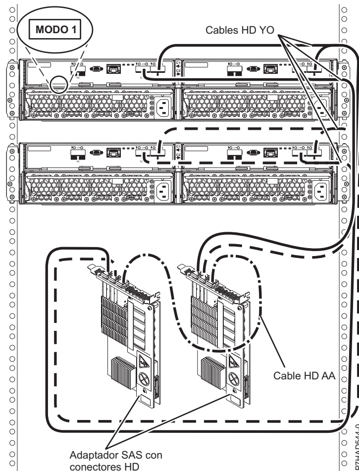
Figura 151. Conexión de modalidad 1 de dos cajones 5887 mediante conectores HD a dos adaptadores SAS
