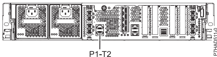
Figura 114. Vista posterior de , 8246-L1C, 8246-L1D, 8246-L1S, 8246-L1T, 8246-L2C, 8246-L2D, 8246-L2S y 8246-L2T con la ubicación de instalación de los cables
