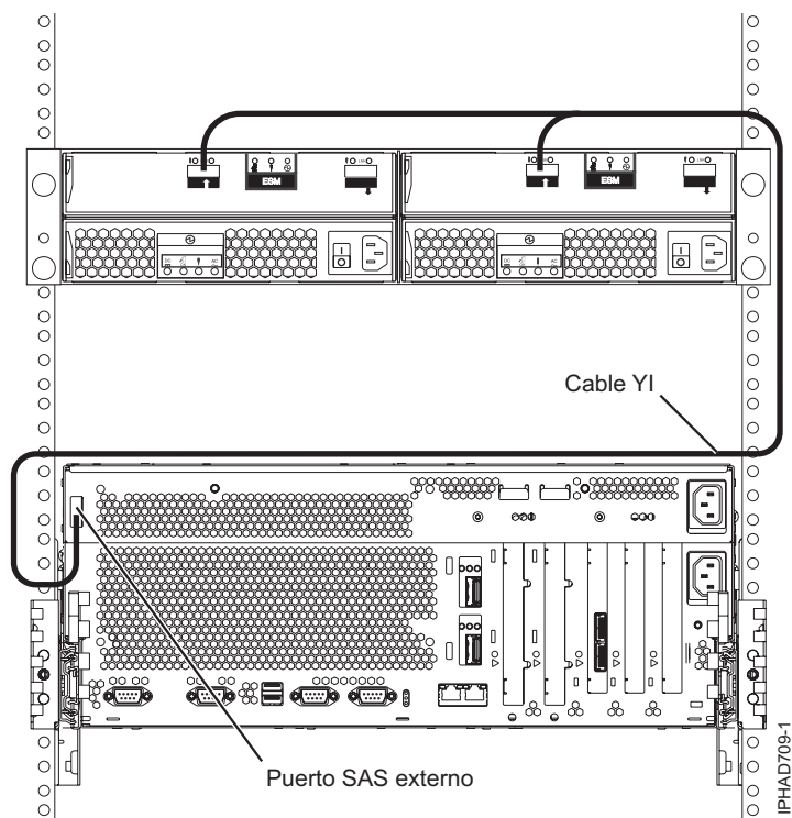
Figura 128. Conexión de un puerto de adaptador SAS externo del sistema con un cajón de expansión de disco
