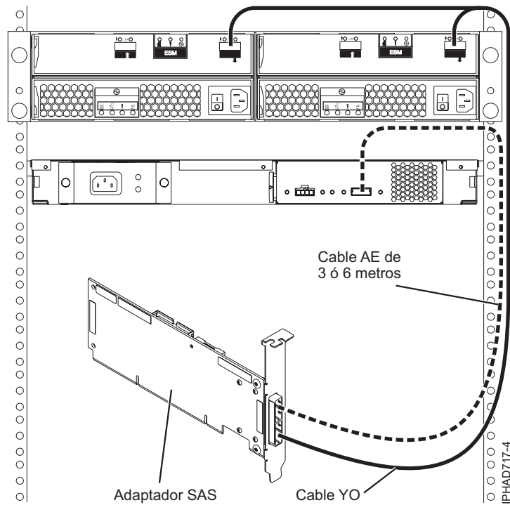
Figura 127. Conexión de un adaptador SAS con un cajón de expansión de disco y con un cajón de expansión de soporte
