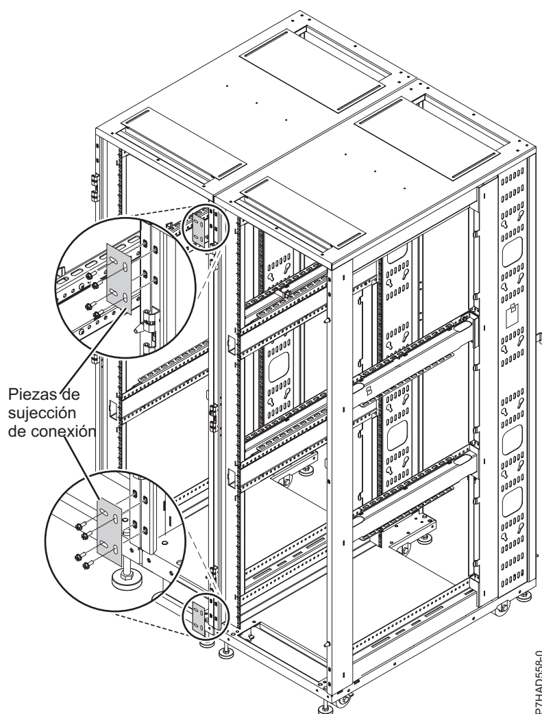
Figura 17. Piezas de sujeción de conexión
