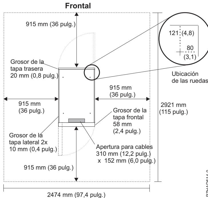
Figura 11. Ubicación de las ruedas giratorias y espacios libres de servicio de los bastidores 7014-T00, 7014-T42 y 0553
