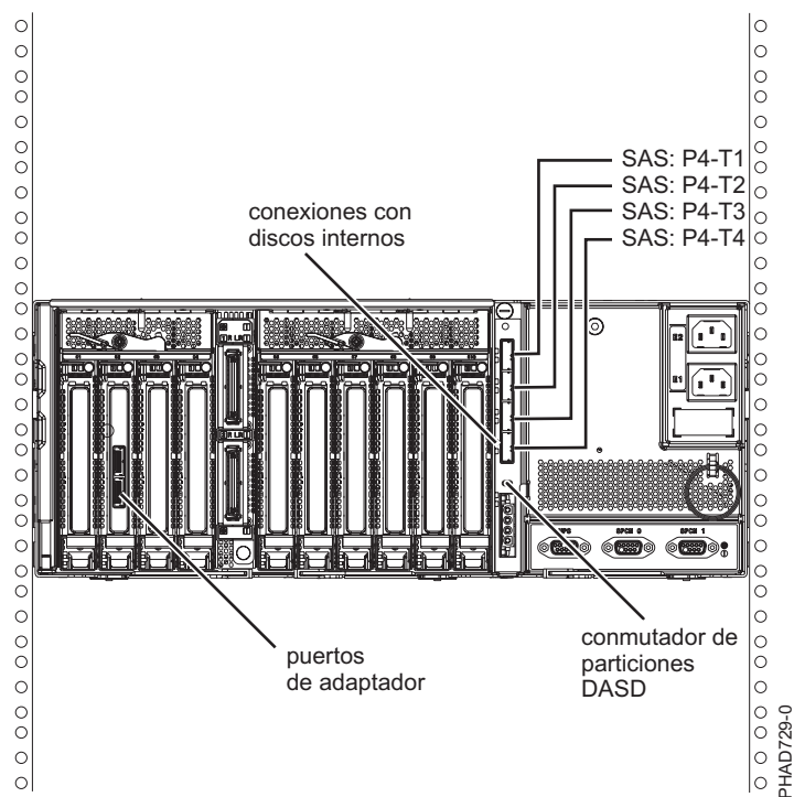
Figura 140. Conexión de dos adaptadores RAID SAS con un cajón de expansión de disco en una configuración JBOD HA de multi-iniciador.
