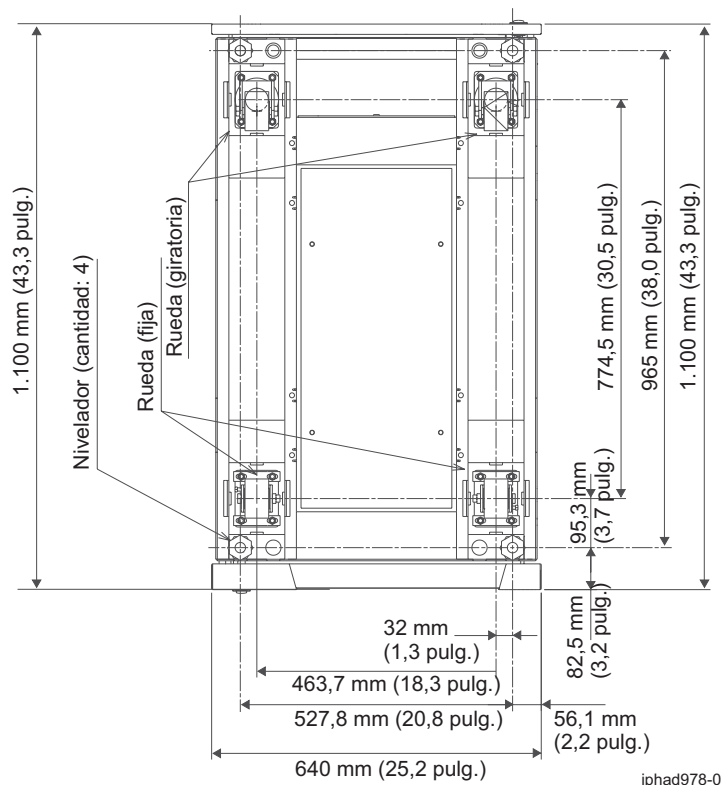
Figura 10. Ubicaciones de ruedas giratorias y niveladores
