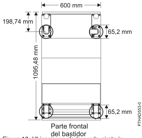
Figura 12. Ubicaciones de la rueda giratoria
