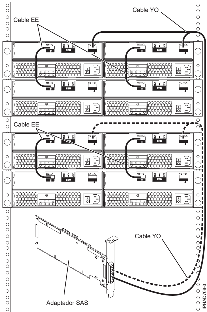
Figura 124. Conexión de un adaptador SAS con cuatro cajones de expansión de disco
