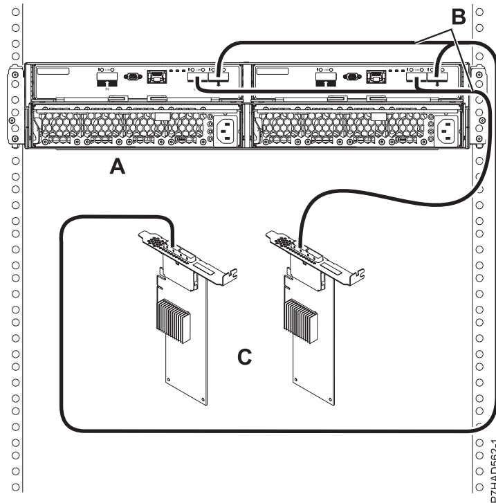
Figura 142. Conexión de modalidad 1 de un cajón 5887 mediante cables YO a adaptadores SAS duales
