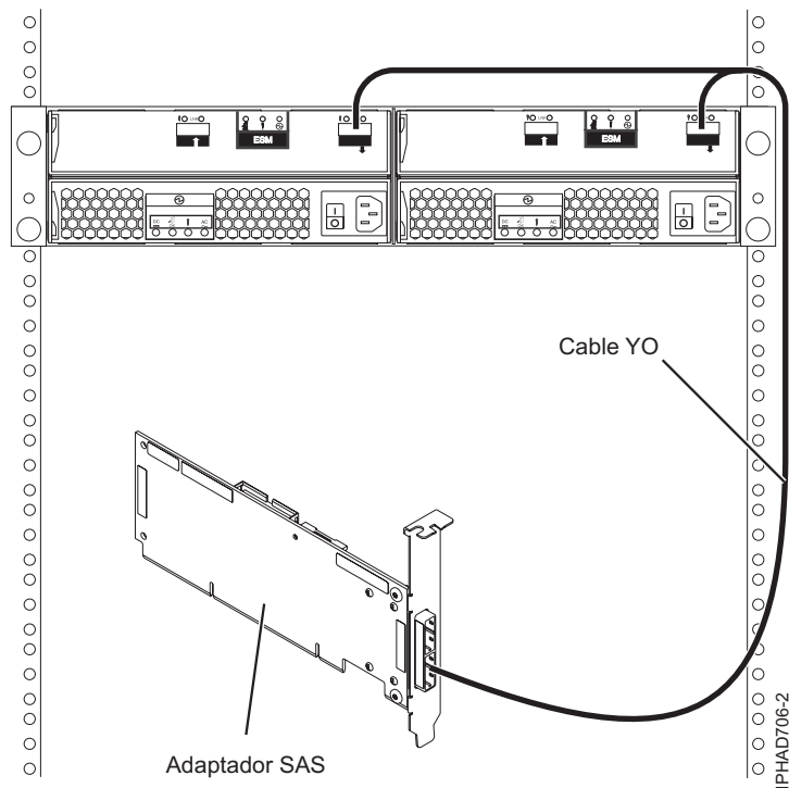
Figura 122. Conexión de un adaptador SAS con un cajón de expansión de disco
