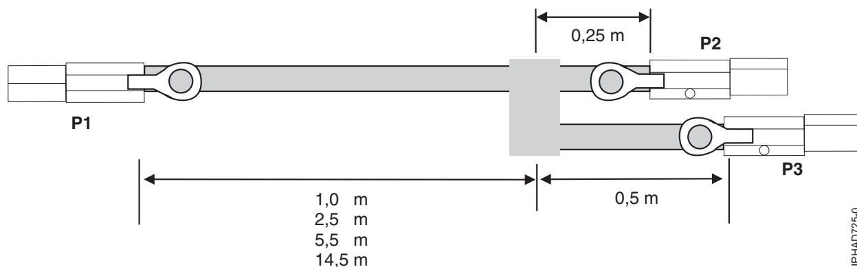
Figura 120. Longitudes de cable de conjunto de cables YO SAS externos
