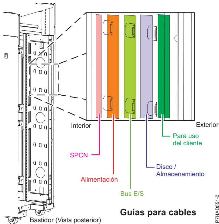
Figura 116. Lanzas puente portacables
