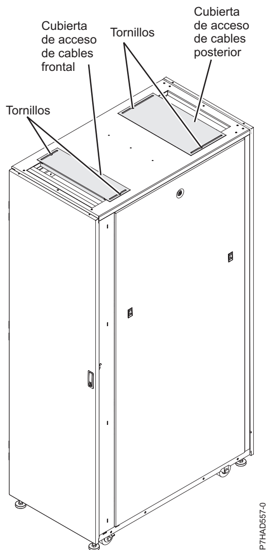
Figura 15. Cubiertas de acceso de cables
