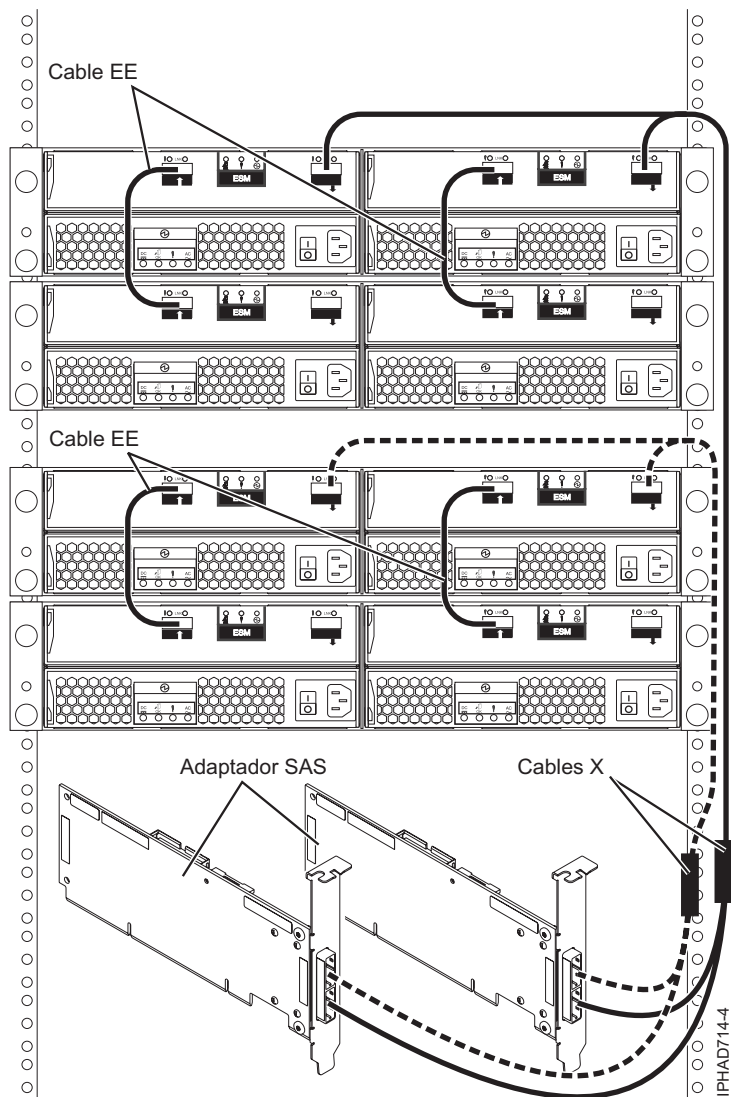
Figura 133. Conexión de dos adaptadores RAID SAS con cuatro cajones de expansión de disco en una configuración RAID HA de multi-iniciador
