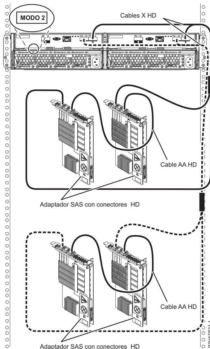
Figura 153. Conexión de modalidad 2 de un cajón 5887 mediante conectores HD a dos pares de adaptadores SAS
