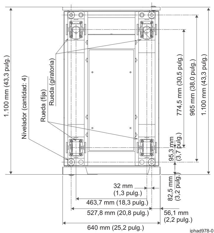
Figura 3. Ubicaciones de ruedas giratorias y niveladores
