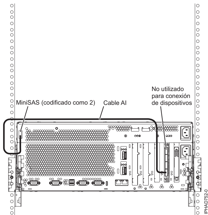
Figura 130. Adaptador FC5904 o FC5908 conectado a cajones de expansión de disco
