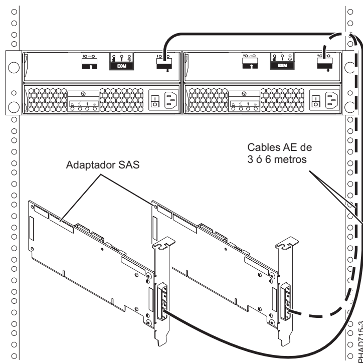
Figura 139. Conexión de dos adaptadores RAID SAS con un cajón de expansión de disco en una configuración JBOD HA de multi-iniciador.
