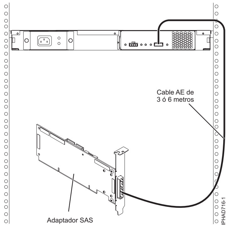
Figura 126. Conexión de un adaptador SAS con un cajón de expansión de soporte
