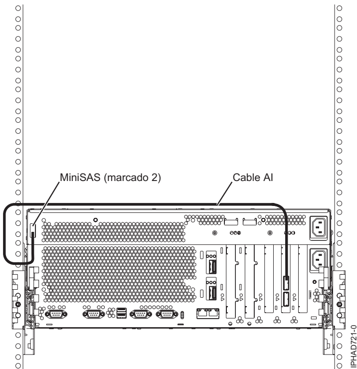
Figura 129. Conexión de un adaptador SAS con ranuras de disco SAS internas mediante el puerto SAS externo del sistema
