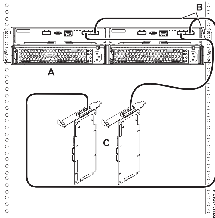
Figura 146. Conexión de modalidad 1 de un cajón 5887 mediante cables YO a adaptadores SAS duales
