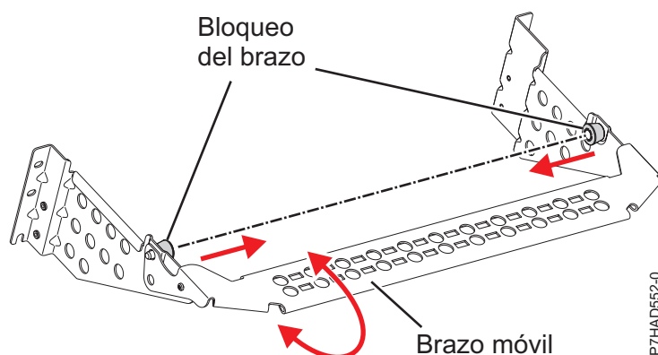
Figura 118. Abrazadera portacables
