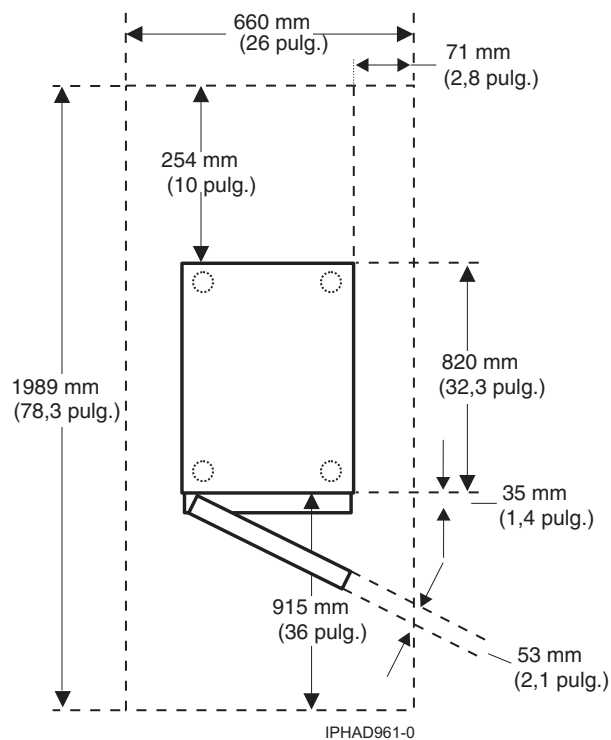
Figura 5. Vista de planta del modelo 0554 y 7014-S11
