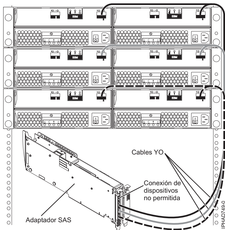
Figura 125. Conexión de adaptador SAS de tres puertos con cajones de expansión de disco
