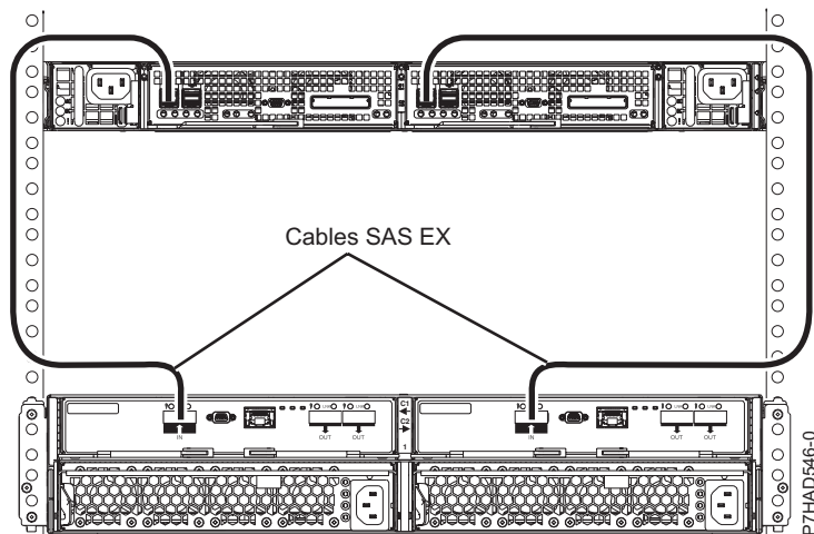
Figura 154. Conexión de un cajón 5887 mediante cables HD EX con un EDR1
