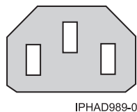
Figura 107. Tipo de receptáculo 15
