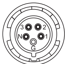
Figura 32. Sujeción de enchufe
