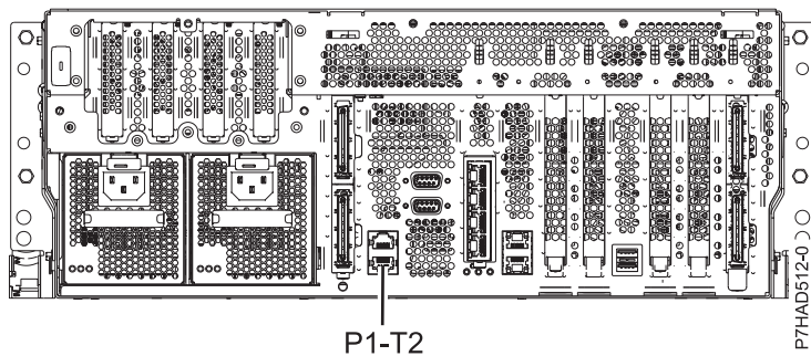
Figura 133. Vista posterior de 8202-E4B, 8202-E4C, 8202-E4D, 8205-E6B, 8205-E6C y 8205-E6D con la ubicación de instalación de los cables
