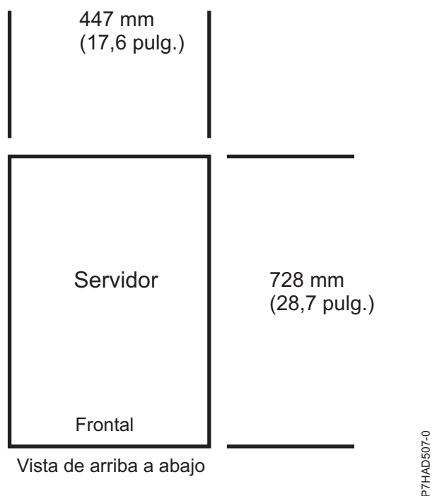
Figura 1. Vista de planificación de los modelos 8231-E2B, 8231-E1C, 8231-E1D, 8231-E2C, 8231-E2D y 8268-E1D (servidor montado en bastidor)
