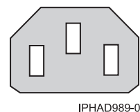
Figura 82. Tipo de receptáculo 26
