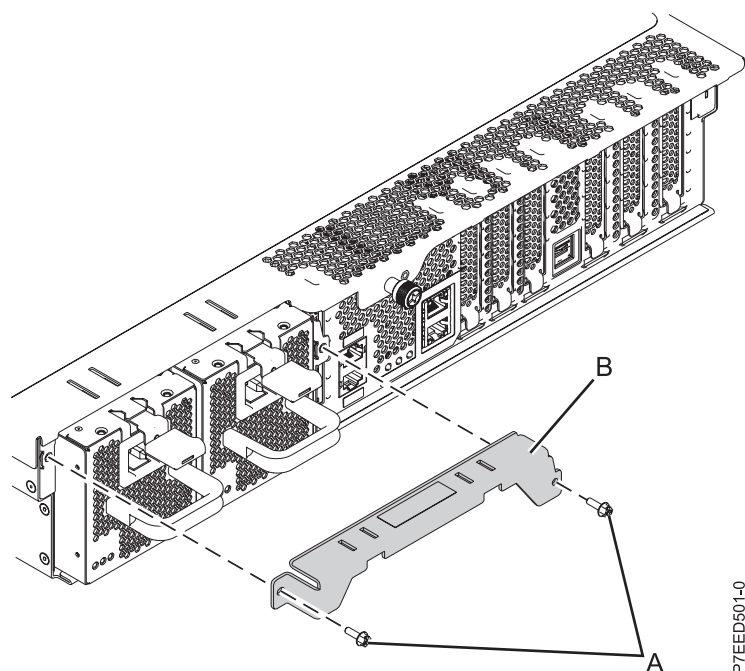
Figura 10. Extracción de la abrazadera de transporte
