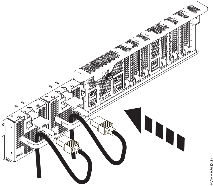
Figura 20. Cómo hacer pasar y conectar el cable de alimentación
