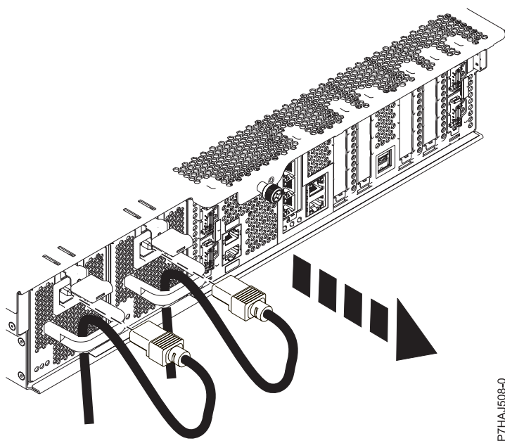
Figura 9. Extracción de los cables de alimentación
