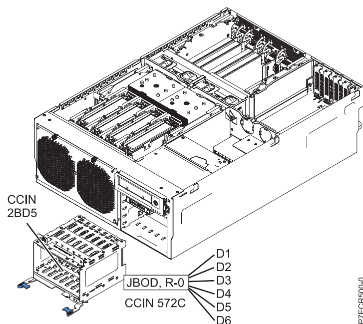
Figura 4. Bahías de disco controladas por la placa posterior base
