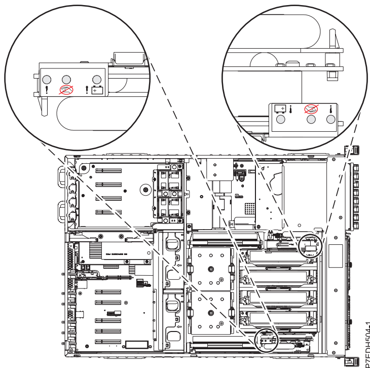
Figura 9. LED de datos de memoria caché presentes
