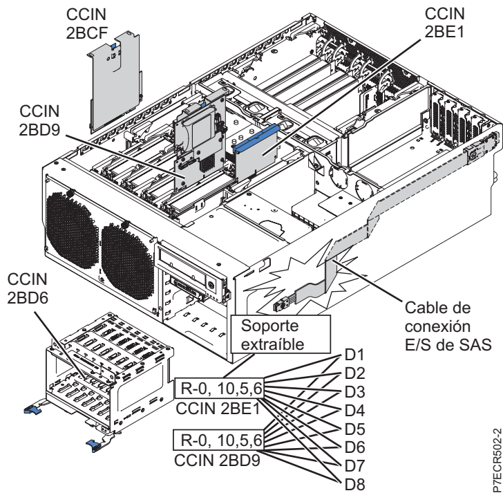
Figura 7. Bahías de disco controladas por ambos adaptadores SAS incorporados cuando se utiliza el subsistema dual-RAID SAS con unidades externas
