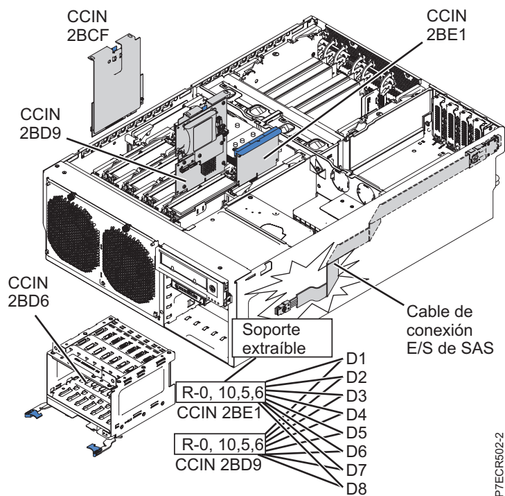
Figura 6. Bahías de disco controladas por ambos adaptadores SAS incorporados cuando se utiliza el subsistema dual-RAID SAS con unidades internas
