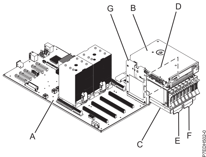
Figura 2. Visión general de la placa posterior de unidad dividida en dos vías SAS
