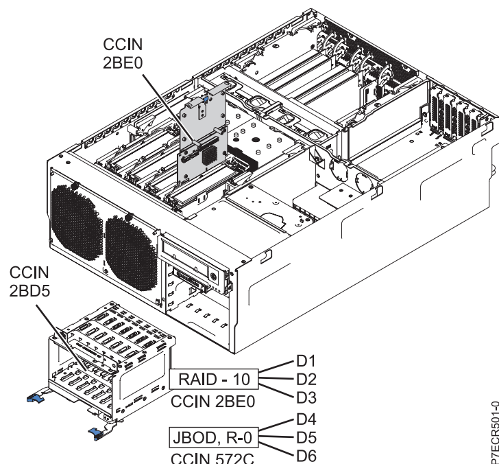
Figura 5. Adaptador SAS incorporado en una placa posterior de unidad dividida en dos vías
