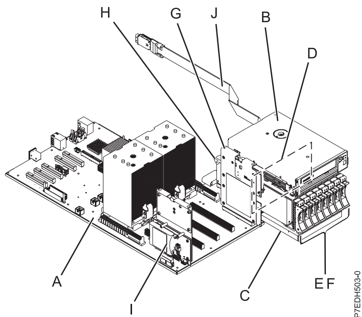
Figura 3. Visión general del subsistema dual-RAID SAS
