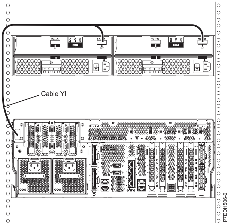
Figura 8. Conexión física para conectar alojamientos de discos externos
