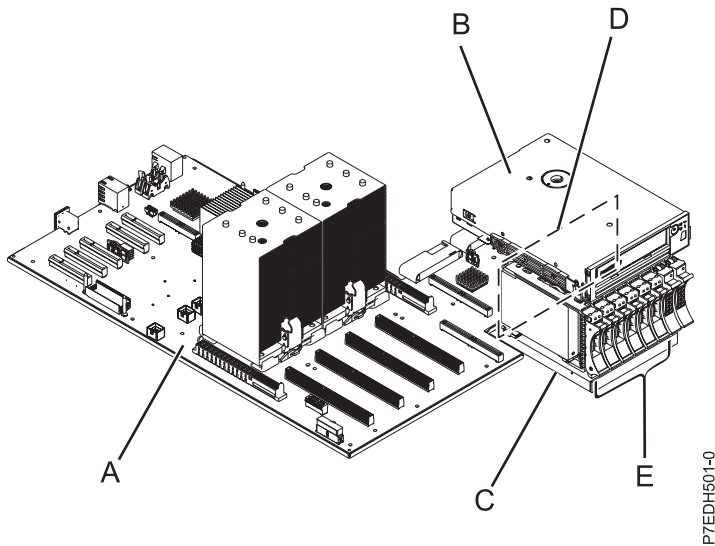
Figura 1. Visión general del subsistema base SAS
