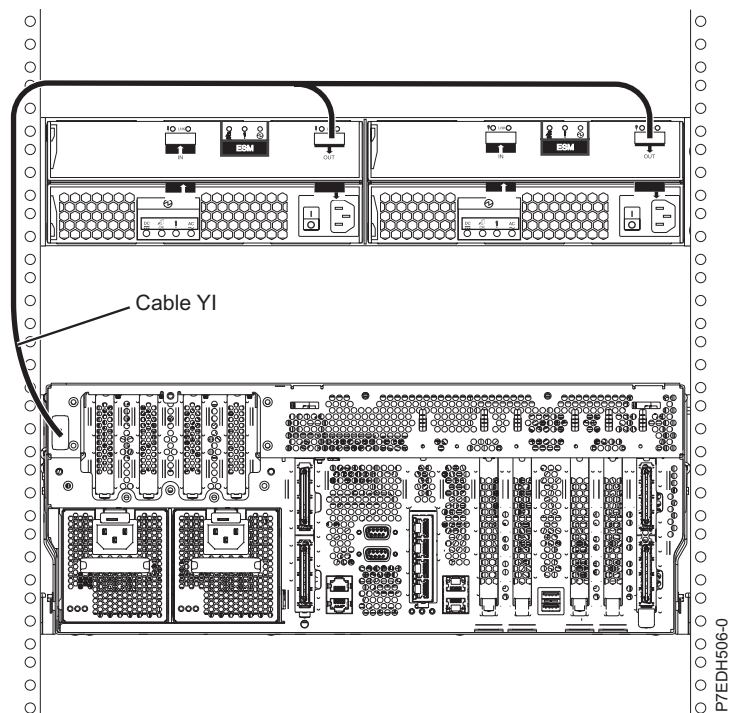
Figura 8. Conexión física para conectar un alojamiento de unidad de disco 5886
