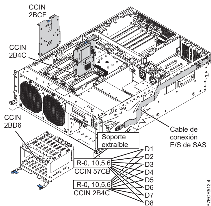
Figura 7. Bahías de discos controladas por ambos adaptadores SAS cuando se utiliza un subsistema dual-RAID SAS con unidades internas y externas
