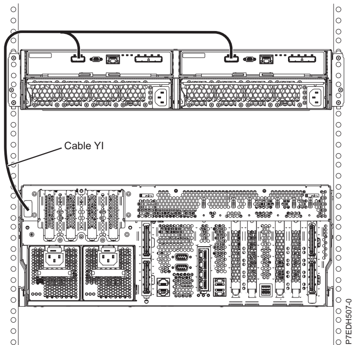
Figura 9. Conexión física para conectar un alojamiento de unidad de disco 5887
