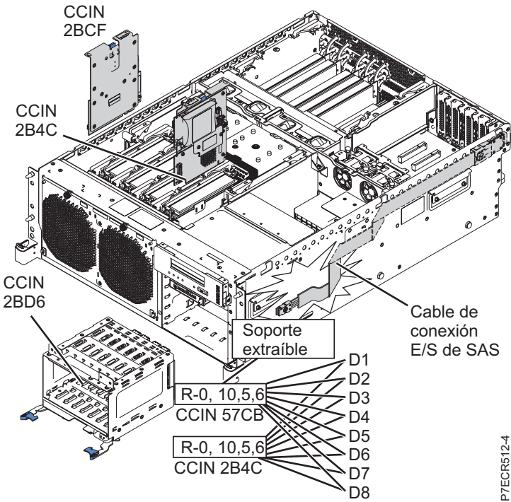
Figura 6. Bahías de disco controladas por ambos adaptadores SAS cuando se utiliza un subsistema dual-RAID SAS con unidades internas
