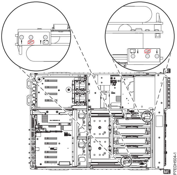
Figura 10. LED de datos de memoria caché presentes
