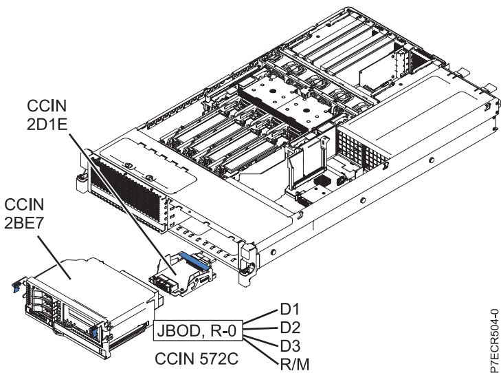
Figura 5. Configuración del subsistema SAS con almacenamiento en cinta
