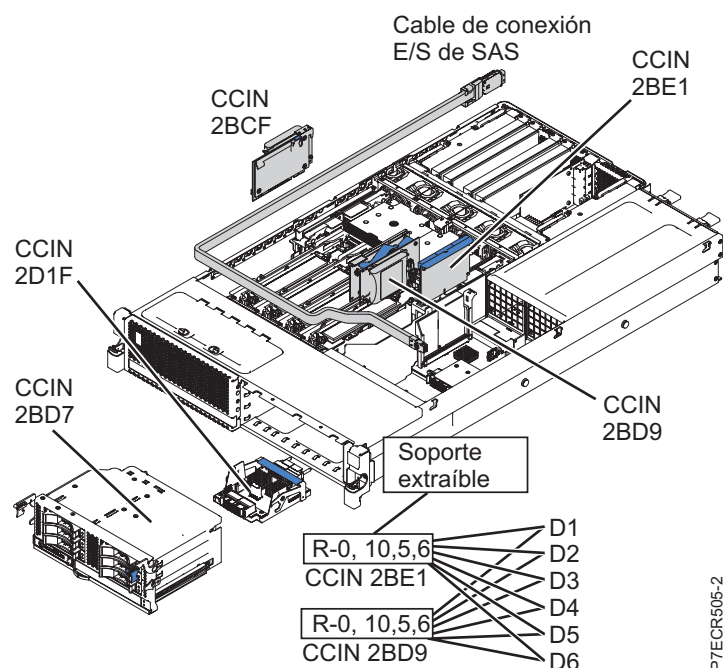
Figura 6. Bahías de disco controladas por los dos adaptadores SAS incluidos cuando se utiliza IOA de almacenamiento dual con unidades internas
