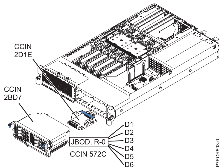
Figura 4. Bahías de disco controladas por la placa posterior del sistema base
