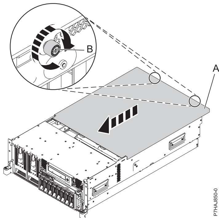
Figura 3. Instalación de la cubierta de acceso de servicio
