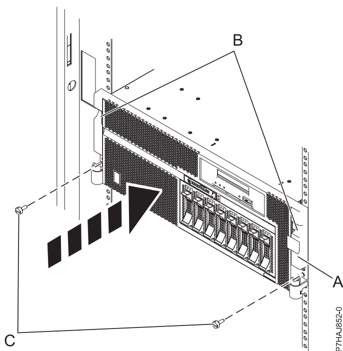
Figura 8. Volver a colocar los tornillos de mano
