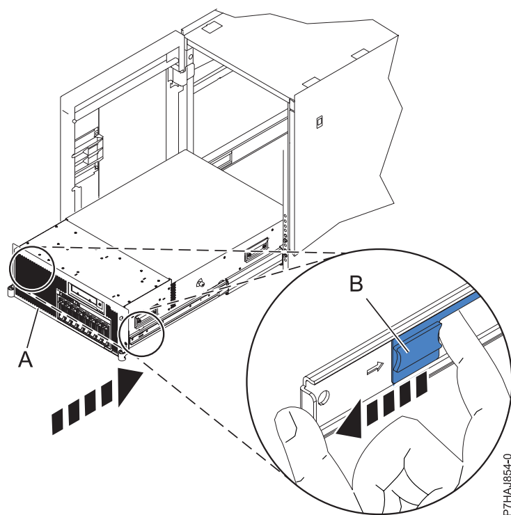
Figura 7. Liberación de los pestillos de seguridad de los rieles
