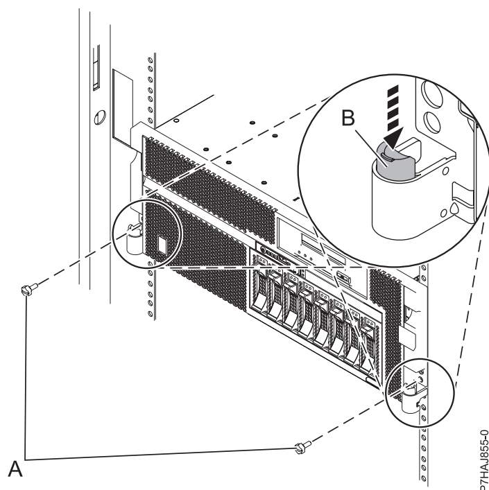
Figura 6. Cómo soltar los pestillos del bastidor
