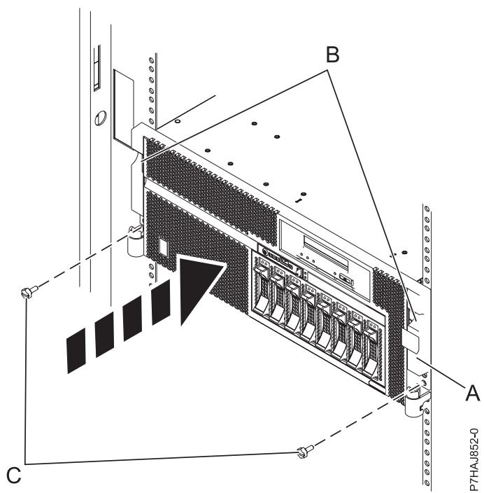
Figura 5. Instalación de la cubierta frontal
