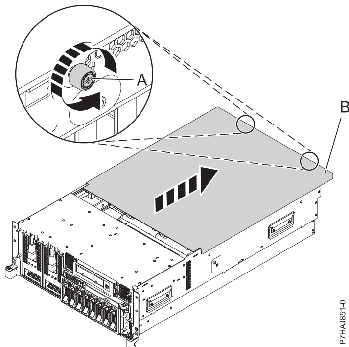
Figura 2. Quitar la cubierta de acceso de servicio
