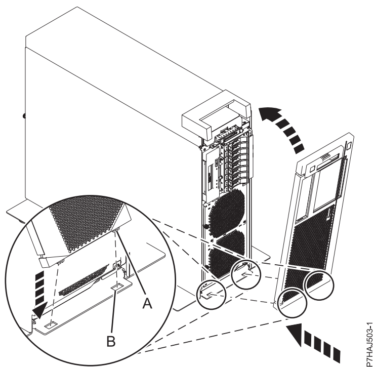
Figura 9. Instalar la cubierta frontal
