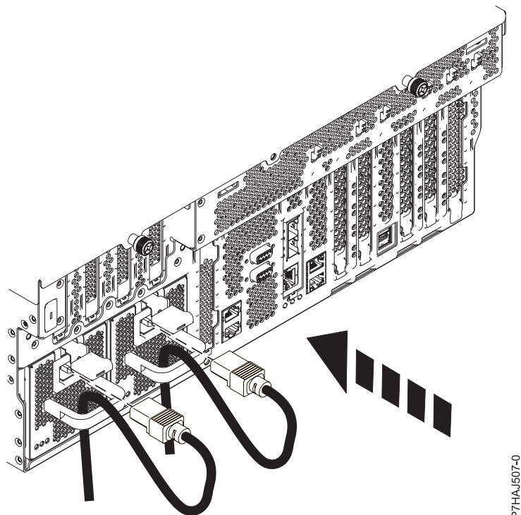
Figura 23. Conexión de los cables de alimentación
