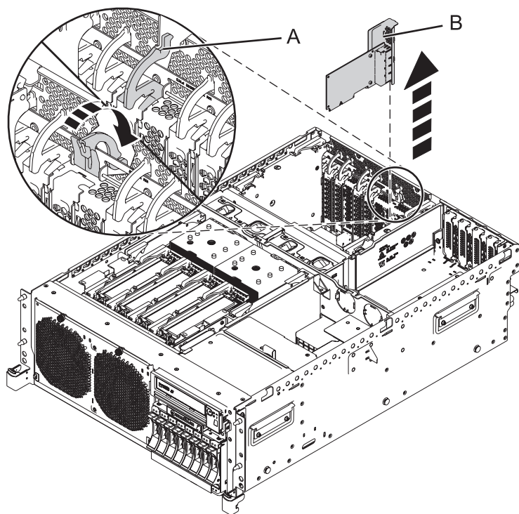
Figura 1. Extracción de un Adaptador Ethernet de sistema principal (1 GB o 10 GB) para 8202-E4B o 8205-E6B
