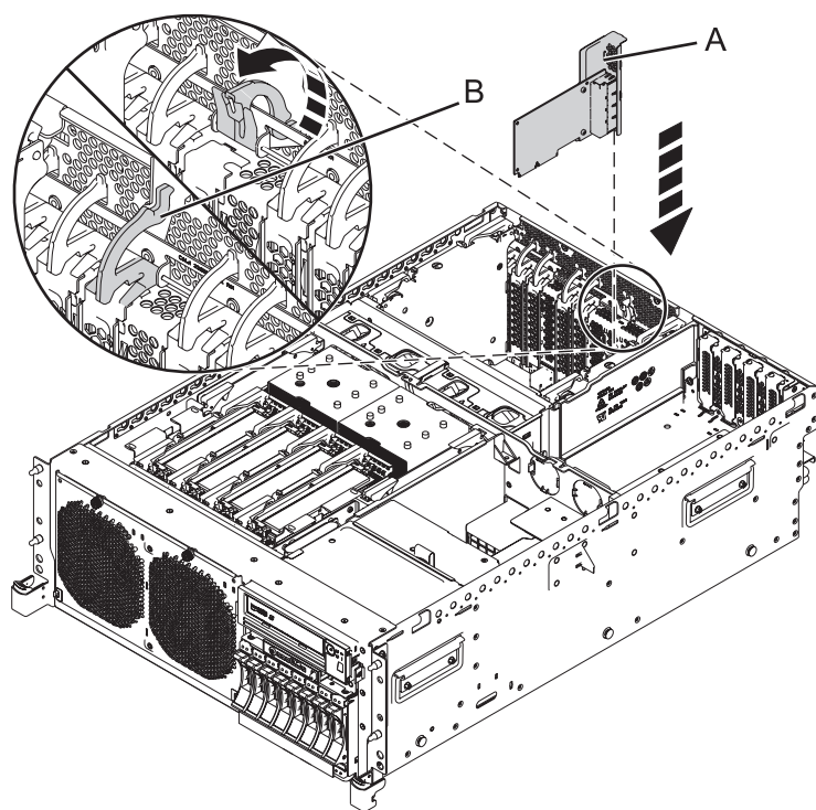
Figura 2. Instalar el Adaptador Ethernet de sistema principal (1 GB o 10 GB) en un modelo montado en bastidor para 8202-E4B o 8205-E6B
