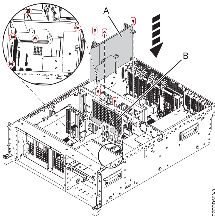
Figura 46. Sustitución de la cubierta protectora del receptáculo de la unidad de disco de 8202-E4B o 8205-E6B
