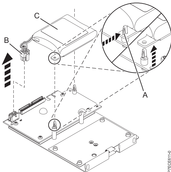
Figura 18. Extraer la batería de caché
