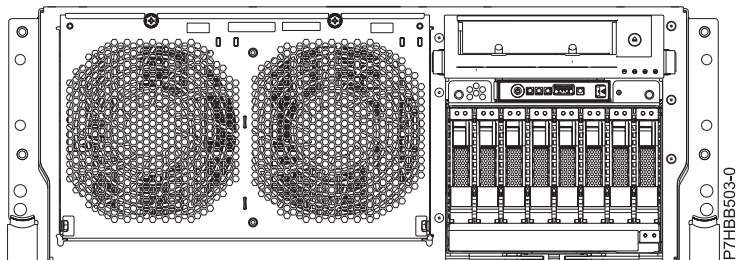
Figura 20. Placa posterior de la unidad de disco de un sistema montado en bastidor
