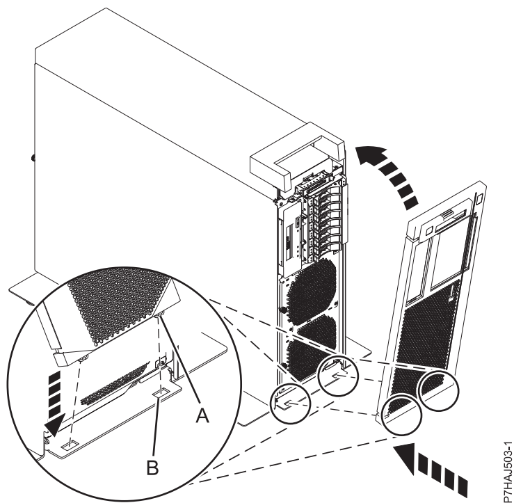
Figura 59. Instalar la cubierta frontal
