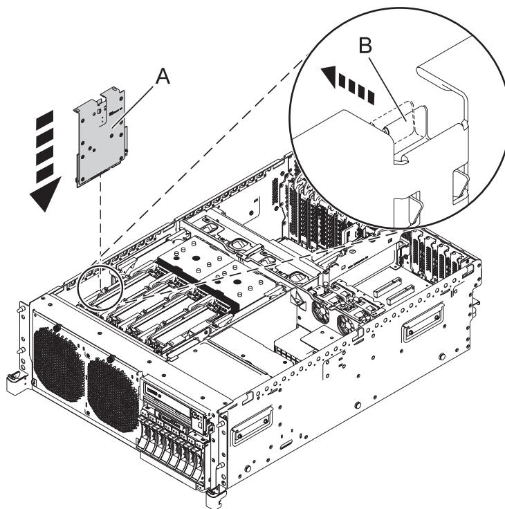
Figura 17. Instalar la tarjeta de la batería de caché
