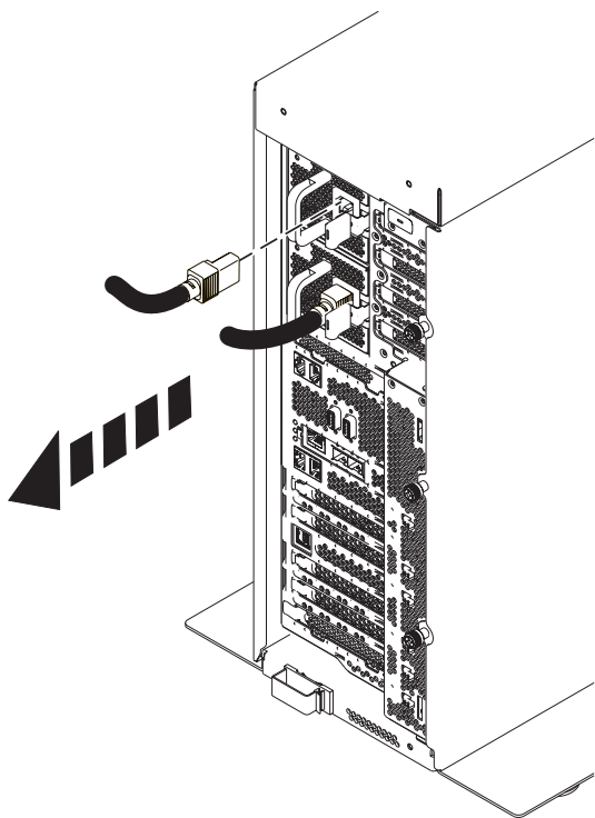
Figura 72. Quitar los cables de alimentación para un sistema autónomo
