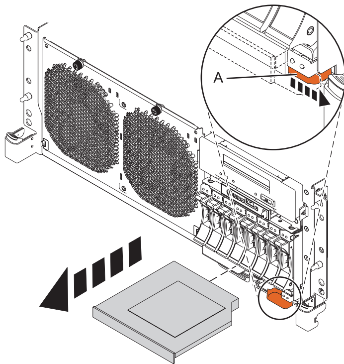
Figura 23. Extraer el dispositivo de soporte de la placa posterior de la unidad de disco
