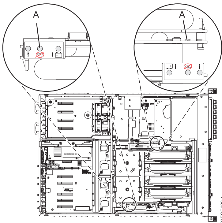
Figura 15. LED de presencia de datos de caché
