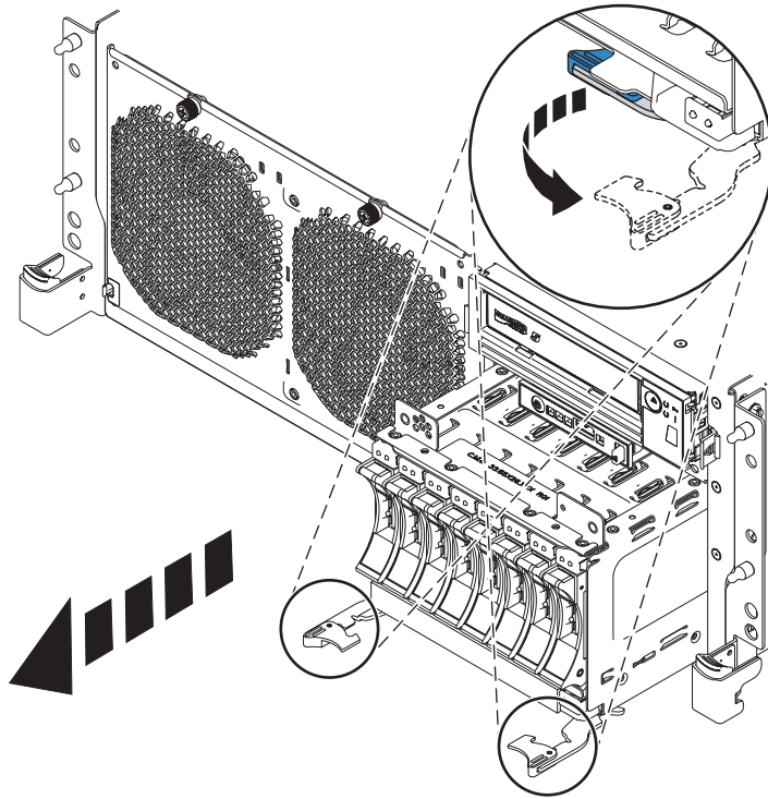
Figura 31. Extraer el receptáculo de la unidad de disco
