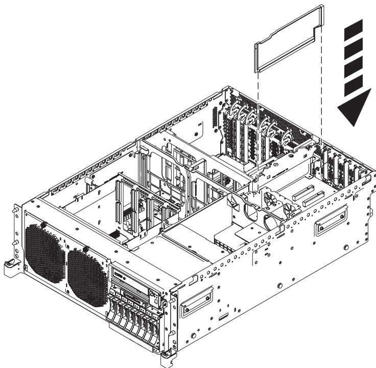
Figura 49. Sustituir el separador de aire de la tarjeta de expansión PCI
