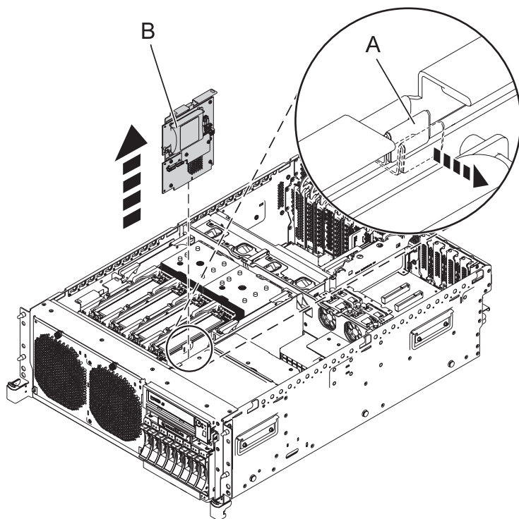
Figura 13. Extracción del controlador de almacenamiento RAID/caché de una unidad del sistema montada en bastidor
