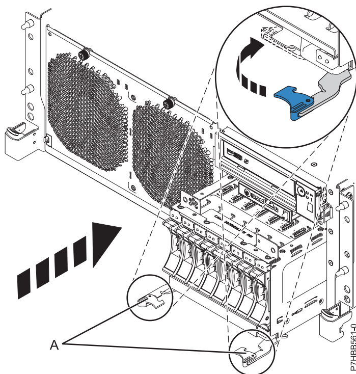
Figura 27. Instalación de la placa posterior con unidades de disco en un modelo montado en bastidor
