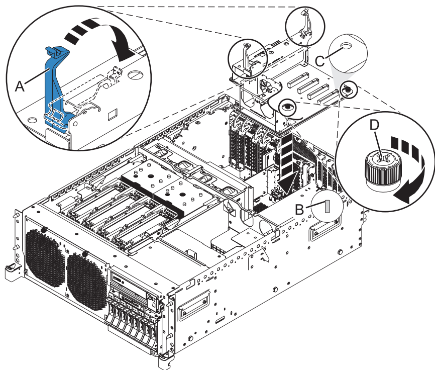
Figura 48. Sustituir la tarjeta de expansión PCI
