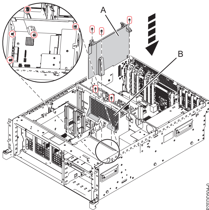
Figura 47. Sustitución de la cubierta protectora del receptáculo de la unidad de disco de 8202-E4C, 8202-E4D, 8205-E6C o 8205-E6D
