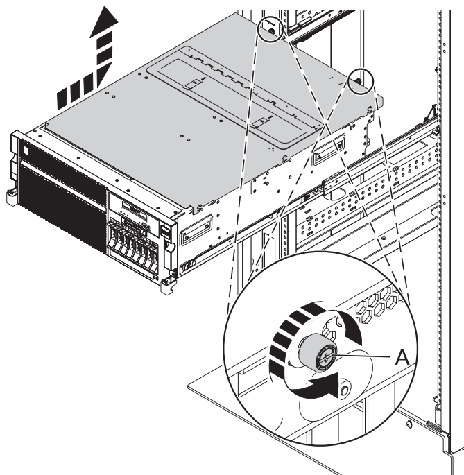
Figura 61. Extraer la cubierta de acceso de servicio
