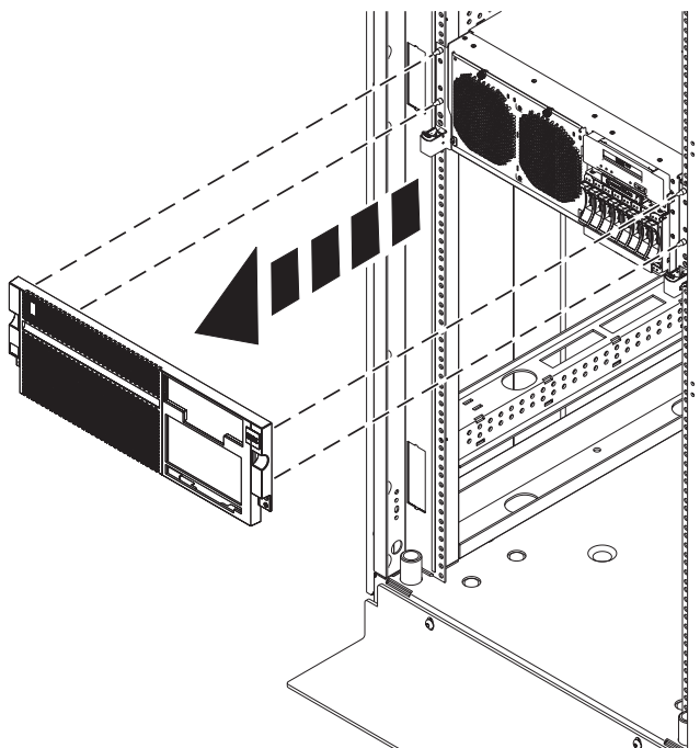
Figura 56. Extraer la cubierta frontal
