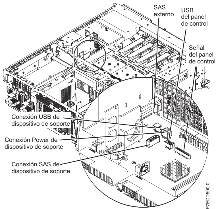
Figura 30. Desconectar los cables internos
