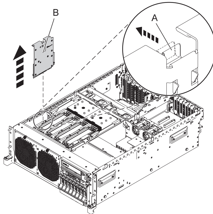
Figura 16. Extraer la tarjeta de la batería de caché
