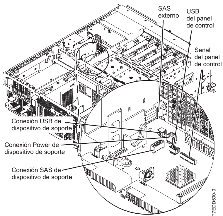
Figura 51. Conectar los cables internos
