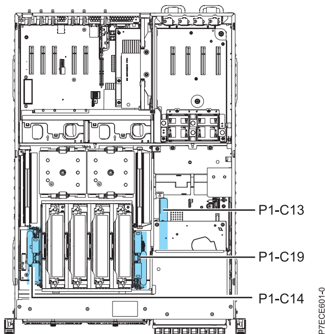
Figura 10. Ubicación de la ranura de la tarjeta de habilitación RAID (P1-C13)
