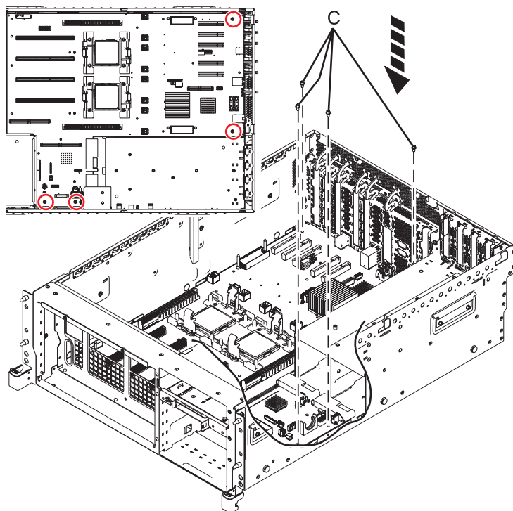
Figura 42. Instalar la placa posterior del sistema
