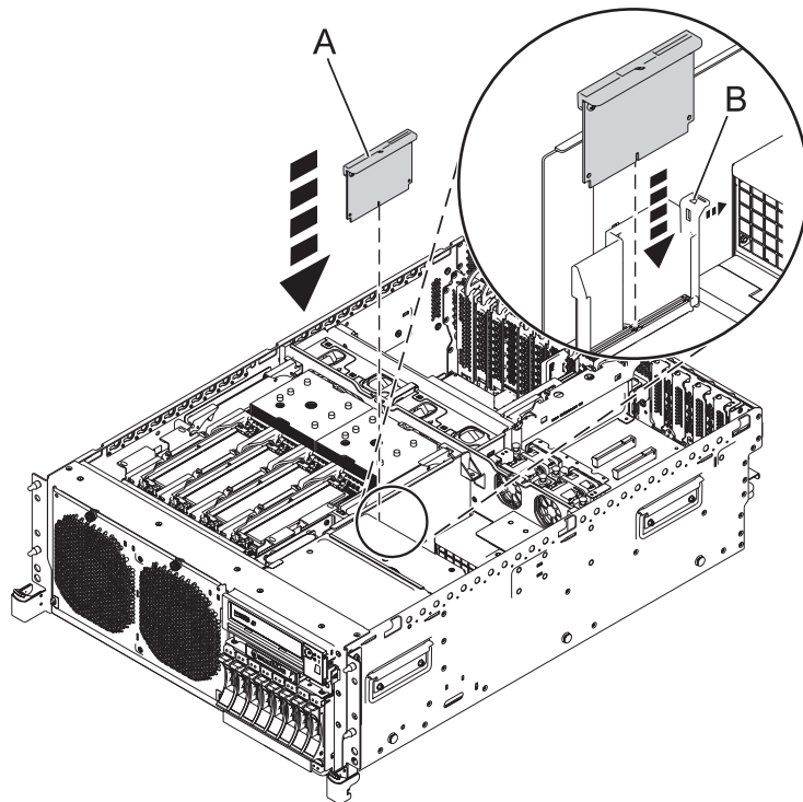
Figura 12. Sustitución de la tarjeta de habilitación RAID en una unidad del sistema montada en bastidor
