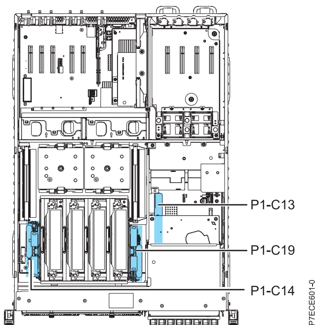
Figura 5. Ubicación de la ranura de la tarjeta de habilitación RAID, el controlador de almacenamiento RAID/caché y la tarjeta de batería de caché
