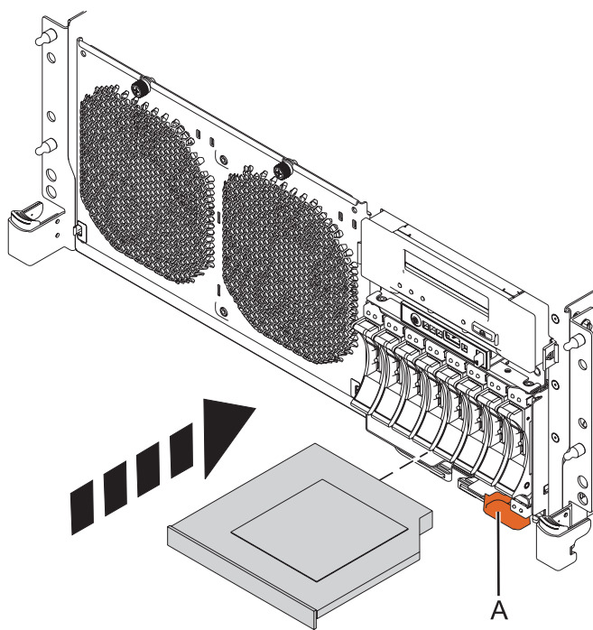
Figura 29. Instalar el dispositivo de soporte
