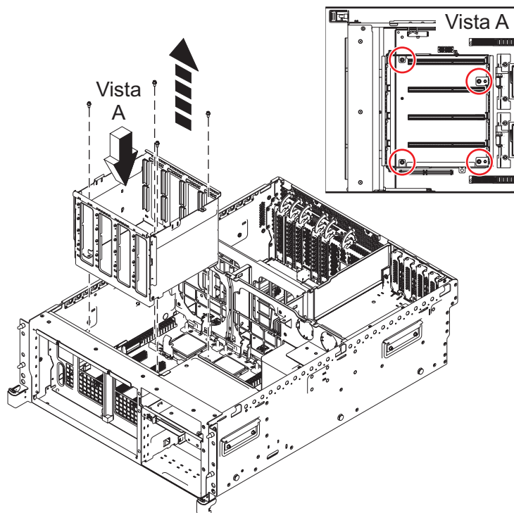
Figura 36. Extraer el receptáculo DIMM
