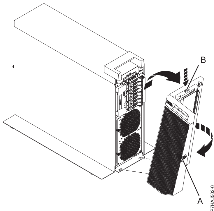
Figura 57. Extraer la cubierta frontal
