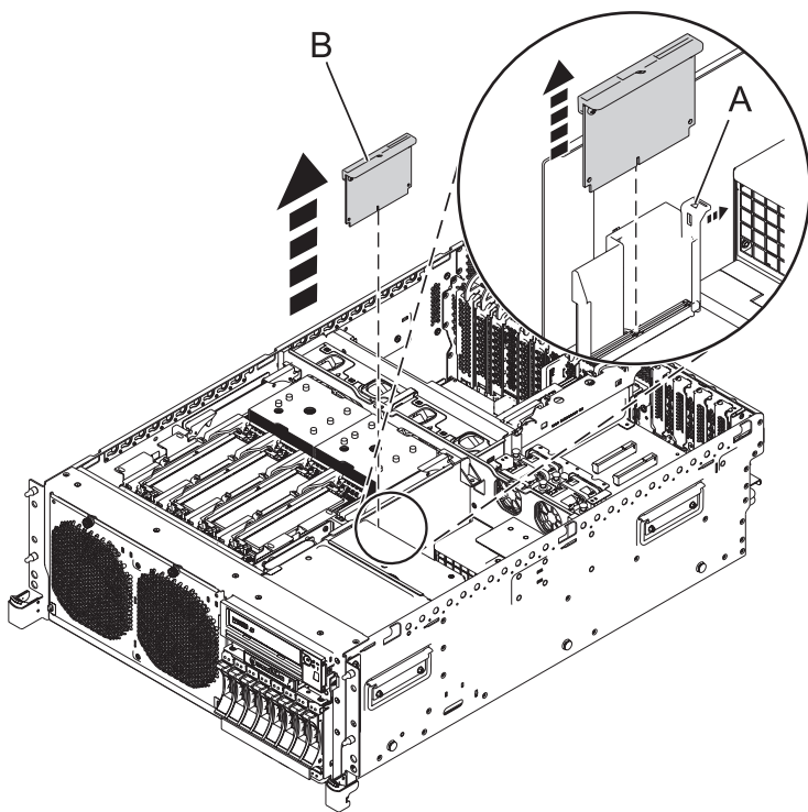
Figura 11. Extraer la tarjeta de habilitación RAID desde una unidad del sistema montada en bastidor
