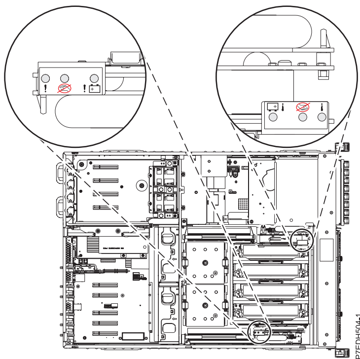
Figura 53. LED de presencia de datos de caché
