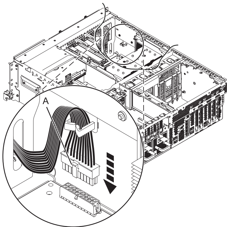
Figura 44. Conectar el cable del ventilador frontal
