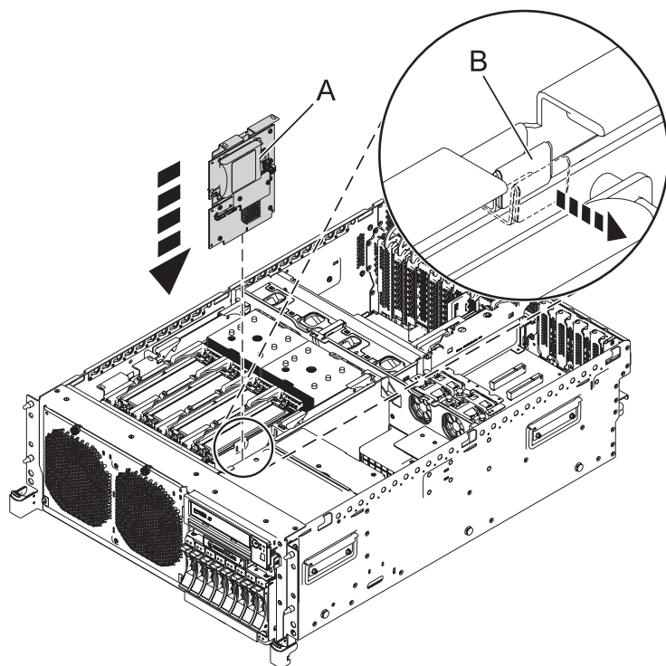
Figura 14. Sustitución del controlador de almacenamiento RAID/caché en una unidad del sistema montada en bastidor
