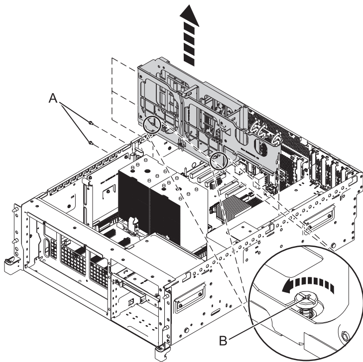
Figura 38. Extraer el receptáculo del ventilador central
