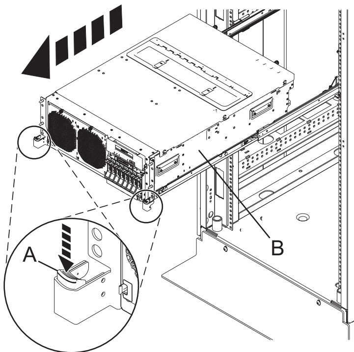
Figura 68. Bloquear la unidad del sistema en la posición de servicio
