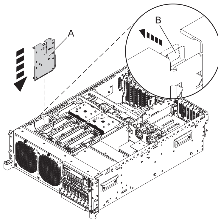
Figura 9. Sustitución de la tarjeta de batería de caché RAID de un modelo montado en bastidor
