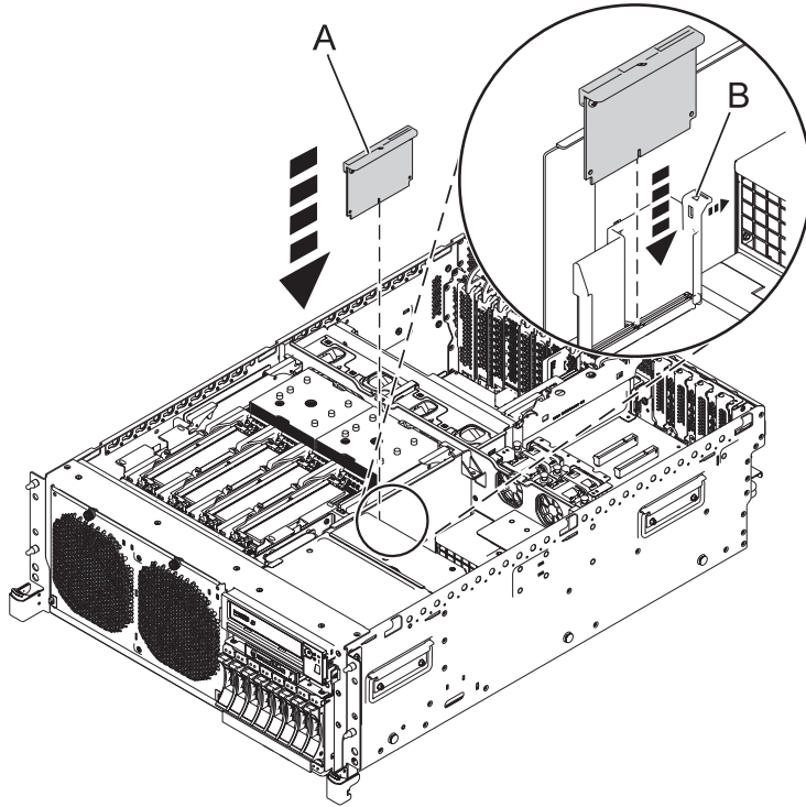
Figura 7. Sustitución de la tarjeta de habilitación RAID de un modelo montado en bastidor
