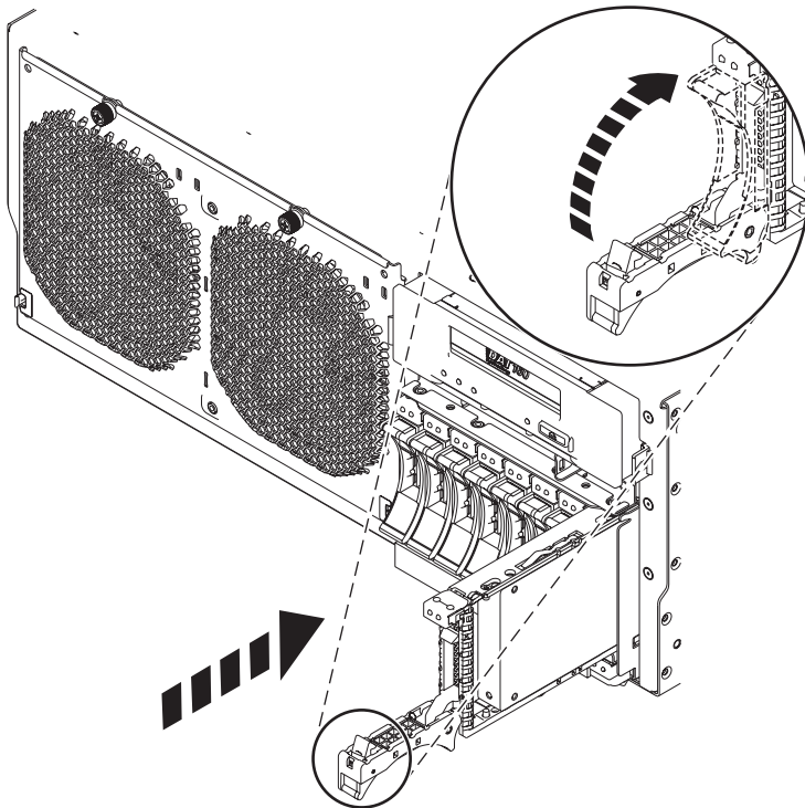
Figura 28. Instalar unidades de disco de la placa posterior
