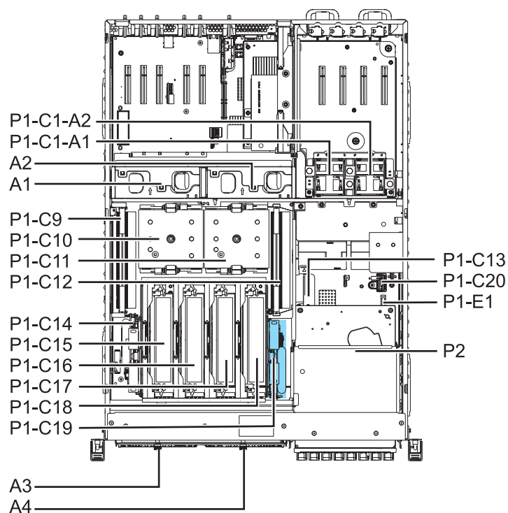
Figura 1. Ubicaciones de la ranura del controlador de almacenamiento RAID-10 (P1-C19) para 8202-E4B o 8205-E6B
