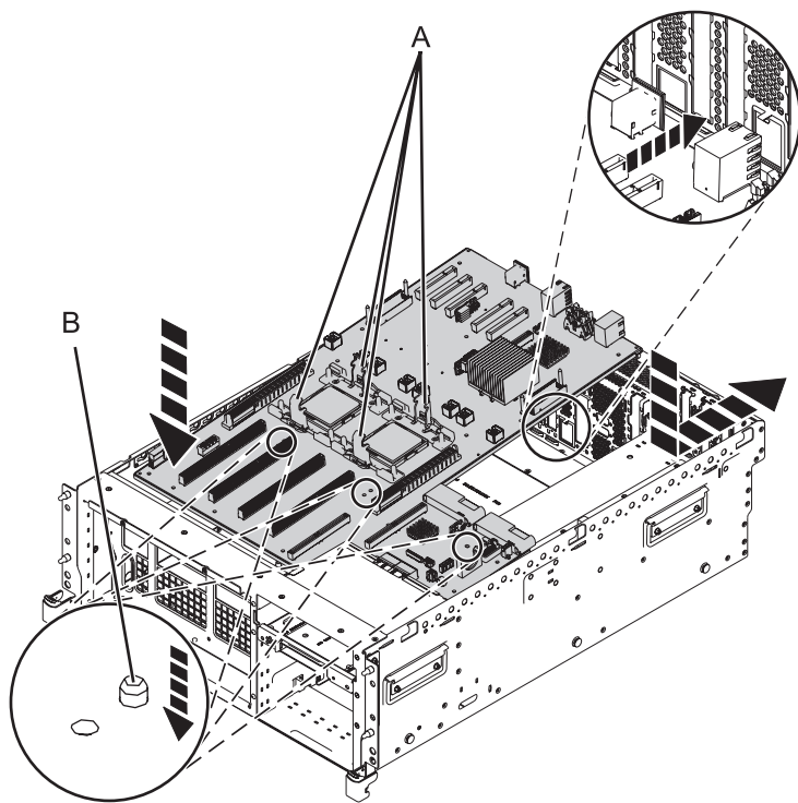
Figura 41. Instalación de la placa posterior del sistema en 8202-E4B o 8205-E6B
