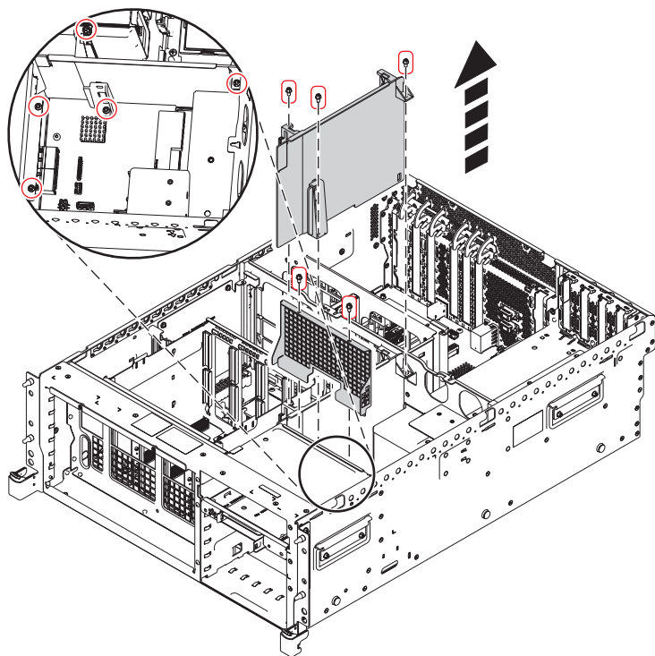
Figura 35. Extracción de la cubierta protectora del receptáculo de la unidad de disco de 8202-E4C, 8202-E4D, 8205-E6C o 8205-E6D
