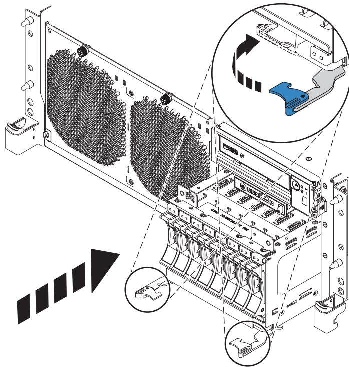
Figura 50. Sustituir el receptáculo de la unidad de disco
