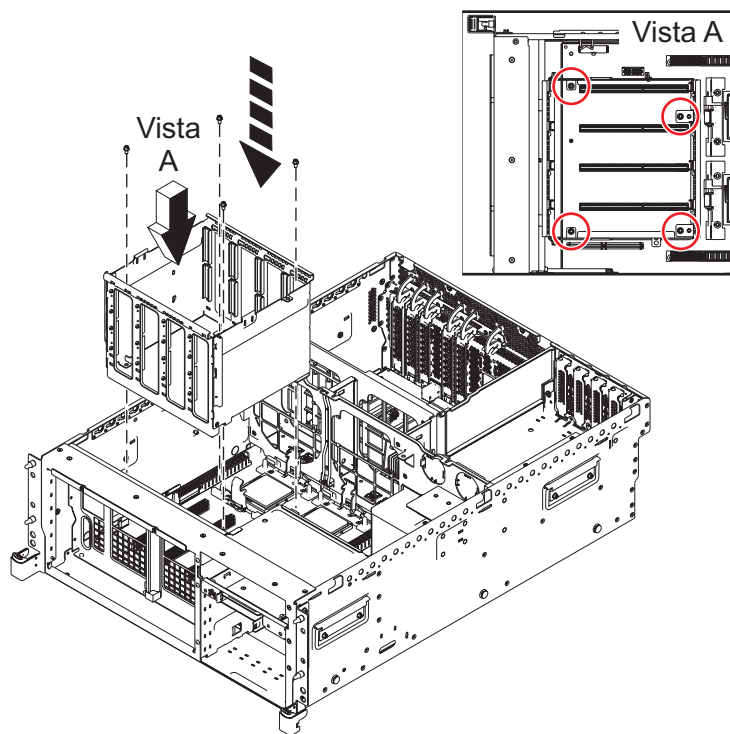
Figura 45. Sustituir el receptáculo DIMM
