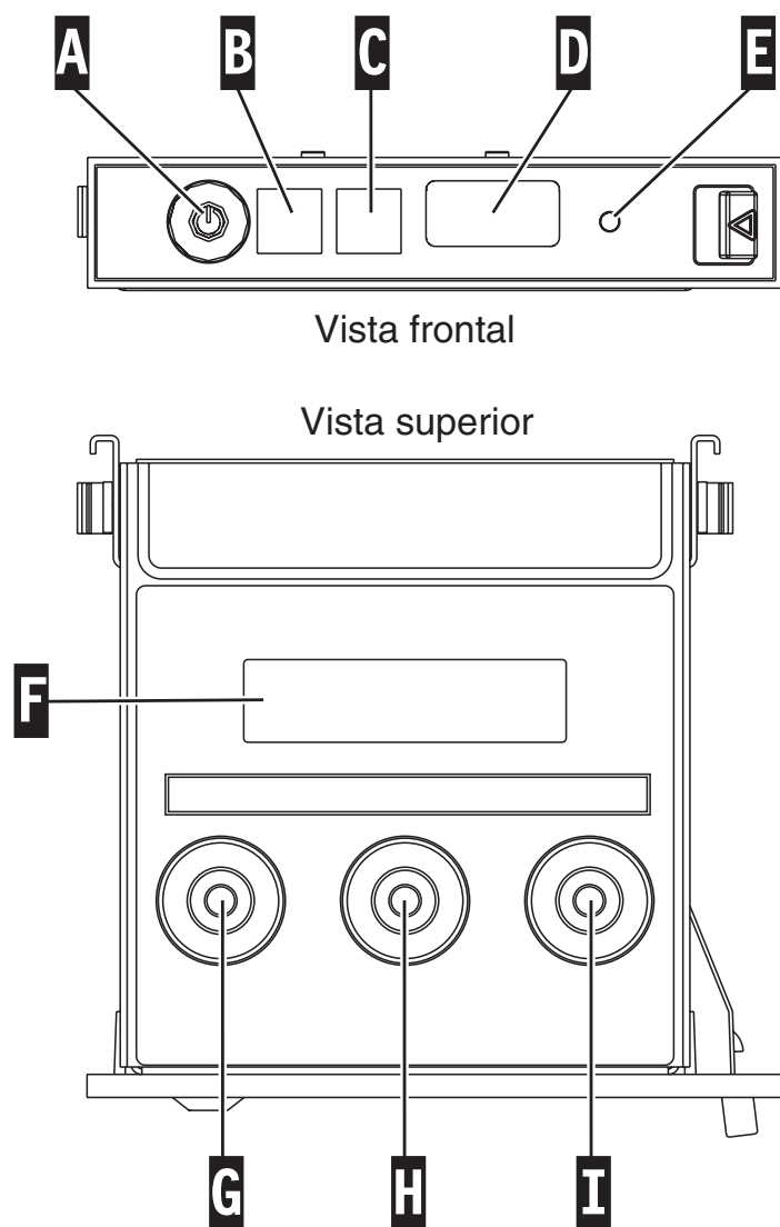
Figura 52. Conmutador pequeño del panel de información del operador
