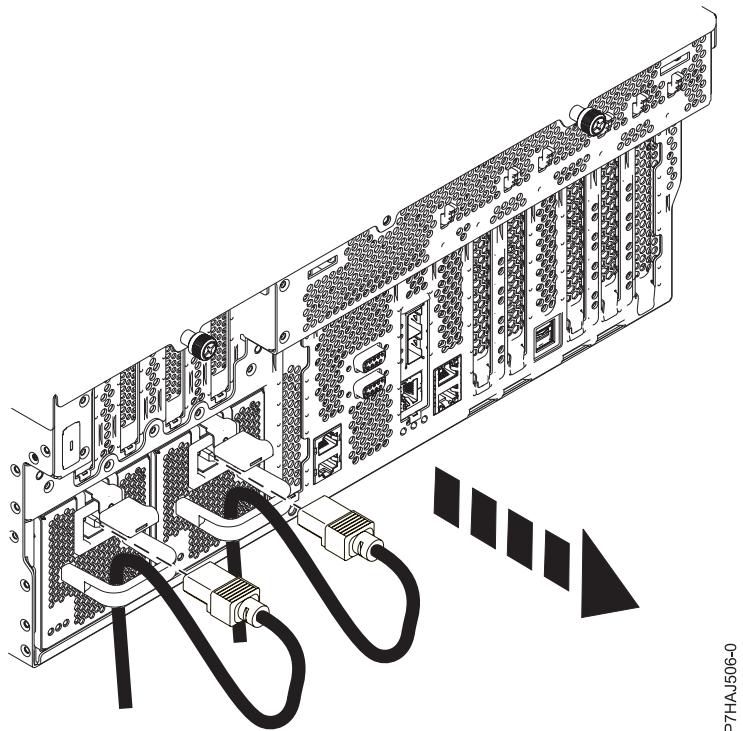
Figura 71. Quitar los cables de alimentación para un sistema montado en bastidor
