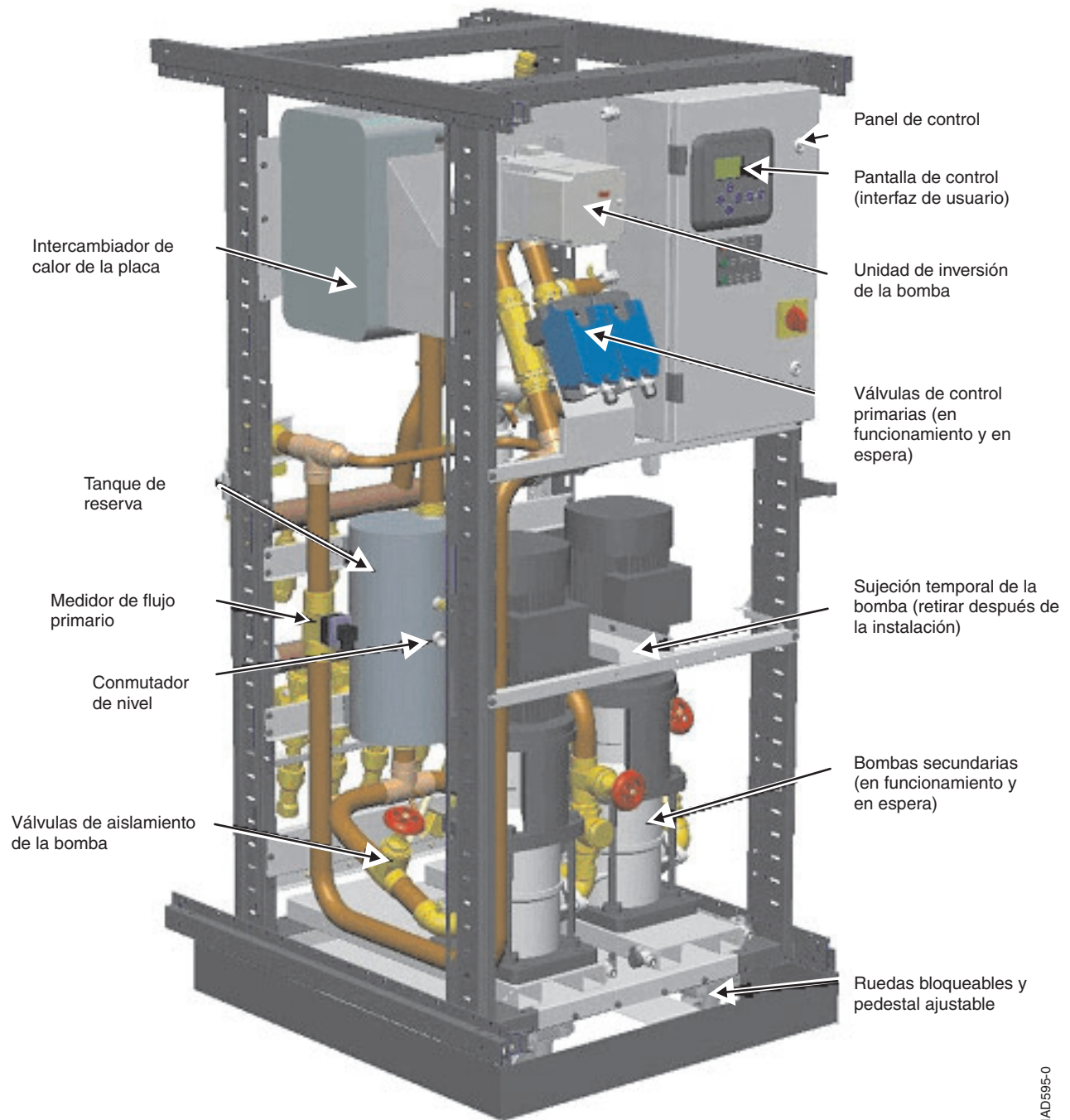
Figura 44. Unidad de distribución de refrigeración
