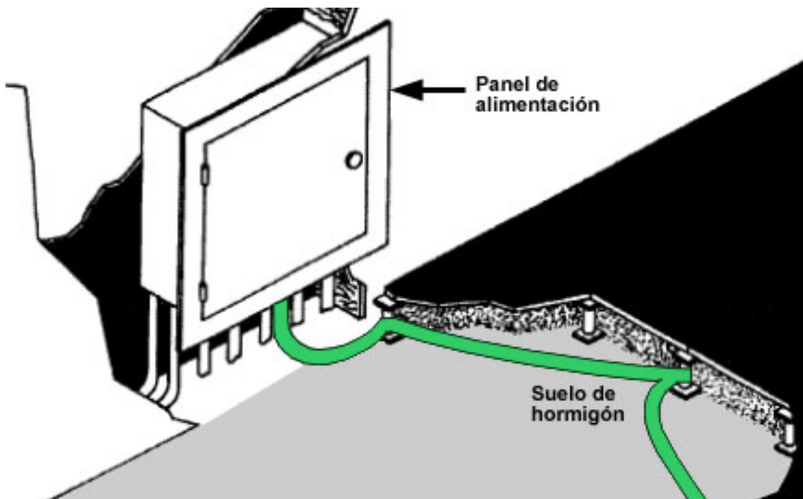
Figura 10. Toma de tierra temporal utilizando la estructura de soporte del pavimento elevado
