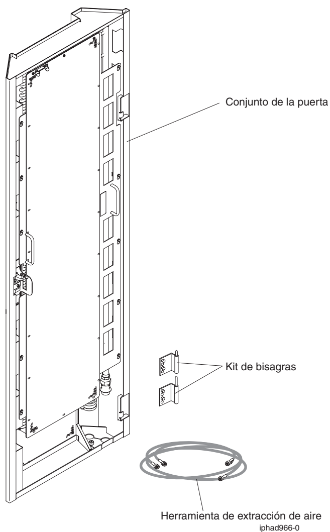
Figura 23. Componentes del kit de intercambiador de calor para bastidores de riel EIA de 19 pulgadas
