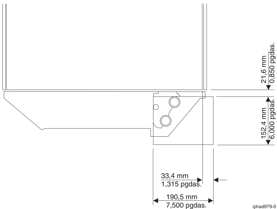
Figura 37. Ejemplo 1 de manejo de mangueras en suelo elevado; definición y ubicación de la abertura de entarimado para bastidores de riel EIA de 24 pulgadas
