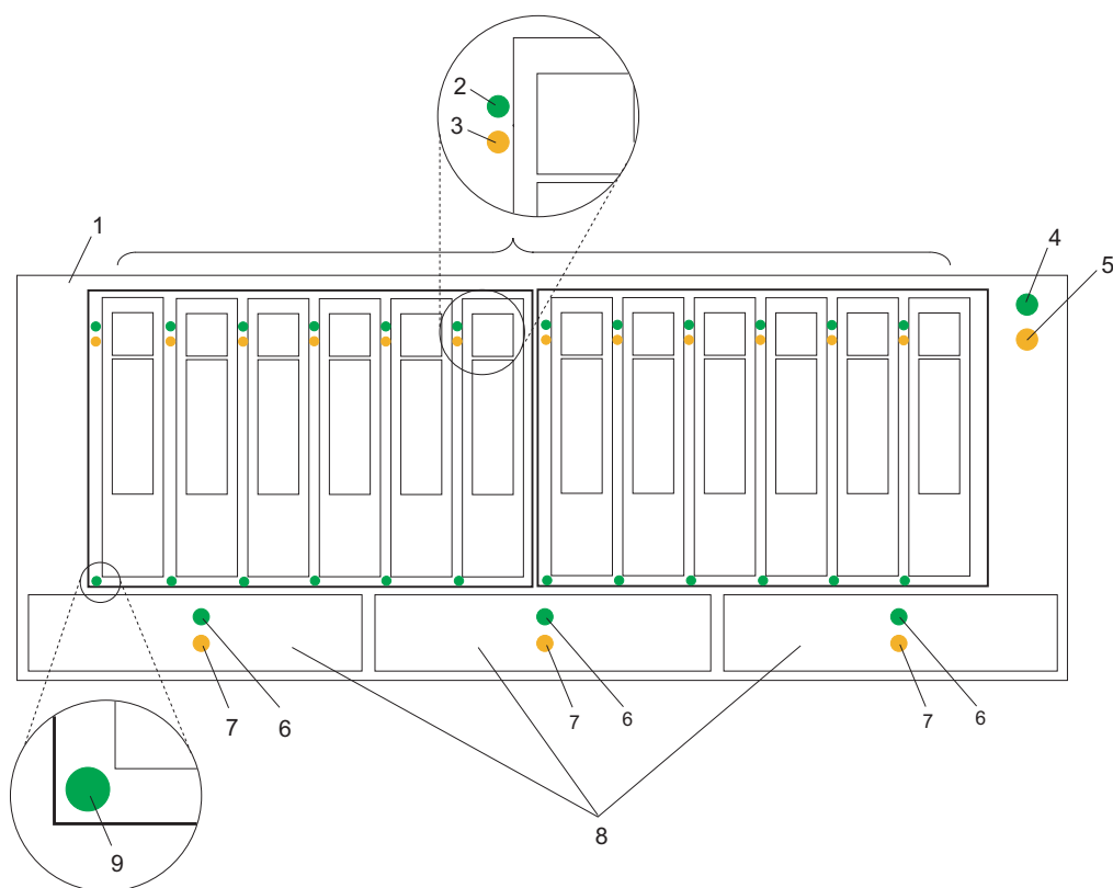
Figura 1. Vista frontal mostrando los LED de mantenimiento en 7031-D24 y 7031-T24
