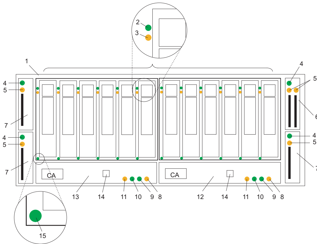
Figura 2. Vista posterior mostrando los LED de mantenimiento en 7031-D24 y 7031-T24
