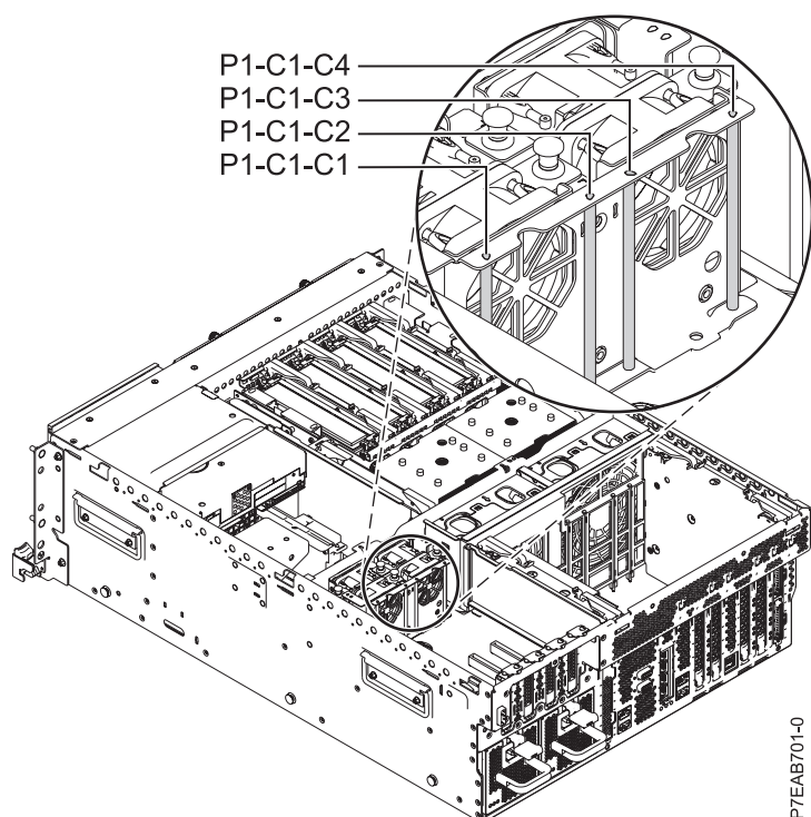
Figura 3. tarjeta de expansión PCI con los códigos de ubicación en los sistemas 8202-E4B y 8205-E6B
