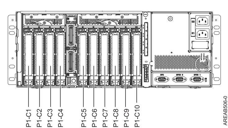
Figura 6. Vista posterior. La figura muestra la vista posterior de la unidad de expansión.
