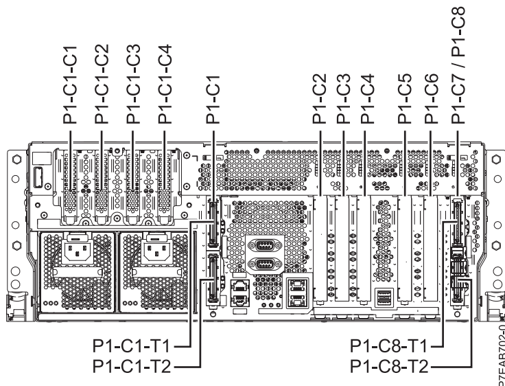
Figura 4. Vista posterior del sistema, que muestra las ranuras PCI con sus códigos de ubicación
