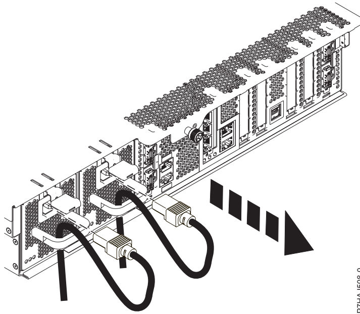
Abbildung 9. Netzkabel abziehen
