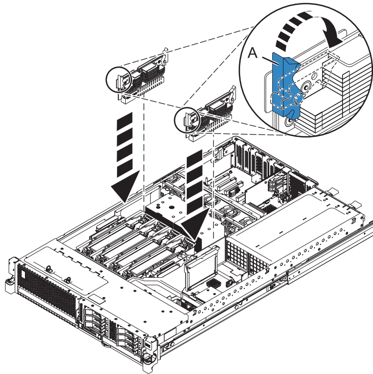
Abbildung 1. Spannungsreglermodule
