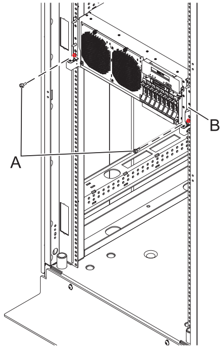
Abbildung 15. Systemeinheit in die Serviceposition bringen
