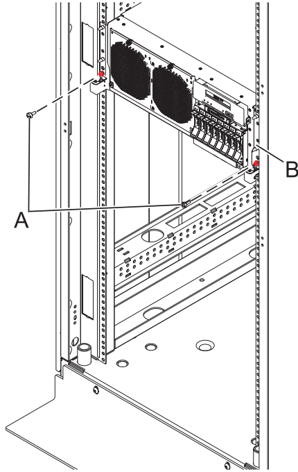
Abbildung 18. Systemeinheit in die Betriebsposition bringen
