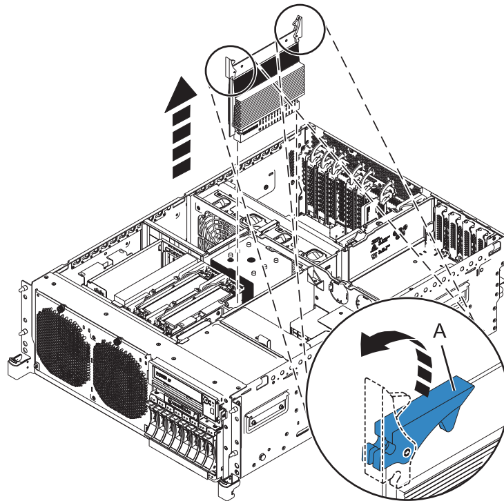
Abbildung 1. Spannungsreglermodule
