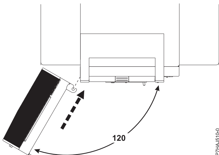
Abbildung 8. Vordere Klappe installieren
