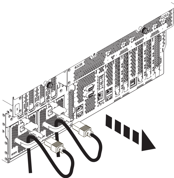
Abbildung 19. Netzkabel abziehen - Einschubsystem
