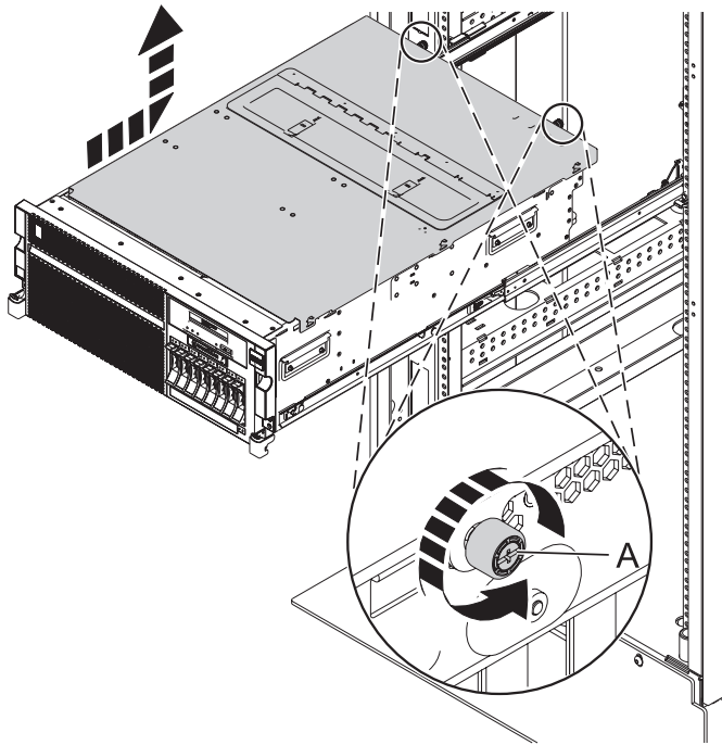
Abbildung 9. Serviceabdeckung ausbauen
