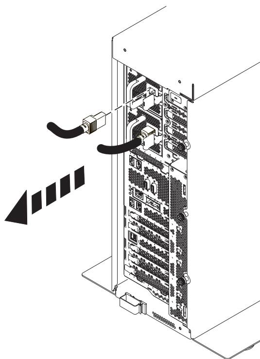
Abbildung 20. Netzkabel eines Standalone-Systems abziehen
