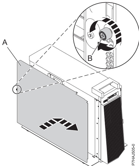
Abbildung 14. Äußere Serviceabdeckung installieren
