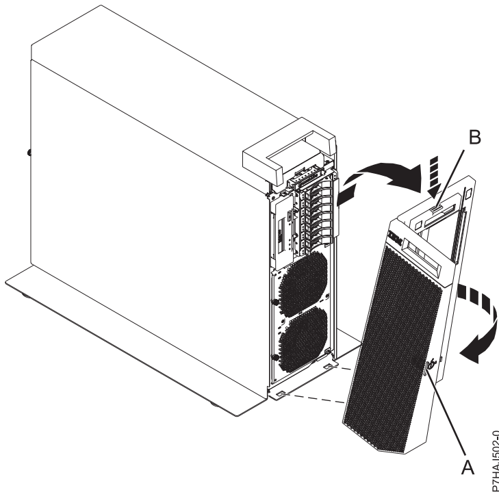
Abbildung 5. Vordere Abdeckung ausbauen
