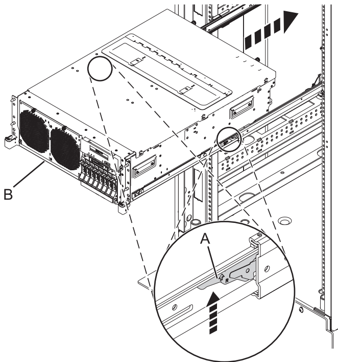
Abbildung 17. Systemeinheit in die Betriebsposition bringen
