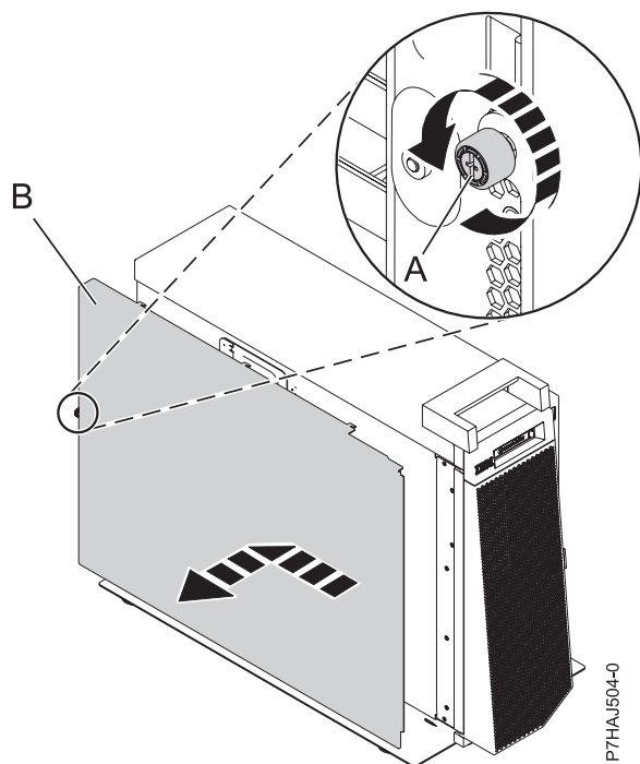
Abbildung 10. Äußere Serviceabdeckung installieren
