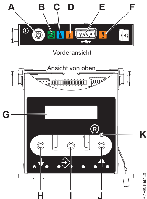
Abbildung 3. Steuerkonsole
