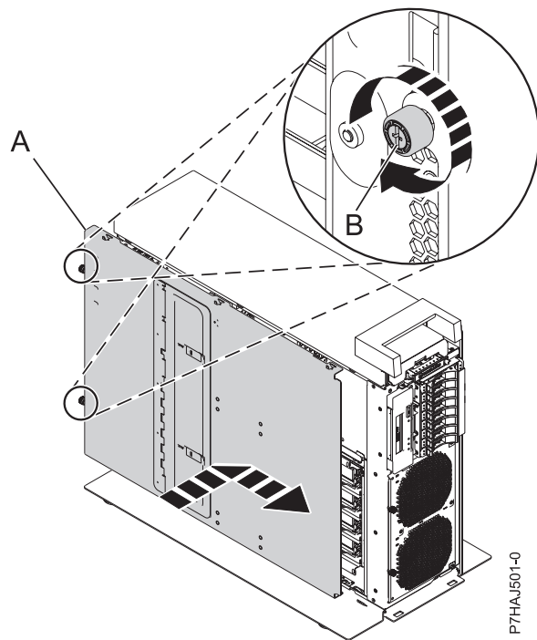
Abbildung 13. Innere Serviceabdeckung installieren
