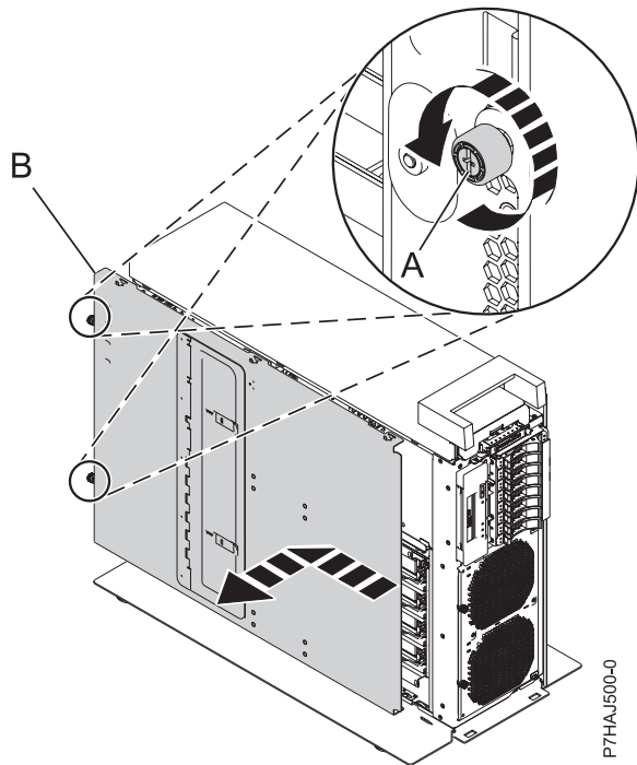
Abbildung 11. Innere Serviceabdeckung ausbauen
