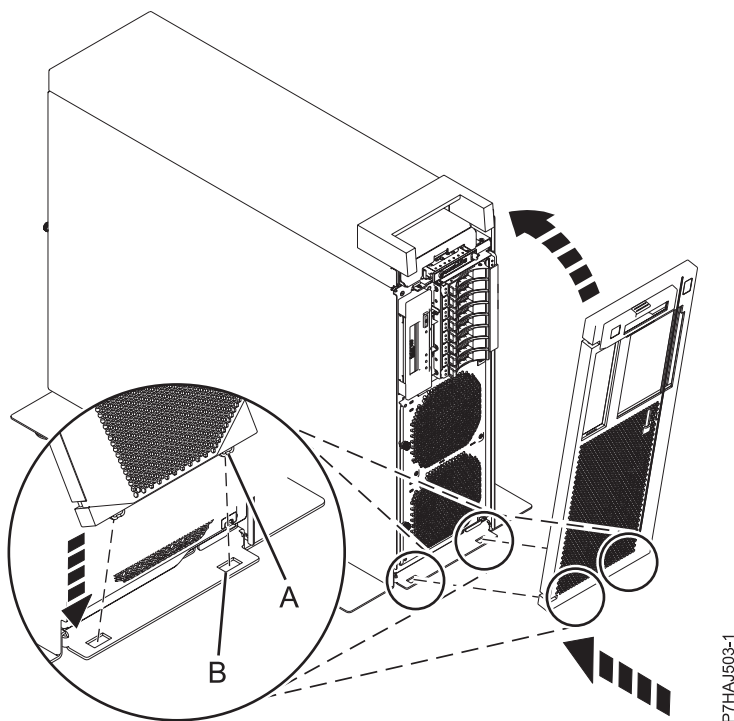
Abbildung 7. Vordere Abdeckung installieren
