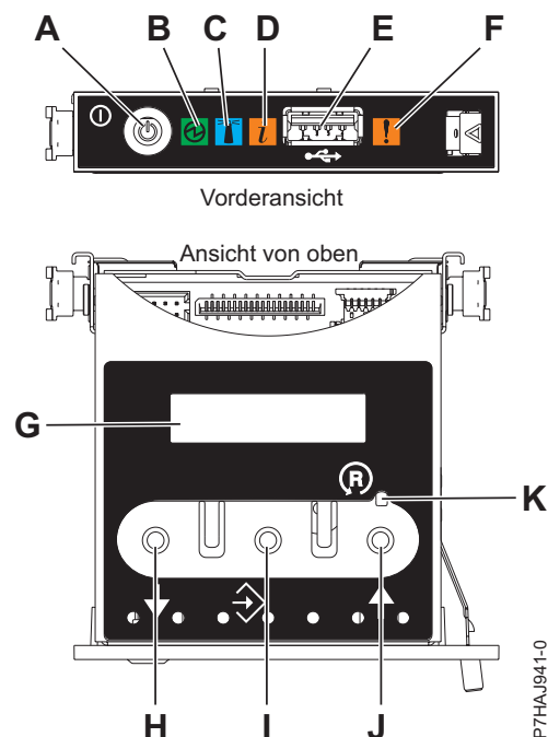
Abbildung 2. Steuerkonsole
