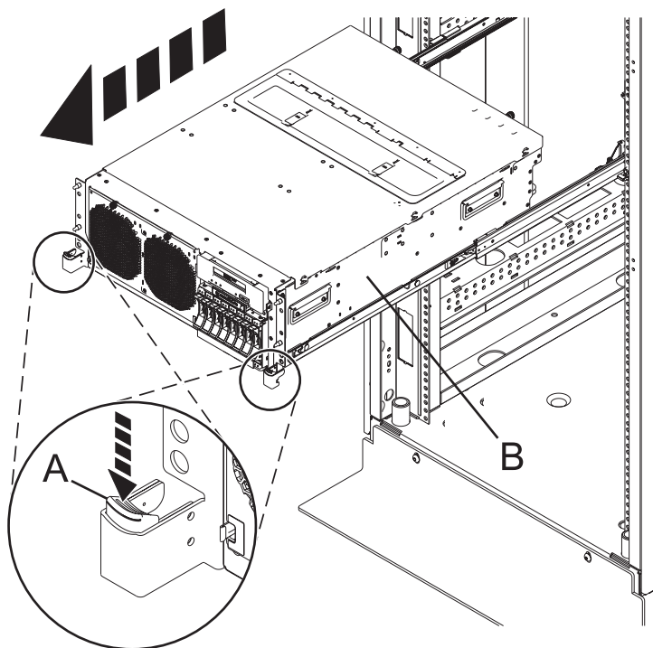
Abbildung 16. Systemeinheit in Serviceposition verriegeln
