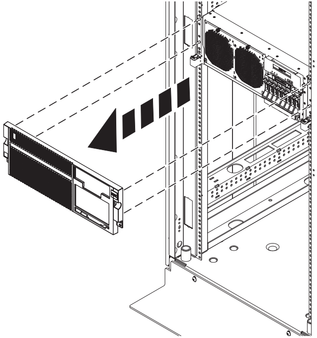
Abbildung 4. Vordere Abdeckung ausbauen
