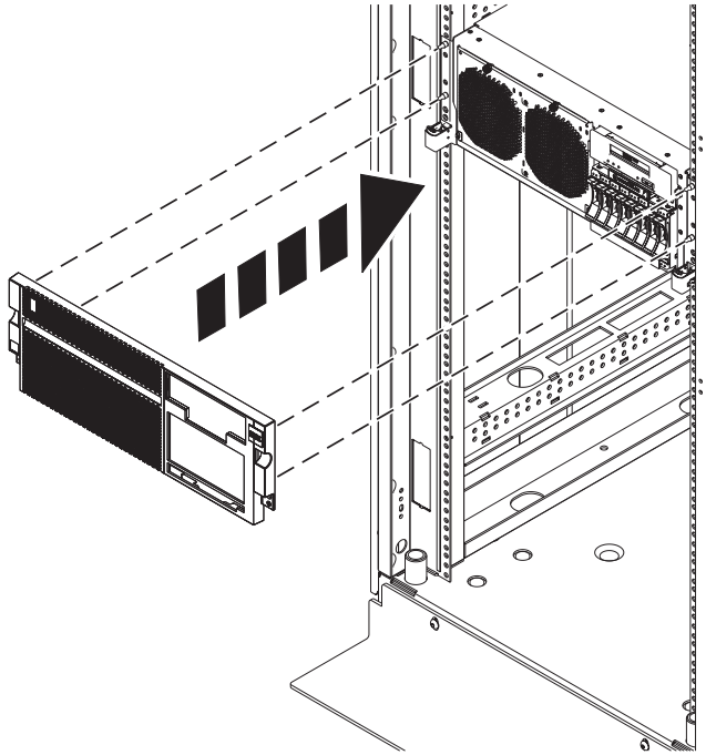
Abbildung 6. Vordere Abdeckung ausbauen
