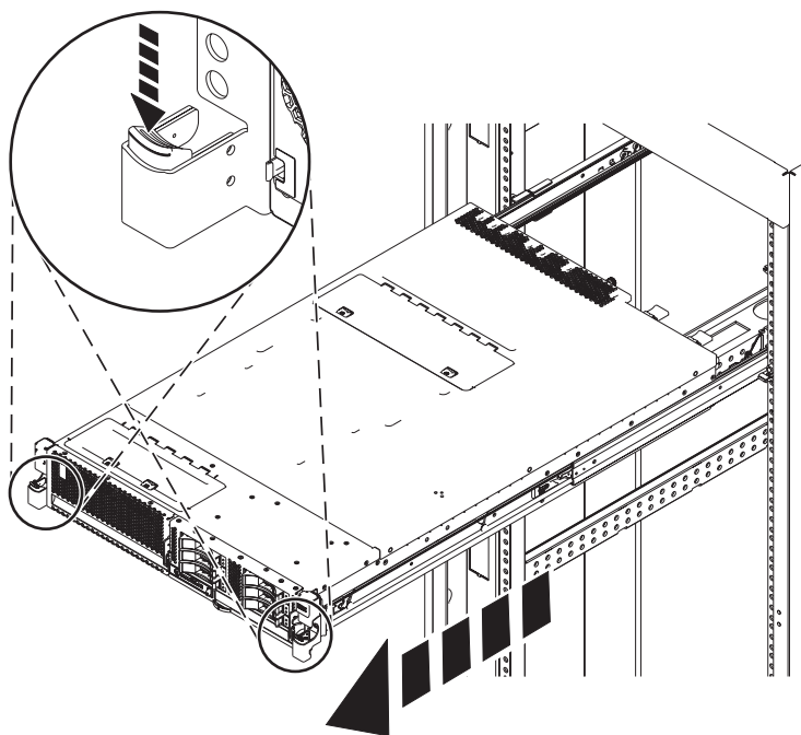
Abbildung 6. System in die Serviceposition bringen
