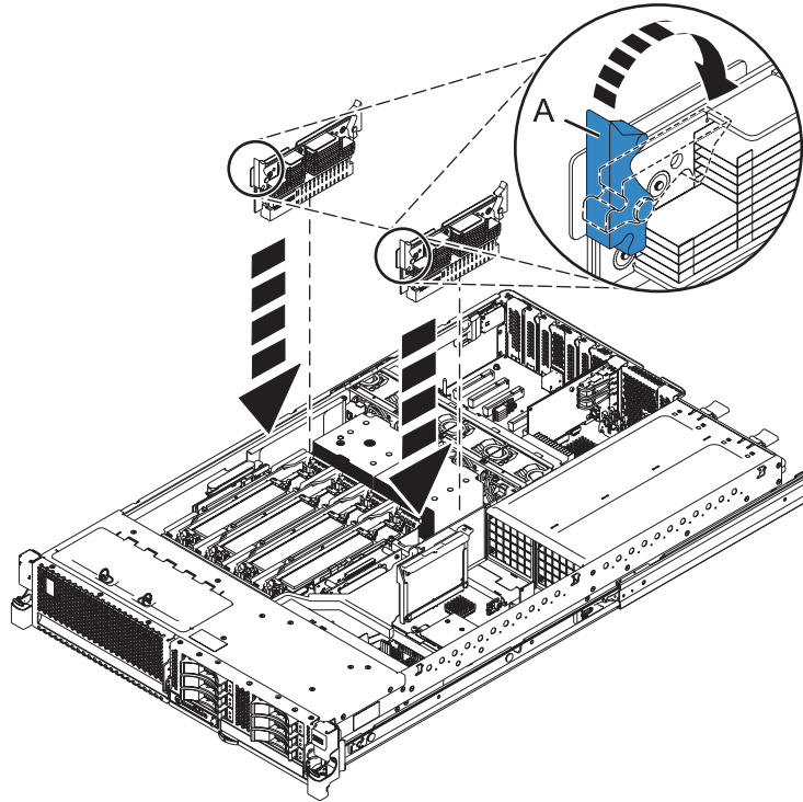
Abbildung 1. Spannungsreglermodule
