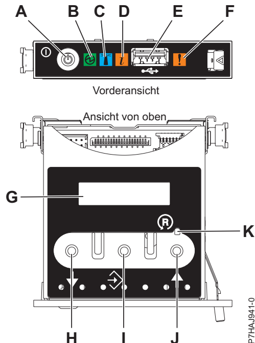
Abbildung 2. Steuerkonsole
