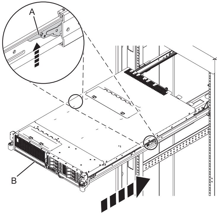
Abbildung 7. Schienensicherheitsverriegelungen entriegeln
