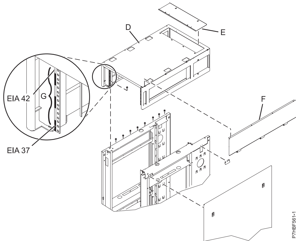
Abbildung 36. Obere Abdeckung ausbauen
