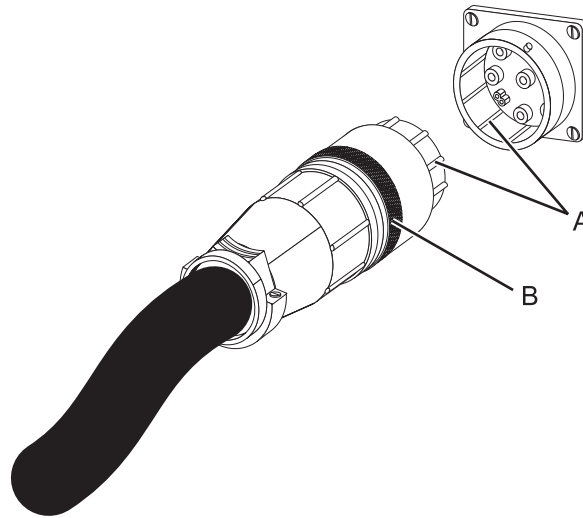
Abbildung 41. Netzkabelstecker an PDU-Modell ausrichten
