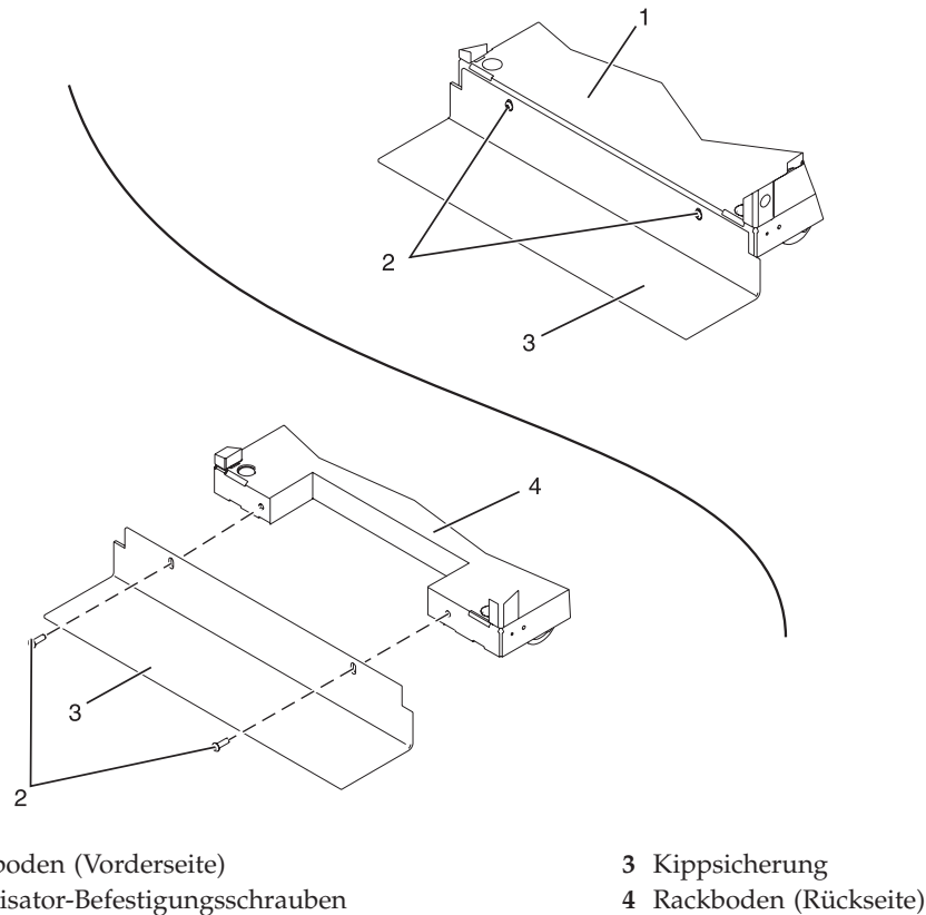
Abbildung 3. Kippsicherungen anbringen
