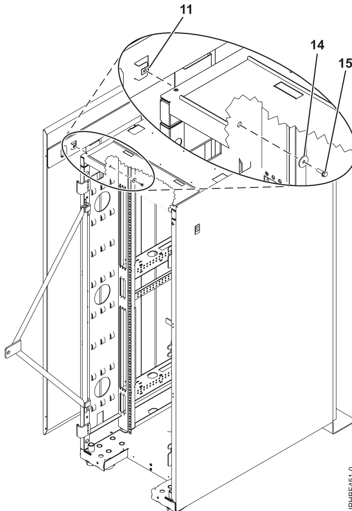
Abbildung 31. Befestigungsschrauben an Seitenabdeckung entfernen
