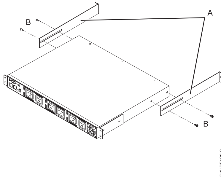
Abbildung 43. Lange Halterungen anbringen
