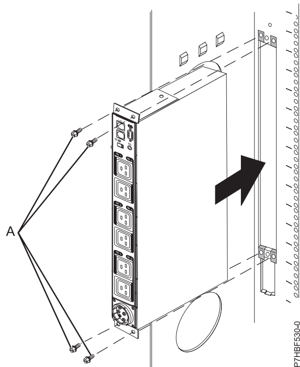
Abbildung 40. PDU+ an der Öffnung an der Seite des Racks ausrichten
