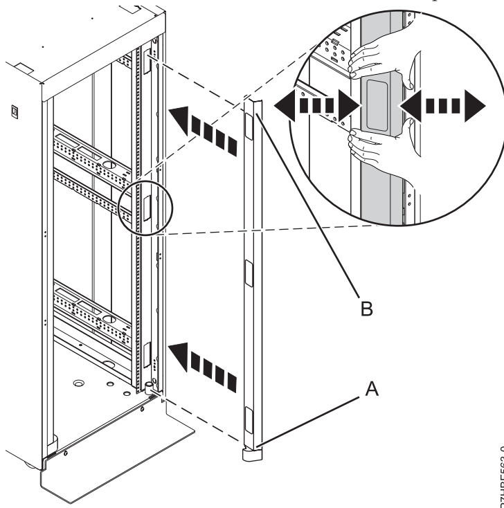
Abbildung 22. Racktrimmplatte installieren
