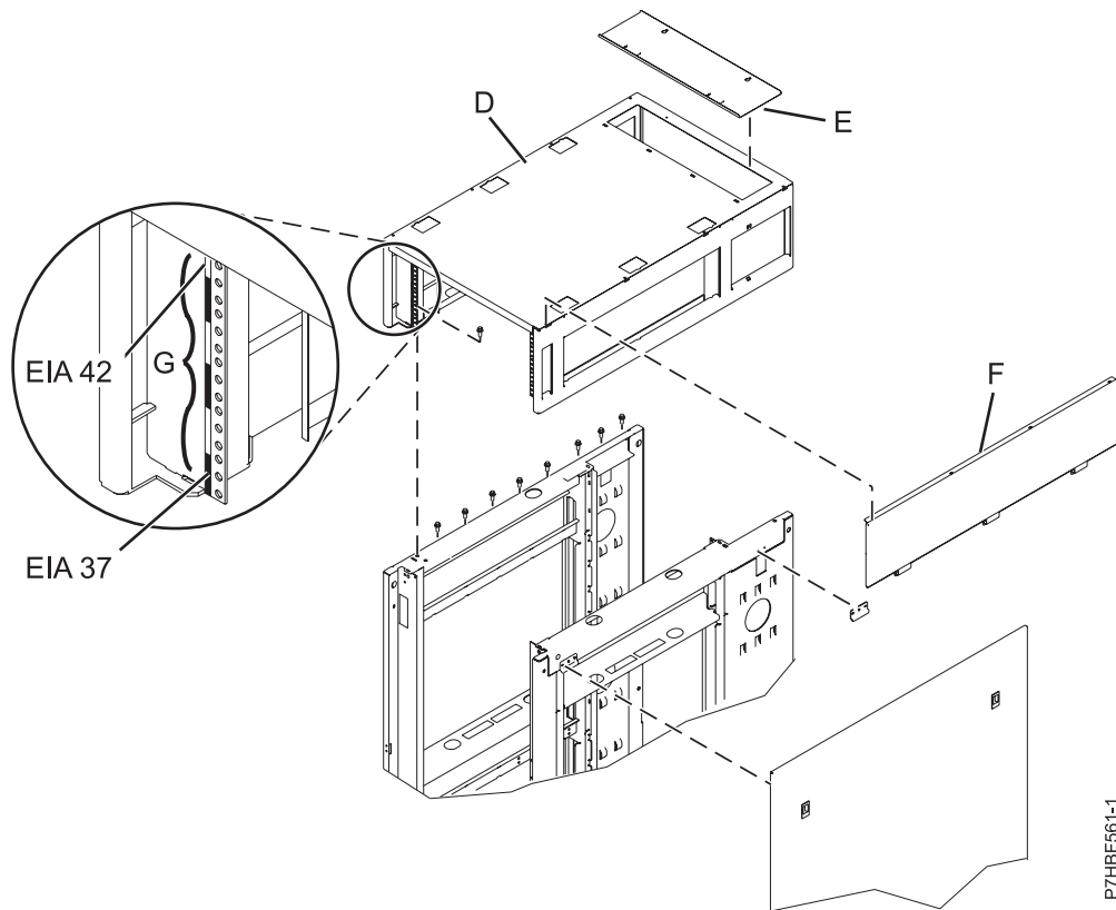
Abbildung 35. Obere Abdeckung ausbauen
