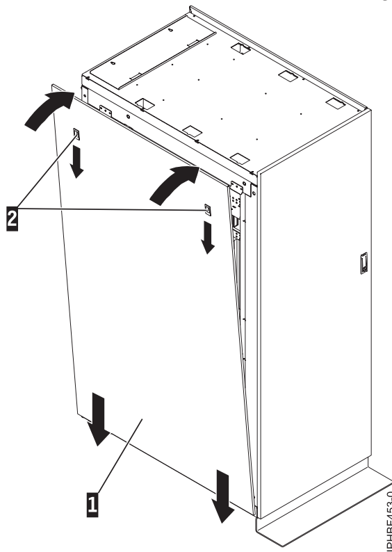
Abbildung 20. Seitenabdeckung austauschen
