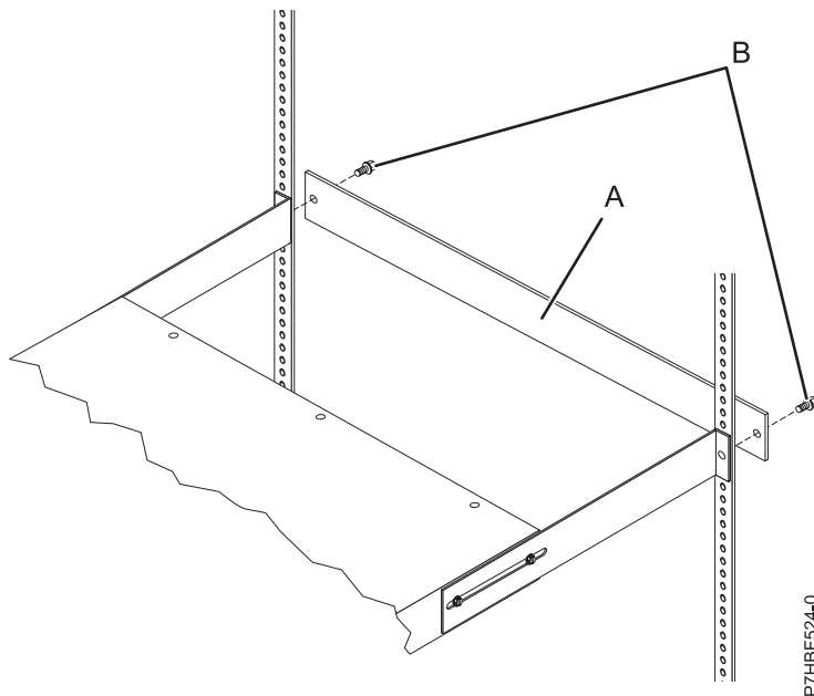
Abbildung 45. Halterungen und Abdeckblende am Rack anbringen
