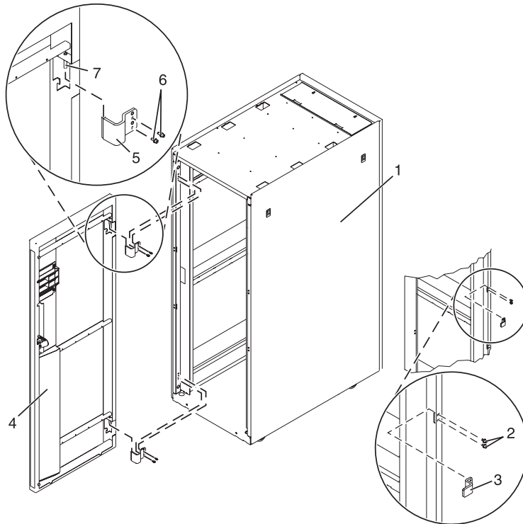
Abbildung 23. Rackklappe installieren
