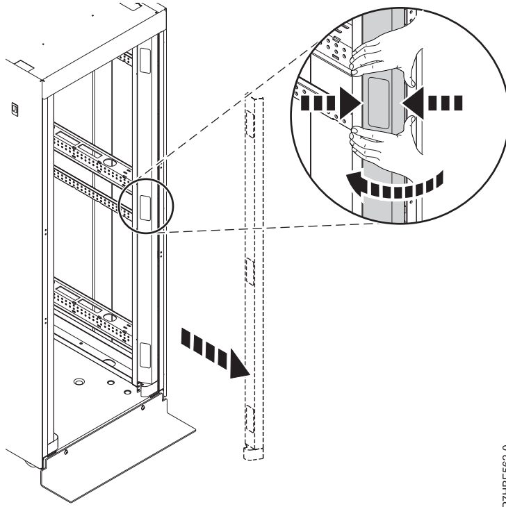
Abbildung 21. Racktrimmplatte ausbauen
