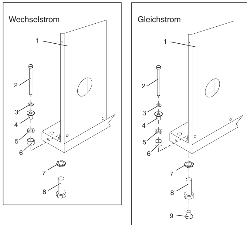
Abbildung 5. Wechselstrommontageplatten installieren
