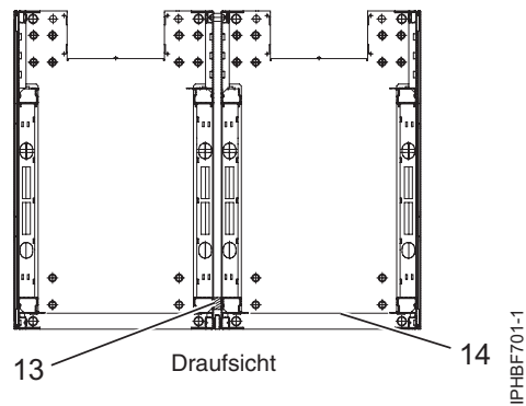
Abbildung 33. Position der Schaumstoffstreifen (Ansicht von oben)
