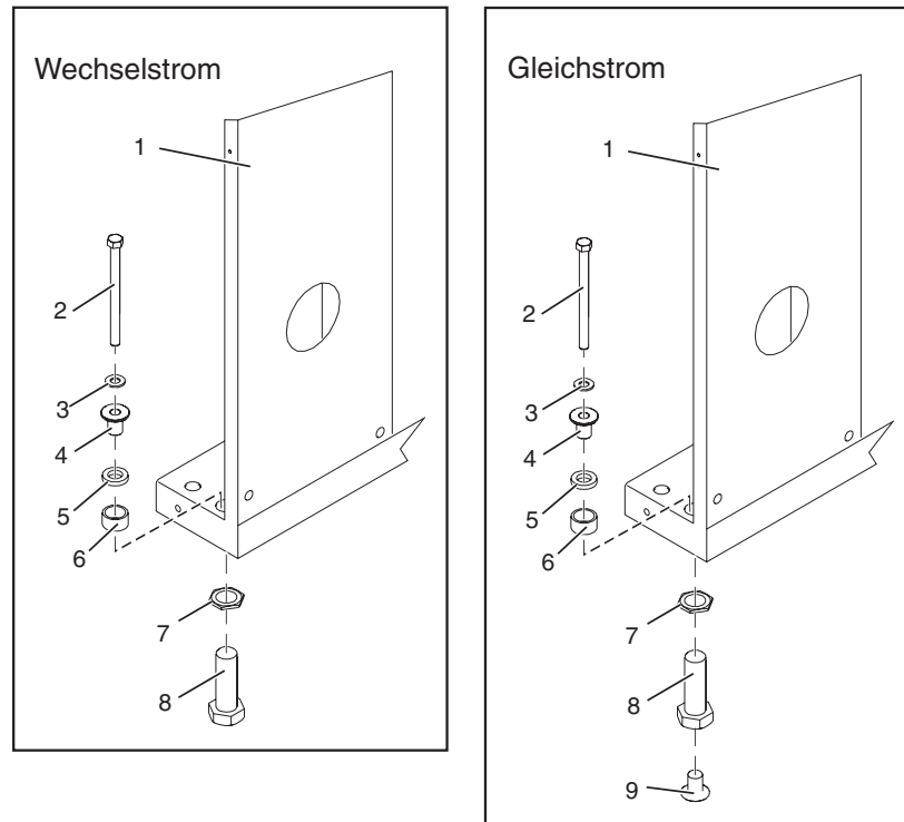
Abbildung 9. Montageplatten mit Wechselstrom-Netzsteckdosen installieren
