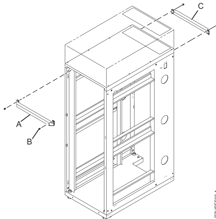
Abbildung 34. Rackklammer befestigen
