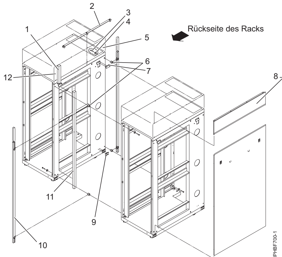
Abbildung 32. Seitenabdeckungen, Z-Halterung und J-Halterung ausbauen und Abstandsschrauben und langen Schaumstoffstreifen zum Verbinden mehrerer Racks installieren
