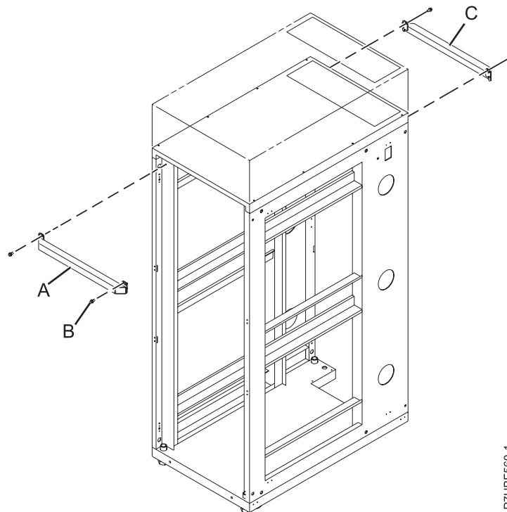
Abbildung 37. Obere Abdeckung ausbauen
