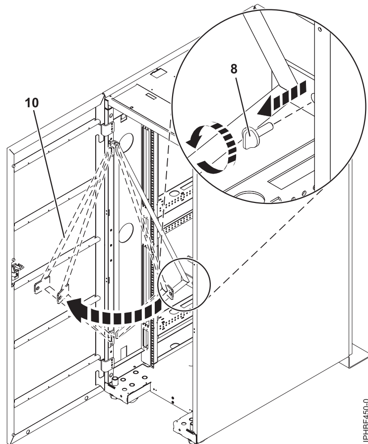
Abbildung 30. Verstärkungsrahmen lösen, um auf Systeme zuzugreifen
