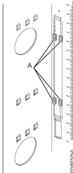
Abbildung 39. Klemmmuttern an Rackbefestigungsflanschen anbringen
