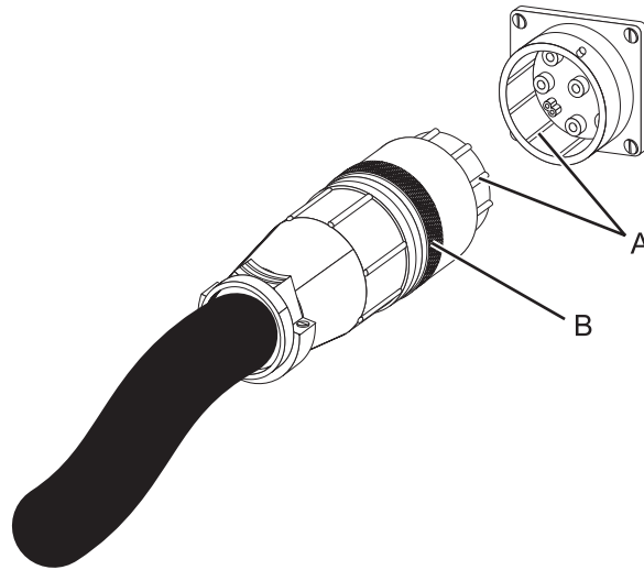
Abbildung 46. Netzkabelstecker an PDU-Modell ausrichten
