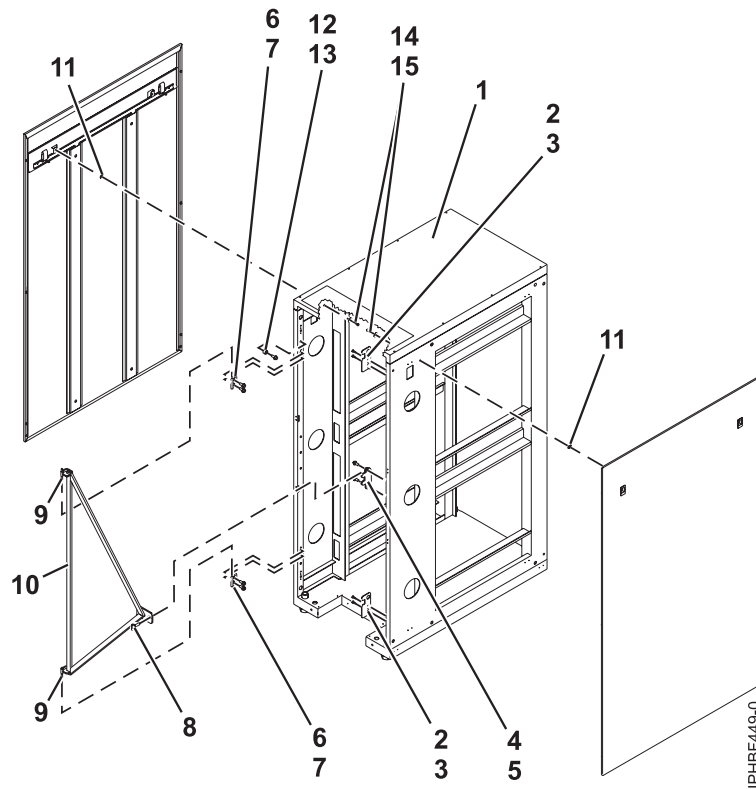
Abbildung 29. Teile des Verstärkungskits
