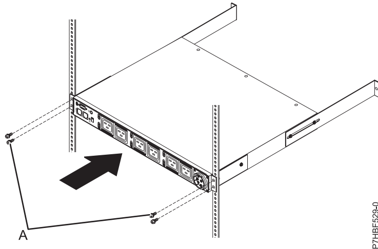
Abbildung 44. Vorderseite des PDU+-Modells am Rack befestigen
