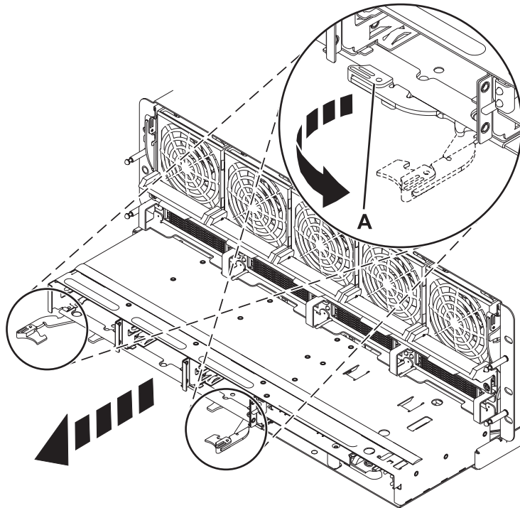
Abbildung 2. Plattenlaufwerk-Rückwandplatine ausbauen
