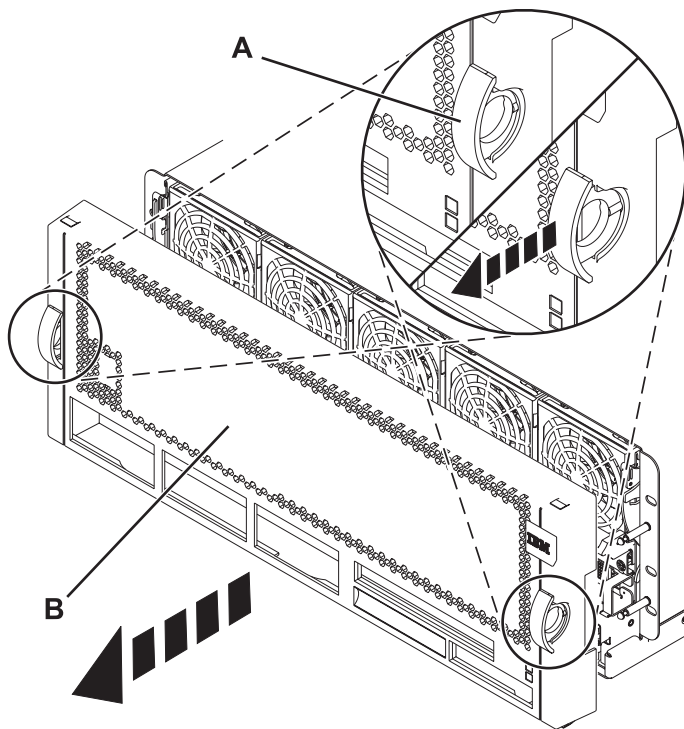
Abbildung 7. Vordere Abdeckung ausbauen
