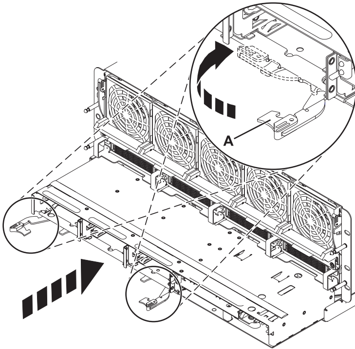
Abbildung 3. Plattenlaufwerk-Rückwandplatine installieren
