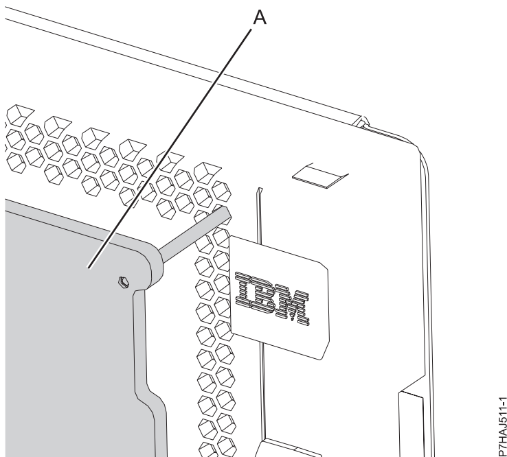
Abbildung 9. Ausbauwerkzeug ausrichten
