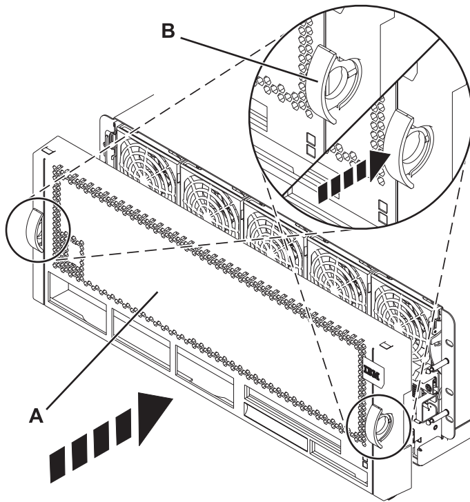
Abbildung 14. Vordere Abdeckung installieren
