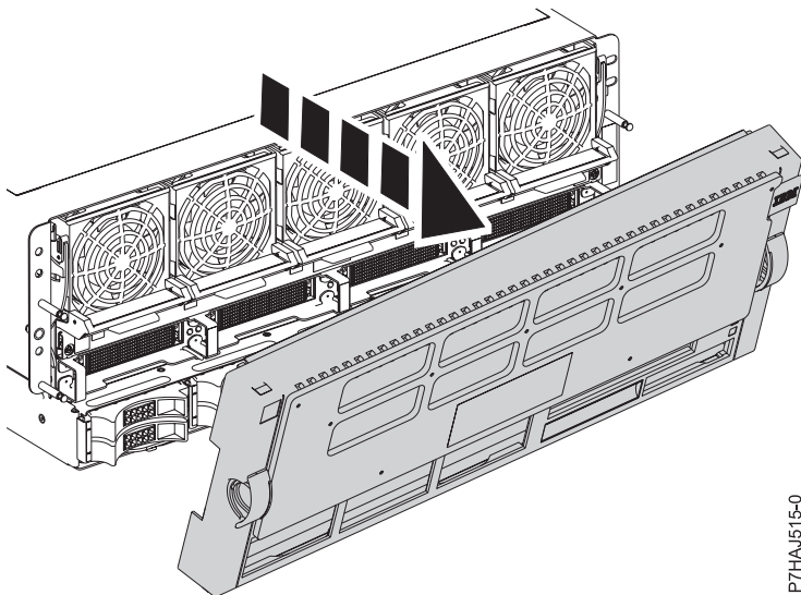
Abbildung 13. Abdeckung ausbauen
