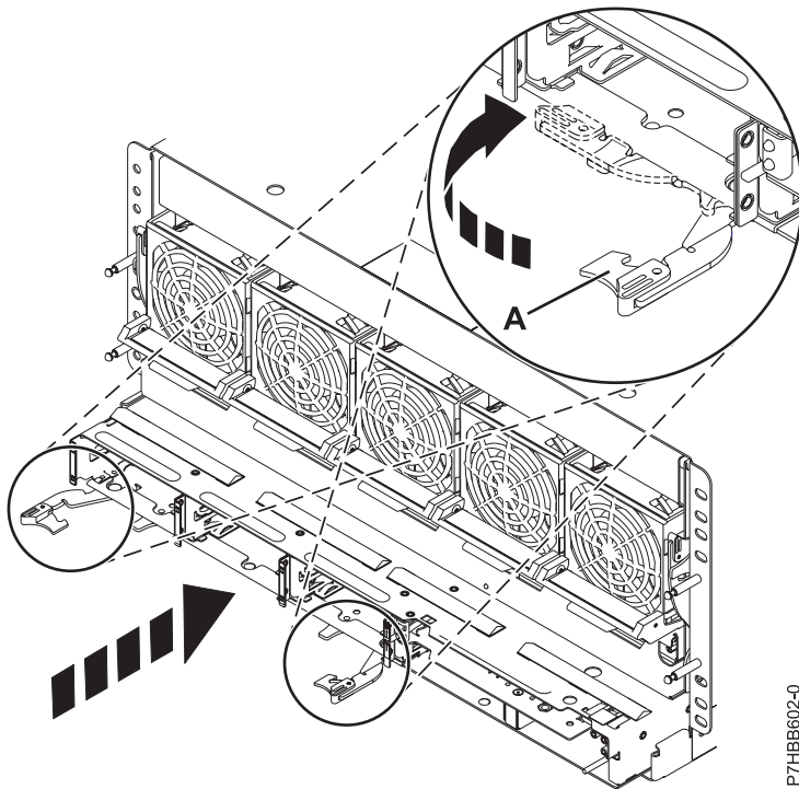
Abbildung 3. Plattenlaufwerk-Rückwandplatine installieren
