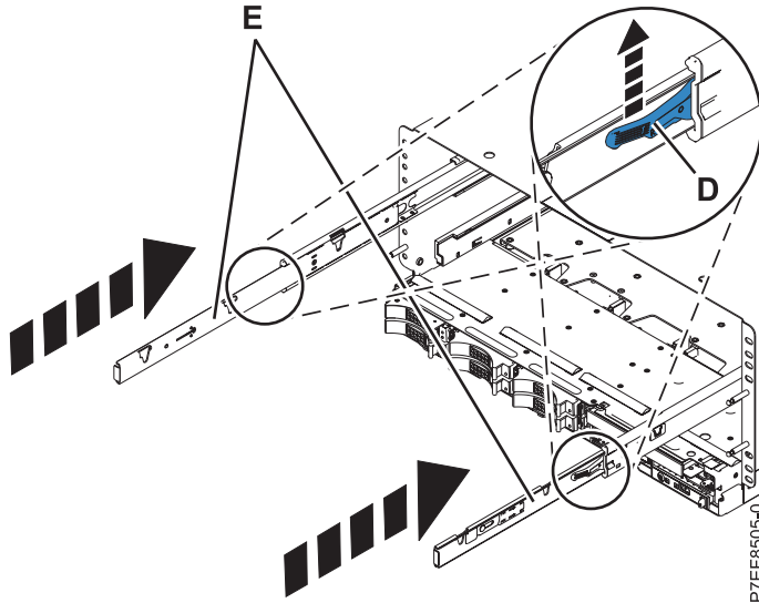
Abbildung 10. Schienensicherheitsverriegelungen entriegeln
