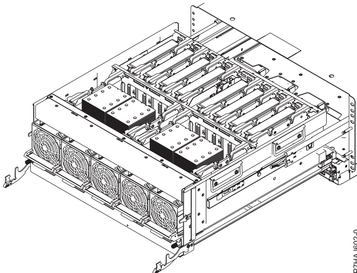
Abbildung 9. System in die Serviceposition bringen
