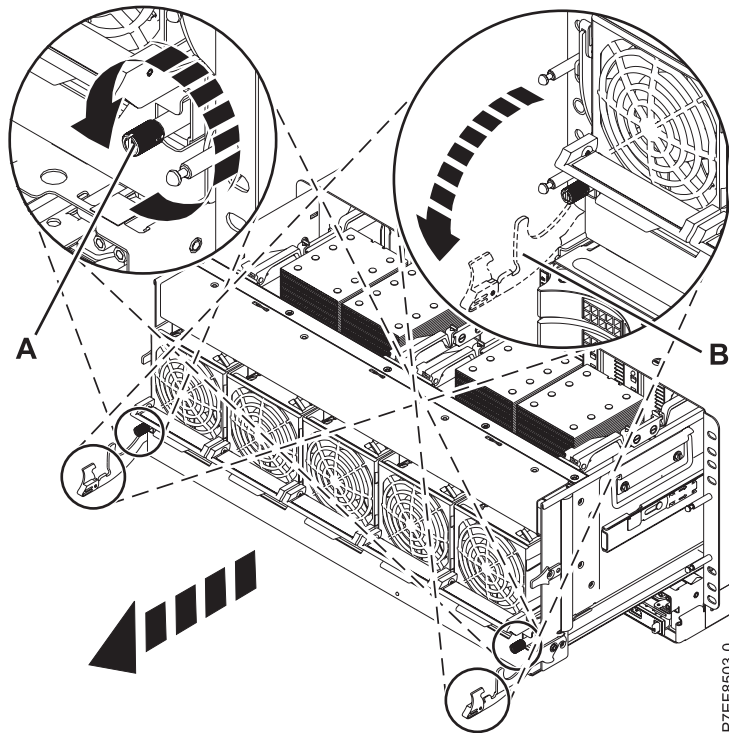
Abbildung 8. Seitliche Verriegelungen entriegeln
