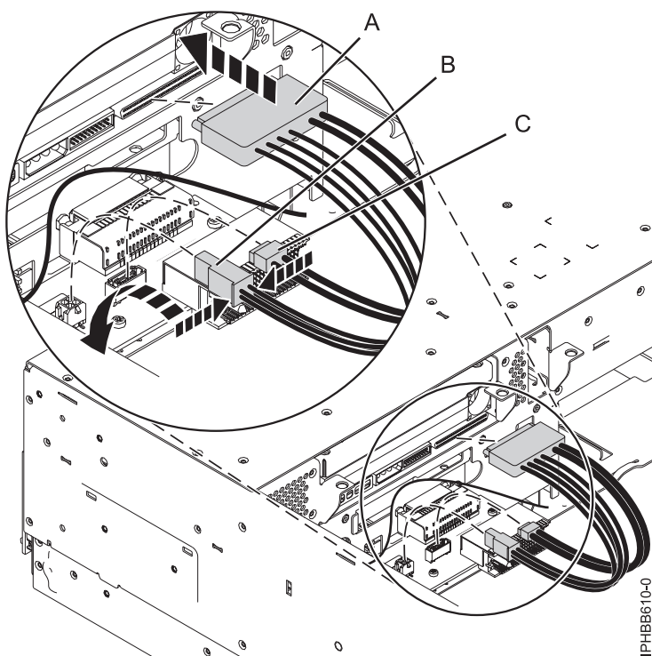
Abbildung 13. Kabel an Plattenlaufwerk-Rückwandplatine anschließen
