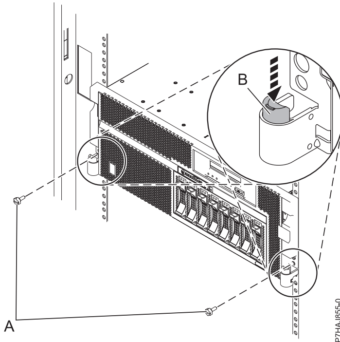
Abbildung 24. Rack-Verriegelungen entriegeln
