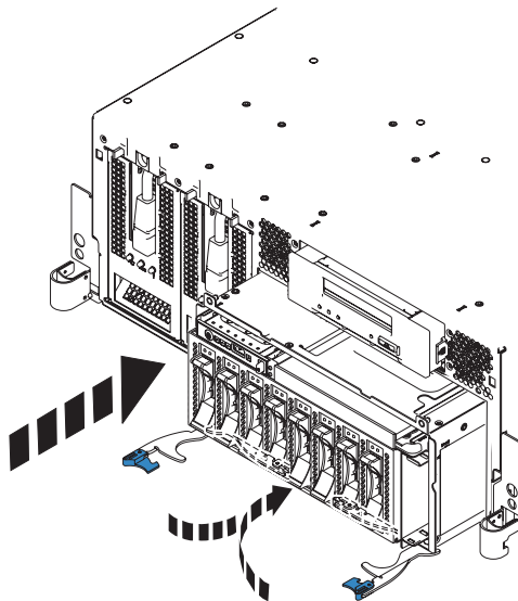
Abbildung 12. Gefüllte Plattenlaufwerk-Rückwandplatine in Einschubmodell installieren
