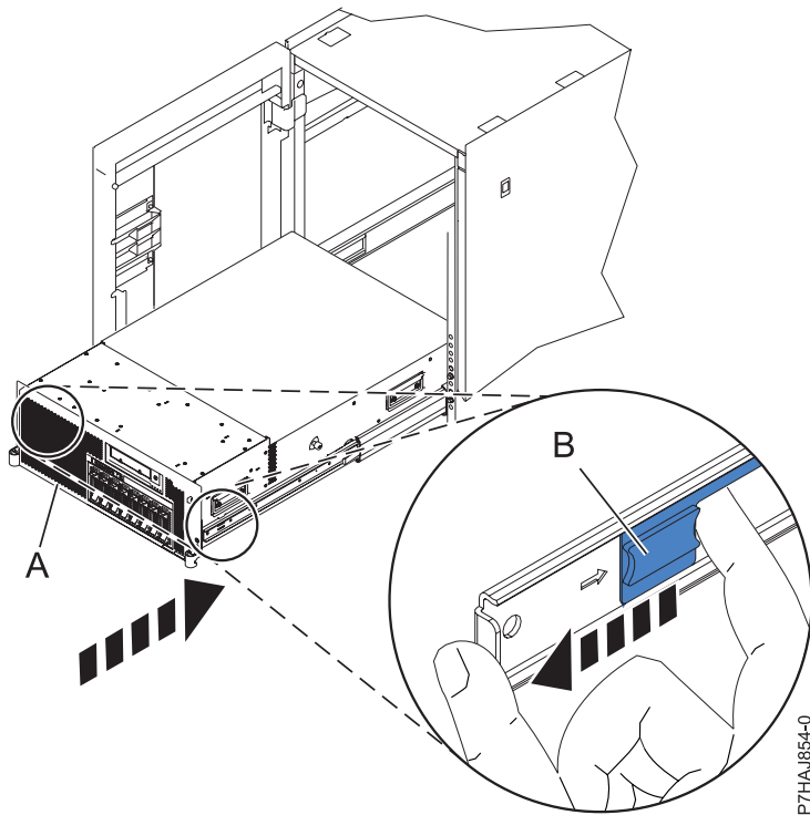
Abbildung 25. Schienensicherheitsverriegelungen entriegeln
