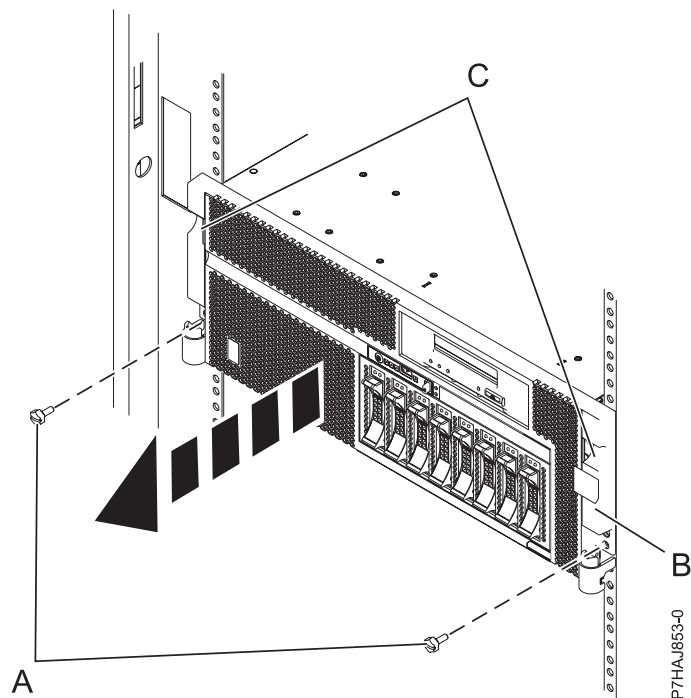
Abbildung 20. Vordere Abdeckung ausbauen
