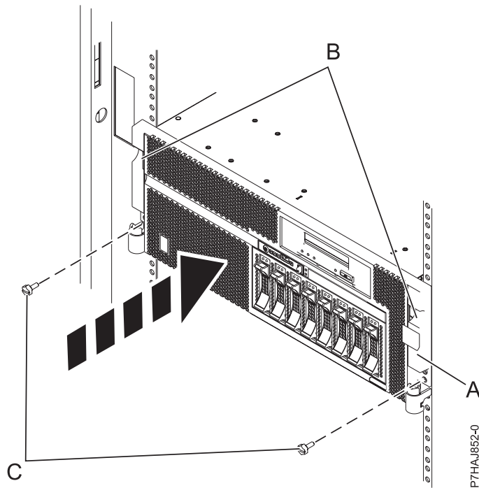
Abbildung 26. Rändelschrauben ersetzen
