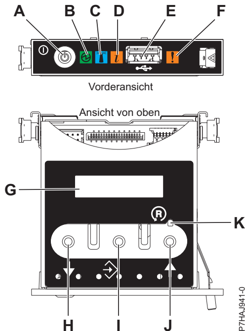
Abbildung 18. Steuerkonsole
