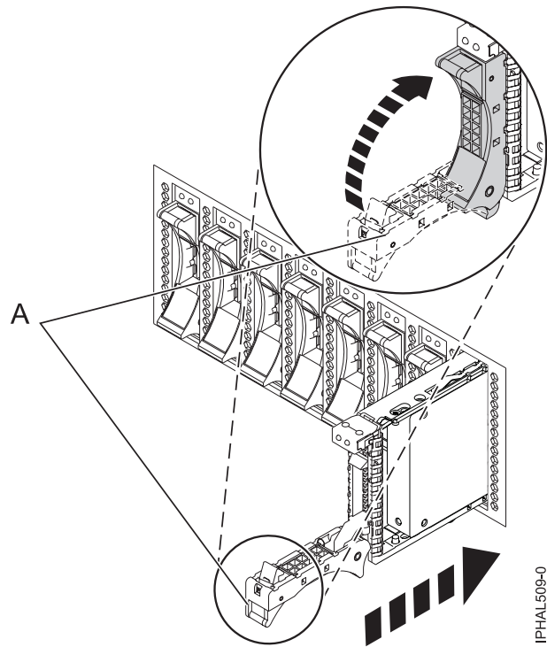
Abbildung 14. Rückwandplatten-Plattenlaufwerke installieren
