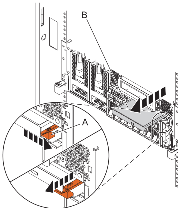
Abbildung 7. Datenträgereinheit aus Plattenlaufwerk-Rückwandplatine ausbauen
