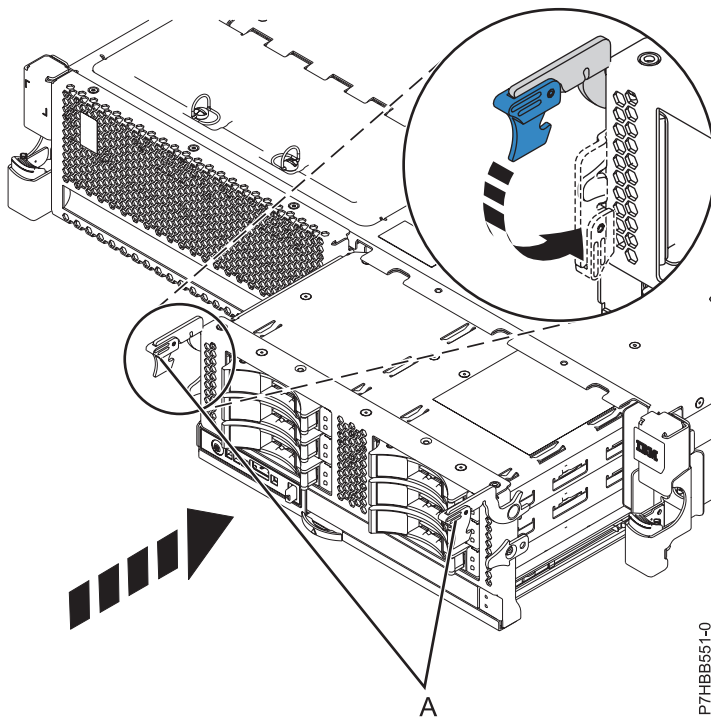
Abbildung 9. Rückwandplatine, die mit Plattenlaufwerken gefüllt ist, in Einschubmodell installieren
