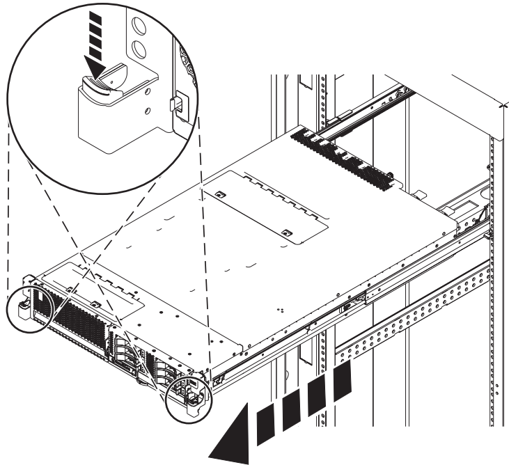
Abbildung 17. System in die Serviceposition bringen
