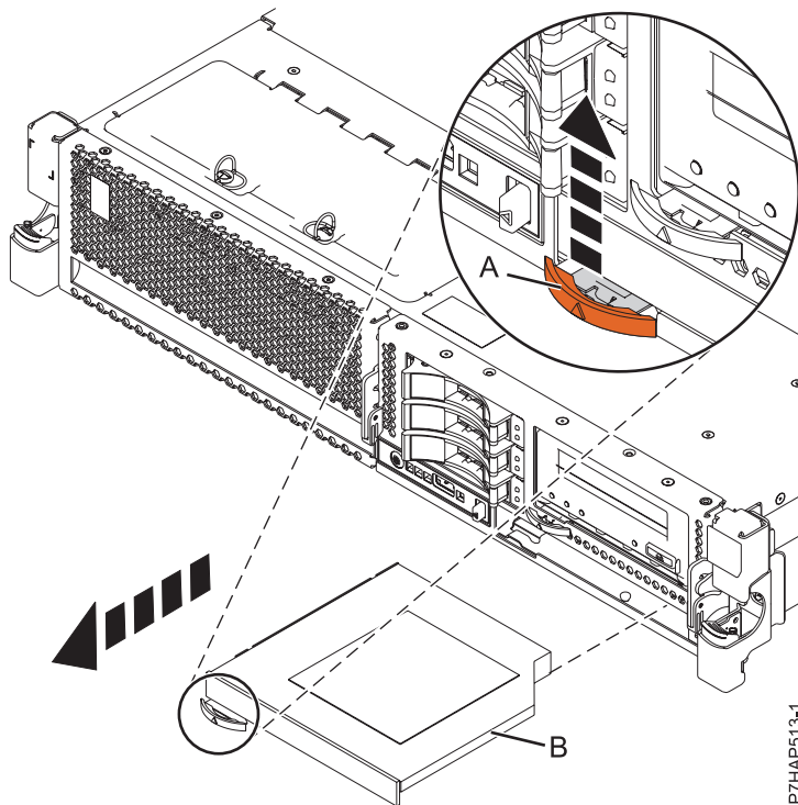
Abbildung 5. SAS-Datenträgereinheit aus Plattenlaufwerk-Rückwandplatine ausbauen
