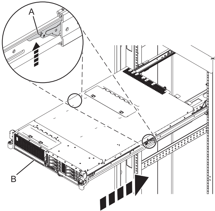
Abbildung 18. Schienensicherheitsverriegelungen entriegeln
