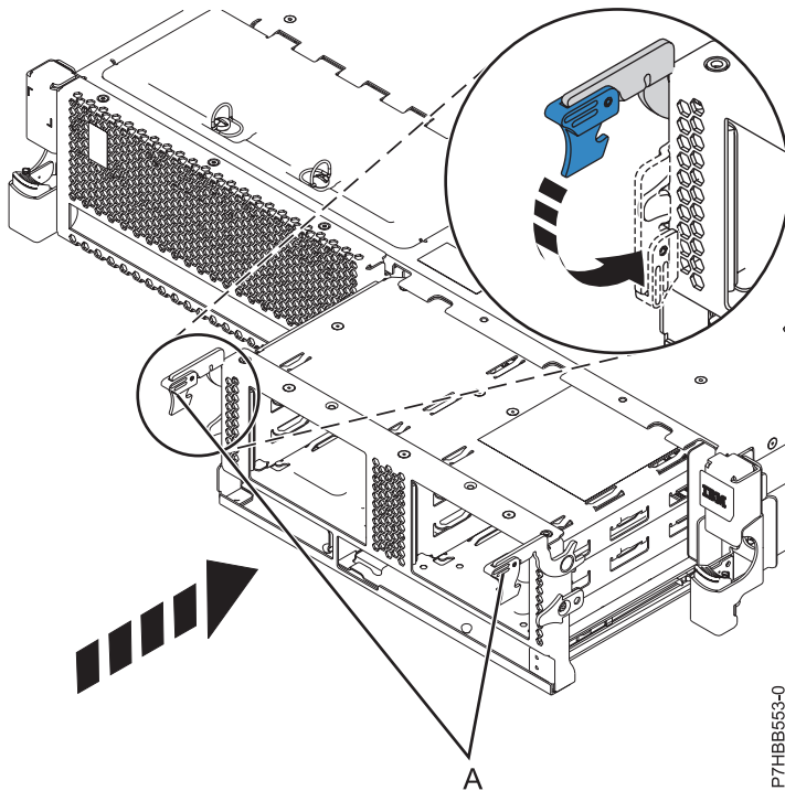
Abbildung 8. Rückwandplatine, die nicht mit Plattenlaufwerken gefüllt ist, in Einschubmodell installieren
