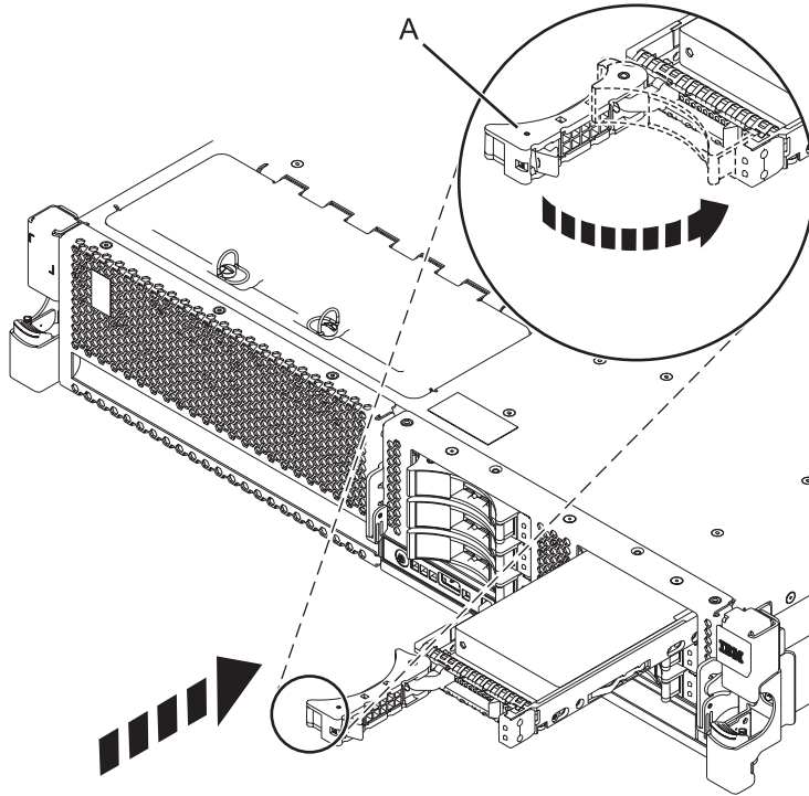
Abbildung 10. Rückwandplatten-Plattenlaufwerke installieren
