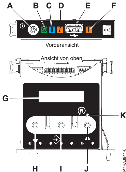
Abbildung 13. Steuerkonsole
