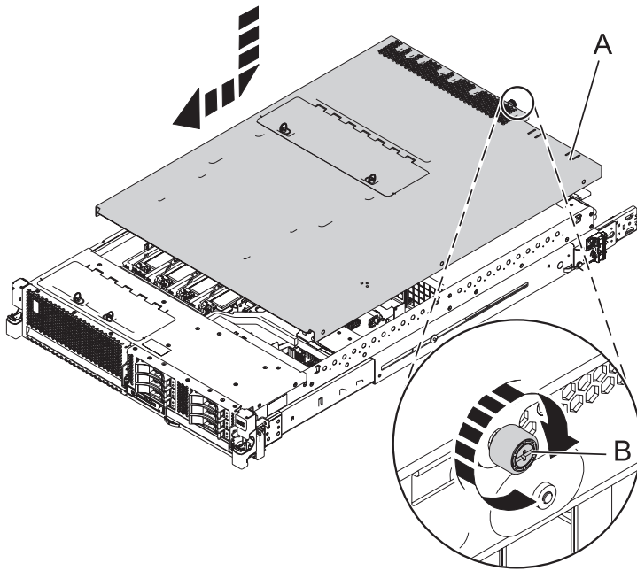
Abbildung 16. Serviceabdeckung installieren
