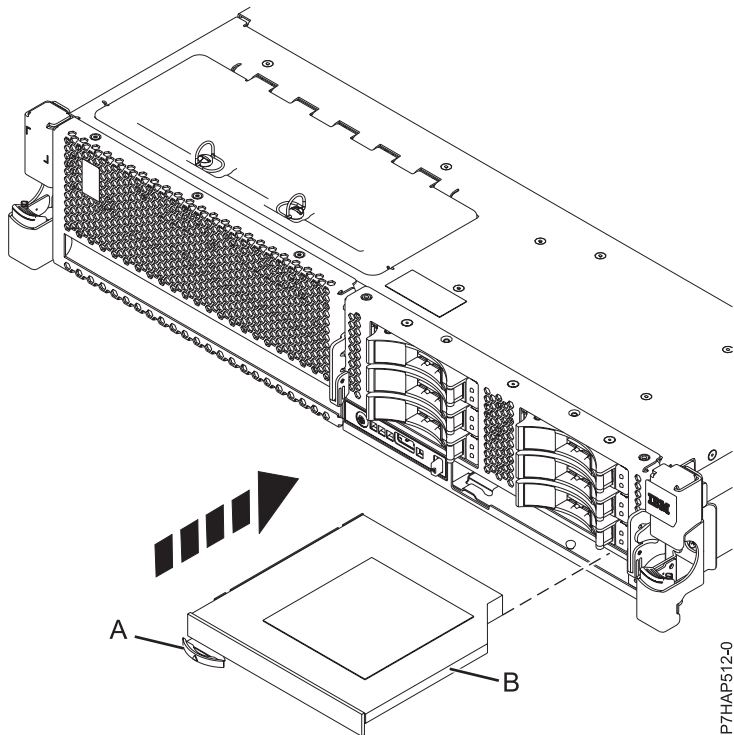
Abbildung 12. Installation der flachen Datenträgereinheit
