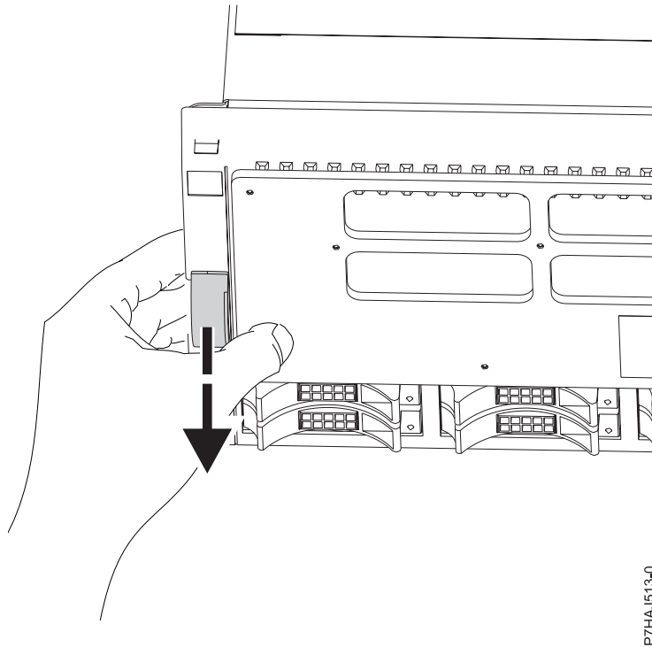
Abbildung 12. Abdeckungsverriegelungen entriegeln
