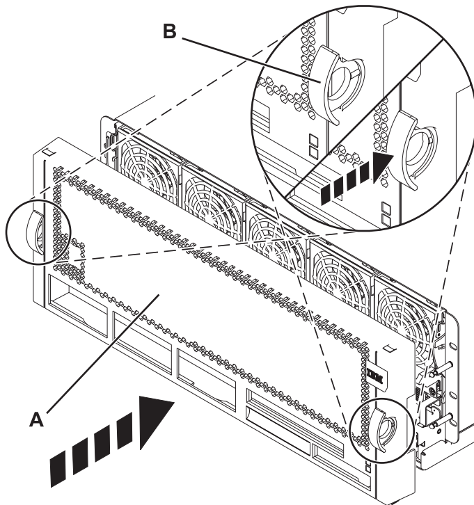
Abbildung 15. Vordere Abdeckung installieren
