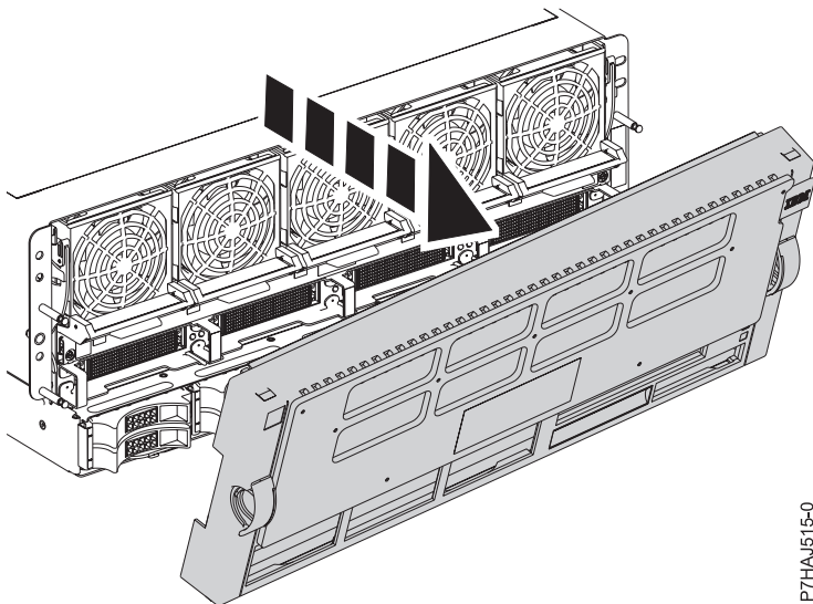
Abbildung 14. Abdeckung ausbauen
