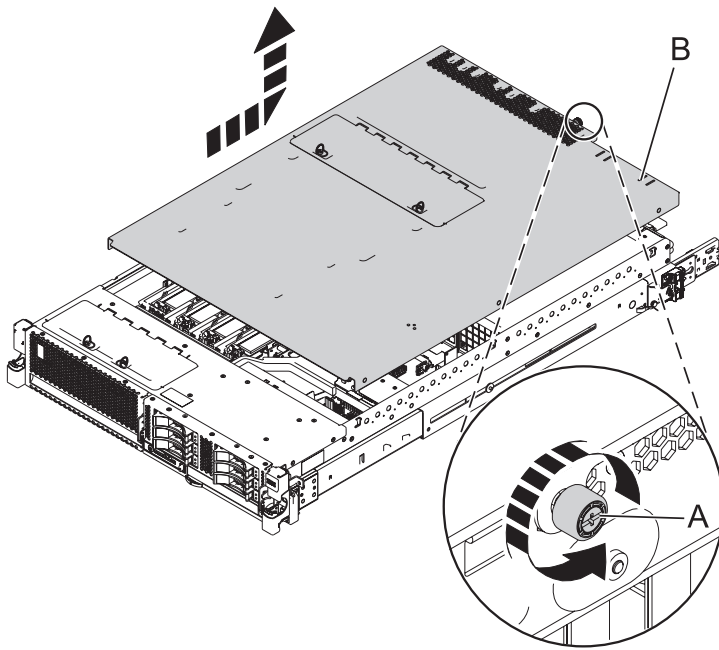
Abbildung 11. Serviceabdeckung ausbauen
