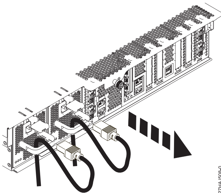
Abbildung 16. Abziehen der Netzkabel
