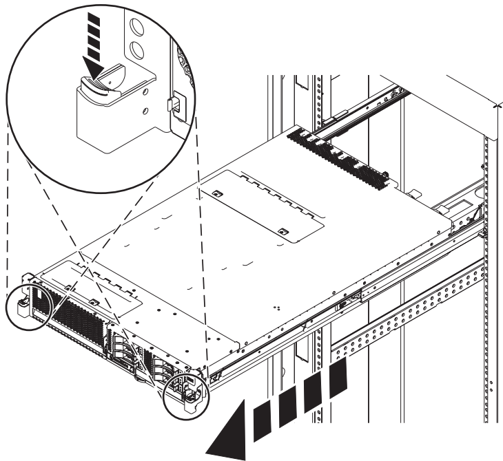
Abbildung 13. Bringen des Systems in die Serviceposition
