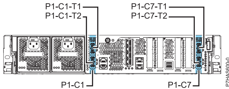
Abbildung 1. Rückansicht des Systems 8231-E2B mit den GX-Adaptersteckplätzen und Positionscodes
