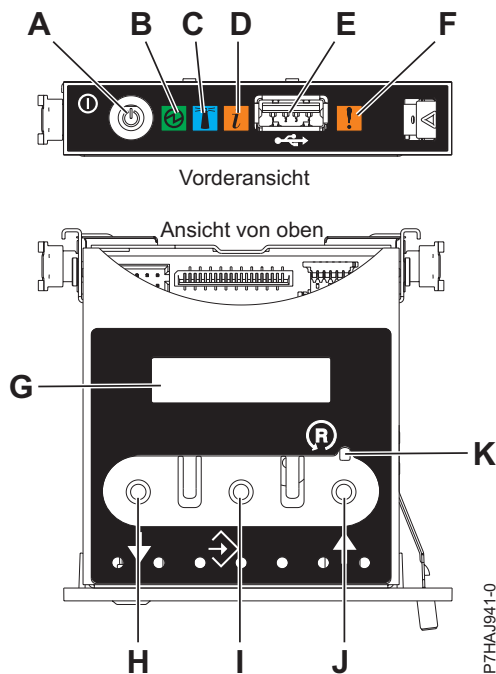
Abbildung 10. Steuerkonsole
