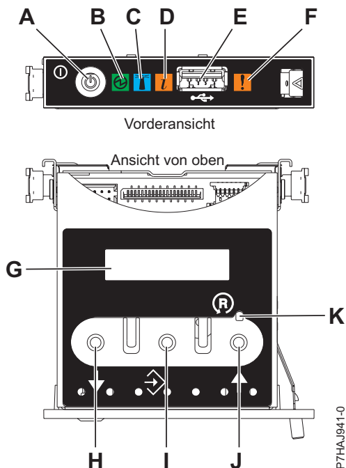
Abbildung 21. Steuerkonsole
