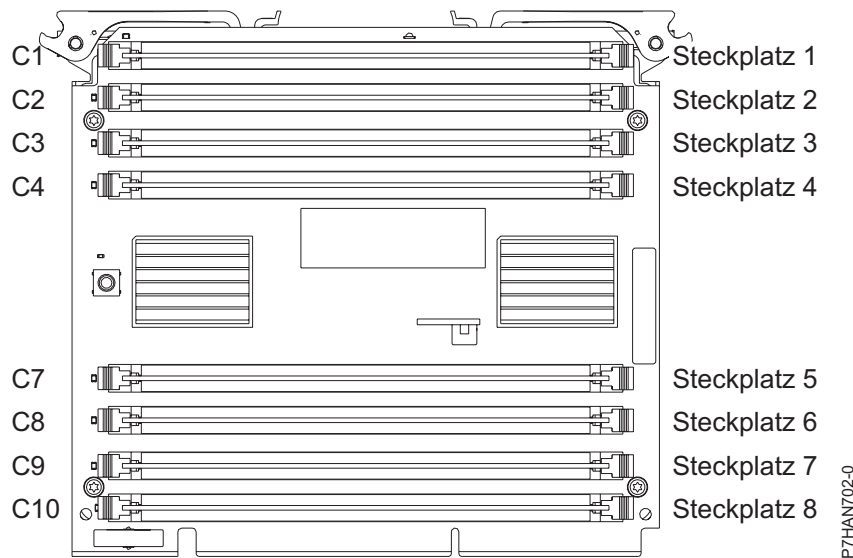
Abbildung 12. Steckplätze für Speichermodule bei 8202-E4C, 8202-E4D, 8205-E6C oder 8205-E6D
