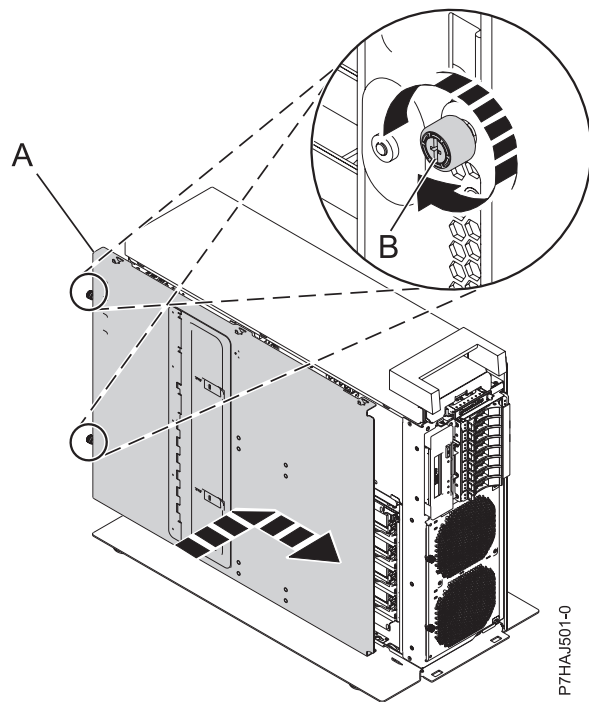
Abbildung 31. Innere Serviceabdeckung installieren
