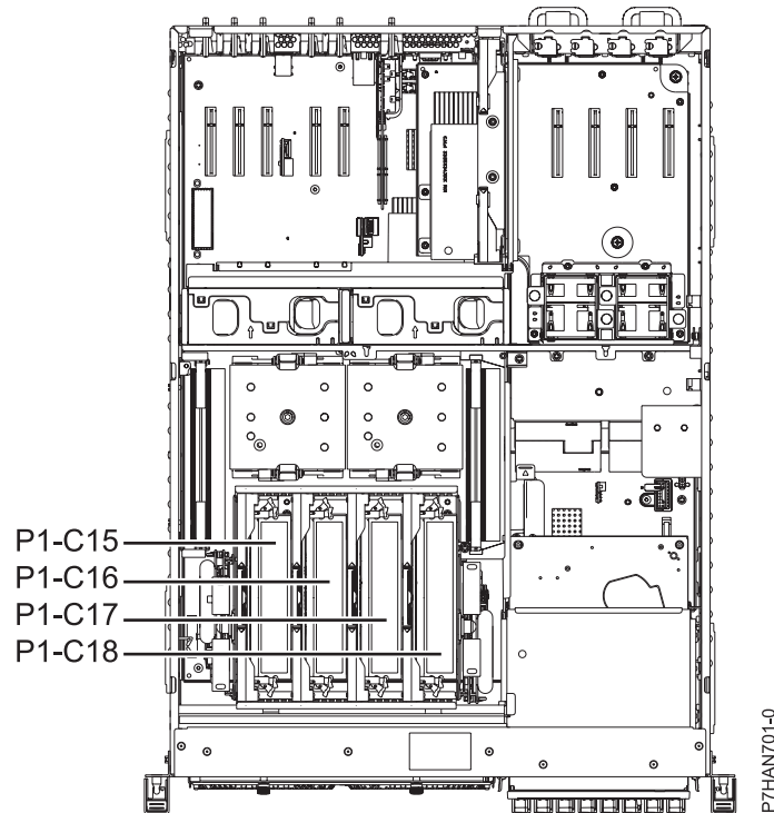
Abbildung 10. Einbaureihenfolge der Speicherriserkarten
