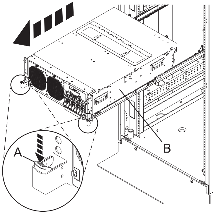
Abbildung 34. Systemeinheit in der Serviceposition verriegeln
