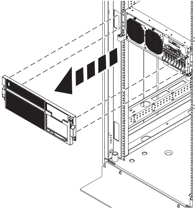
Abbildung 22. Vordere Abdeckung ausbauen
