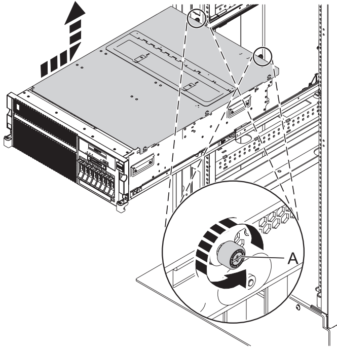
Abbildung 27. Serviceabdeckung ausbauen
