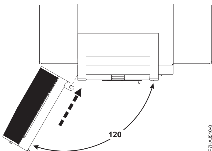
Abbildung 26. Vordere Klappe installieren
