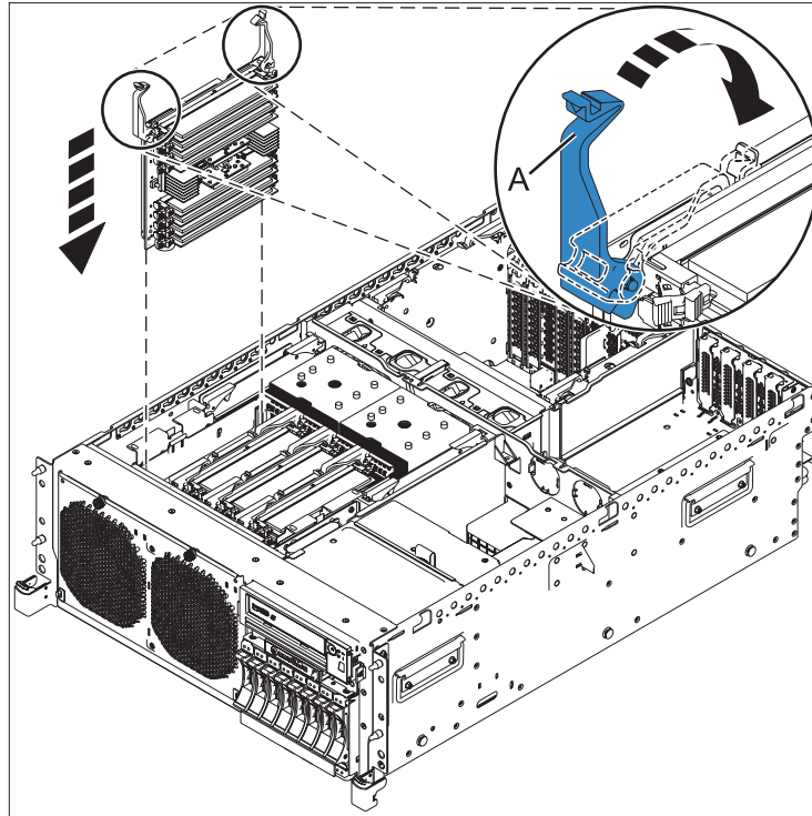
Abbildung 6. Austausch einer Speicherriserkarte
