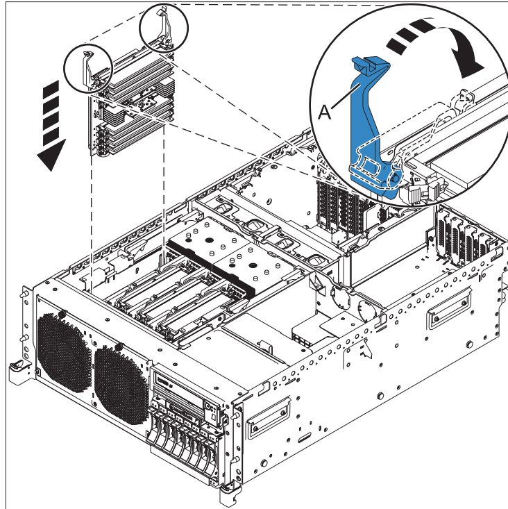
Abbildung 19. Austausch einer Speichermoduladapterkarte
