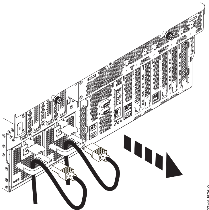
Abbildung 5. Abziehen der Netzkabel
