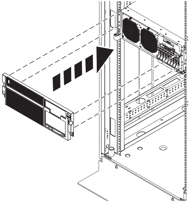
Abbildung 24. Vordere Abdeckung ausbauen
