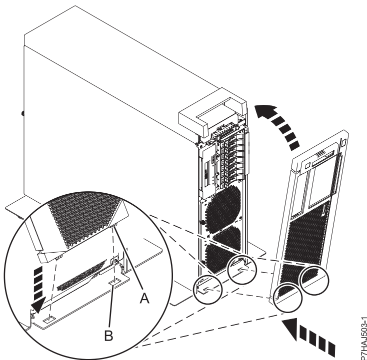
Abbildung 25. Vordere Abdeckung installieren
