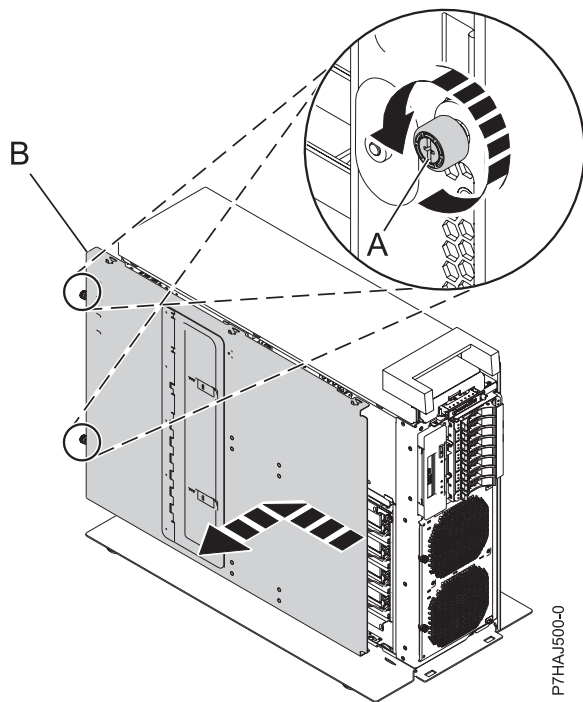
Abbildung 29. Innere Serviceabdeckung ausbauen
