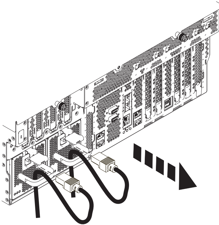
Abbildung 17. Abziehen der Netzkabel
