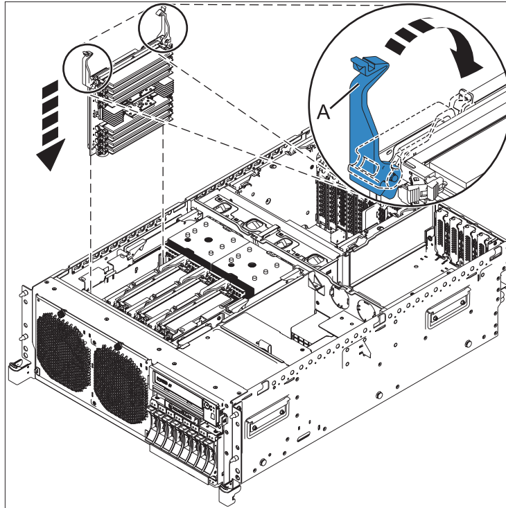
Abbildung 2. Installieren einer Speicherreiserkarte
