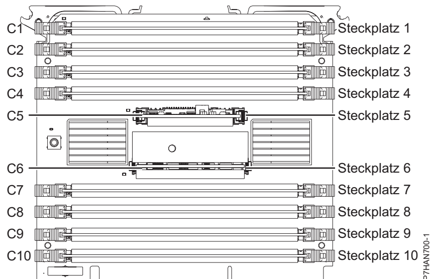
Abbildung 11. Steckplätze für Speichermodule bei 8202-E4B oder 8205-E6B
