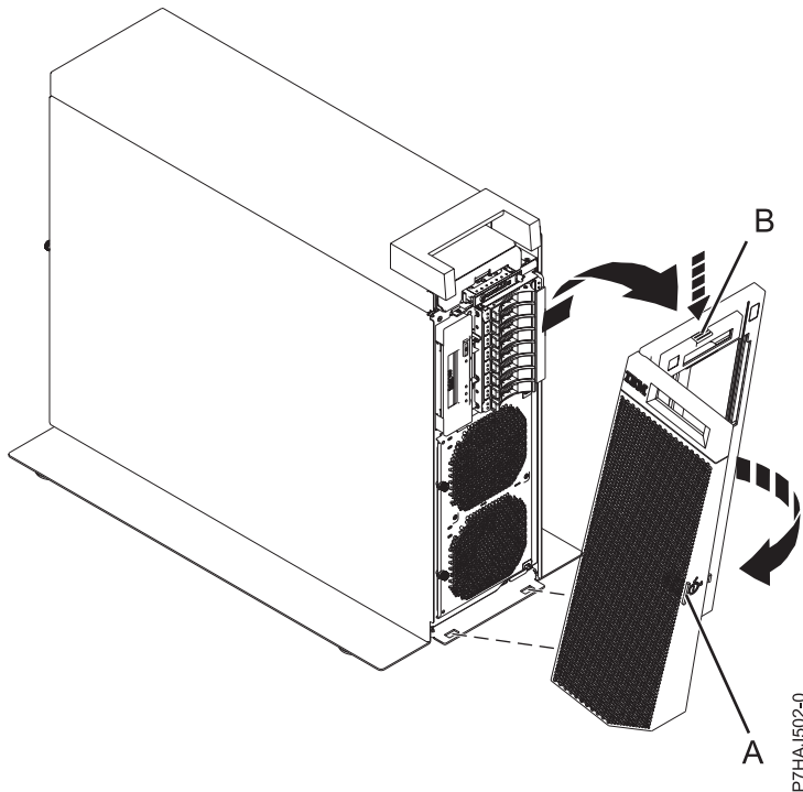
Abbildung 23. Vordere Abdeckung ausbauen
