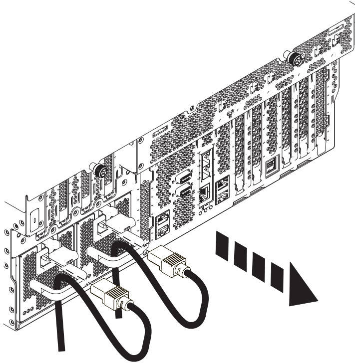
Abbildung 7. Abziehen der Netzkabel
