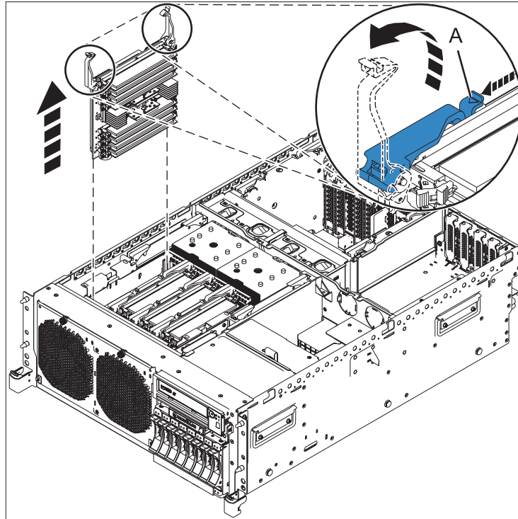
Abbildung 14. Ausbau einer Speicherriserkarte
