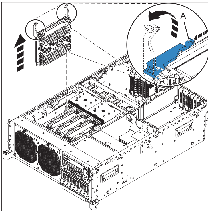
Abbildung 4. Ausbau einer Speicherriserkarte
