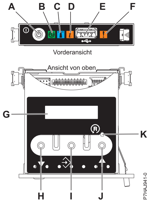
Abbildung 20. Steuerkonsole
