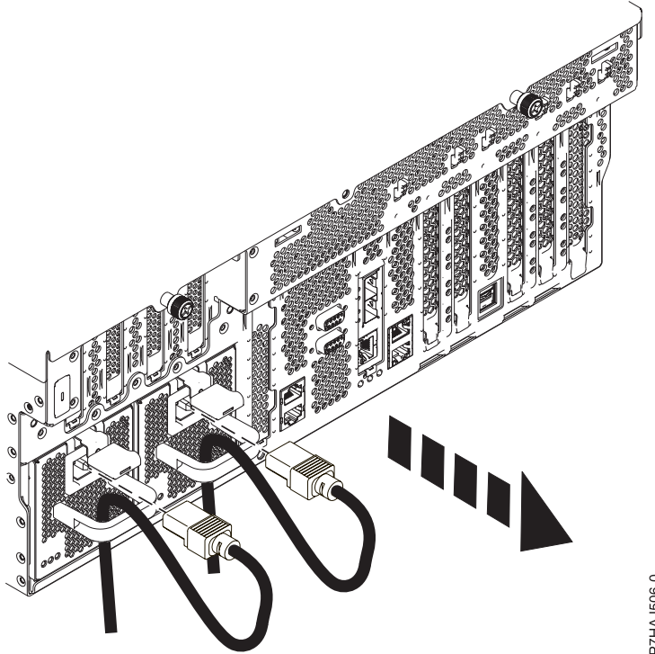
Abbildung 13. Abziehen der Netzkabel
