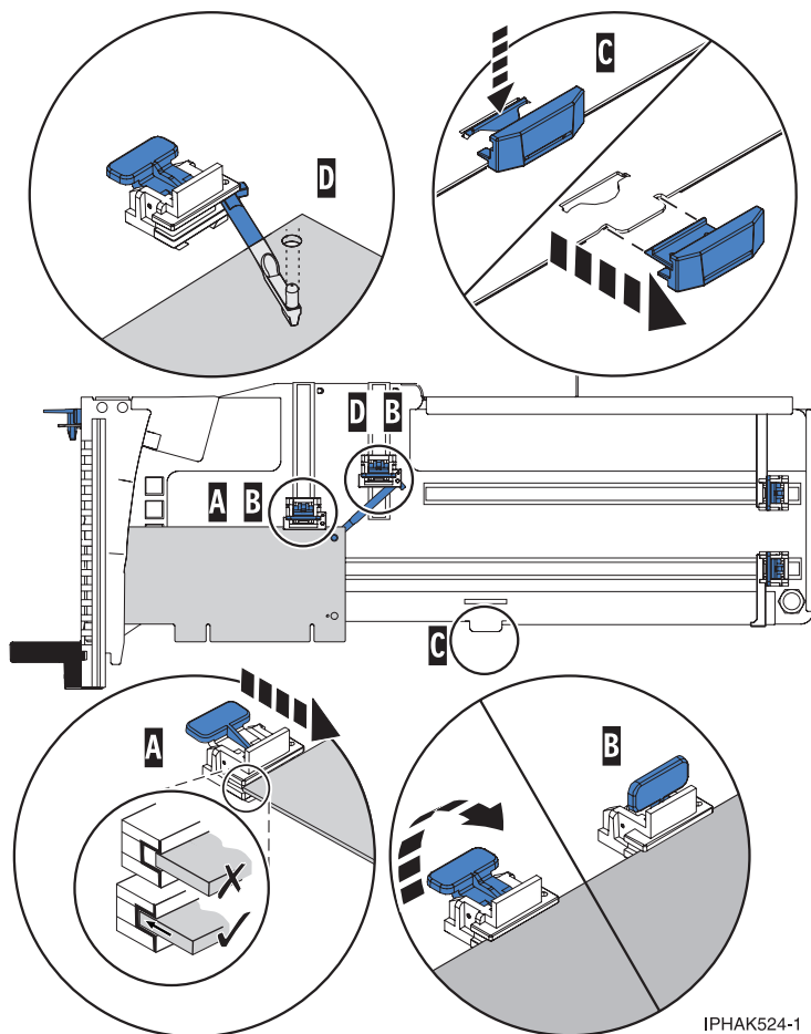
Abbildung 81. Kleiner Adapter in PCI-Adapterkassette, Halterungen und Verankerung an korrekter Position
