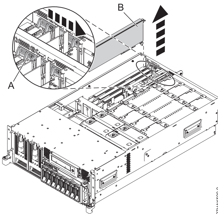
Abbildung 11. PCI-Adapter oder PCI-Adapterplatzhalterelement ausbauen - Einschubsystem
