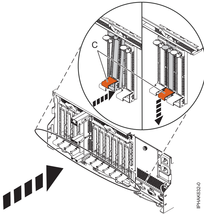
Abbildung 98. PCI-Adapterkassette installieren
