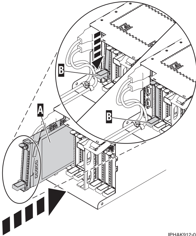
Abbildung 66. Im System installierte PCI-Adapterkassette
