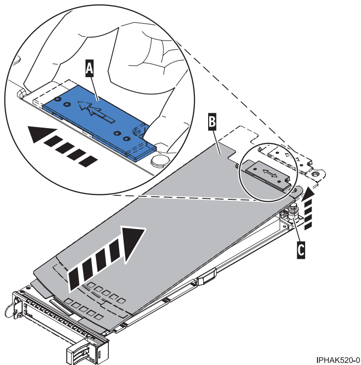
Abbildung 88. Abdeckung der PCI-Adapterkassette ausbauen
