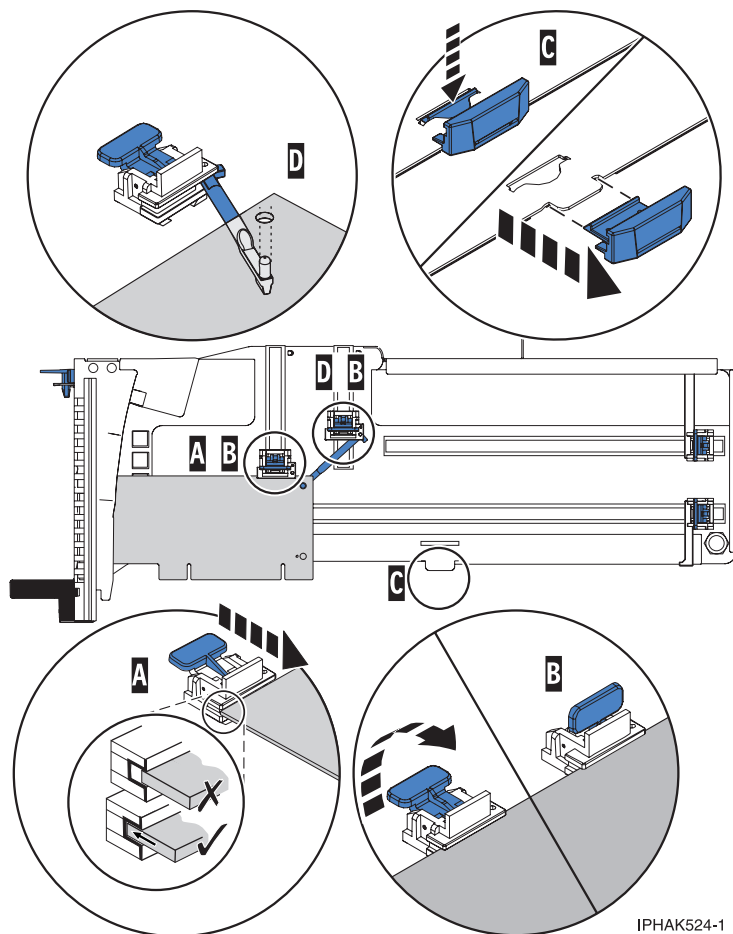
Abbildung 111. Kleiner Adapter in PCI-Adapterkassette, Halterungen und Verankerung an korrekter Position
