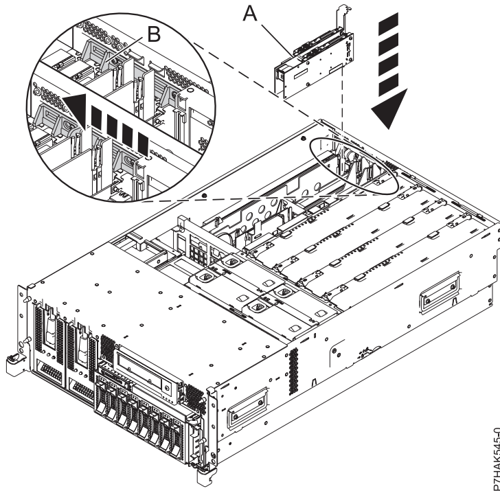
Abbildung 19. In Einschubsystem ausgetauschter PCIe-RAID- und SSD-SAS-Adapter
