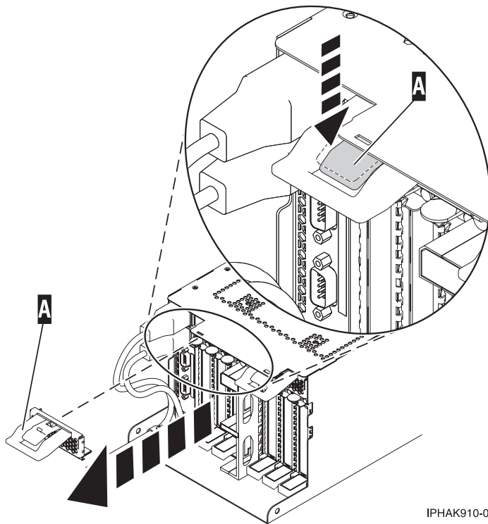
Abbildung 59. EMV-Abschirmung entfernen
