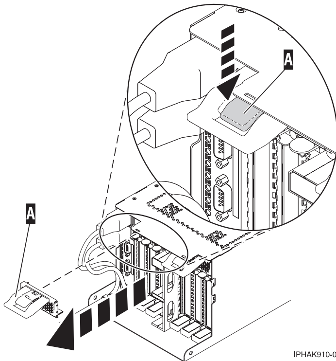
Abbildung 41. EMV-Abschirmung entfernen
