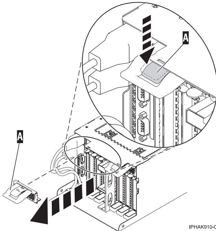
Abbildung 49. EMV-Abschirmung entfernen
