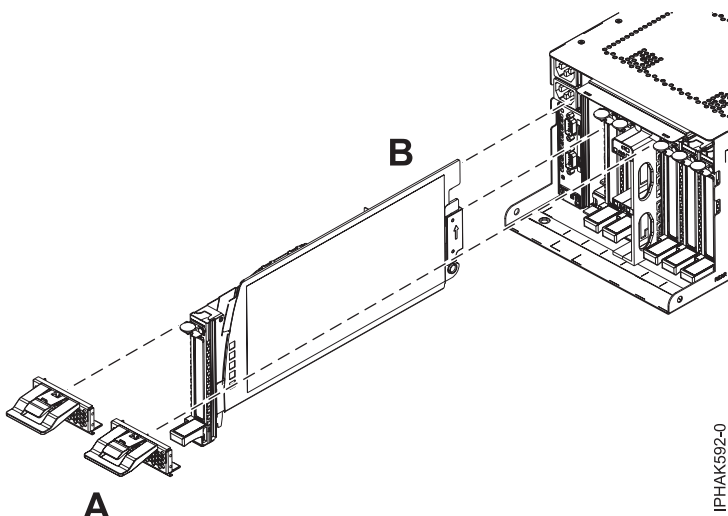
Abbildung 87. Kassette austauschen und EMV-Gitter installieren
