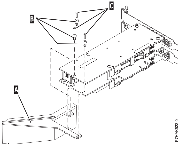
Abbildung 118. Luftklappe auf dem neuen PCIe-RAID- und SSD-SAS-Adapter installieren
