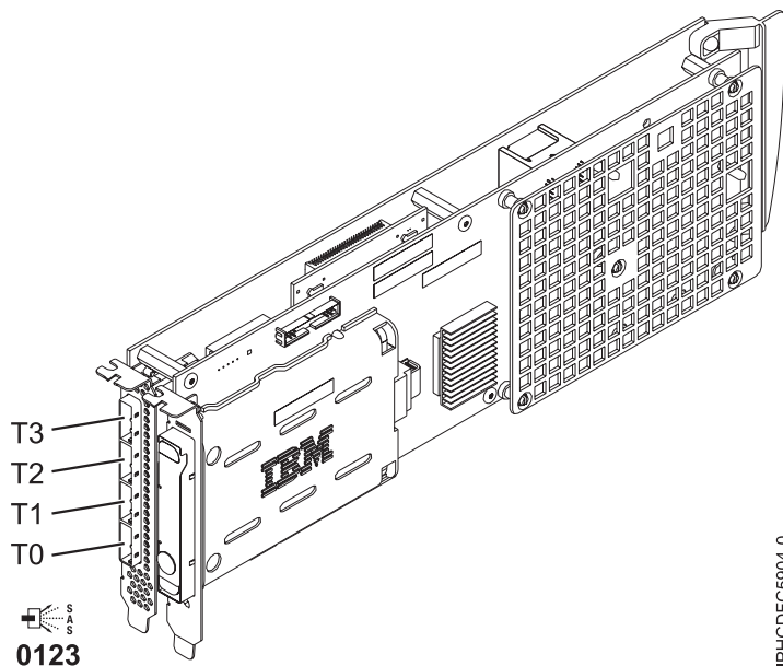
Abbildung 126. PCI-X-SAS-RAID-Adapter, DDR, 1,5 GB Cache
