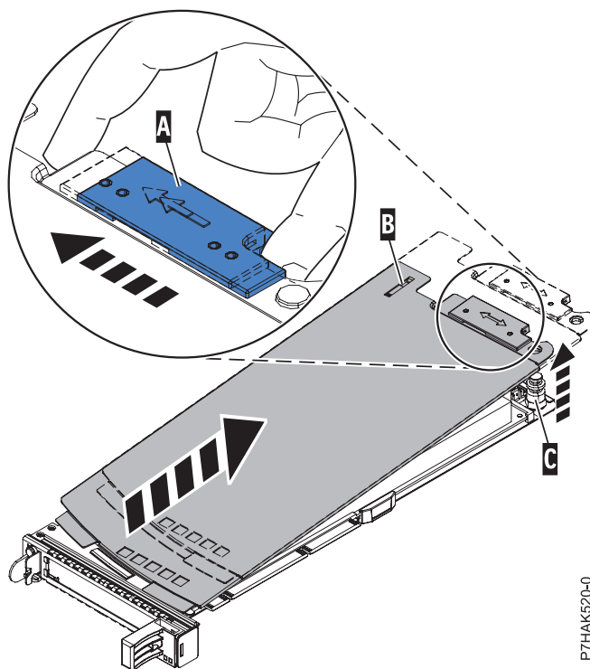
Abbildung 102. Abdeckung der PCI-Adapterkassette ausbauen
