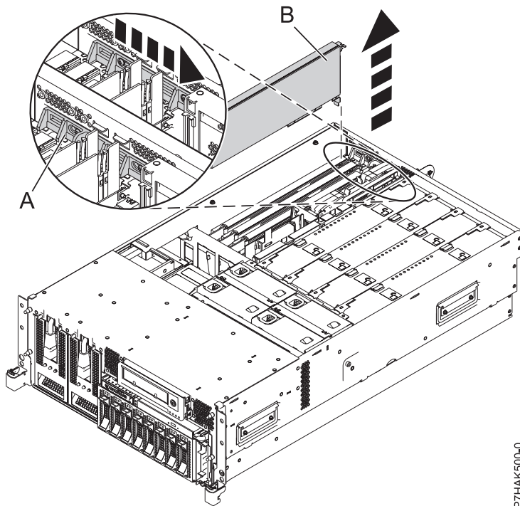
Abbildung 14. PCI-Adapter oder PCI-Adapterplatzhalterelement ausbauen - Einschubsystem
