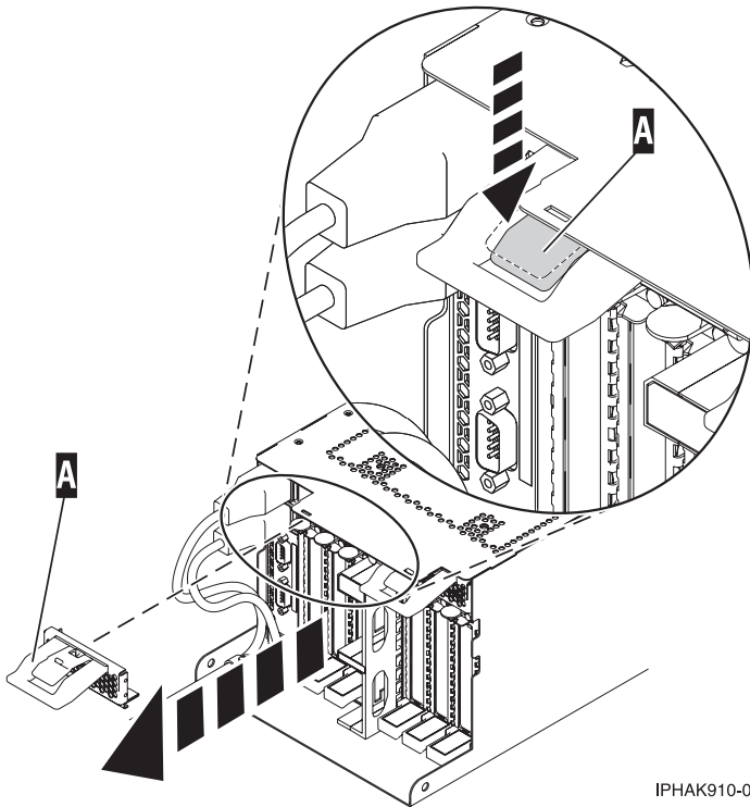
Abbildung 63. EMV-Abschirmung entfernen
