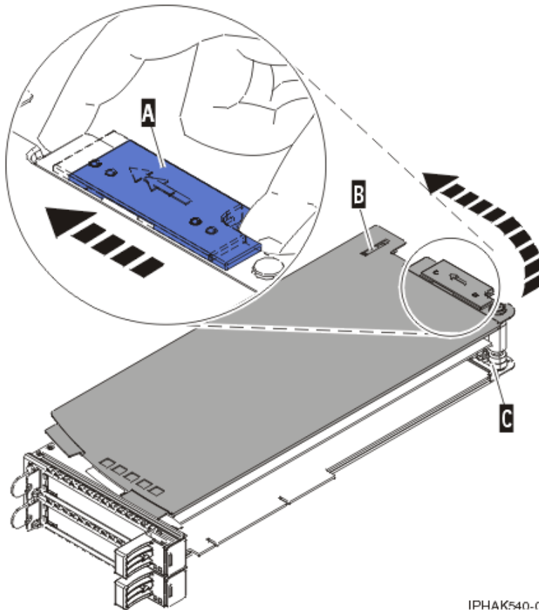
Abbildung 93. Abdeckung der PCI-Adapterkassette anbringen
