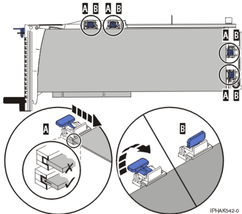
Abbildung 96. Langer Adapter in PCI-Adapterkassette, Halterungen und Stabilisator an korrekter Position
