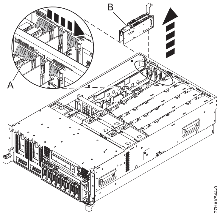
Abbildung 26. Aus Einschubsystem ausgebauter PCI-RAID- und SSD-SAS-Adapter
