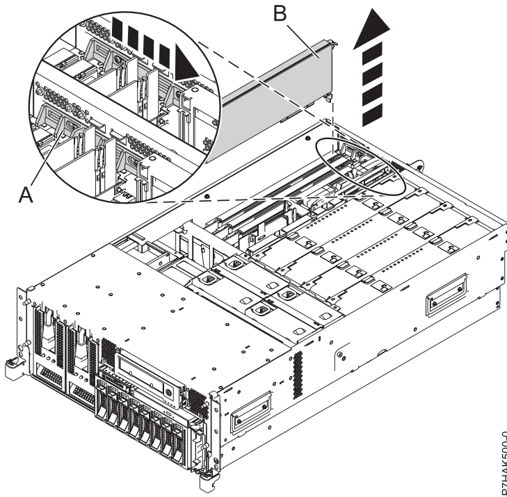
Abbildung 38. PCI-Adapter oder PCI-Adapterplatzhalterelement ausbauen - Einschubsystem
