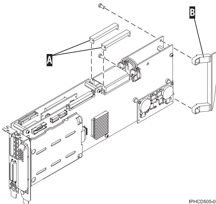
Abbildung 124. Adapter für Platzierung in Kassette vorbereiten
