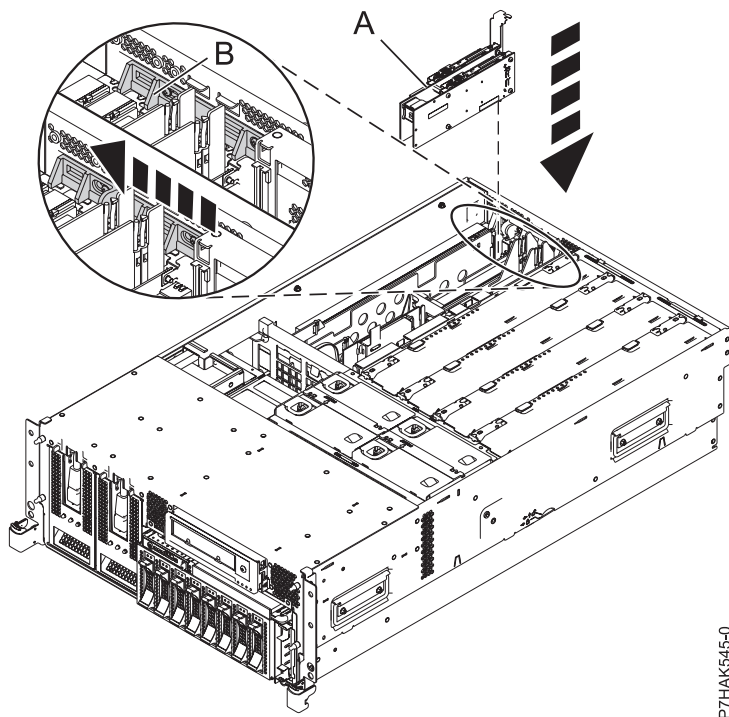
Abbildung 23. In Einschubsystem ausgetauschter PCI-RAID- und SSD-SAS-Adapter
