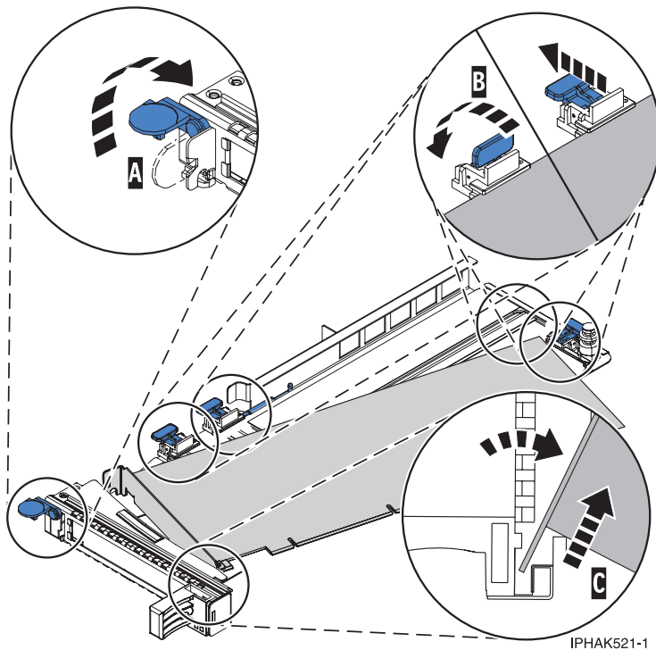
Abbildung 103. Adapter aus PCI-Adapterkassette ausbauen
