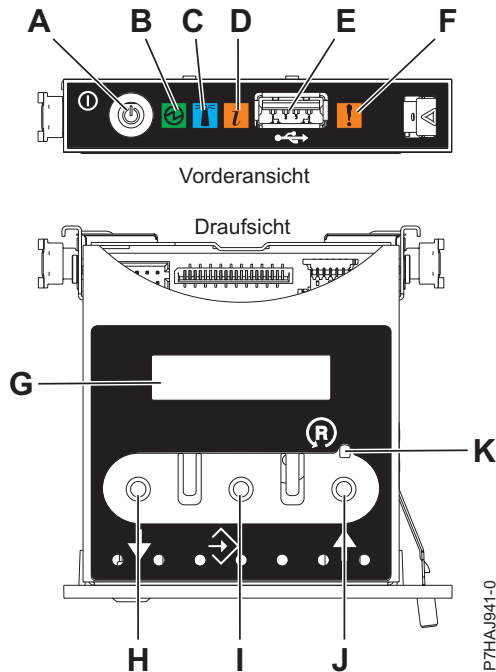
Abbildung 127. Steuerkonsole
