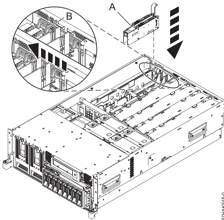
Abbildung 30. In Einschubsystem ausgetauschter PCI-RAID- und SSD-SAS-Adapter
