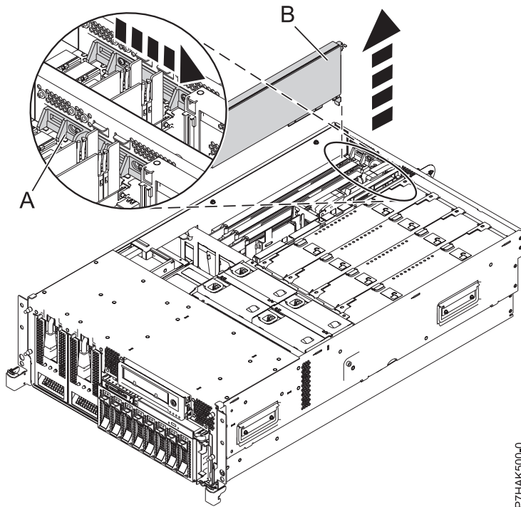
Abbildung 35. PCI-Adapter oder PCI-Adapterplatzhalterelement ausbauen - Einschubsystem
