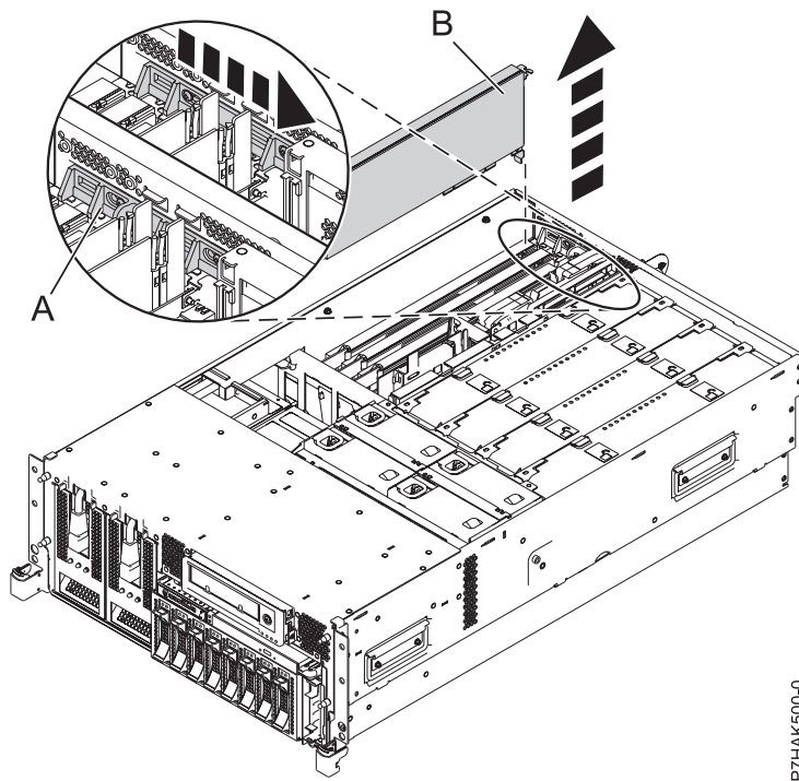
Abbildung 24. PCI-Adapter oder PCI-Adapterplatzhalterelement ausbauen - Einschubsystem
