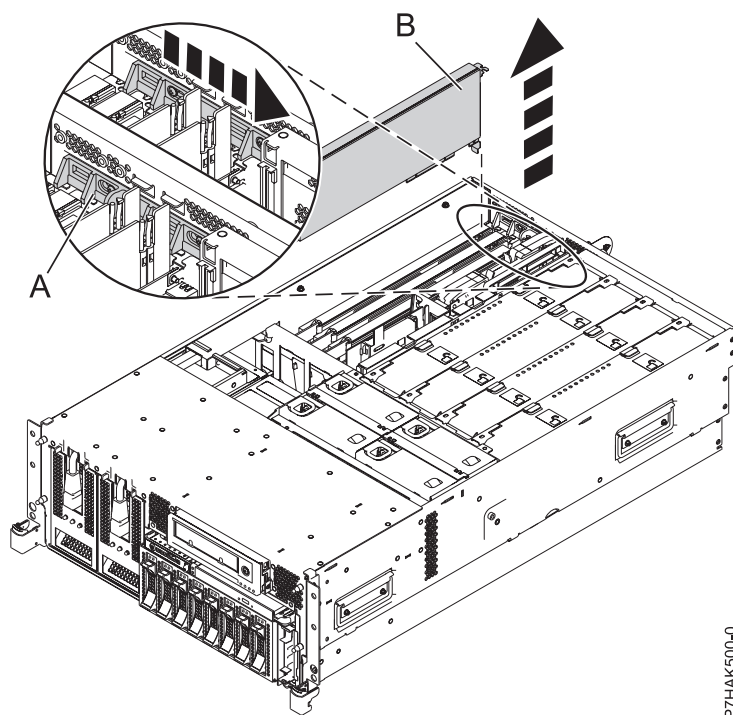
Abbildung 18. PCI-Adapter oder PCI-Adapterplatzhalterelement ausbauen - Einschubsystem
