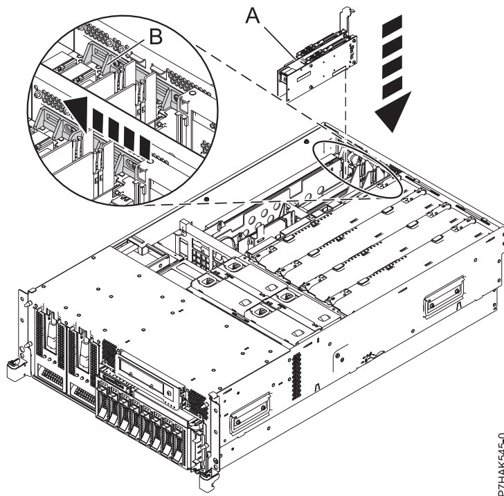
Abbildung 32. In Einschubsystem ausgetauschter PCI-RAID- und SSD-SAS-Adapter
