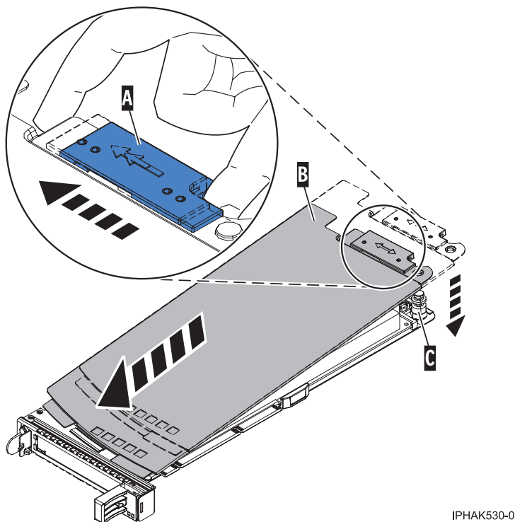
Abbildung 86. Abdeckung der PCI-Adapterkassette anbringen
