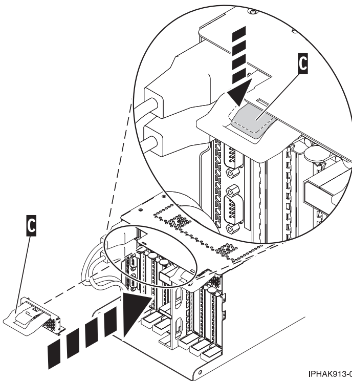
Abbildung 71. EMV-Abschirmung des PCI-Adapters in geschlossene Position bringen
