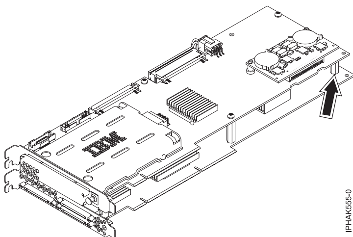
Abbildung 125. Abstandshalter ausbauen
