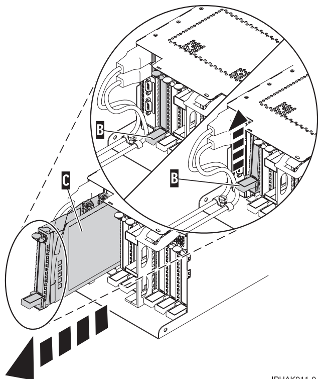
Abbildung 64. PCI-Adapterkassette aus Systemeinheit ausbauen
