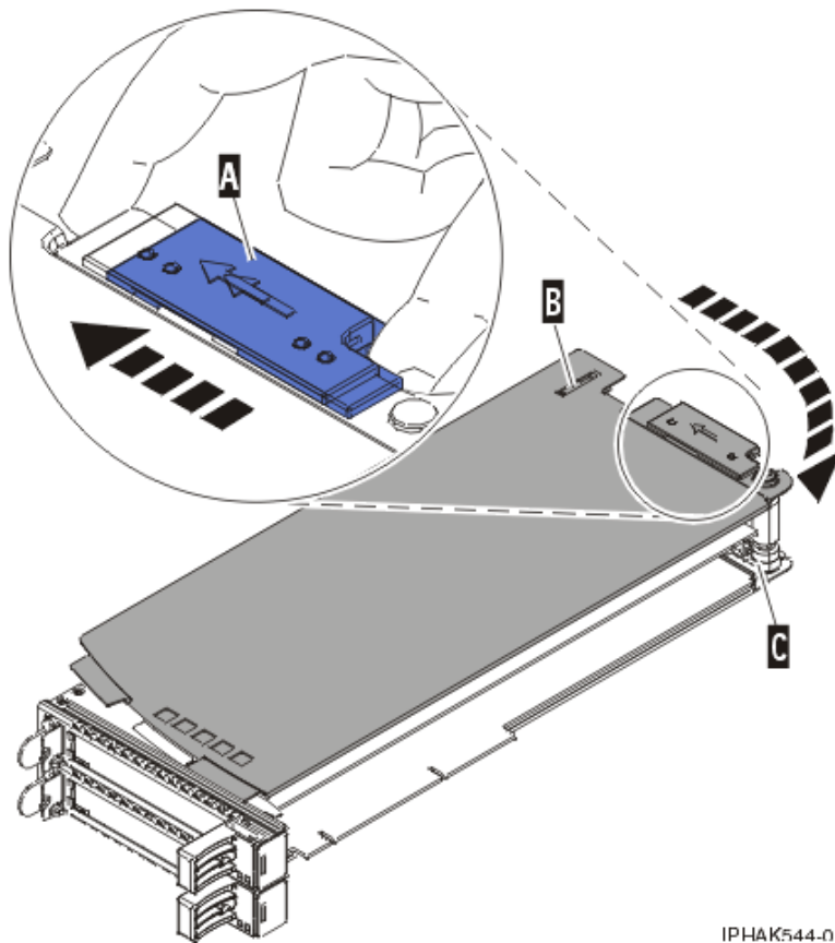
Abbildung 113. Abdeckung der PCI-Adapterkassette ausbauen
