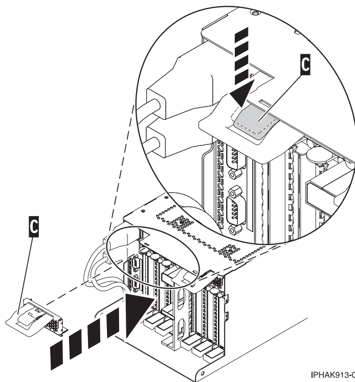
Abbildung 56. EMV-Abschirmung des PCI-Adapters in geschlossene Position bringen
