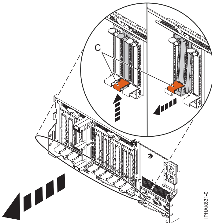
Abbildung 101. PCI-Adapterkassette ausbauen
