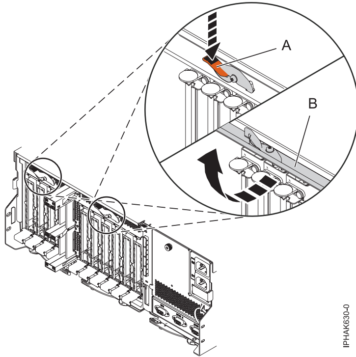
Abbildung 100. Klappe öffnen
