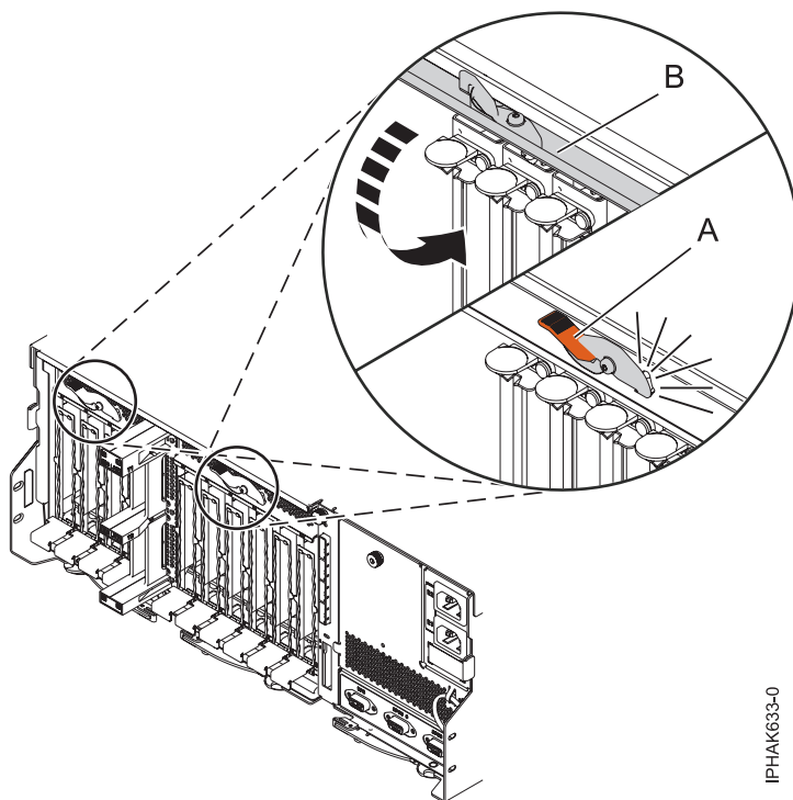
Abbildung 99. Klappe schließen
