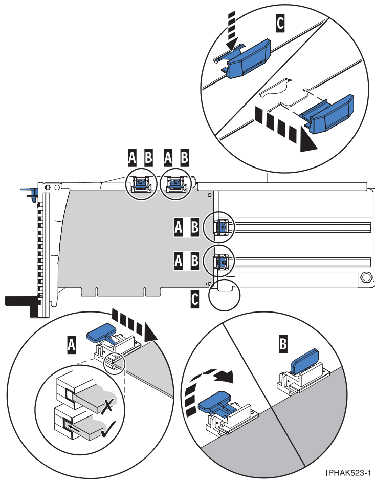
Abbildung 80. Adapter mit mittlerer Länge in PCI-Adapterkassette, Halterungen an korrekter Position
