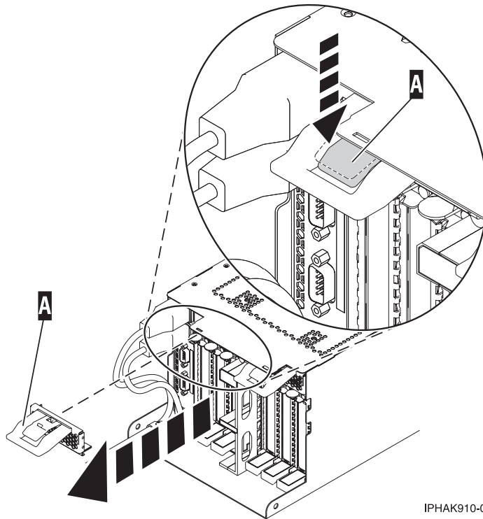
Abbildung 65. EMV-Abschirmung entfernen
