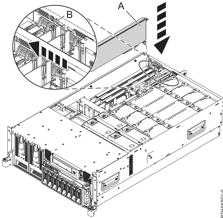
Abbildung 4. PCI-Adapter austauschen - Einschubsystem
