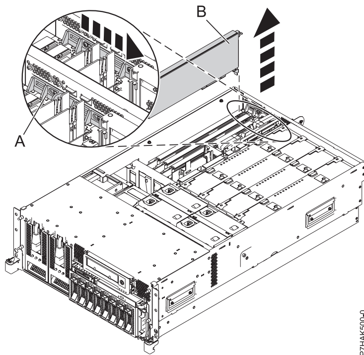
Abbildung 3. PCI-Adapter oder PCI-Adapterplatzhalterelement ausbauen - Einschubsystem
