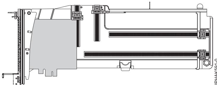
Abbildung 85. Adapter in Kassette (Seitenansicht)
