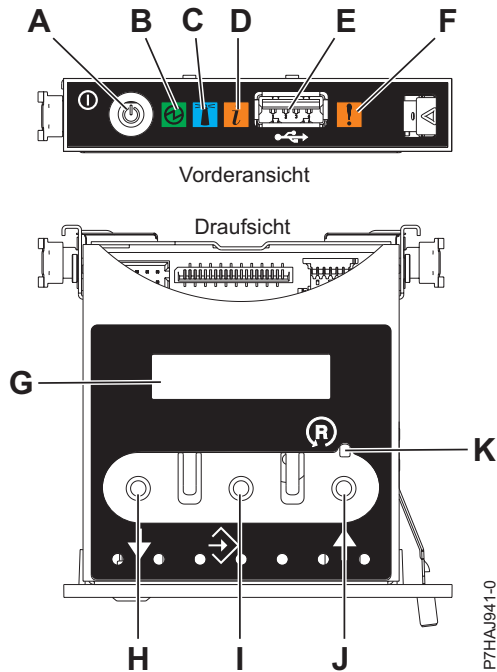
Abbildung 128. Steuerkonsole
