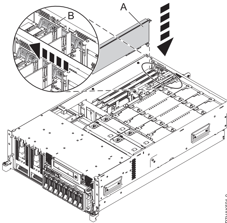
Abbildung 15. PCI-Adapter austauschen - Einschubsystem
