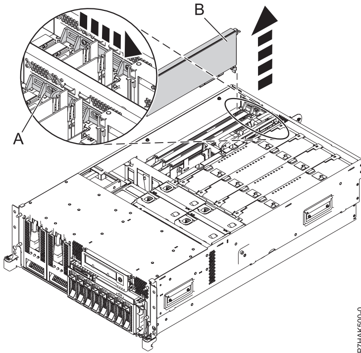
Abbildung 12. PCI-Adapter oder PCI-Adapterplatzhalterelement ausbauen - Einschubsystem
