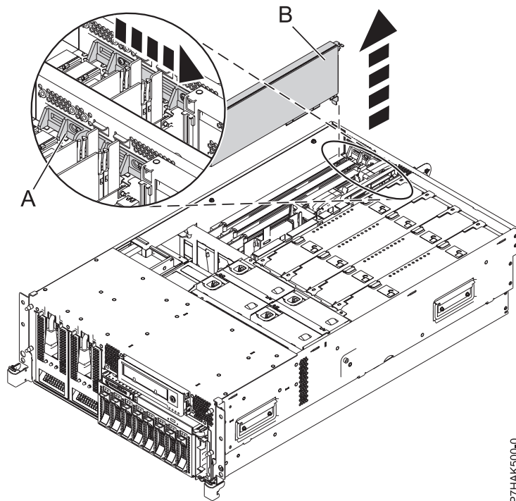
Abbildung 10. PCI-Adapter oder PCI-Adapterplatzhalterelement ausbauen - Einschubsystem
