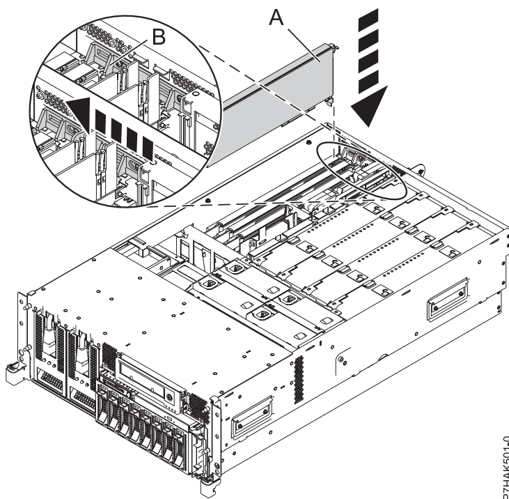
Abbildung 40. PCI-Adapter austauschen - Einschubsystem
