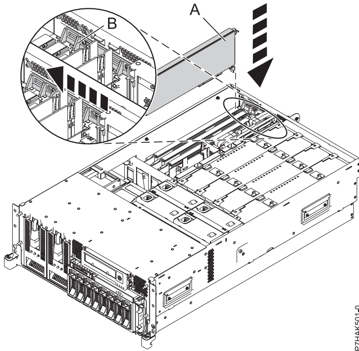
Abbildung 17. PCI-Adapter austauschen - Einschubsystem
