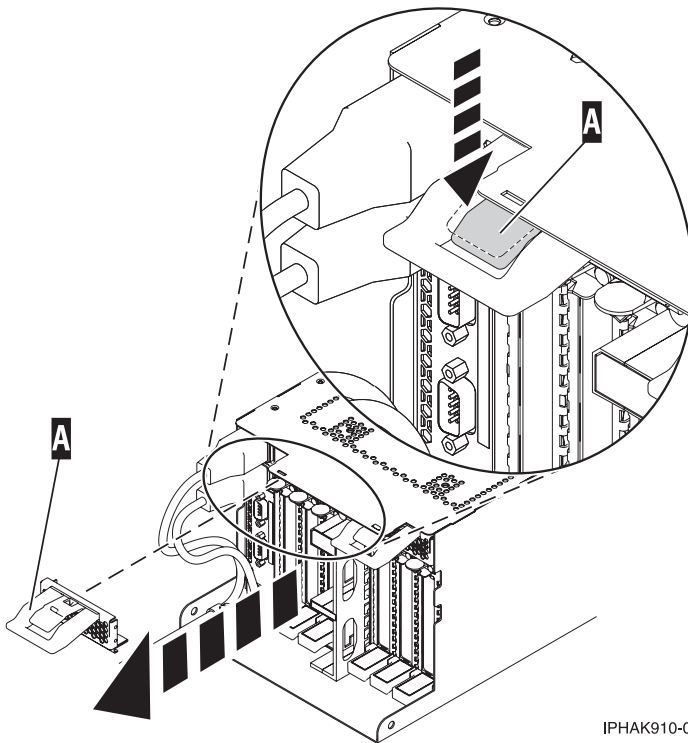
Abbildung 68. EMV-Abschirmung entfernen
