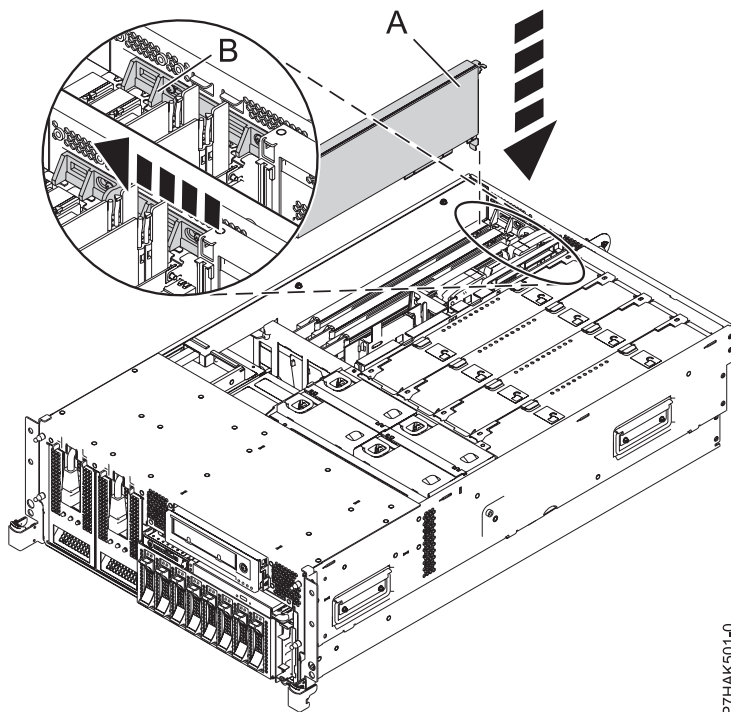
Abbildung 13. PCI-Adapter austauschen - Einschubsystem
