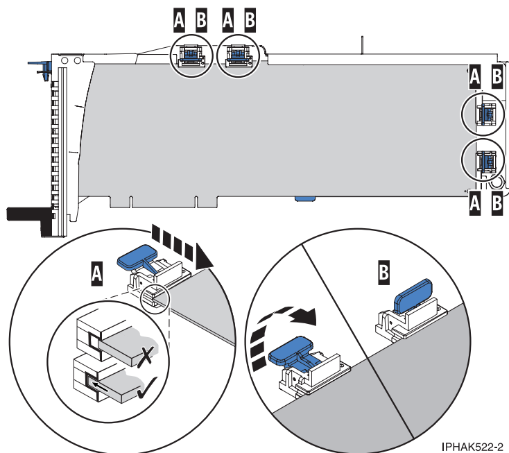
Abbildung 109. Großer Adapter in PCI-Adapterkassette, Halterungen und Stabilisator an korrekter Position
