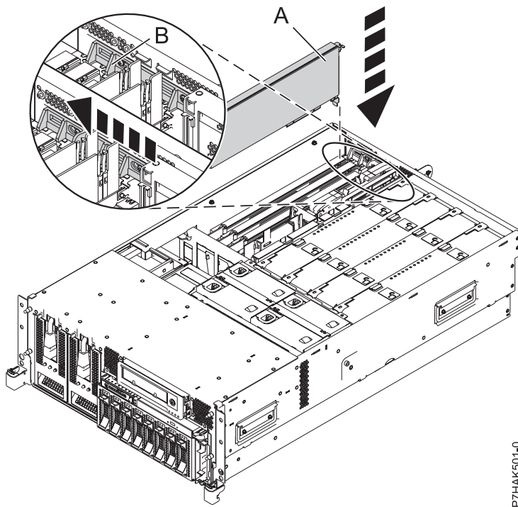
Abbildung 16. PCI-Adapter austauschen - Einschubsystem
