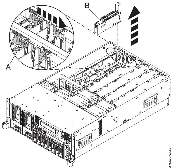
Abbildung 27. Aus Einschubsystem ausgebauter PCI-RAID- und SSD-SAS-Adapter
