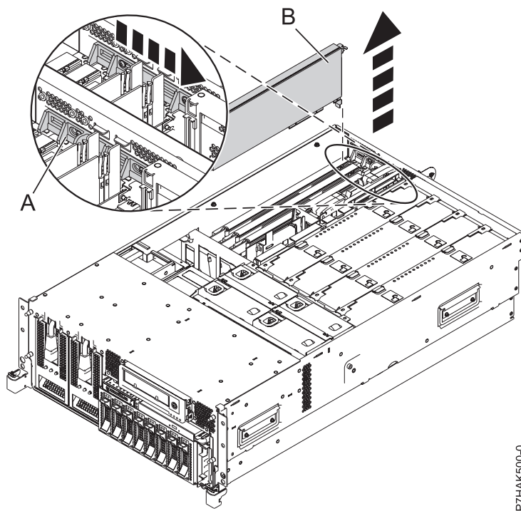
Abbildung 1. PCI-Adapter oder PCI-Adapterplatzhalterelement ausbauen - Einschubsystem
