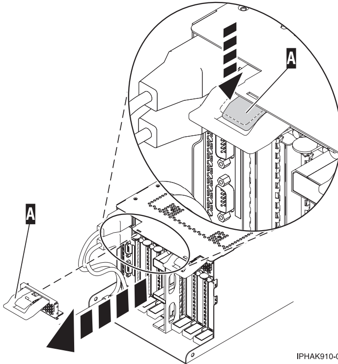
Abbildung 53. EMV-Abschirmung entfernen
