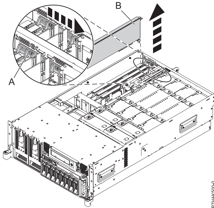
Abbildung 22. PCI-Adapter oder PCI-Adapterplatzhalterelement ausbauen - Einschubsystem
