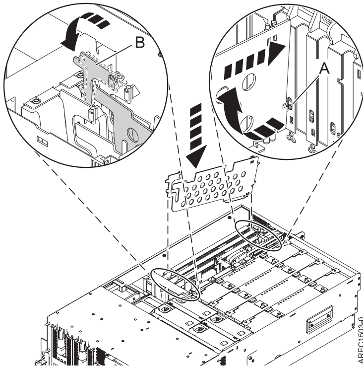
Abbildung 39. PCI-Adaptertrennplatte in Systemeinheit installieren
