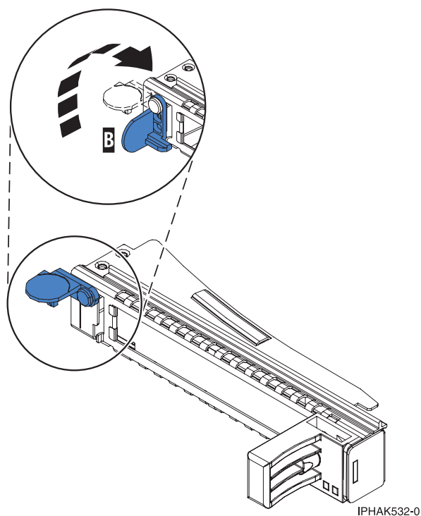
Abbildung 77. Kassettenhalteklemme in geöffneter Position
