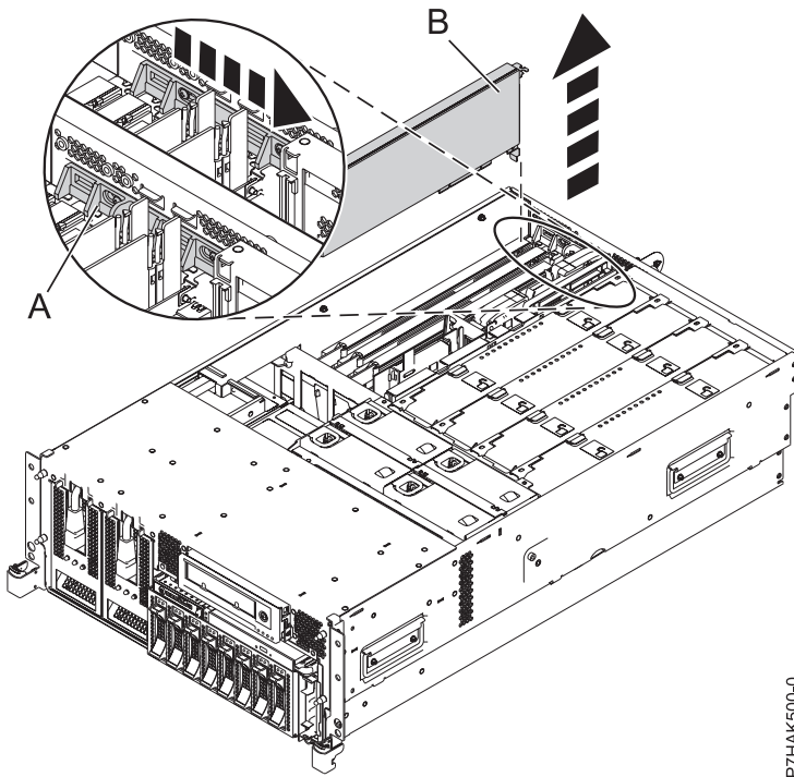
Abbildung 31. PCI-Adapter oder PCI-Adapterplatzhalterelement ausbauen - Einschubsystem
