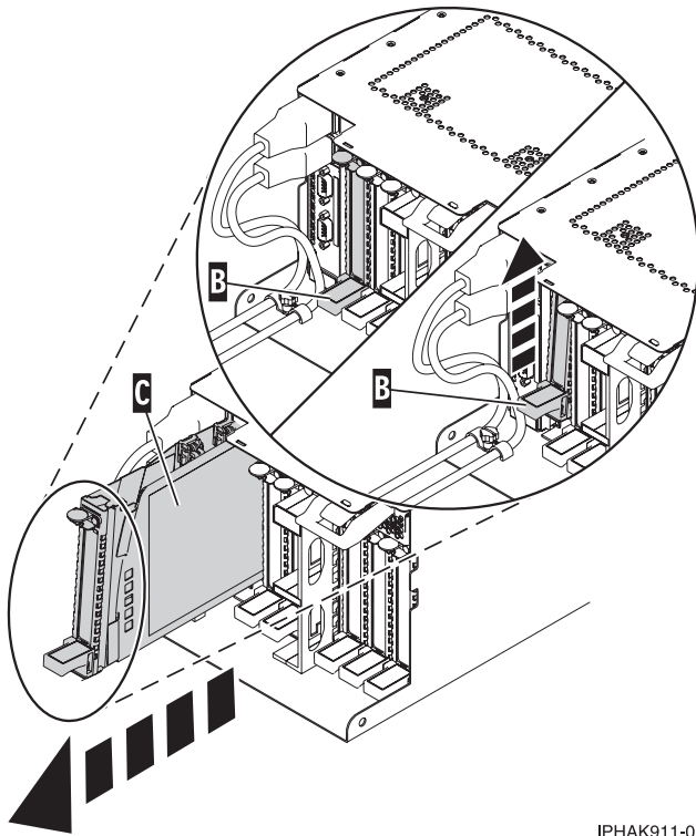
Abbildung 58. PCI-Adapterkassette aus Systemeinheit ausbauen
