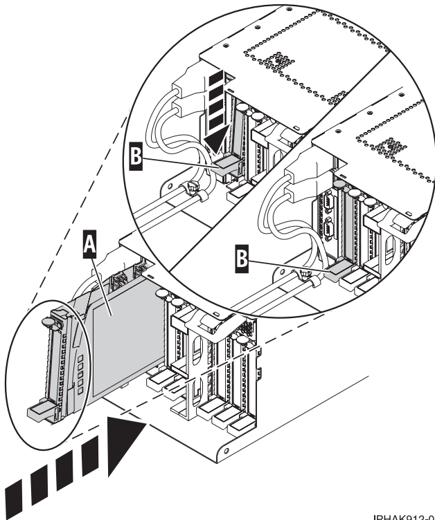
Abbildung 70. In Systemeinheit installierte PCI-Adapterkassette
