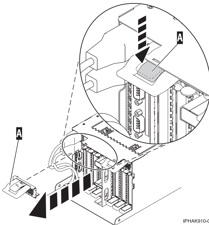
Abbildung 72. EMV-Abschirmung entfernen
