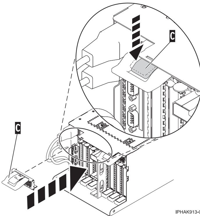
Abbildung 67. EMV-Abschirmung des PCI-Adapters in geschlossene Position bringen
