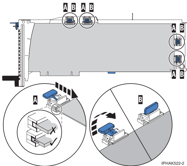
Abbildung 79. Großer Adapter in PCI-Adapterkassette, Halterungen und Stabilisator an korrekter Position
