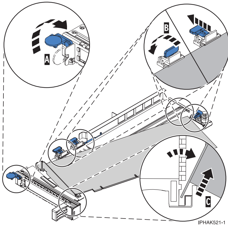
Abbildung 89. Adapter aus PCI-Adapterkassette ausbauen
