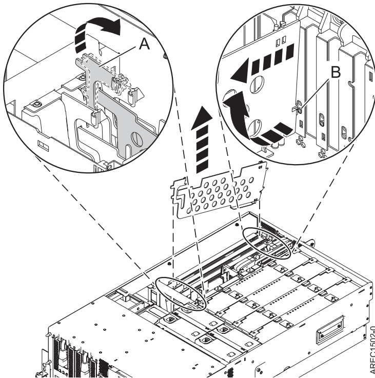
Abbildung 36. PCI-Adaptertrennplatte aus Systemeinheit ausbauen
