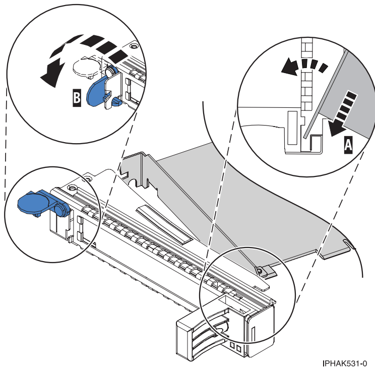
Abbildung 78. PCI-Adapter aus PCI-Adapterkassette mit einfacher Breite ausbauen
