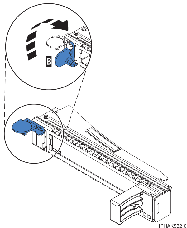
Abbildung 56. Kassettenhalteklemme in geöffneter Position
