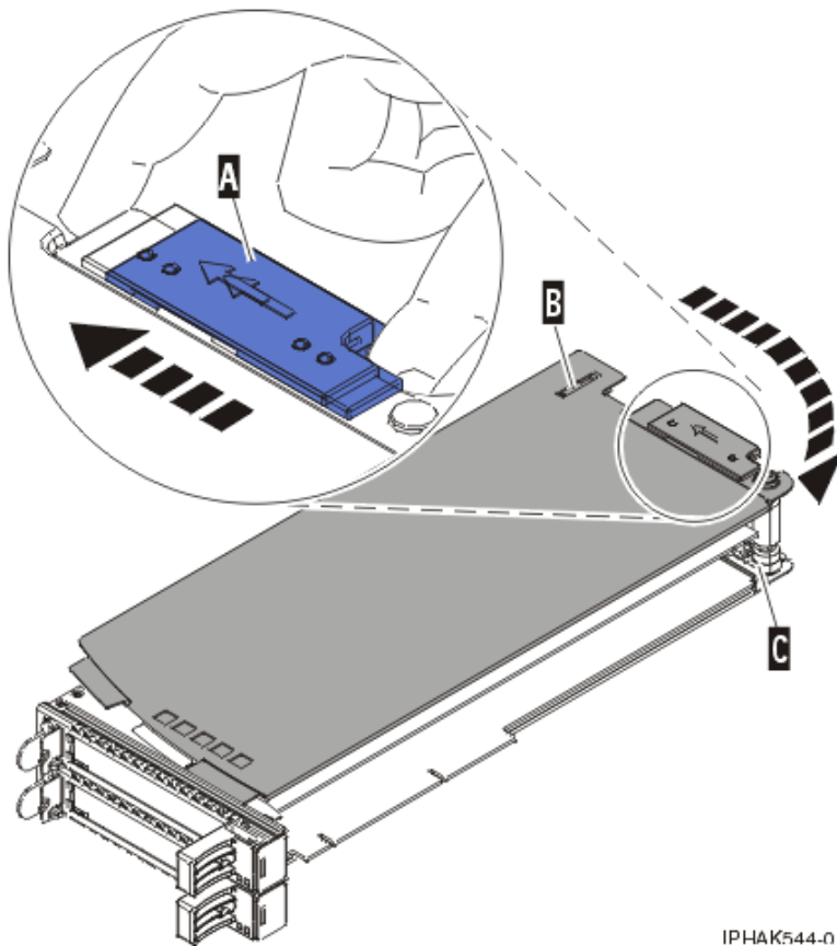
Abbildung 73. Abdeckung der PCI-Adapterkassette ausbauen
