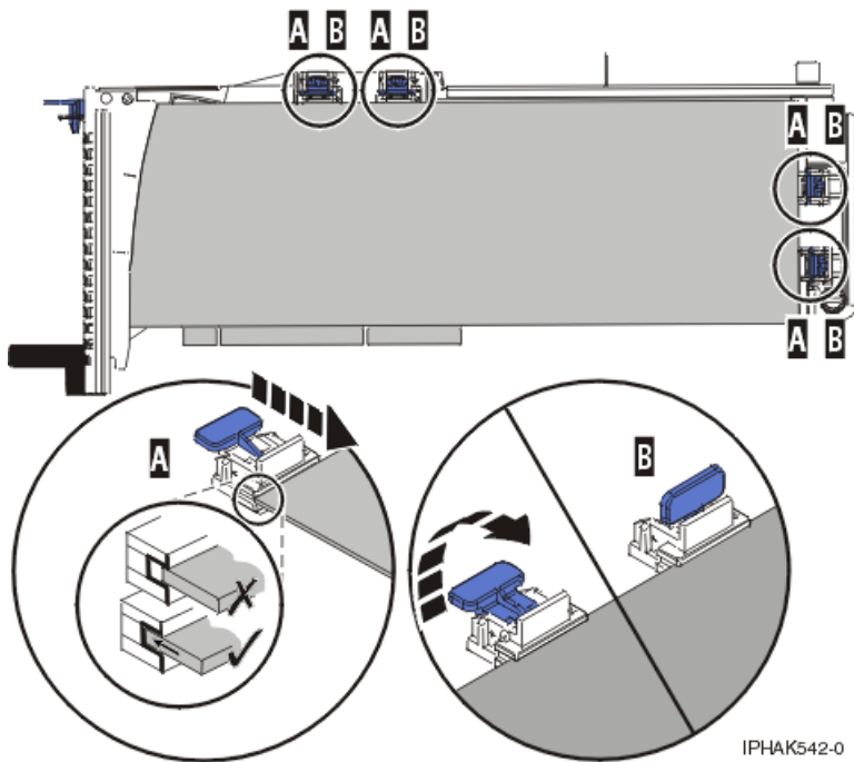
Abbildung 75. Langer Adapter in PCI-Adapterkassette, Halterungen und Stabilisator an korrekter Position
