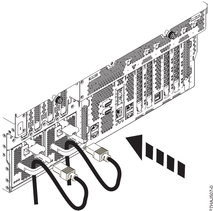
Abbildung 124. Netzkabel anschließen
