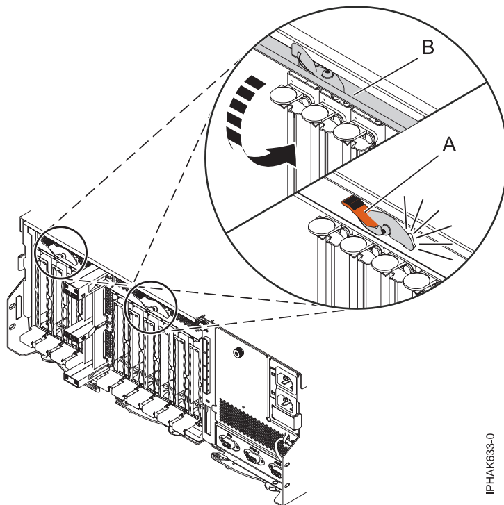
Abbildung 78. Klappe schließen
