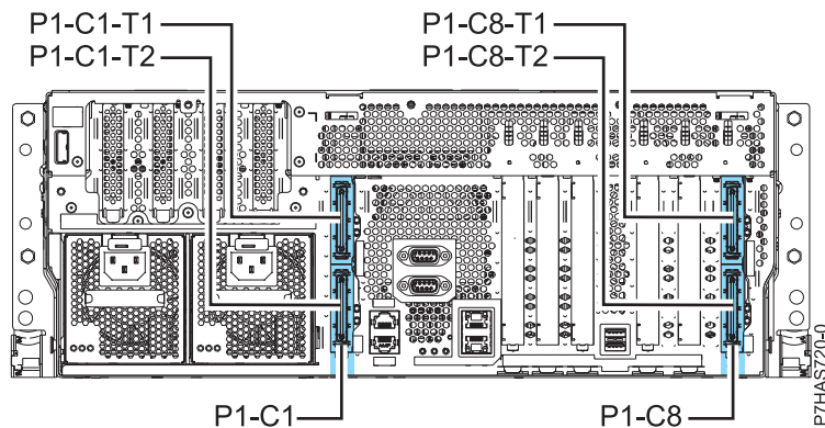
Abbildung 37. Steckplätze P1-C1 und P1-C8 - Rückansicht
