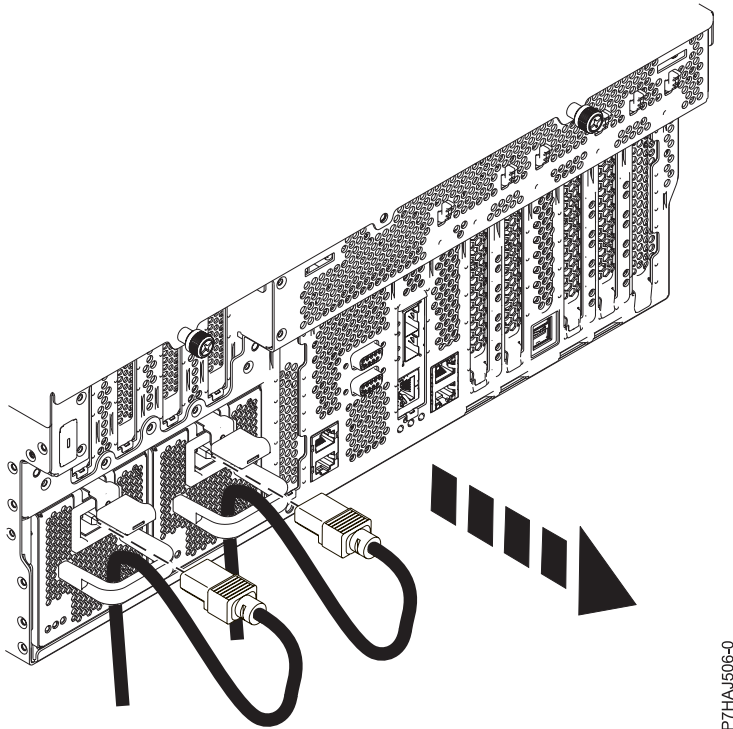
Abbildung 16. Netzkabel abziehen
