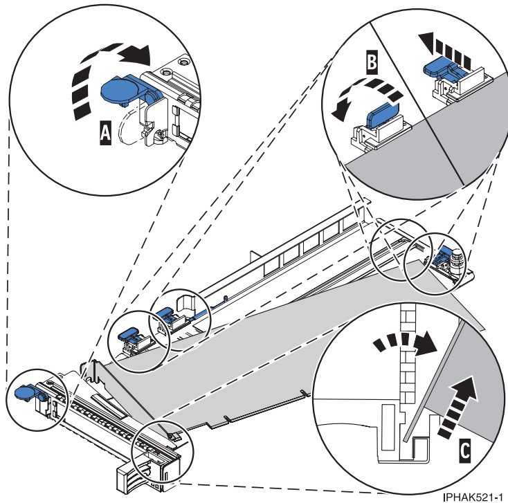
Abbildung 68. Adapter aus PCI-Adapterkassette ausbauen
