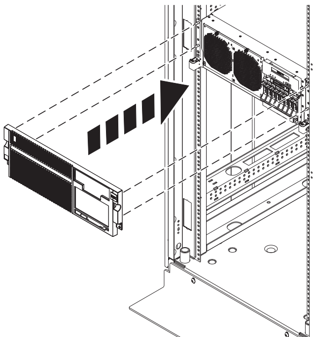
Abbildung 109. Vordere Abdeckung installieren
