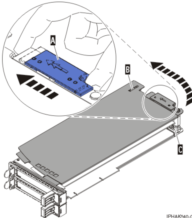
Abbildung 76. Abdeckung der PCI-Adapterkassette anbringen
