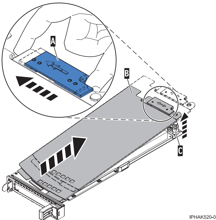
Abbildung 67. Abdeckung der PCI-Adapterkassette ausbauen
