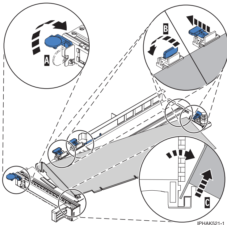
Abbildung 82. Adapter aus PCI-Adapterkassette ausbauen
