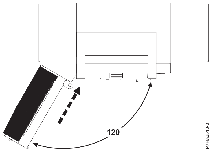
Abbildung 111. Vordere Klappe installieren
