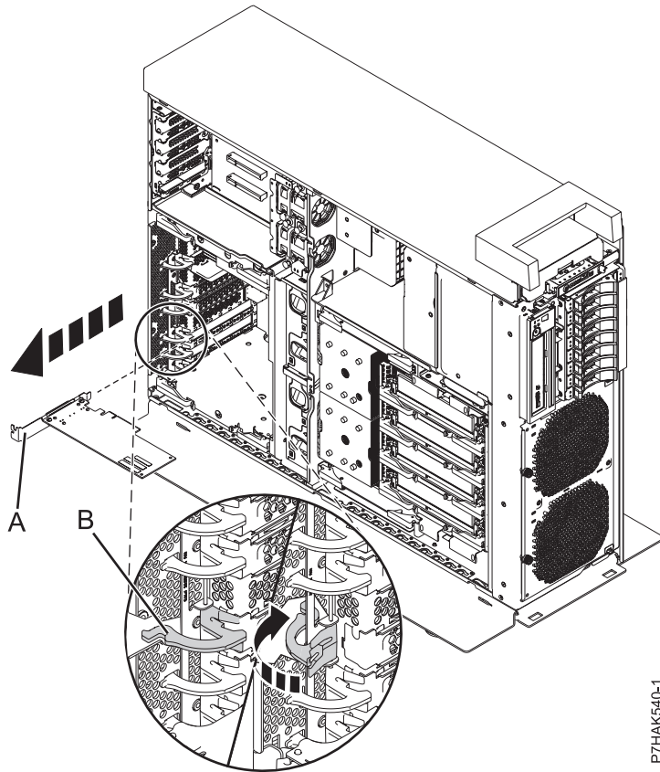
Abbildung 8. Ausbau eines PCI-Adapters aus einem Standalone-System
