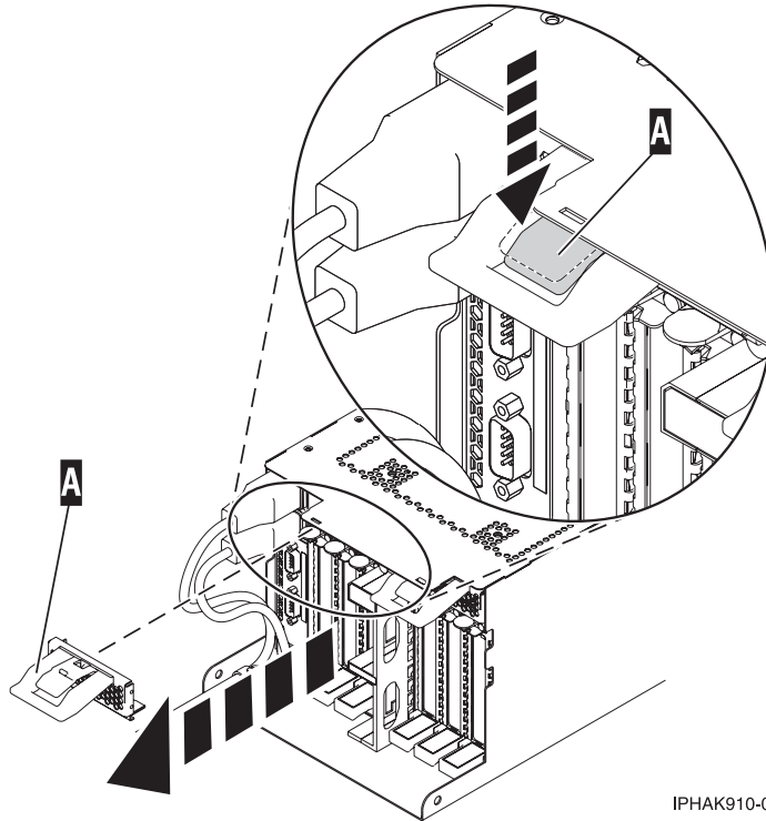
Abbildung 51. EMV-Abschirmung entfernen
