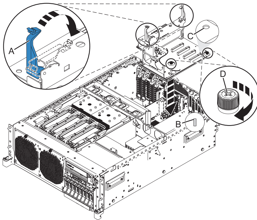
Abbildung 43. Austausch einer Erweiterungseinheit bei einem Einschubsystem
