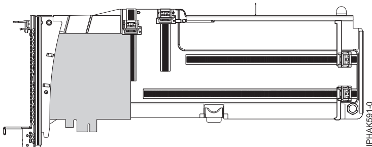
Abbildung 64. Adapter in Kassette (Seitenansicht)
