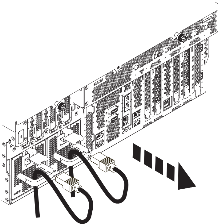
Abbildung 35. Netzkabel abziehen
