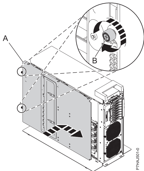
Abbildung 116. Innere Serviceabdeckung installieren
