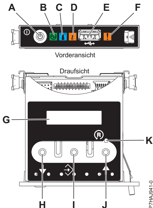
Abbildung 125. Steuerkonsole
