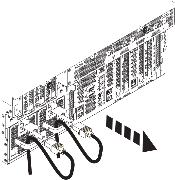
Abbildung 26. Netzkabel abziehen
