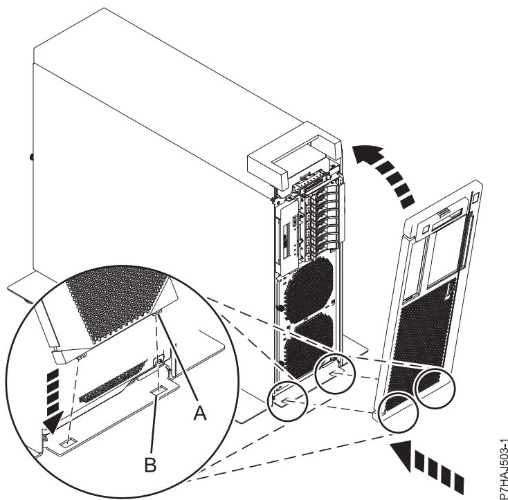
Abbildung 110. Vordere Abdeckung installieren
