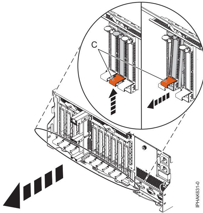
Abbildung 80. PCI-Adapterkassette ausbauen
