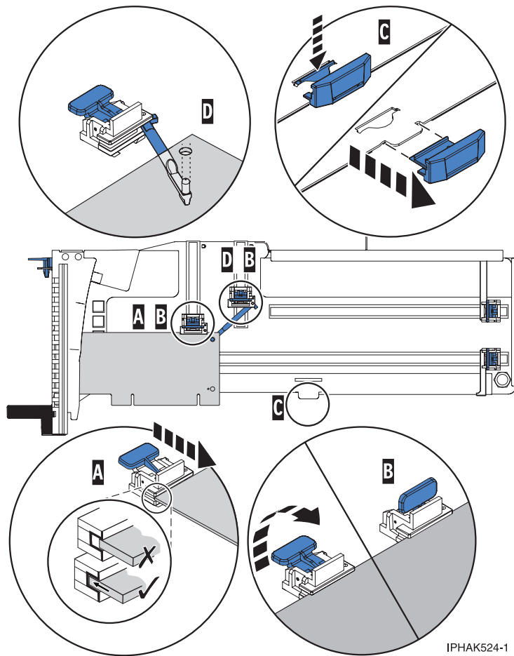
Abbildung 90. Kleiner Adapter in PCI-Adapterkassette, Halterungen und Verankerung an korrekter Position
