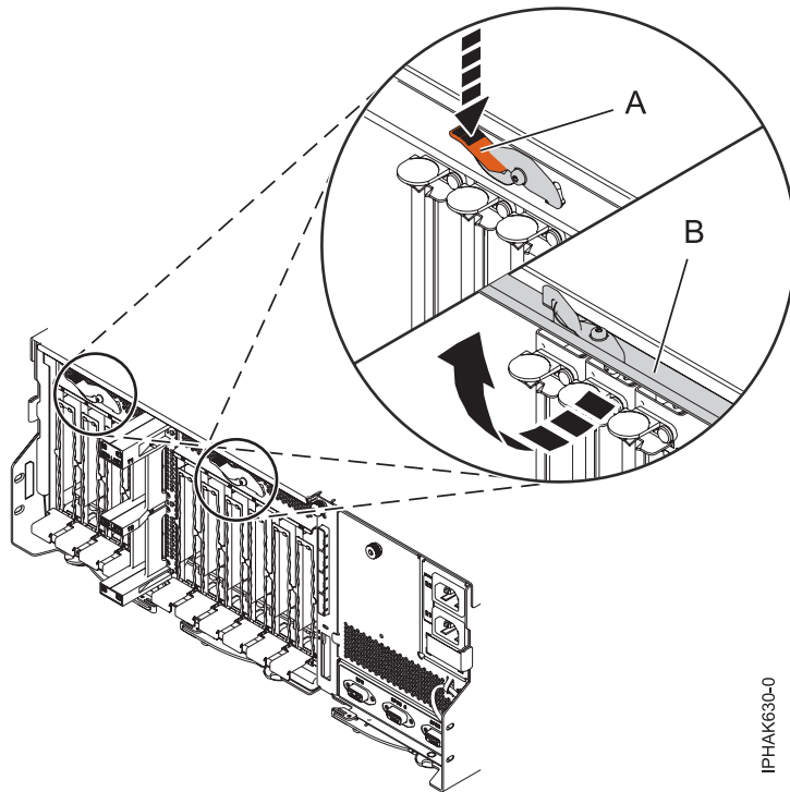
Abbildung 79. Klappe öffnen
