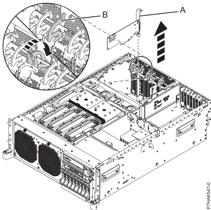
Abbildung 7. Ausbau eines PCI-Adapters aus einem Einschubsystem
