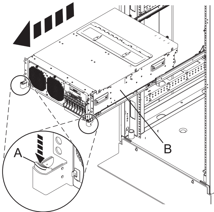
Abbildung 119. Systemeinheit in Serviceposition einrasten lassen
