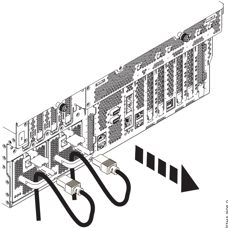
Abbildung 11. Netzkabel abziehen
