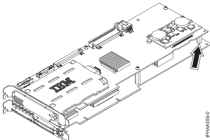
Abbildung 104. Abstandshalter ausbauen
