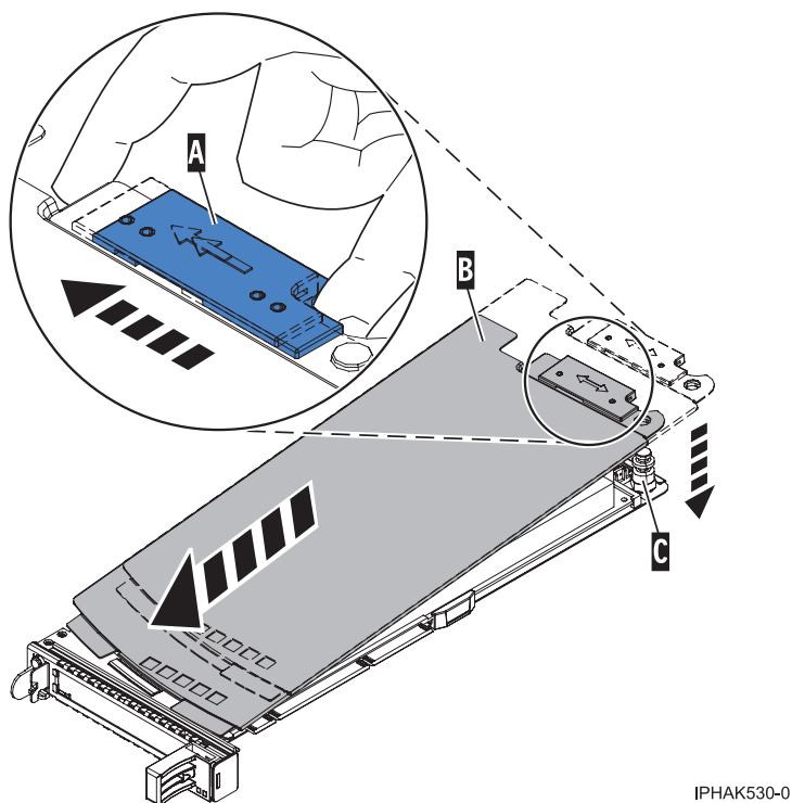
Abbildung 65. Abdeckung der PCI-Adapterkassette anbringen
