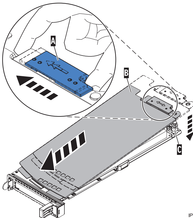
Abbildung 91. Abdeckung der PCI-Adapterkassette anbringen
