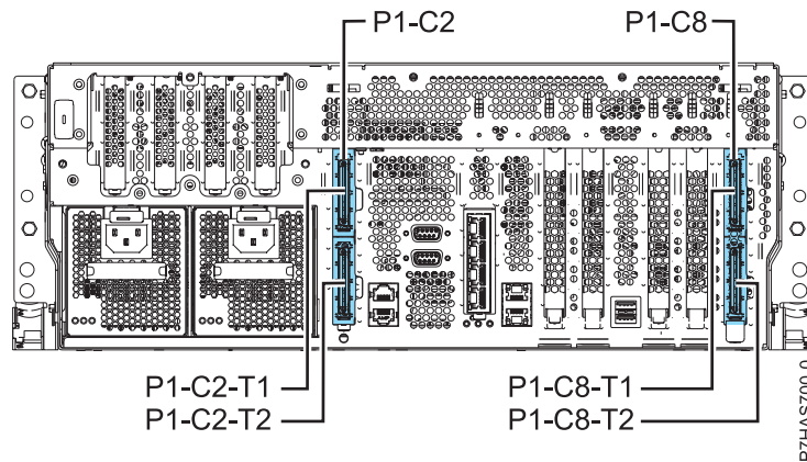
Abbildung 36. Steckplätze P1-C2 und P1-C8 - Rückansicht
