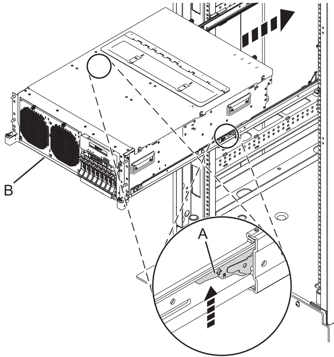
Abbildung 120. Systemeinheit in Betriebsposition bringen
