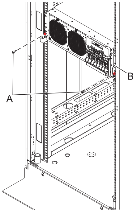
Abbildung 118. Systemeinheit in Serviceposition bringen
