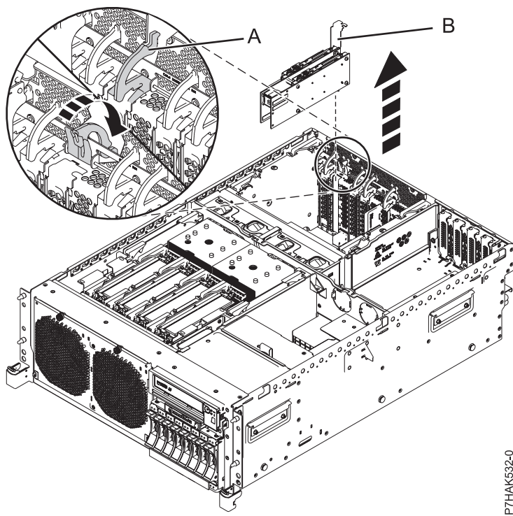
Abbildung 22. Ausbau eines PCIe-RAID- und SSD-SAS-Adapters aus einem Einschubsystem
