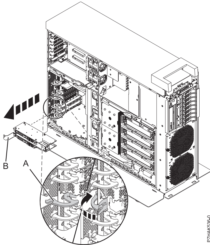
Abbildung 23. Ausbau eines PCIe-RAID- und SSD-SAS-Adapters aus einem Standalone-System
