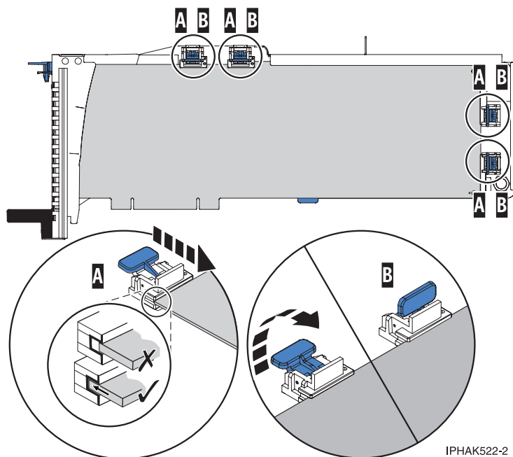
Abbildung 58. Großer Adapter in PCI-Adapterkassette, Halterungen und Stabilisator an korrekter Position
