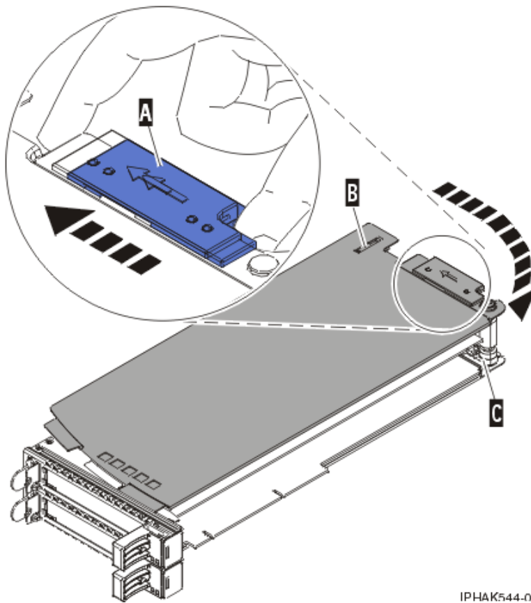
Abbildung 96. Abdeckung der PCI-Adapterkassette ausbauen
