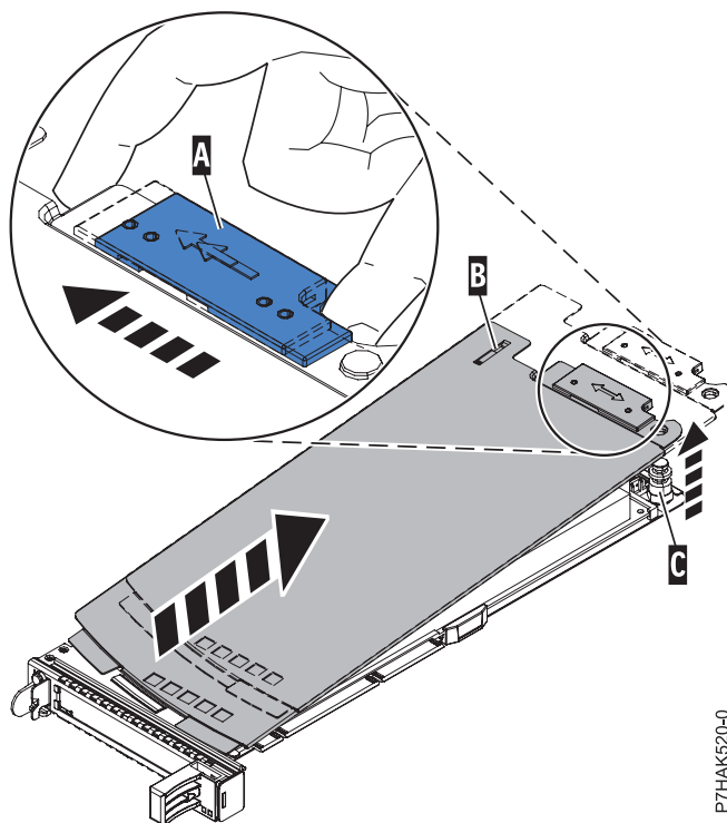
Abbildung 81. Abdeckung der PCI-Adapterkassette ausbauen
