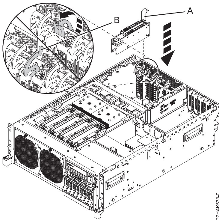
Abbildung 17. PCIe-RAID- und SSD-SAS-Adapter in einem Einschubsystem installieren
