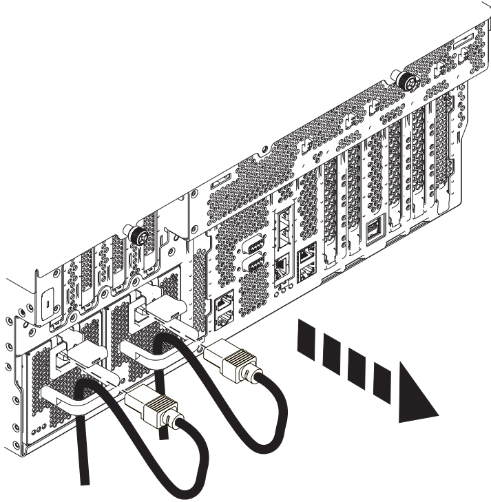
Abbildung 122. Netzkabel abziehen - Einschubsystem
