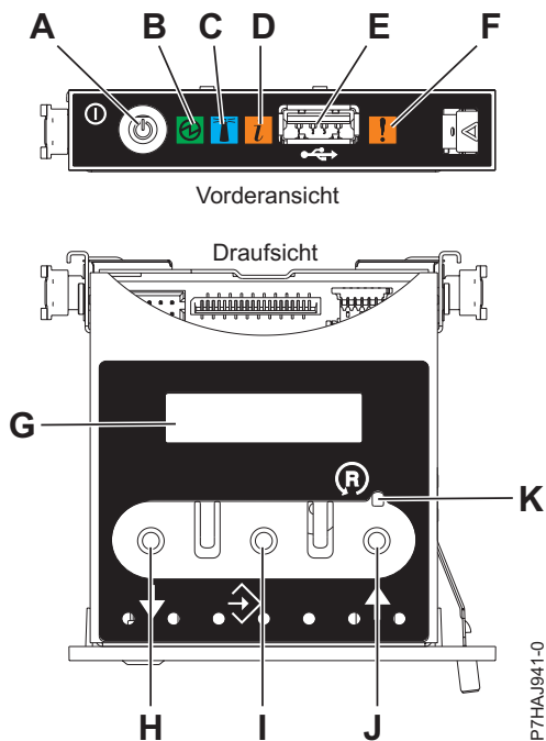
Abbildung 5. Steuerkonsole
