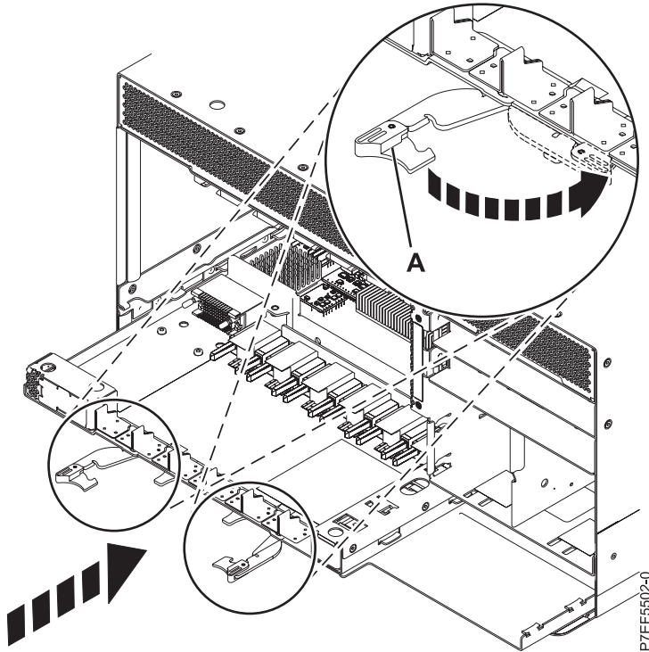
Abbildung 3. E/A-Rückwandplatine installieren
