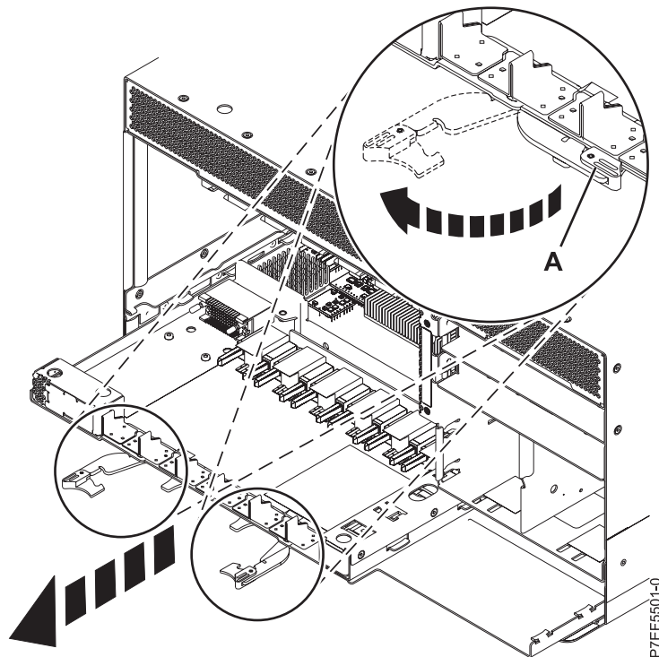
Abbildung 2. E/A-Rückwandplatine ausbauen
