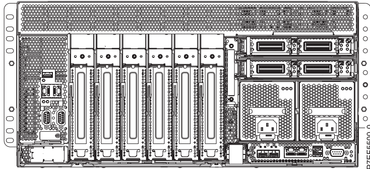
Abbildung 1. E/A-Rückwandplatine
