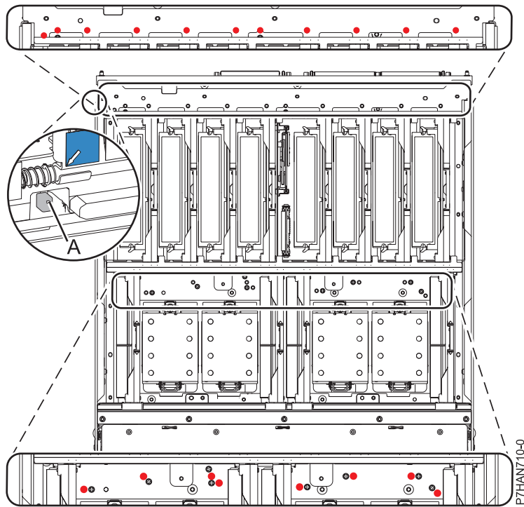
Abbildung 3. Schaltfläche auf der Platine
