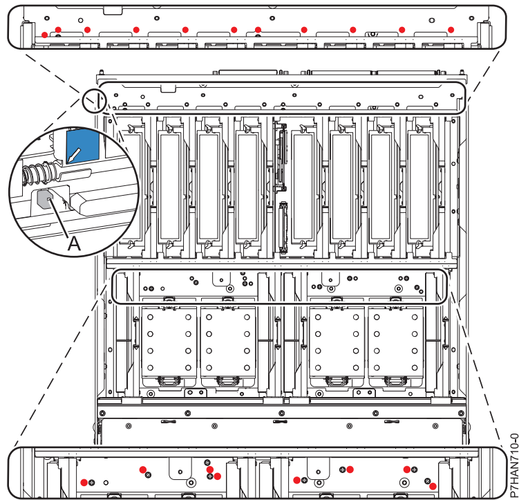
Abbildung 2. Schaltfläche auf der Platine
