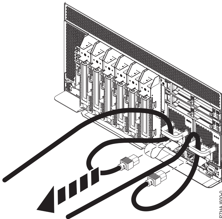
Abbildung 1. Netzkabel abziehen
