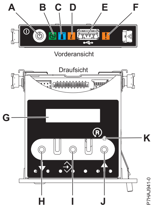
Abbildung 4. Steuerkonsole
