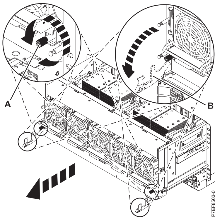
Abbildung 8. Seitliche Verriegelungen lösen
