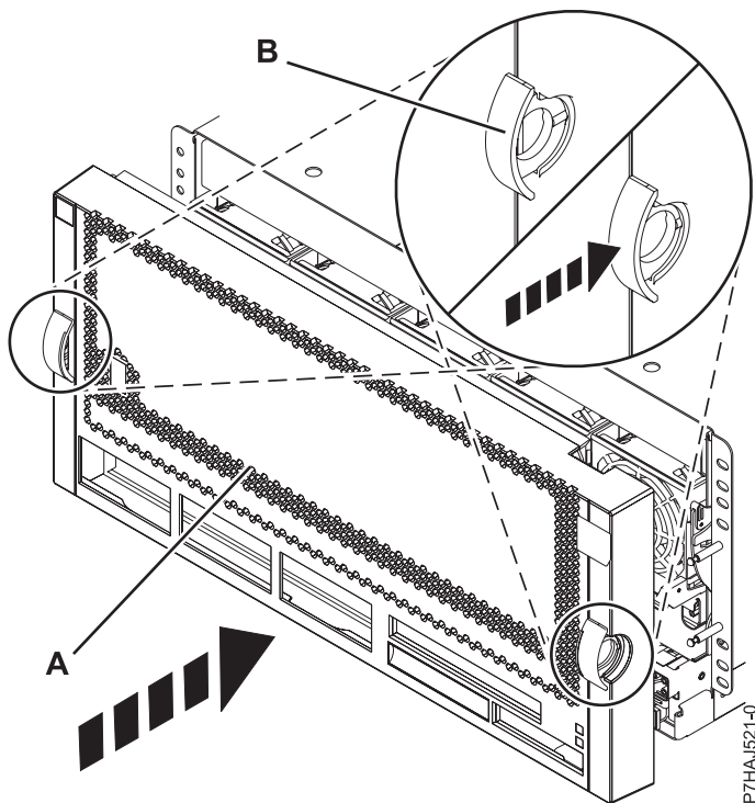
Abbildung 7. Vordere Abdeckung installieren
