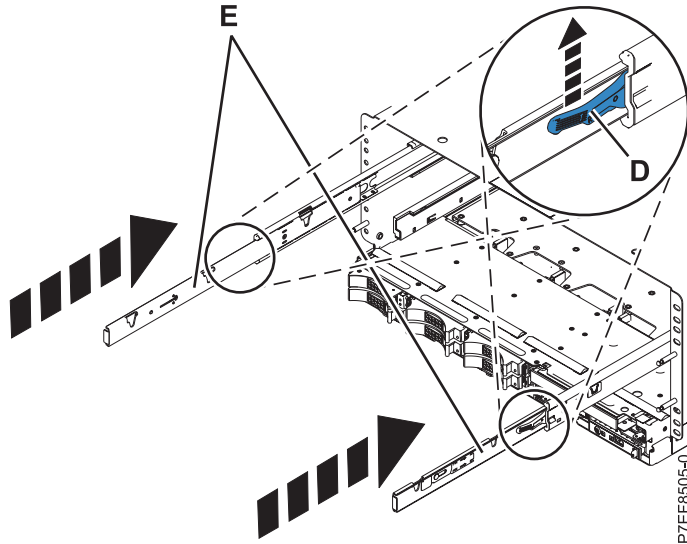
Abbildung 10. Schienensicherheitsverriegelungen entriegeln
