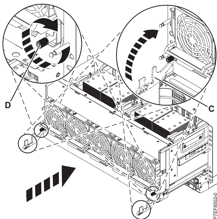
Abbildung 11. Entriegelungshebel an der Systemeinheit verriegeln
