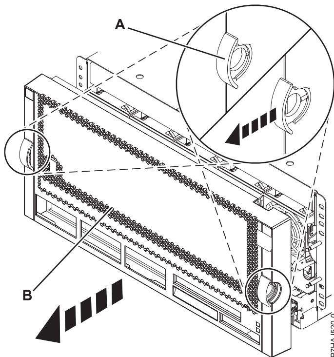
Abbildung 6. Vordere Abdeckung ausbauen
