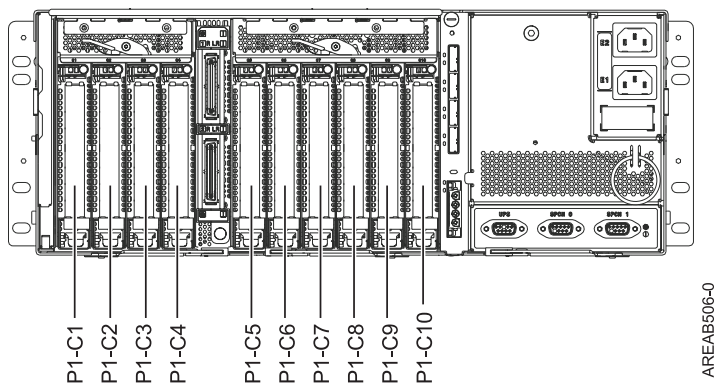
Abbildung 4. Rückansicht. In dieser Abbildung ist die Rückansicht der Erweiterungseinheit dargestellt.
