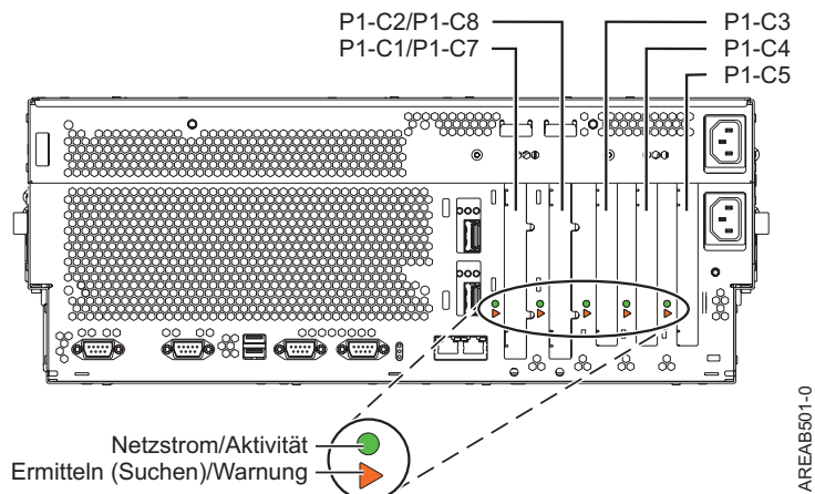
Abbildung 1. Rückansicht des Systems mit Positionscodes. Tabelle 4 zeigt die Rückansicht des Systems mit den Positionscodes der Steckplätze für die PCI- und GX-Adapter.
