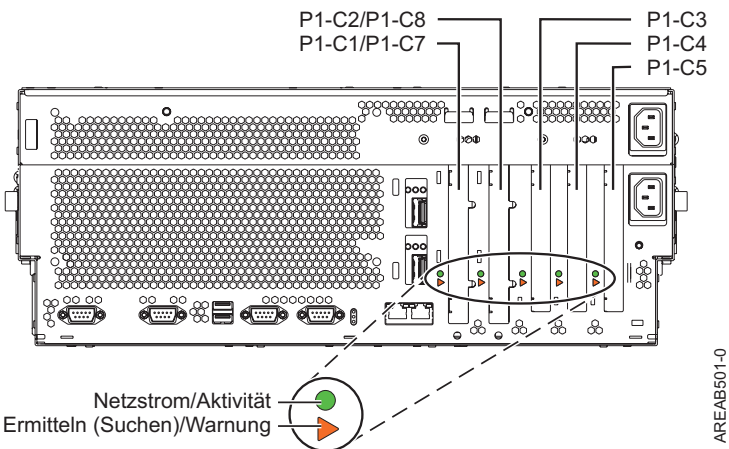
Abbildung 2. Rückansicht des Gehäuses mit Positionscodes. Tabelle 11 zeigt die Rückansicht der Systemeinheit mit den Positionscodes für die PCI- und GX+-Steckplätze.
