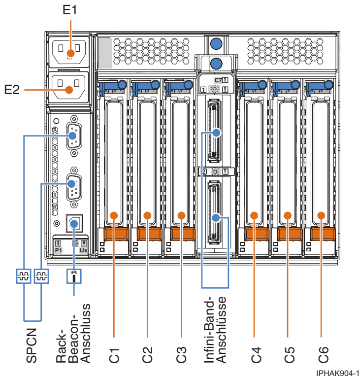
Abbildung 3. Rückansicht
