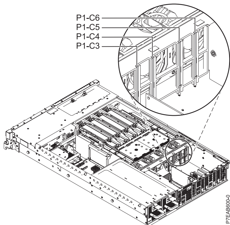
Abbildung 1. Rückansicht von 8231-E2B mit den Positionscodes für die PCI-Steckplätze
