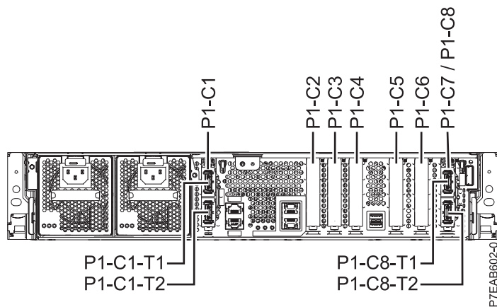
Abbildung 3. Rückansicht des Systems mit Positionscodes
