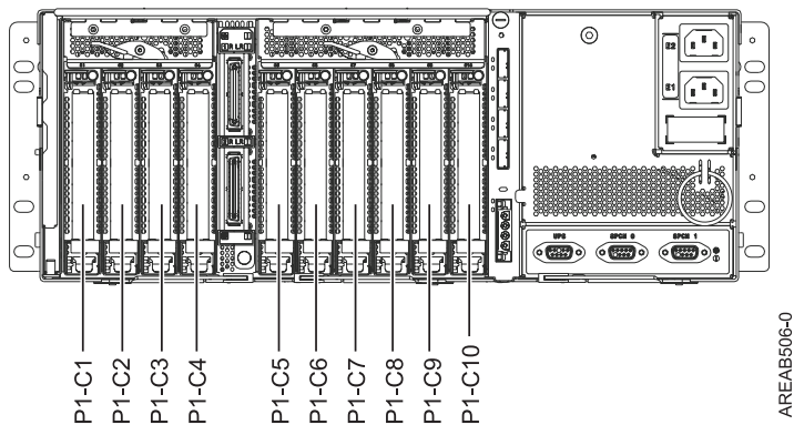
Abbildung 4. Rückansicht. In dieser Abbildung ist die Rückansicht der Erweiterungseinheit dargestellt.
