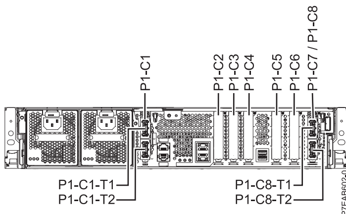
Abbildung 2. Rückansicht des Systems mit Positionscodes
