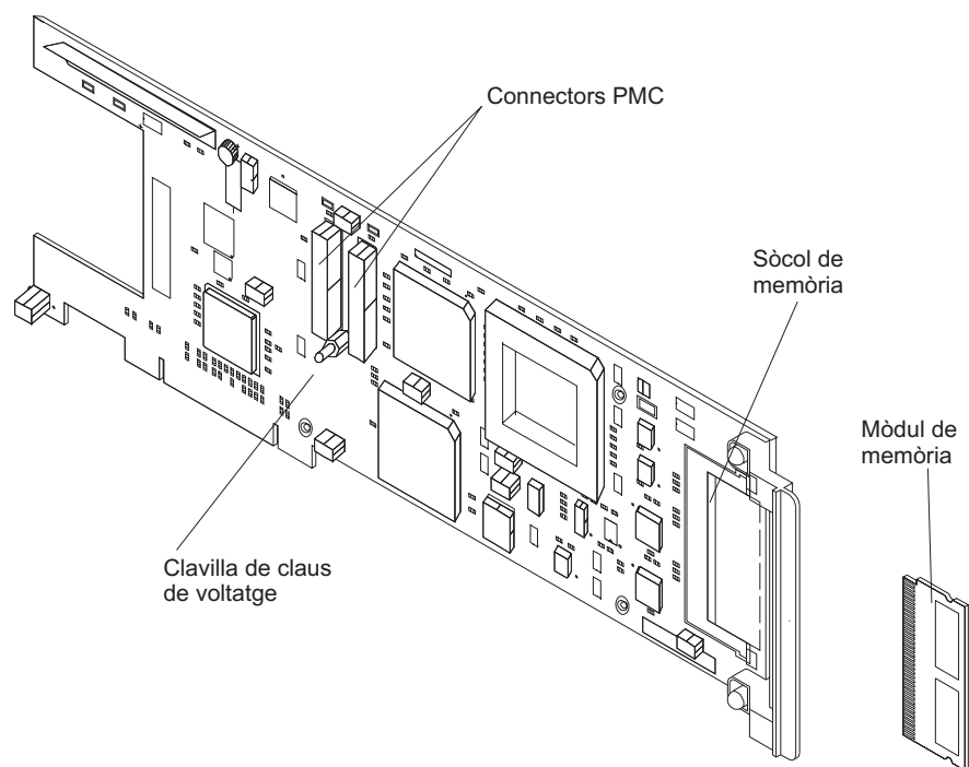
Figura 60. Adaptador PCI base ARTIC960HX d'IBM
