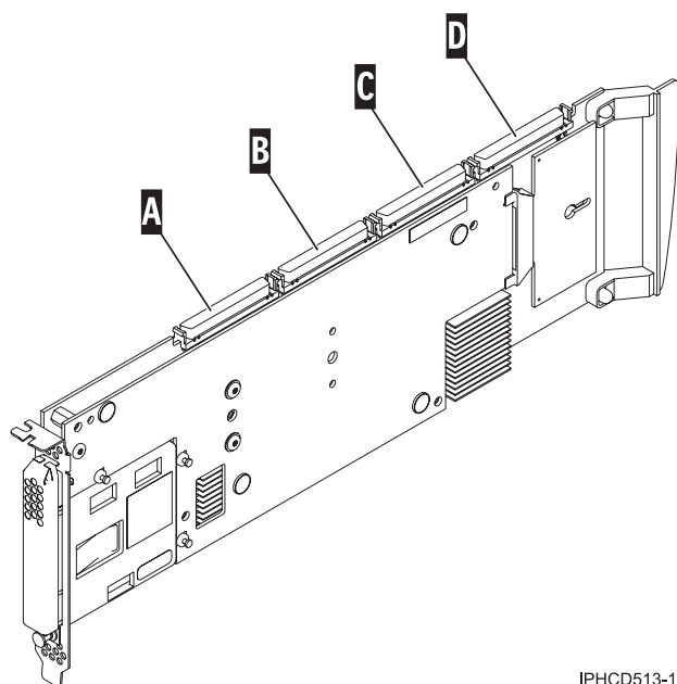
Figura 55. Connectors SCSI de l'adaptador
