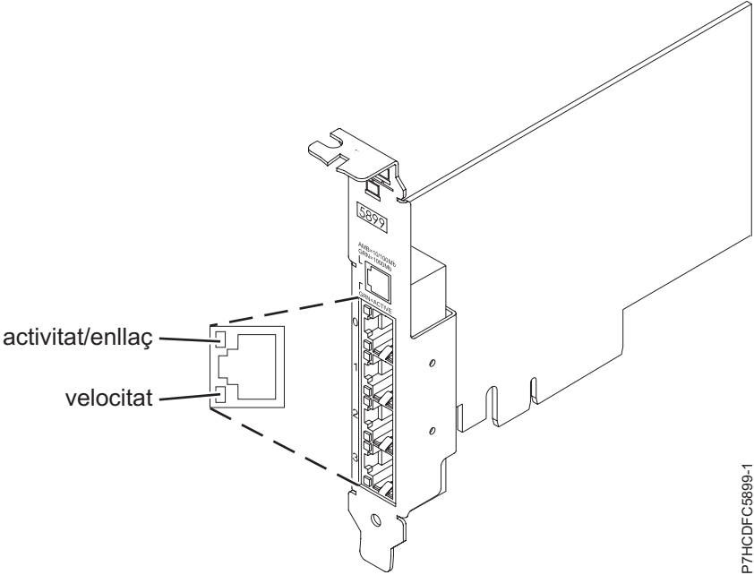
Figura 35. Adaptador
