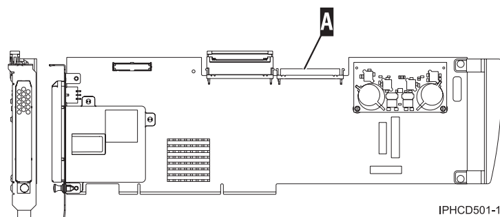
Figura 52. IOA de memòria cau d'escriptura auxiliar
