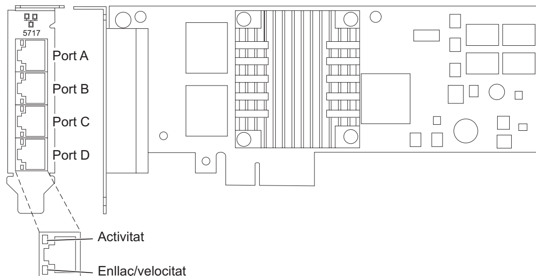
Figura 27. Adaptador 10/100/1000 Base-TX PCIe de 4 ports
