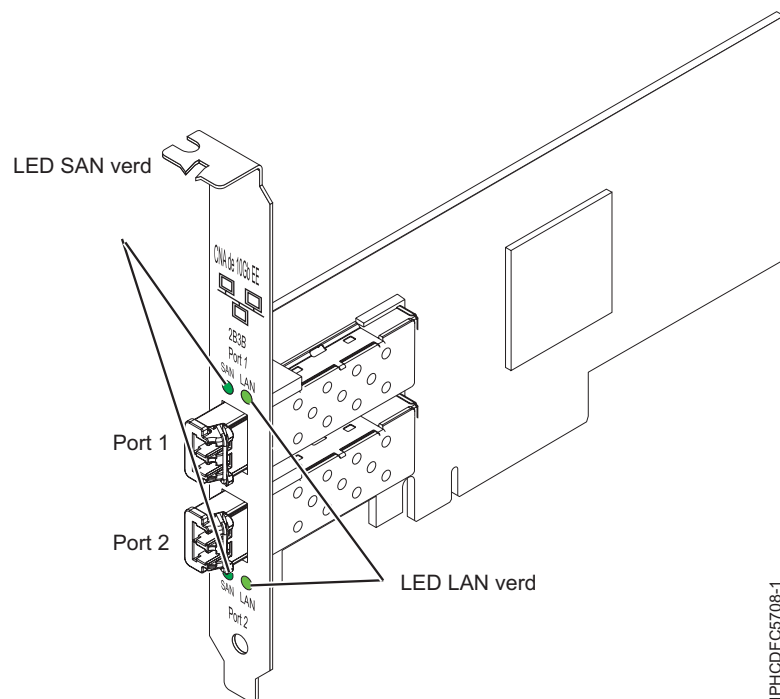
Figura 22. Adaptador FCoE PCIe de 10 Gb de dos ports
