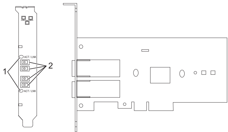
Figura 32. Adaptador Gigabit Ethernet-SX PCI Express de dos ports
