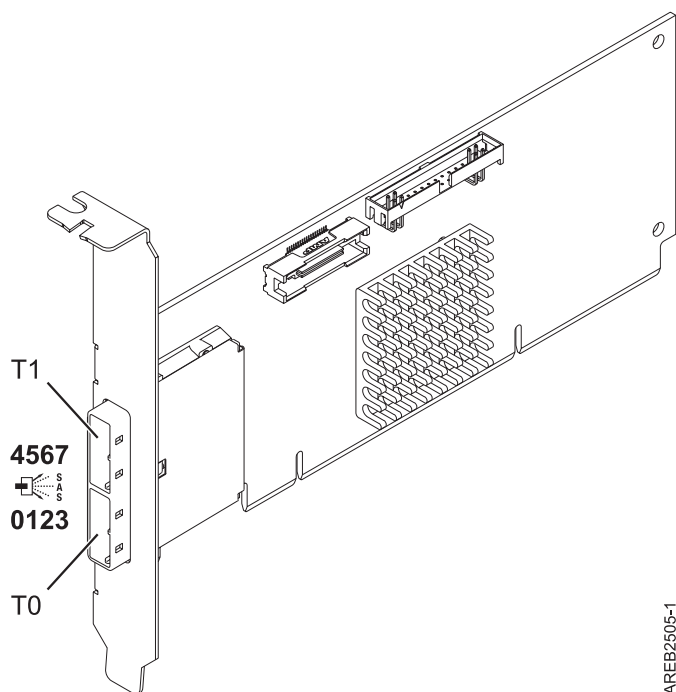
Figura 42. Adaptador PCI-X SAS DDR Dual extern de 4 ports
