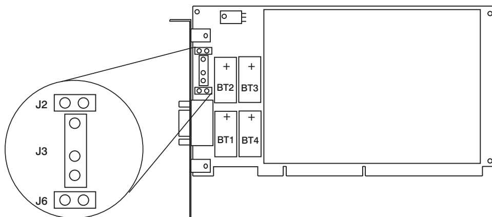
Figura 40. Substitució de les bateries de coprocessador
