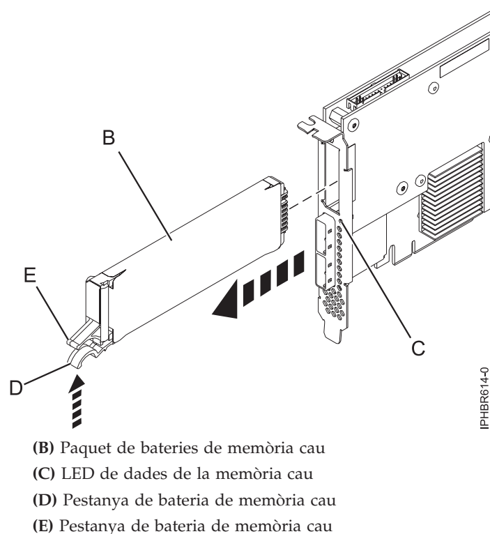
Figura 66. Substitució de la bateria de memòria cau 574E
