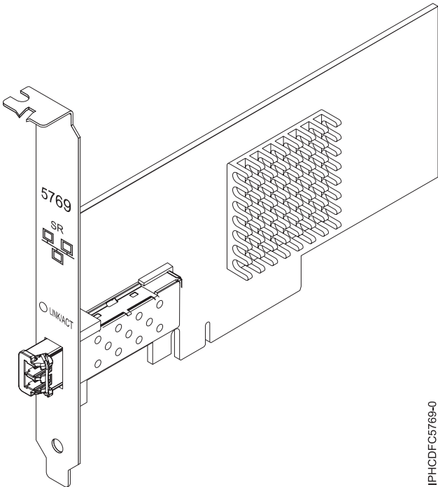
Figura 33. adaptador PCIe Ethernet-SR de 10 Gigabits
