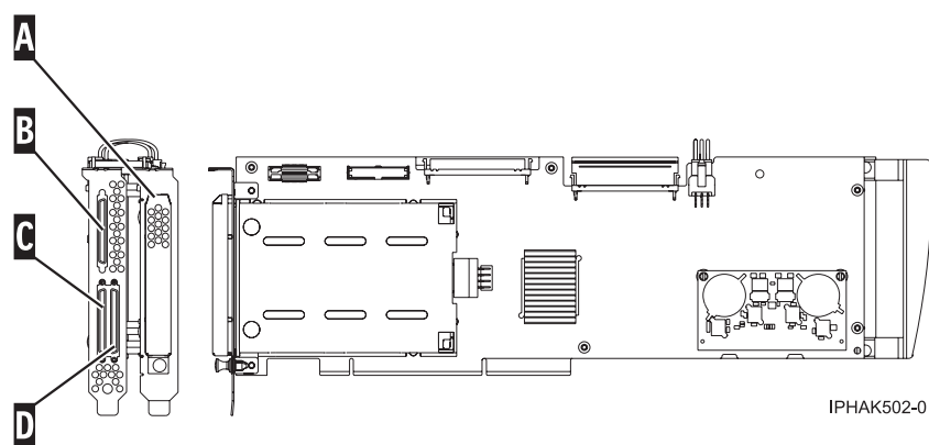
Figura 56. Adaptador
