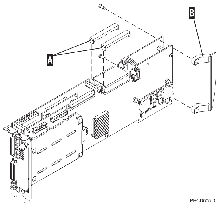
Figura 57. Preparació de l'adaptador per col·locar-lo en un casset
