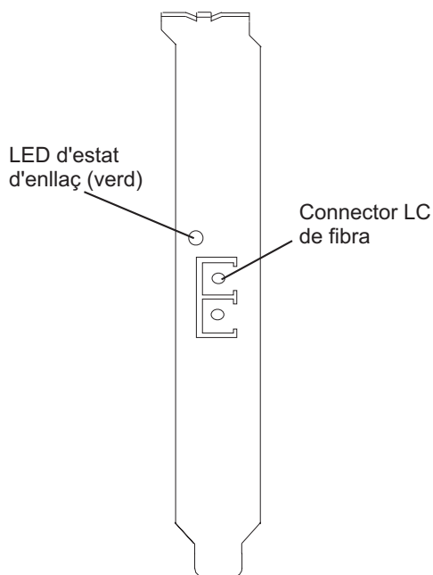
Figura 25. LED de l'adaptador PCI-X 1 Gigabit-SX iSCSI TOE
