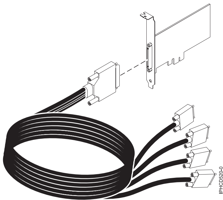
Figura 7. Cable
