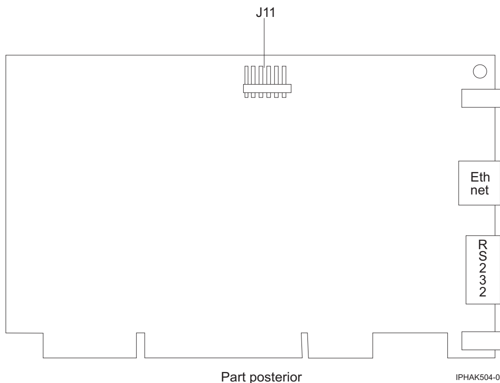
Figura 39. Part posterior de l'adaptador
