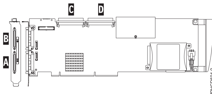
Figura 53. Adaptador PCI-X DDR de canal dual Ultra320 SCSI RAID
