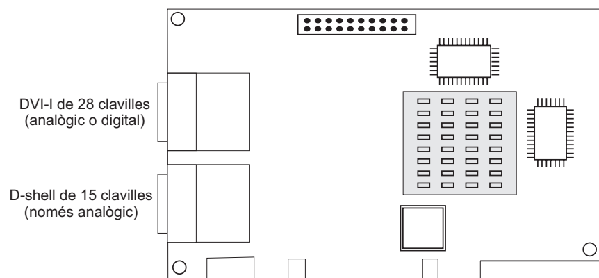
Figura 13. Dispositiu 2849
