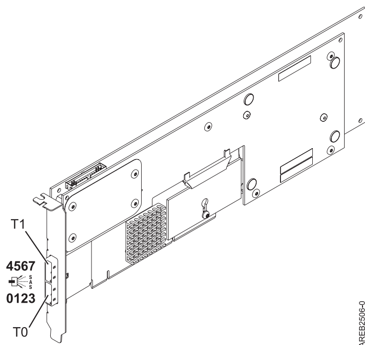
Figura 44. adaptador PCI-X DDR port x4 dual SAS RAID
