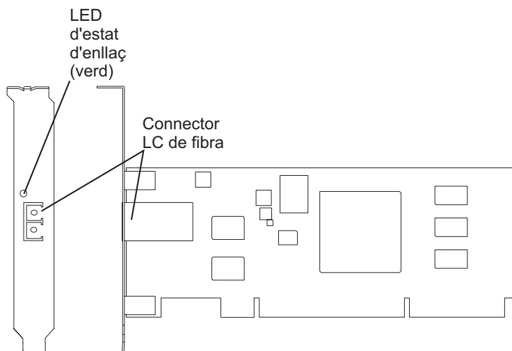
Figura 23. Adaptador PCI-X 1 Gigabit-SX iSCSI TOE
