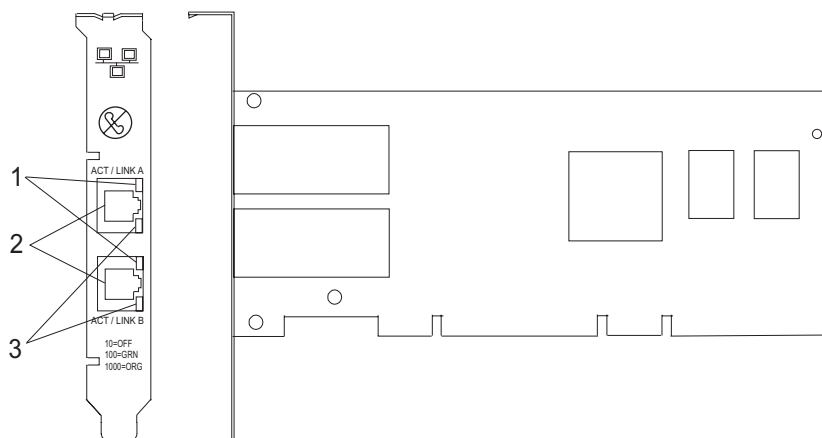
Figura 20. Adaptador 10/100/1000 Base-TX Ethernet PCI-X de 2 ports
