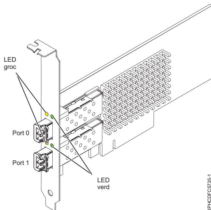
Figura 8. Adaptador 5735
