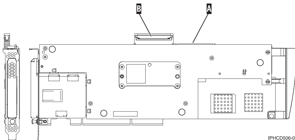
Figura 93. 5708, IOA de memòria cau d'escriptura auxiliar
