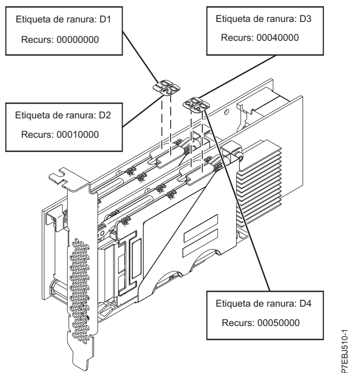
Figura 82. Adaptador SAS RAID PCIe Dual - x4 de 3 Gb
