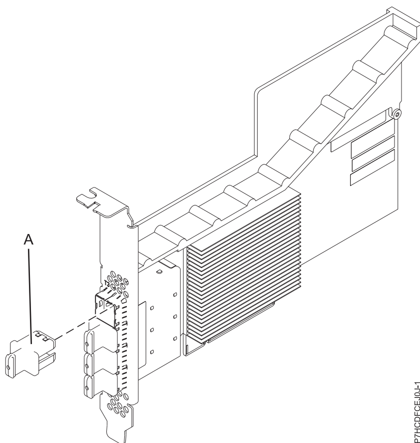
Figura 28. Adaptador port SAS PCIe3 4 x8
