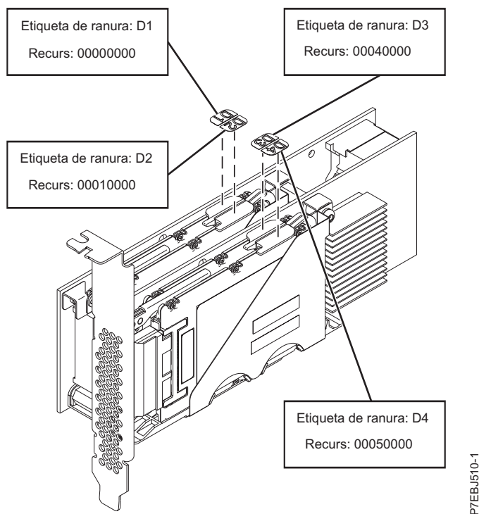
Figura 81. Adaptador SAS RAID PCIe Dual - x4 de 3 Gb
