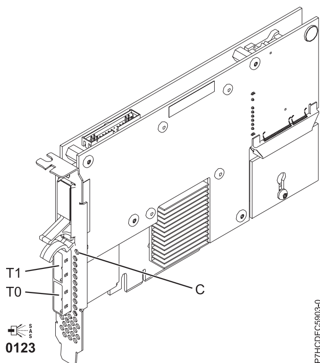
Figura 87. Adaptador SAS RAID PCIe Dual - x4 de 3 Gb
