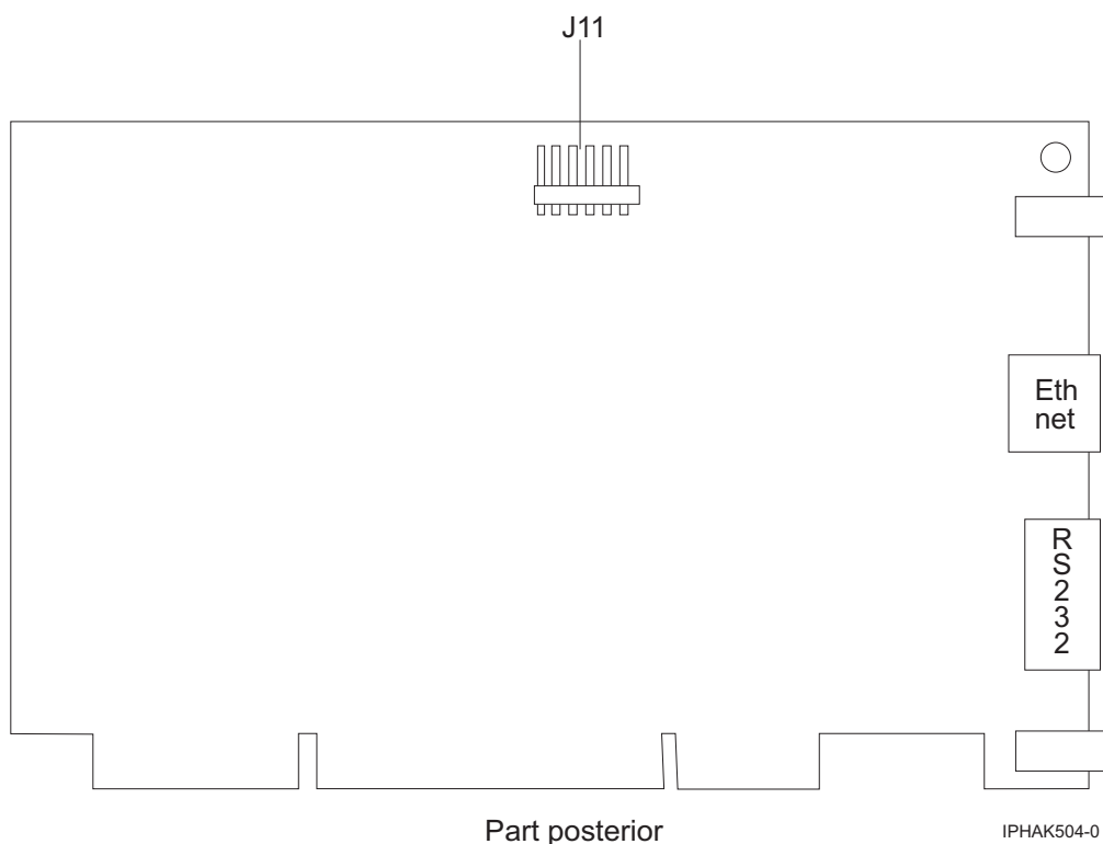
Figura 79. Part posterior de l'adaptador
