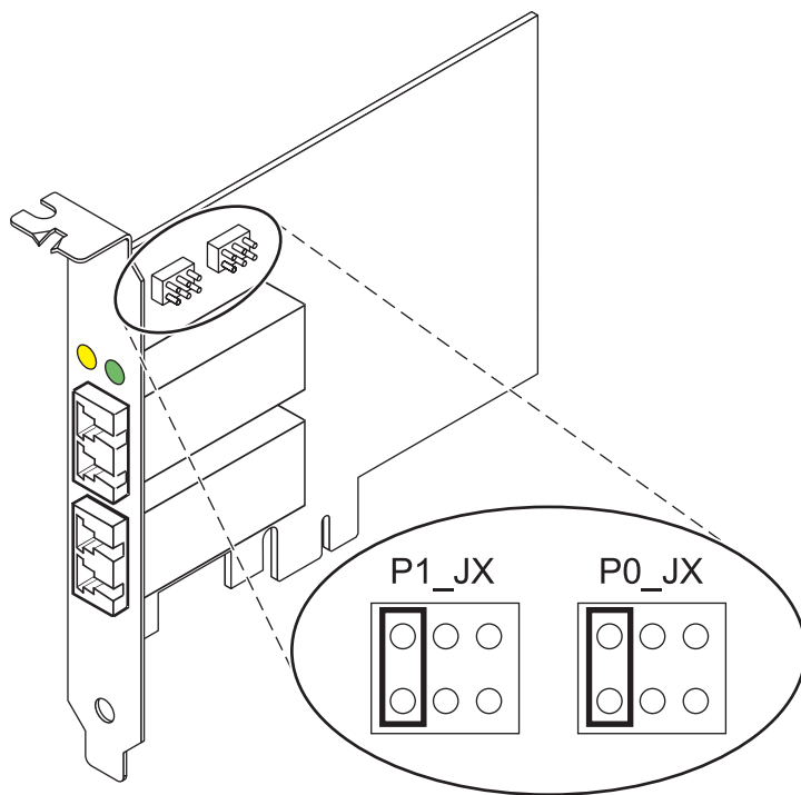
Figura 18. Pont d'ID de dispositiu
