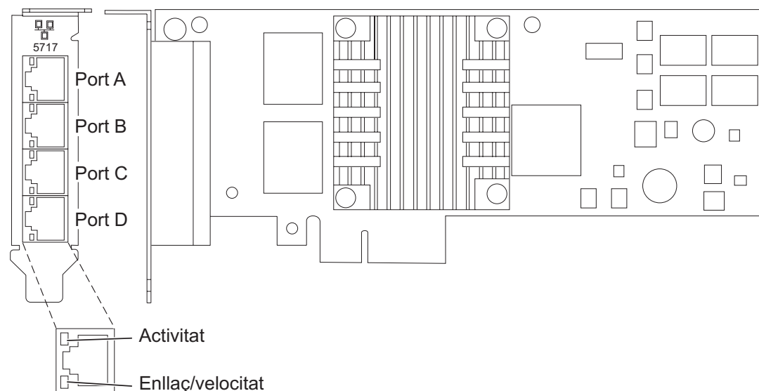
Figura 51. Adaptador 10/100/1000 Base-TX PCIe de 4 ports
