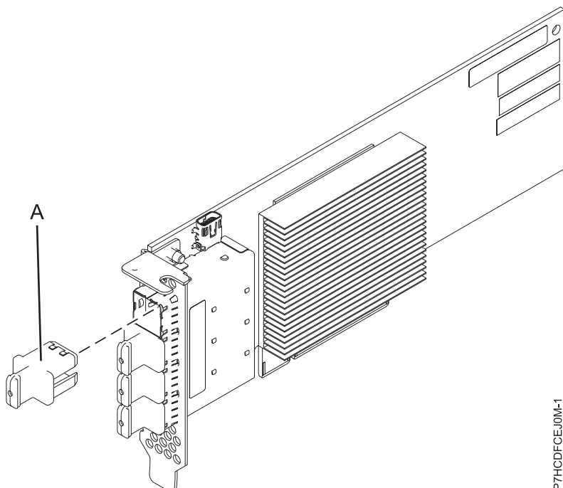
Figura 27. Adaptador PCIe3 RAID SAS de quatre ports 6Gb LP
