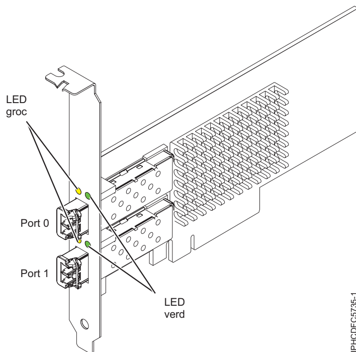
Figura 14. Adaptador 5735
