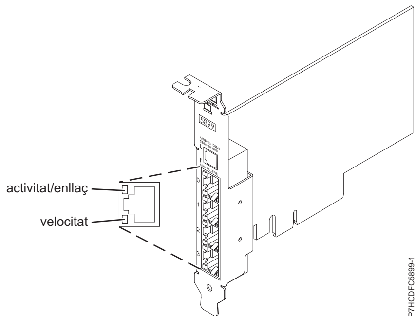
Figura 62. Adaptador
