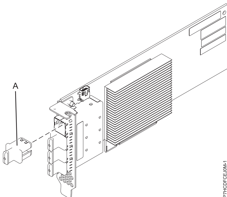
Figura 29. Adaptador de ports PCIe3 LP 4 x8 SAS
