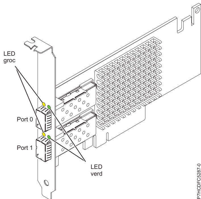
Figura 40. Adaptador SR PCIe2 LP de 2 ports i 10GbE
