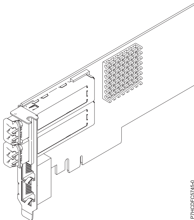
Figura 36. Adaptador UTP PCIe2 LP 2x10GbE SFP+ Copper 2x1GbE
