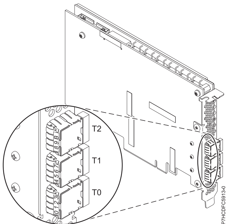
Figura 91. Adaptador 5913
