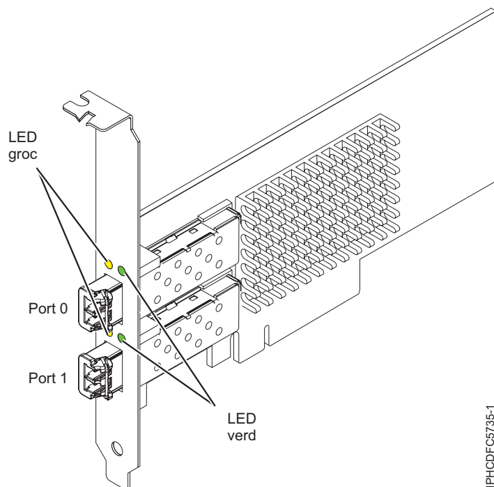
Figura 10. Adaptador 5273
