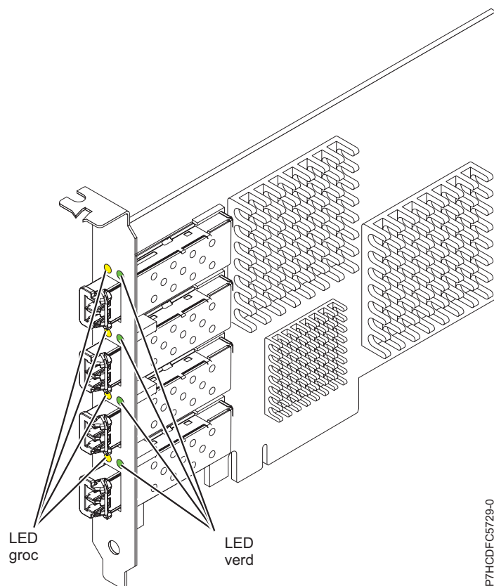
Figura 13. Adaptador FC 5729
