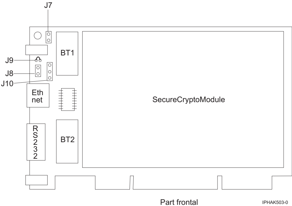
Figura 78. Part frontal de l'adaptador
