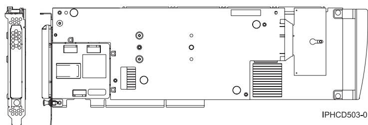
Figura 97. Vista lateral i posterior de l'adaptador
