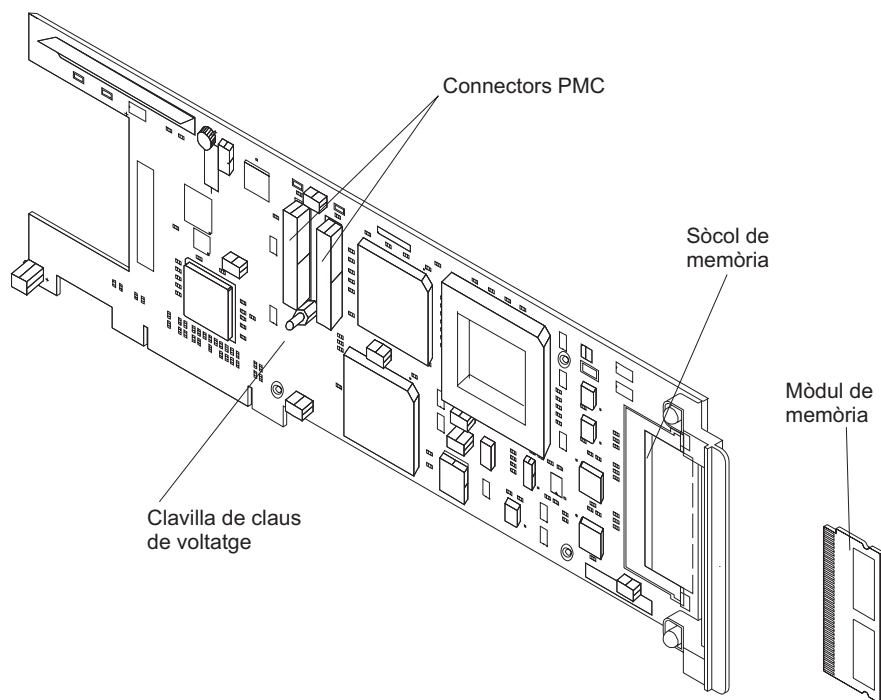
Figura 103. Adaptador PCI base ARTIC960HX d'IBM
