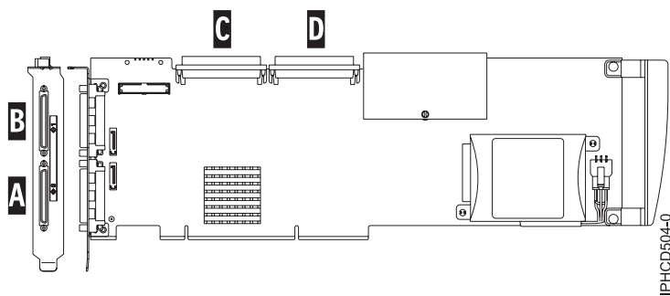
Figura 96. Adaptador PCI-X DDR de canal dual Ultra320 SCSI RAID
