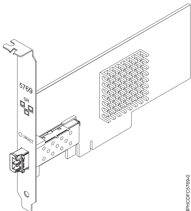
Figura 60. adaptador PCIe Ethernet-SR de 10 Gigabits
