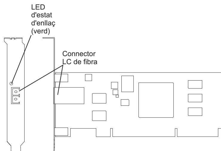
Figura 47. Adaptador PCI-X 1 Gigabit-SX iSCSI TOE
