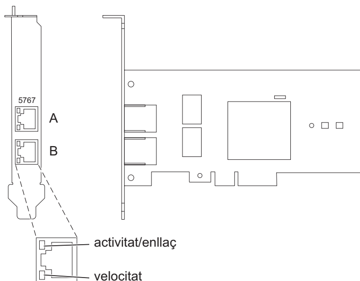
Figura 63. adaptador TX PCIe de dos ports i 1 GbE
