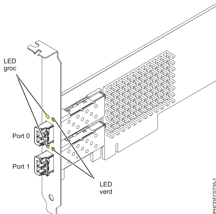
Figura 20. Adaptador EN0B
