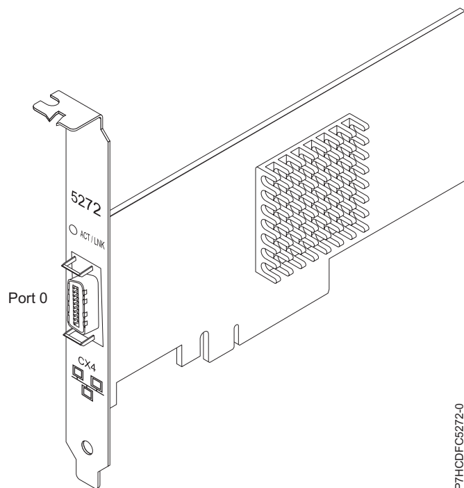
Figura 33. adaptador d'un port PCIe LP 10GbE CX4
