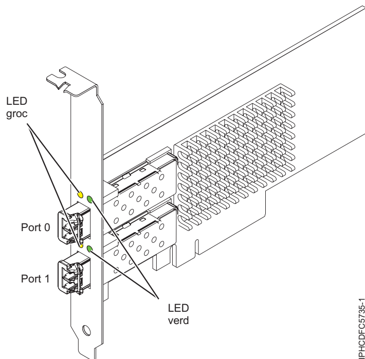
Figura 19. Adaptador EN0A
