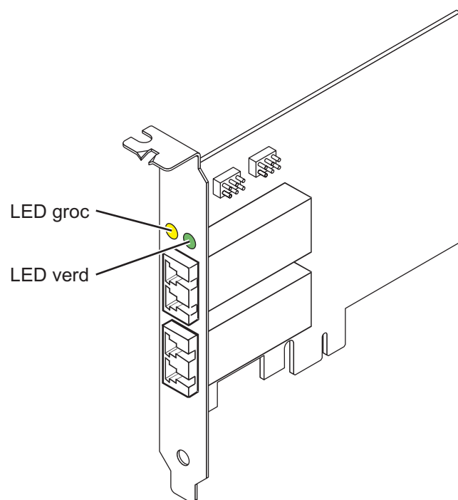
Figura 11. Adaptador 5276
