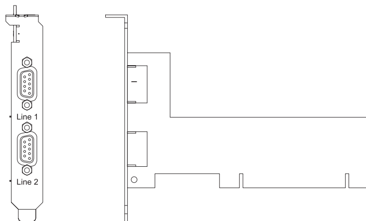
Figura 7. Adaptador PCI de 2 ports EIA-232 asíncron
