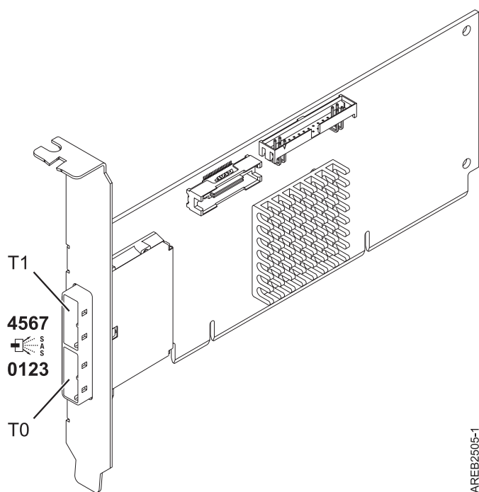
Figura 90. Adaptador PCI-X SAS DDR Dual extern de 4 ports
