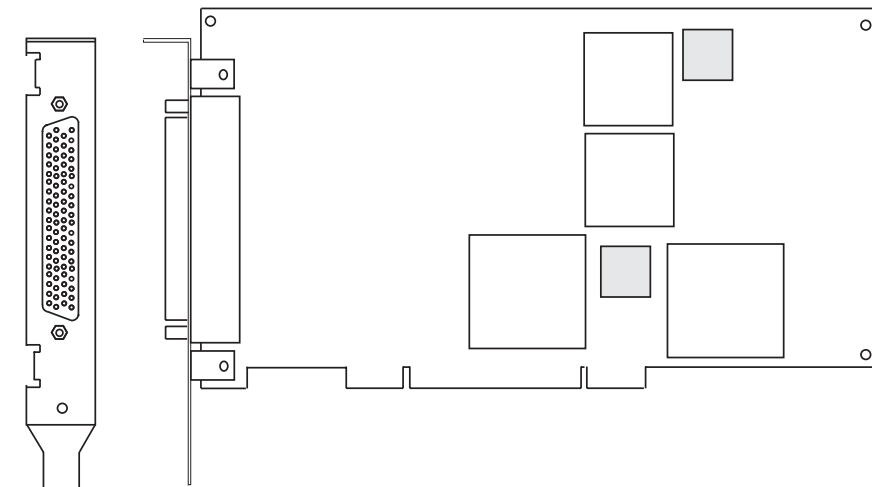
Figura 2. Dispositiu 2943
