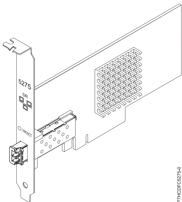
Figura 35. adaptador d'un port PCIe LP 10GbE
