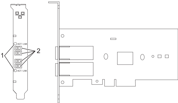
Figura 59. Adaptador Gigabit Ethernet-SX PCI Express de dos ports
