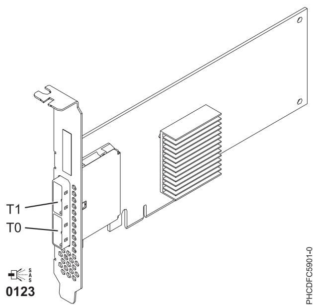
Figura 83. Adaptador SAS PCIe Dual - x4
