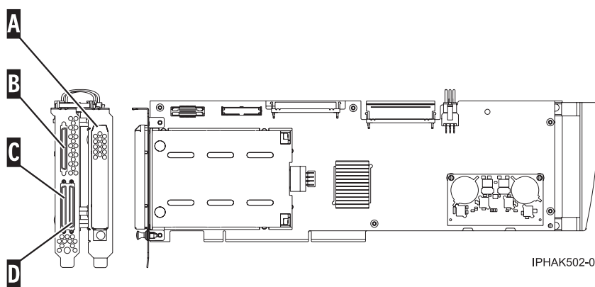
Figura 101. Adaptador 5782
