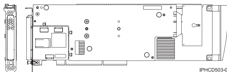
Figura 94. Vista lateral i posterior de l'adaptador
