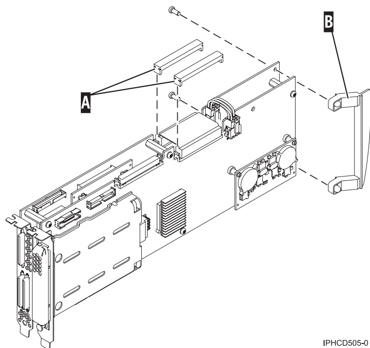
Figura 100. Preparació de l'adaptador per col·locar-lo en un casset
