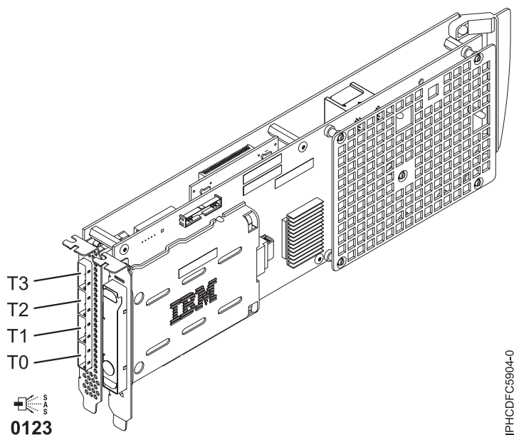
Figura 88. Adaptador RAID SAS PCI-X DDR d'1,5 GB de memòria cau
