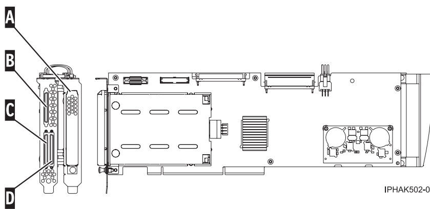
Figura 99. Adaptador
