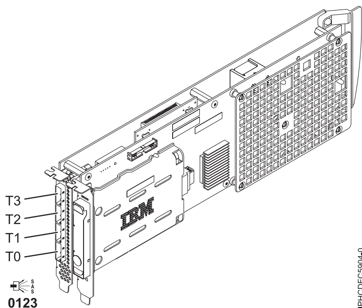
Figura 89. Adaptador RAID SAS PCI-X d'1.5 GB de memòria cau
