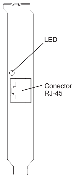
Figura 50. LED de l'adaptador PCI-X 1 Gigabit-TX iSCSI TOE
