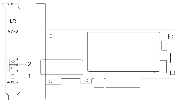
Figura 61. Adaptador PCI Express Ethernet-LR de 10 Gigabits
