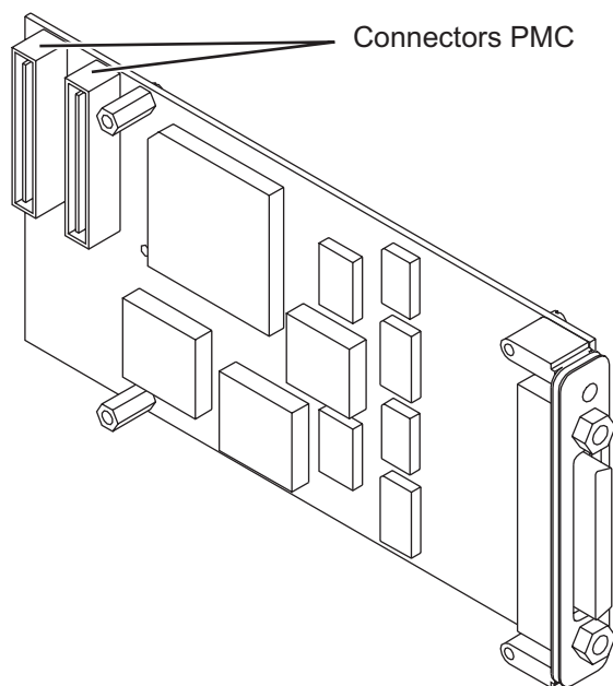
Figura 104. PMC de 4 ports seleccionables
