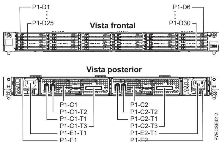
Figura 105. Codis d'ubicació del model adaptador SAS RAID integrat PCIe2 de 3,1 GB de memòria cau
