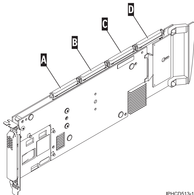
Figura 98. Connectors SCSI de l'adaptador
