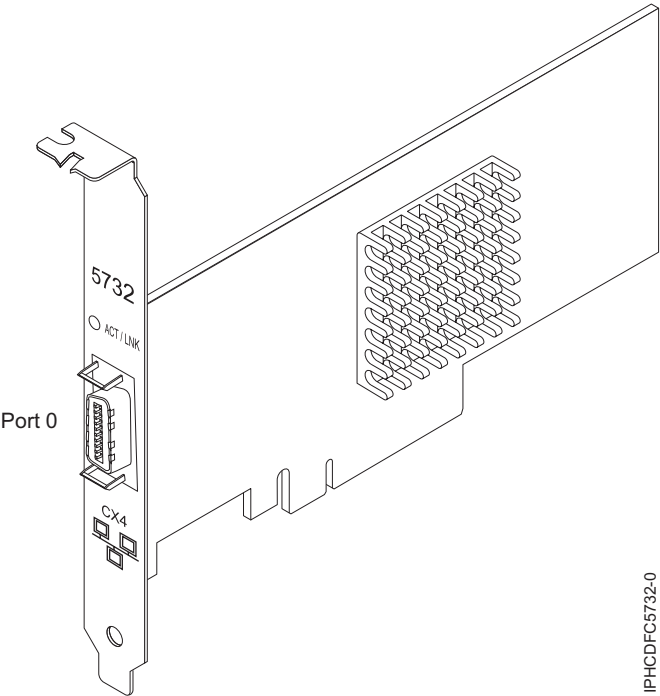
Figura 52. Adaptador Ethernet-CX4 PCI Express (PCIe) de 10 gigabits
