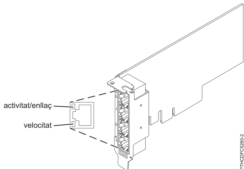
Figura 30. Adaptador
