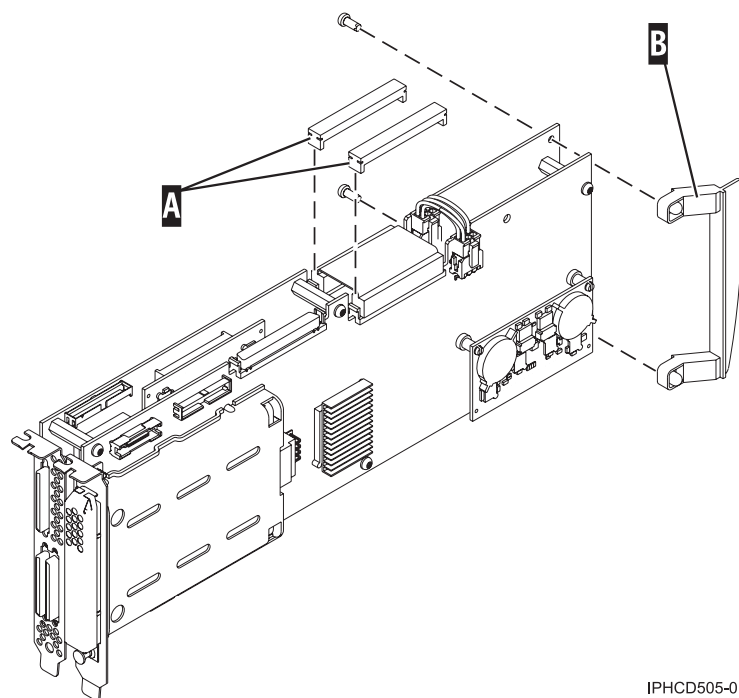
Figura 102. Preparació de l'adaptador per col·locar-lo en un casset
