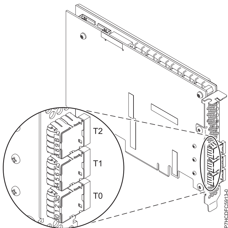
Figura 7. Adaptador 5913
