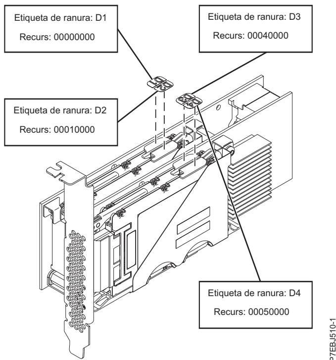
Figura 4. Adaptador SAS RAID PCIe Dual - x4 de 3 Gb
