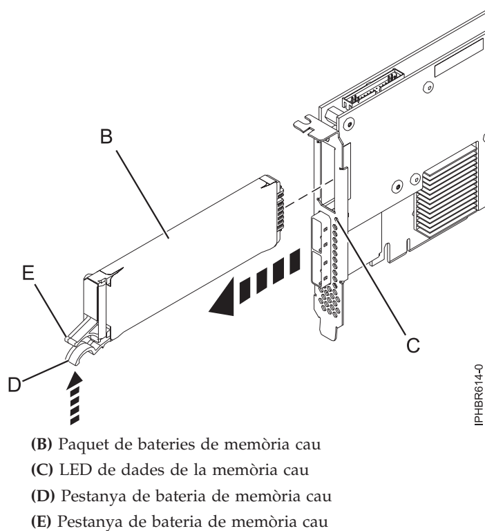
Figura 59. Substitució de la bateria de memòria cau 574E
