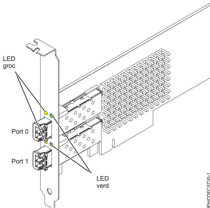
Figura 9. Adaptador 5273
