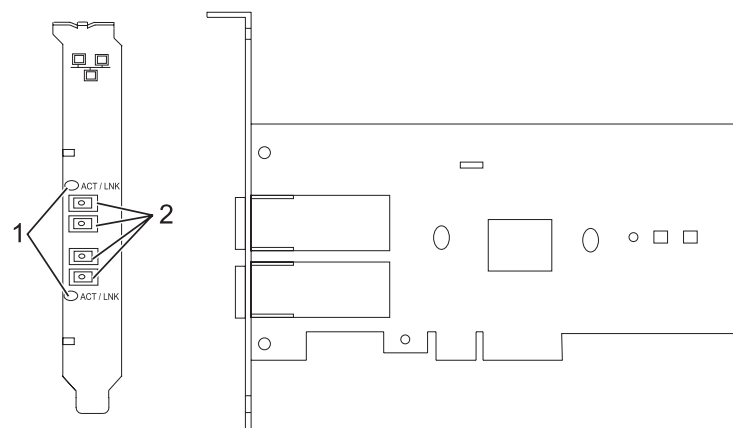
Figura 38. Adaptador Gigabit Ethernet-SX PCI Express de dos ports
