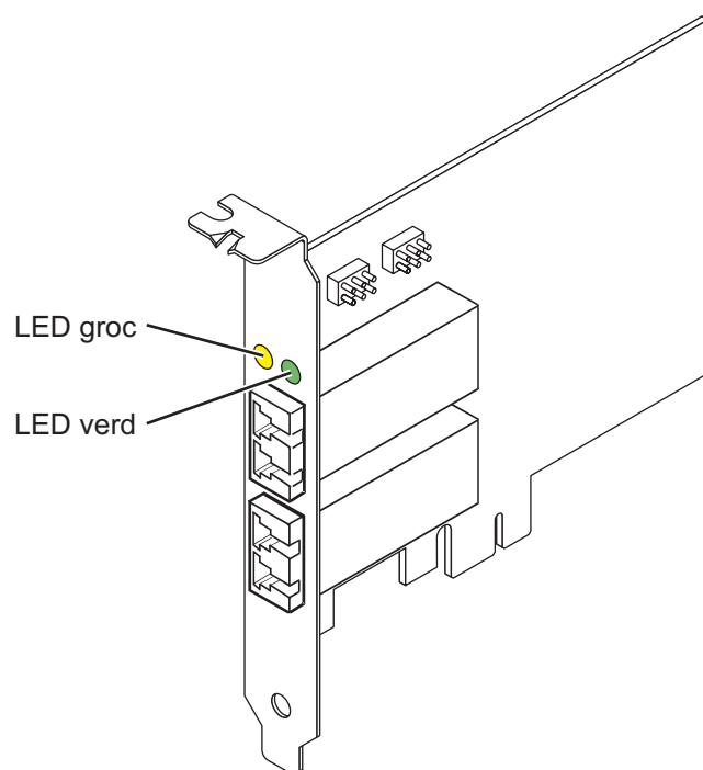
Figura 13. Adaptador EL09
