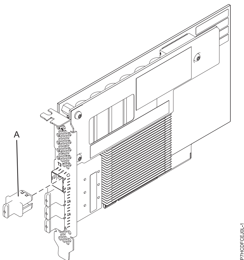
Figura 20. Adaptador SAS RAID PCIe3 amb 12 GB memòria cau i 6 Gb
