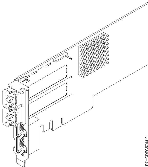
Figura 30. adaptador UTP PCIe2 LP 2x10GbE SR 2x1GbE
