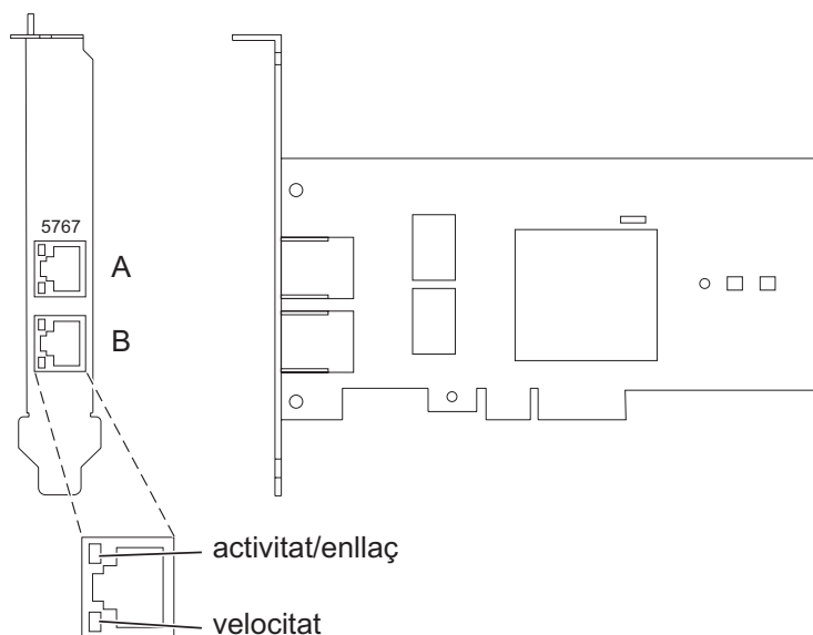
Figura 44. Adaptador TX PCIe LP de dos ports i 1 GbE
