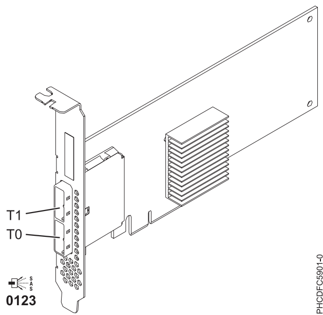
Figura 8. Adaptador SAS x4 - PCIe LP dual
