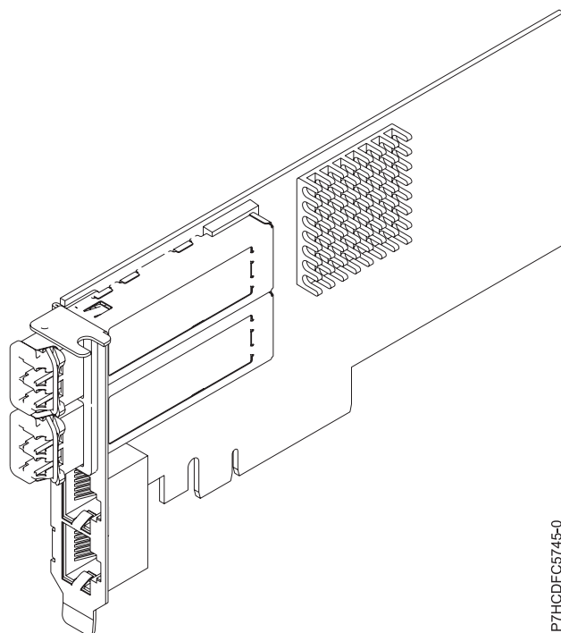
Figura 28. Adaptador UTP PCIe2 LP 2x10GbE SFP+ Copper 2x1GbE
