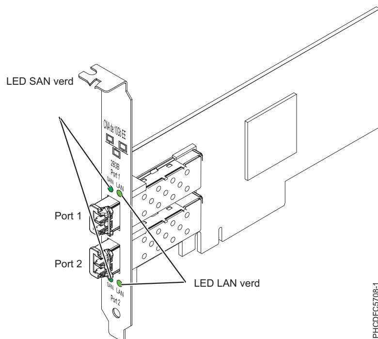
Figura 23. Adaptador de dos ports FCoE PCIe de 10 Gb
