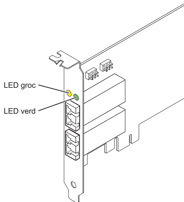
Figura 11. Adaptador 5774
