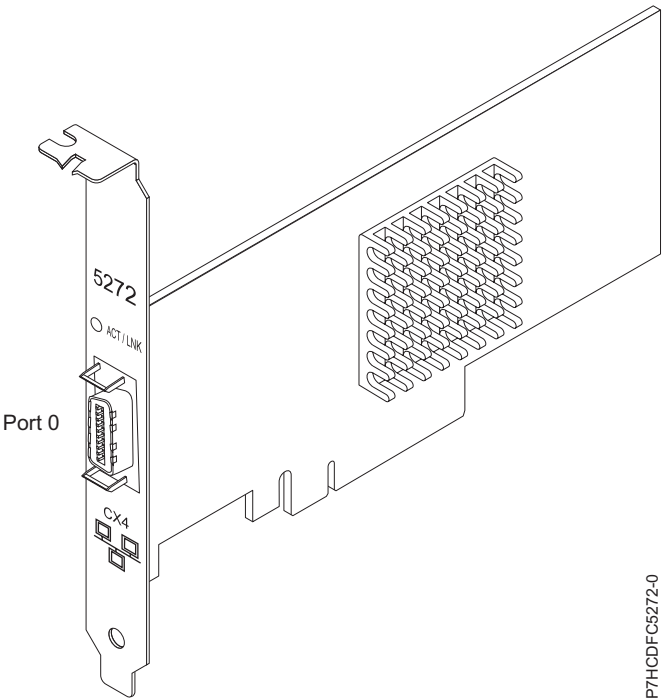
Figura 25. adaptador d'un port PCIe LP 10GbE CX4
