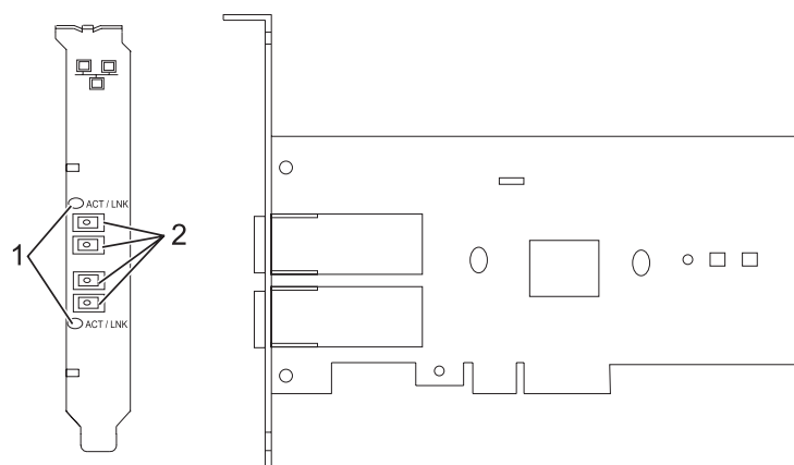
Figura 26. adaptador SX PCIe LP de 2 ports amb 1 GbE
