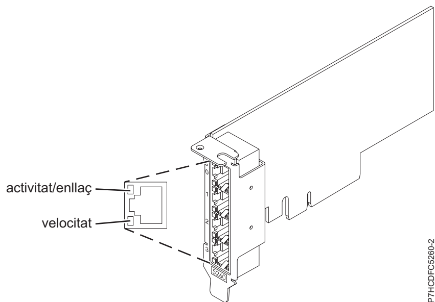
Figura 42. Adaptador
