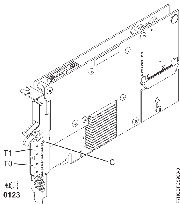
Figura 5. Adaptador SAS RAID PCIe Dual - x4 de 3 Gb
