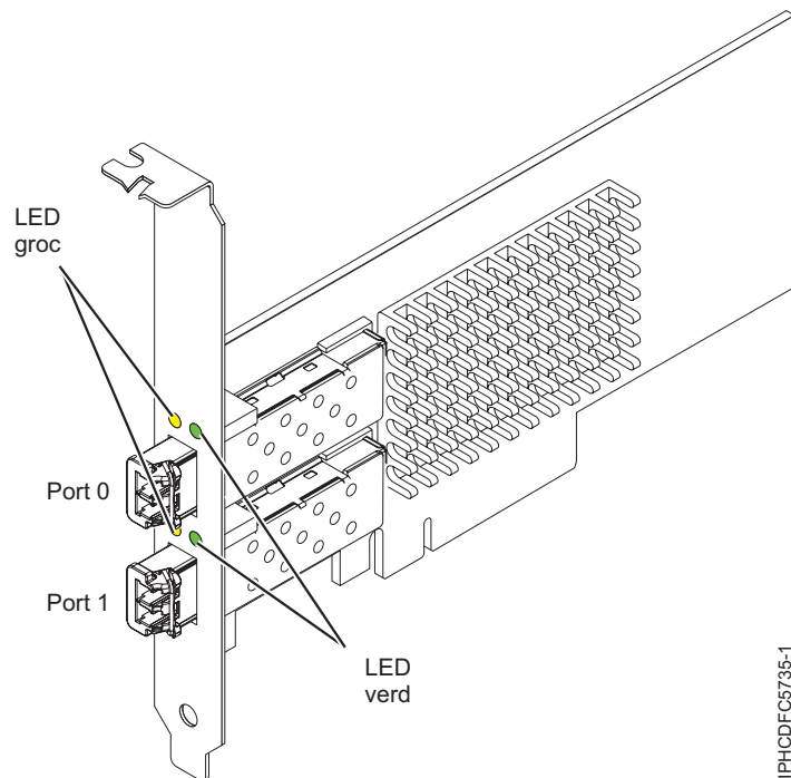
Figura 15. Adaptador EN0B
