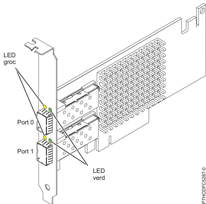
Figura 32. Adaptador SR PCIe2 LP de 2 ports i 10GbE
