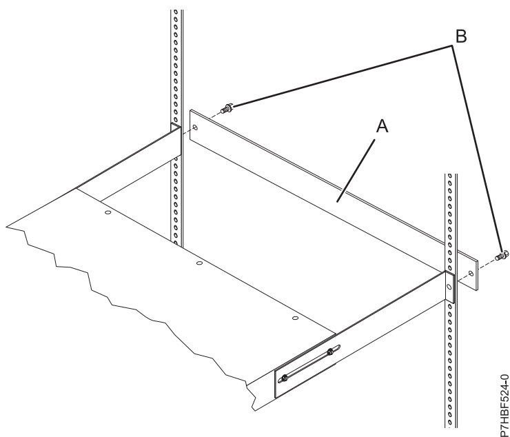
Figura 45. Fixar les peces de subjecció i el panell de reblliment al bastidor
