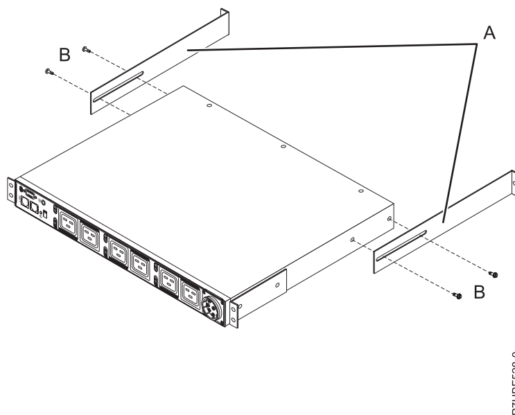
Figura 43. Fixar les peces de subjecció de muntatge llargues
