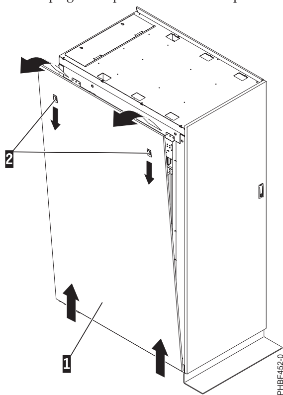
Figura 19. Extracció del panell lateral
