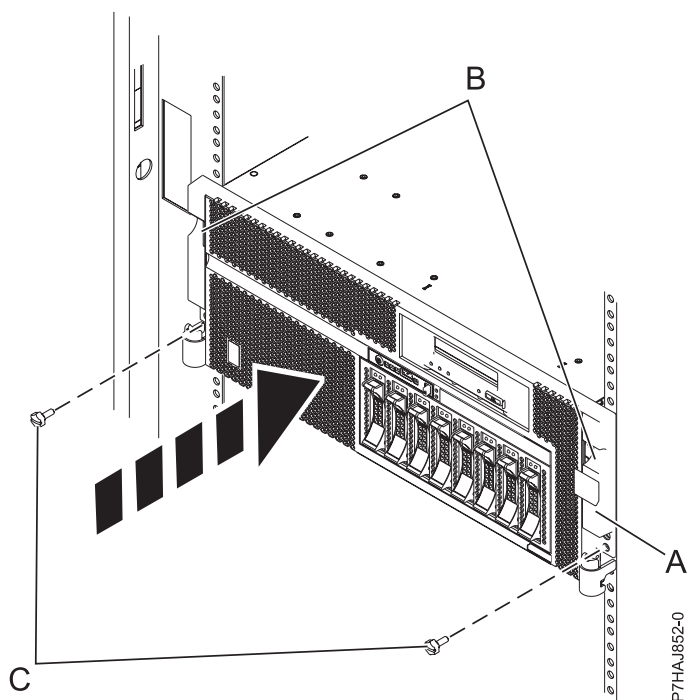
Figura 13. Reco·locació dels cargols de mà
