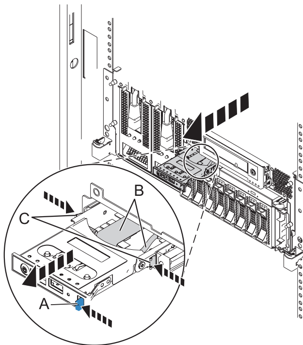
Figura 1. Extracció d'un tauler de control d'un sistema muntat en bastidor
