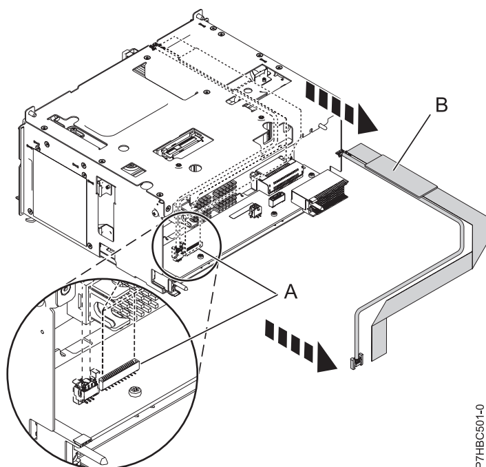
Figura 4. Extracció d'un cable de senyal en un sistema muntat en bastidor
