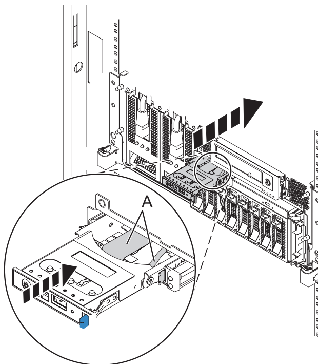
Figura 2. Substitució d'un tauler de control en un sistema muntat en bastidor
