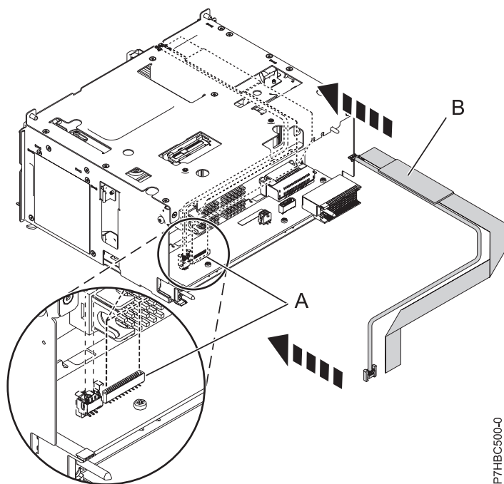
Figura 5. Instal·lació d'un cable de senyal en un sistema muntat en bastidor
