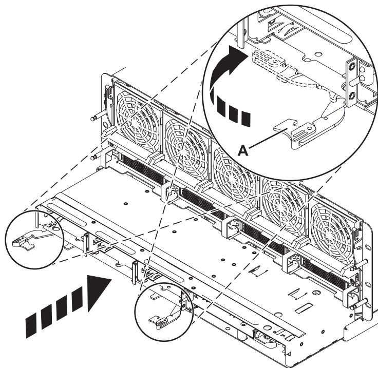
Figura 3. Instal·lació de la placa posterior de la unitat de disc
