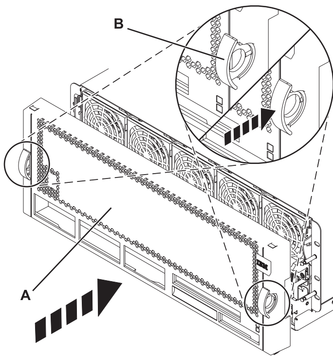
Figura 14. Instal·lació de la coberta frontal
