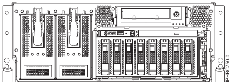
Figura 1. Placa posterior de la unitat de disc
