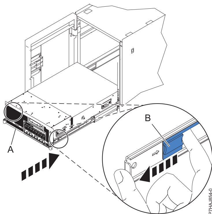
Figura 25. Alliberament dels pestells de seguretat de les guies
