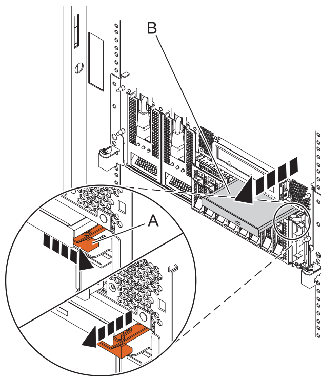
Figura 7. Extracció del dispositiu de suport d'emmagatzematge de la placa posterior de la unitat de disc
