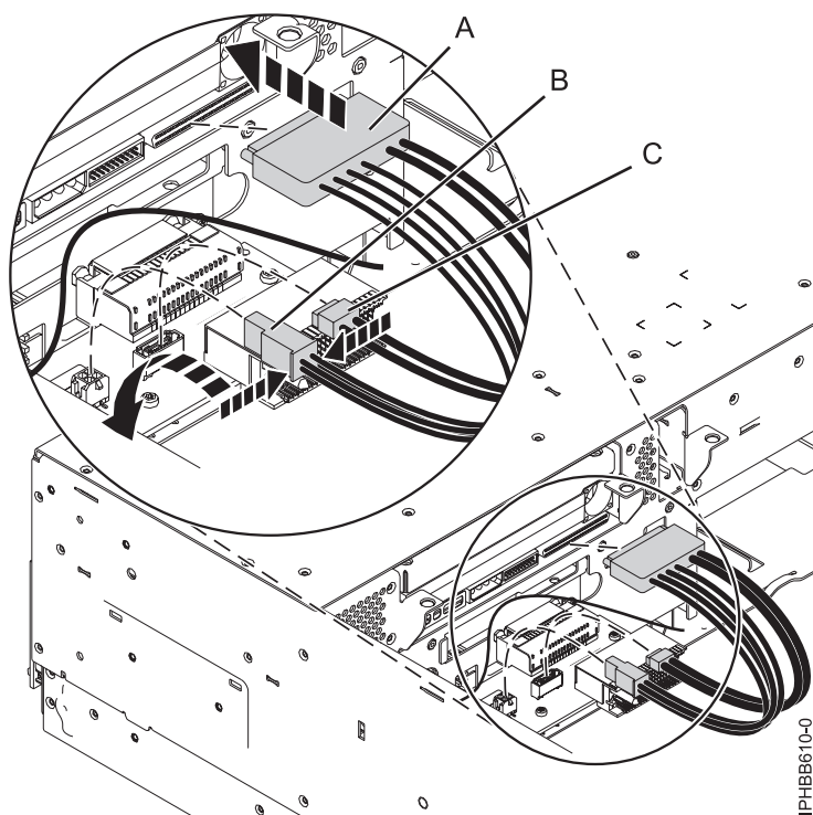
Figura 13. Connexió de cables a la placa posterior de la unitat de disc
