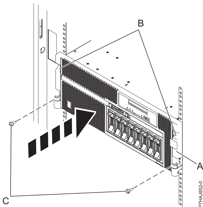
Figura 26. Substitució dels cargols de mà
