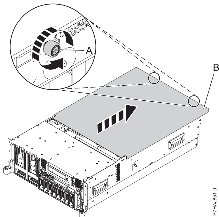
Figura 22. Extracció de la coberta d'accés de servei
