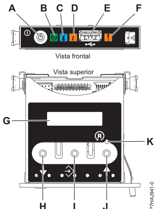
Figura 18. Tauler de control
