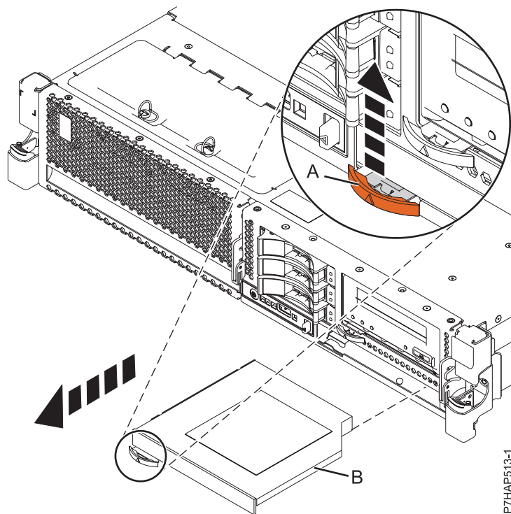
Figura 5. Extracció del dispositiu de suport d'emmagatzematge SAS de la placa posterior de la unitat de disc
