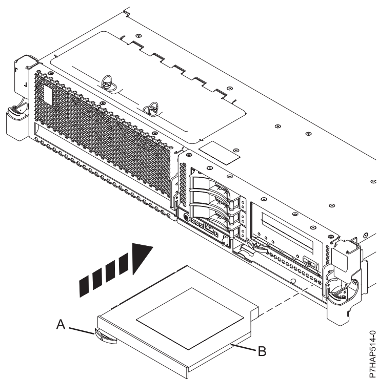
Figura 11. Instal·lació del dispositiu de suport d'emmagatzematge SAS
