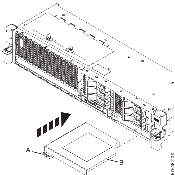
Figura 12. Instal·lació del dispositiu de suport d'emmagatzematge extraplà
