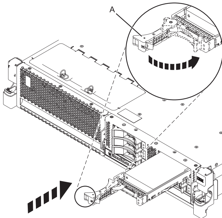
Figura 10. Instal·lació d'unitats de disc de la placa posterior
