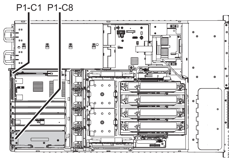
Figura 5. Ubicacions de l'adaptador GX
