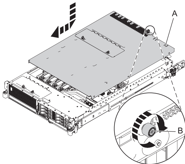
Figura 14. Instal·lació de la coberta d'accés de servei
