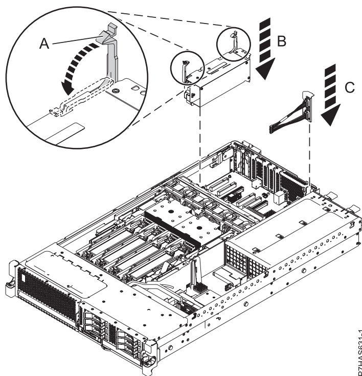
Figura 10. Substitució de l'adaptador GX FC EJ0G al sistema
