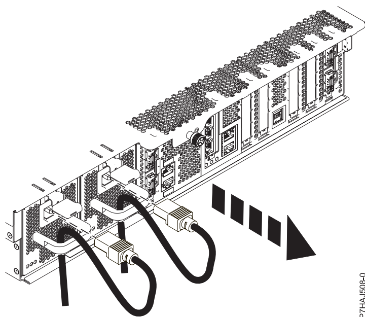
Figura 15. Extracció dels cables d'alimentació
