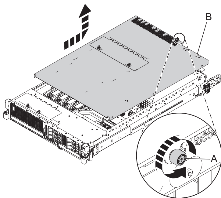
Figura 10. Extracció de la coberta d'accés de servei
