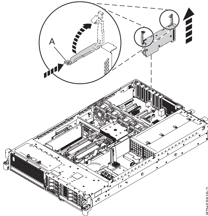
Figura 5. Extracció de l'adaptador d'un sistema
