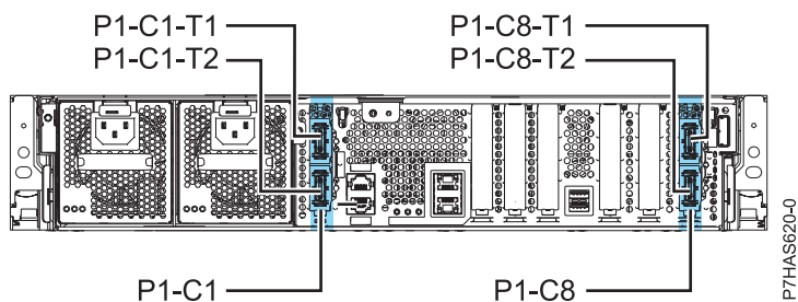
Figura 1. Ranures de l'adaptador GX i codis d'ubicació
