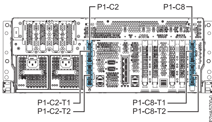
Figura 1. Vista posterior del model 8202-E4B o 8205-E6B que mostra les ranures P1-C2 i P1-C de l'adaptador GX++
