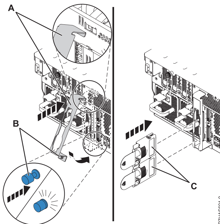
Figura 5. Instal·lació de la peça de retenció del cable
