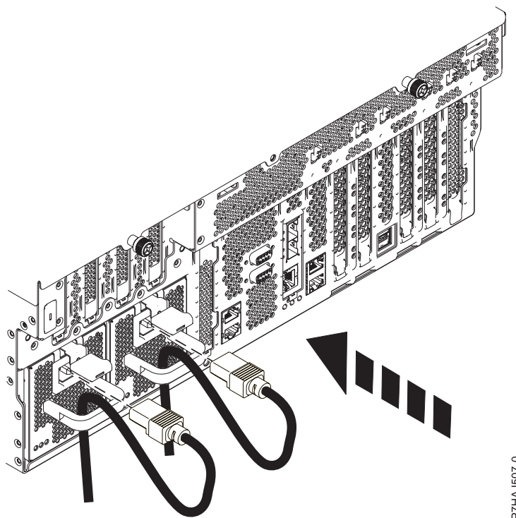
Figura 28. Connexió dels cables d'alimentació
