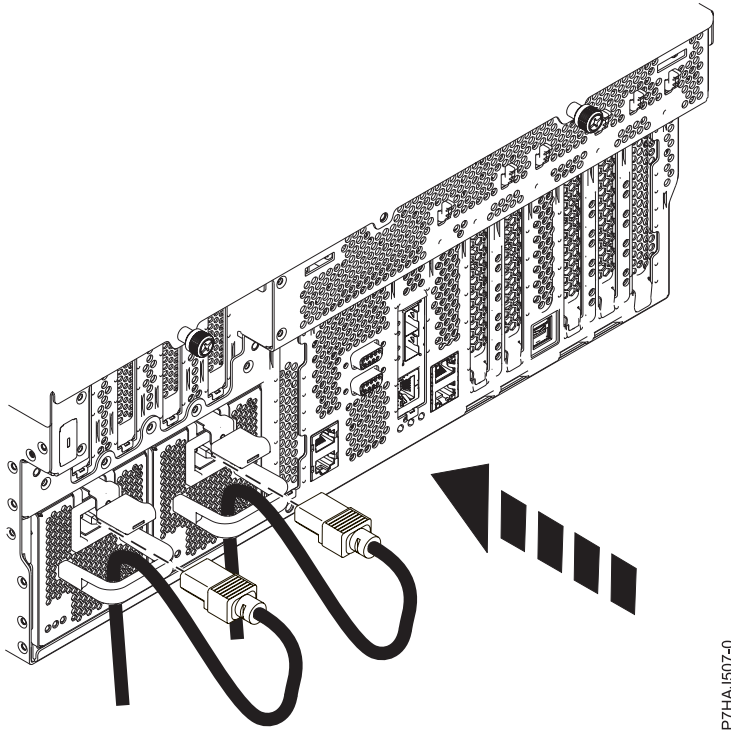
Figura 39. Connexió dels cables d'alimentació
