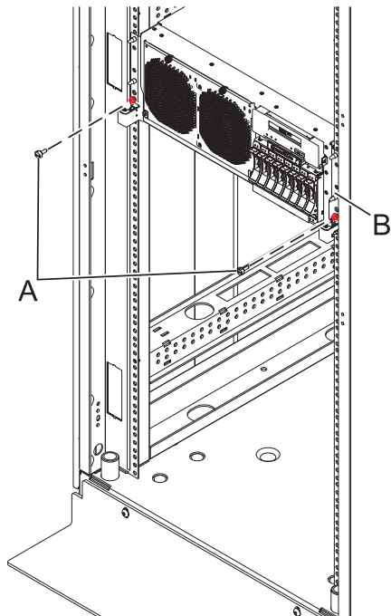
Figura 36. Col·locació de la unitat del sistema en posició operativa
