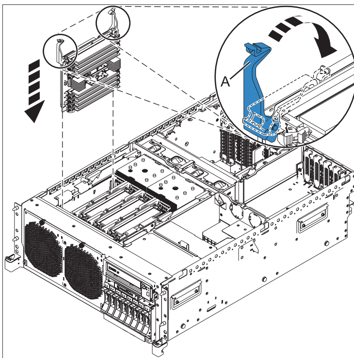
Figura 6. Substitució d'un elevador de memòria
