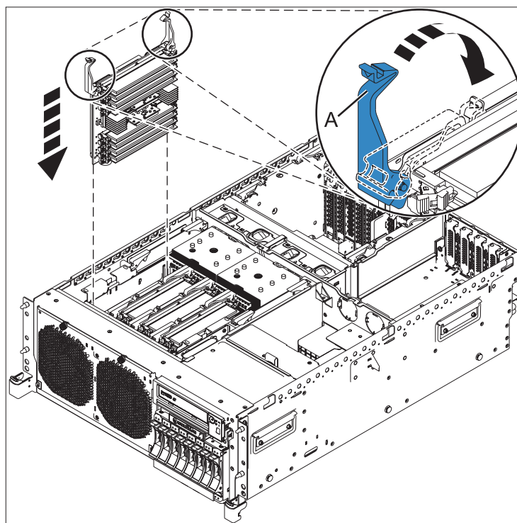
Figura 2. Instal·lació d'un elevador de memòria
