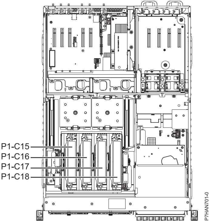
Figura 10. Seqüència de connexions dels elevadors de memòria
