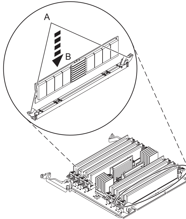
Figura 18. Substitució d'un mòdul de memòria
