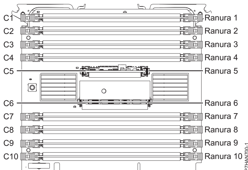
Figura 11. Ubicacions de la ranura dels mòduls de memòria per al model 8202-E4B o 8205-E6B
