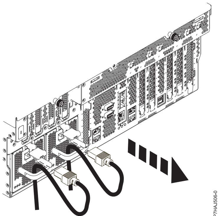
Figura 3. Desconnexió dels cables d'alimentació
