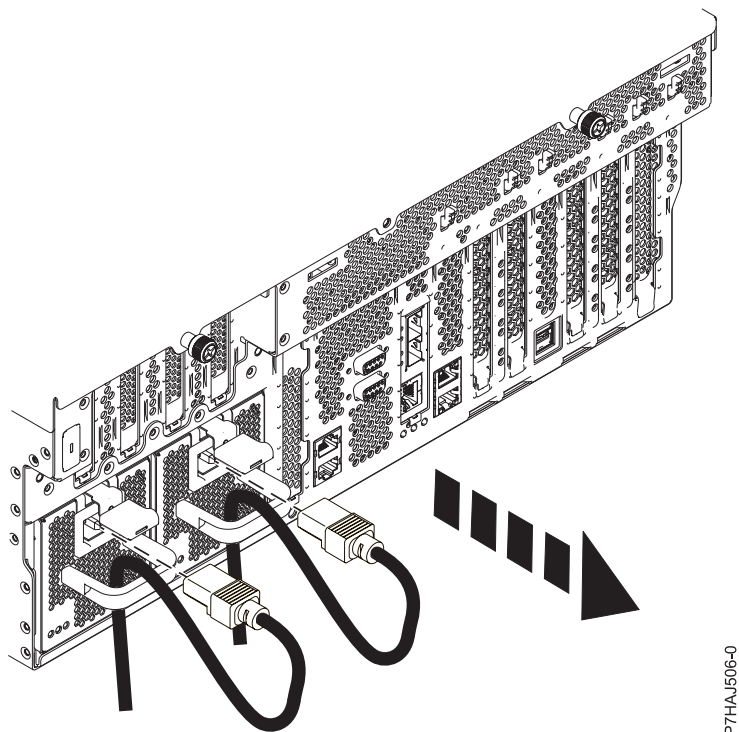
Figura 17. Desconnexió dels cables d'alimentació
