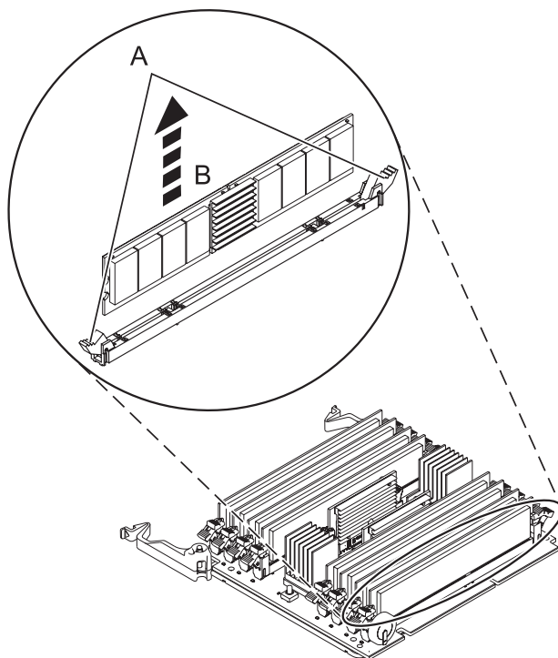
Figura 16. Extracció d'un mòdul de memòria
