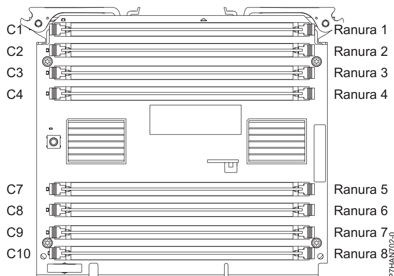
Figura 12. Ubicacions de ranures dels mòduls de memòria per al model 8202-E4C, 8202-E4D, 8205-E6C o 8205-E6D
