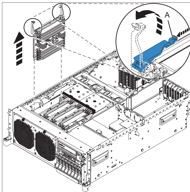
Figura 14. Extracció d'un elevador de memòria
