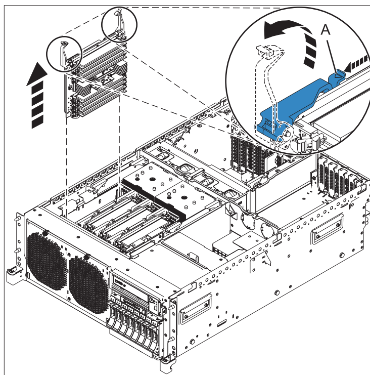
Figura 8. Extracció de l'elevador de memòria
