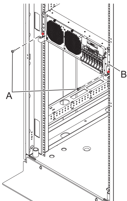
Figura 33. Col·locació de la unitat del sistema en posició de servei
