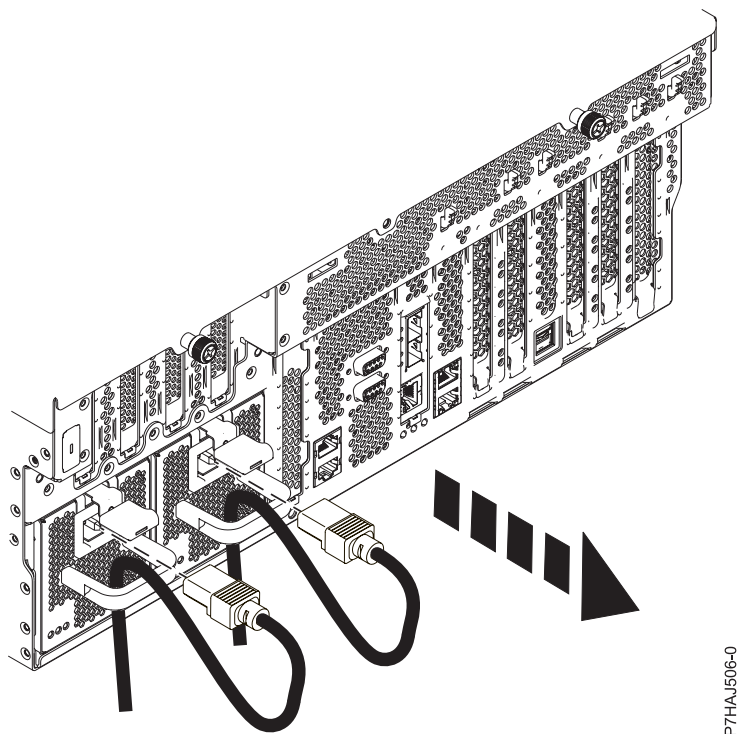
Figura 13. Desconnexió dels cables d'alimentació
