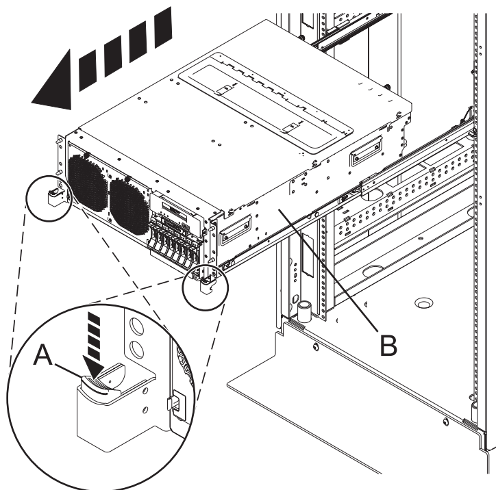
Figura 34. Bloqueig de la unitat del sistema en posició de servei
