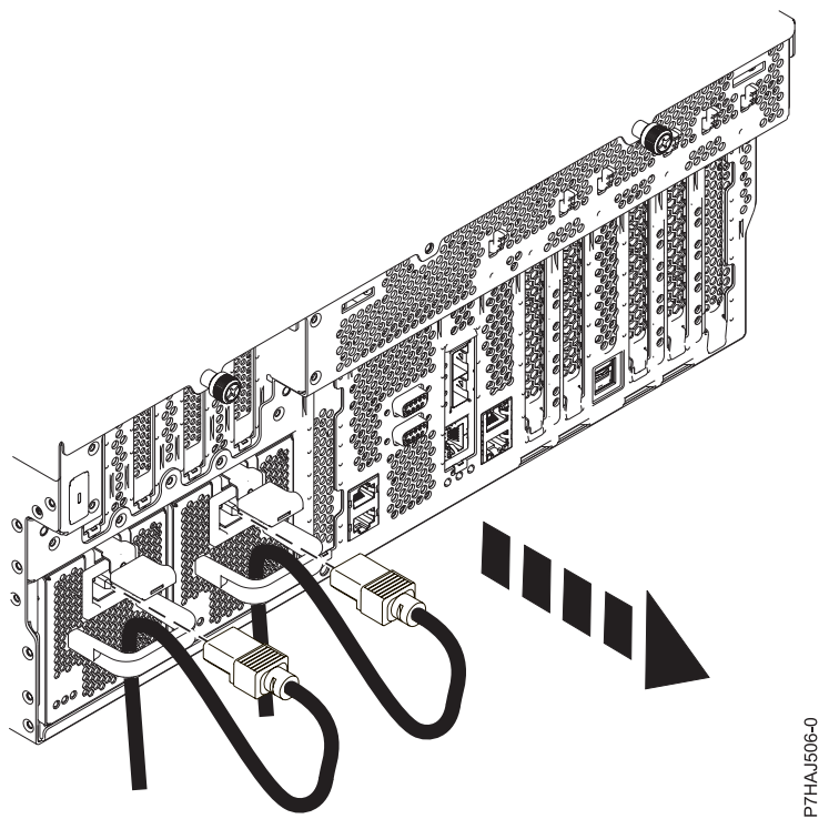
Figura 37. Extracció dels cables d'alimentació per a un sistema muntat en bastidor.
