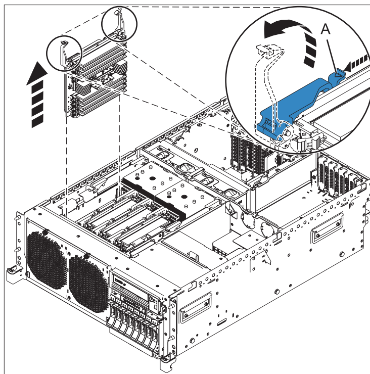
Figura 4. Extracció d'un elevador de memòria
