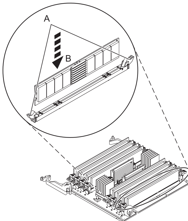
Figura 9. Substitució d'un mòdul de memòria
