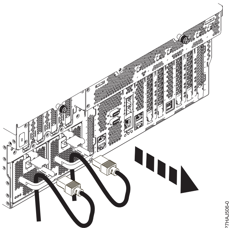
Figura 5. Desconnexió dels cables d'alimentació
