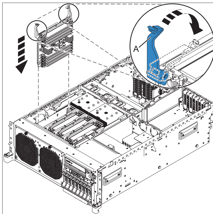
Figura 19. Substitució d'un elevador de memòria
