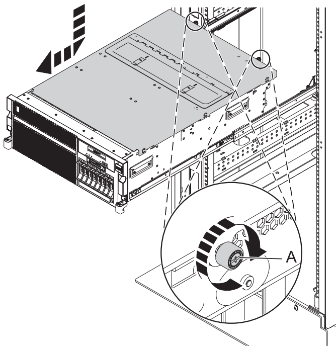
Figura 30. Instal·lació de la coberta d'accés de servei
