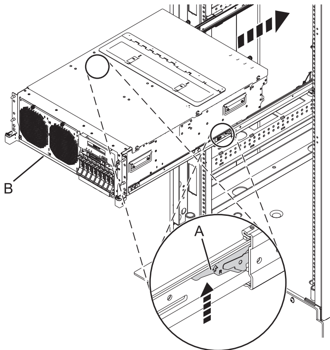
Figura 35. Col·locació de la unitat del sistema en posició operativa
