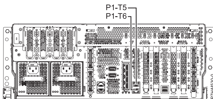
Figura 36. Ubicacions dels ports de l'HMC dels models 8202-E4B o 8205-E6B
