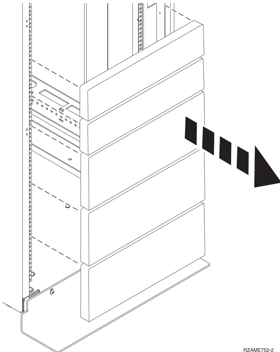
Figura 3. Extracció dels panells de rebliment.
