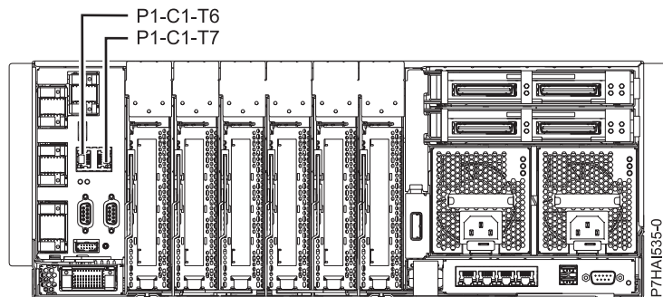
Figura 43. Ubicacions dels ports de l'HMC dels models 9117-MMC, 9117-MMD, 9179-MHC, 9179-MHD o 8412-EAD
