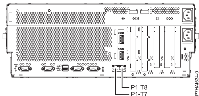
Figura 40. Ubicacions dels ports de l'HMC del models 8233-E8B o 8236-E8C
