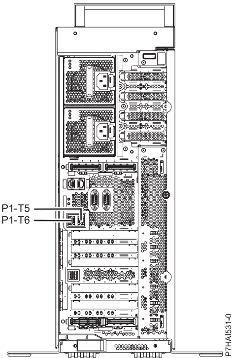
Figura 37. Ubicacions dels ports de l'HMC del models 8202-E4C o 8205-E6C
